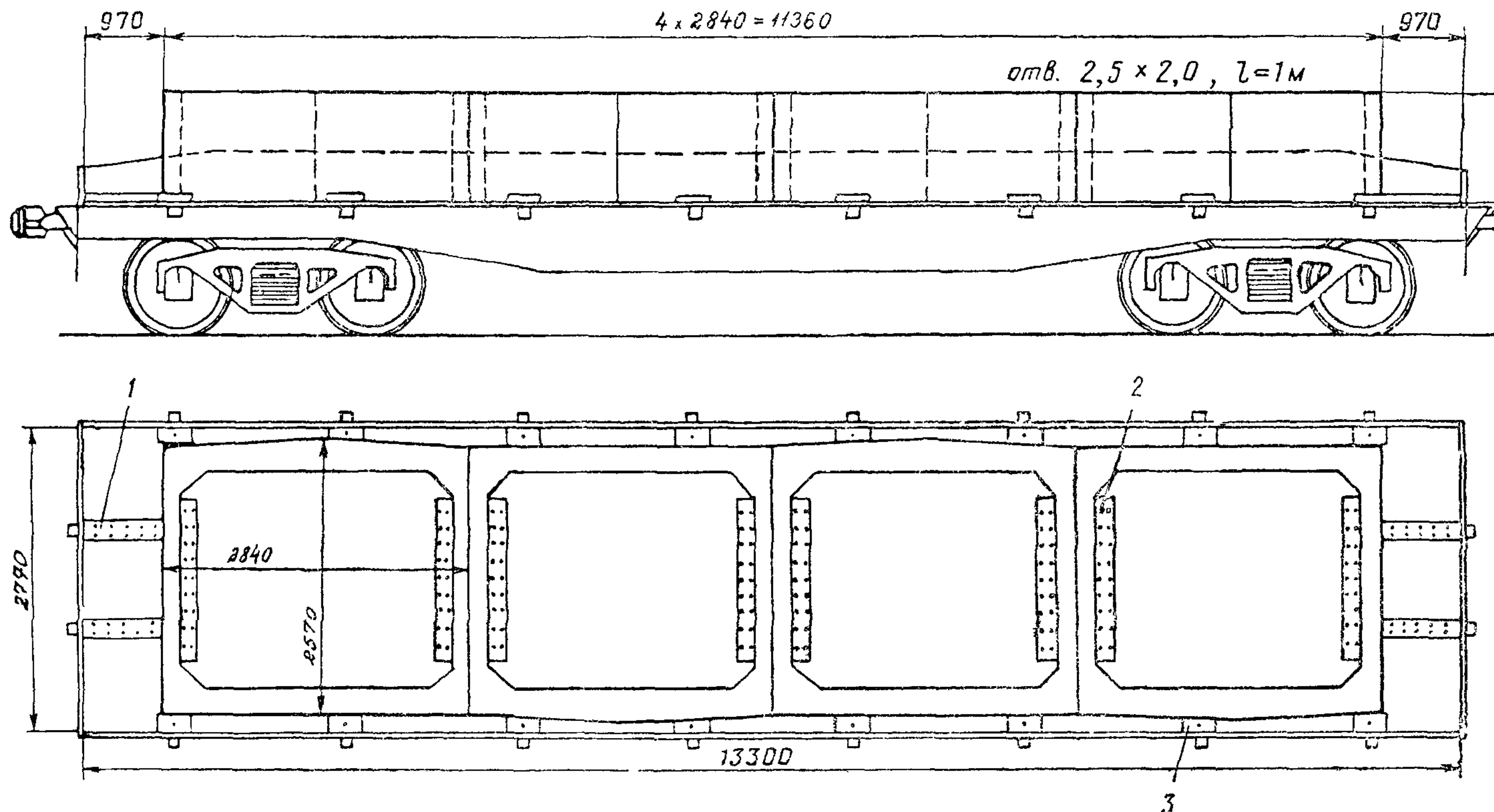
Рис. 3. Прямоугольные звенья отверстием 2,5 \times 2 м.
