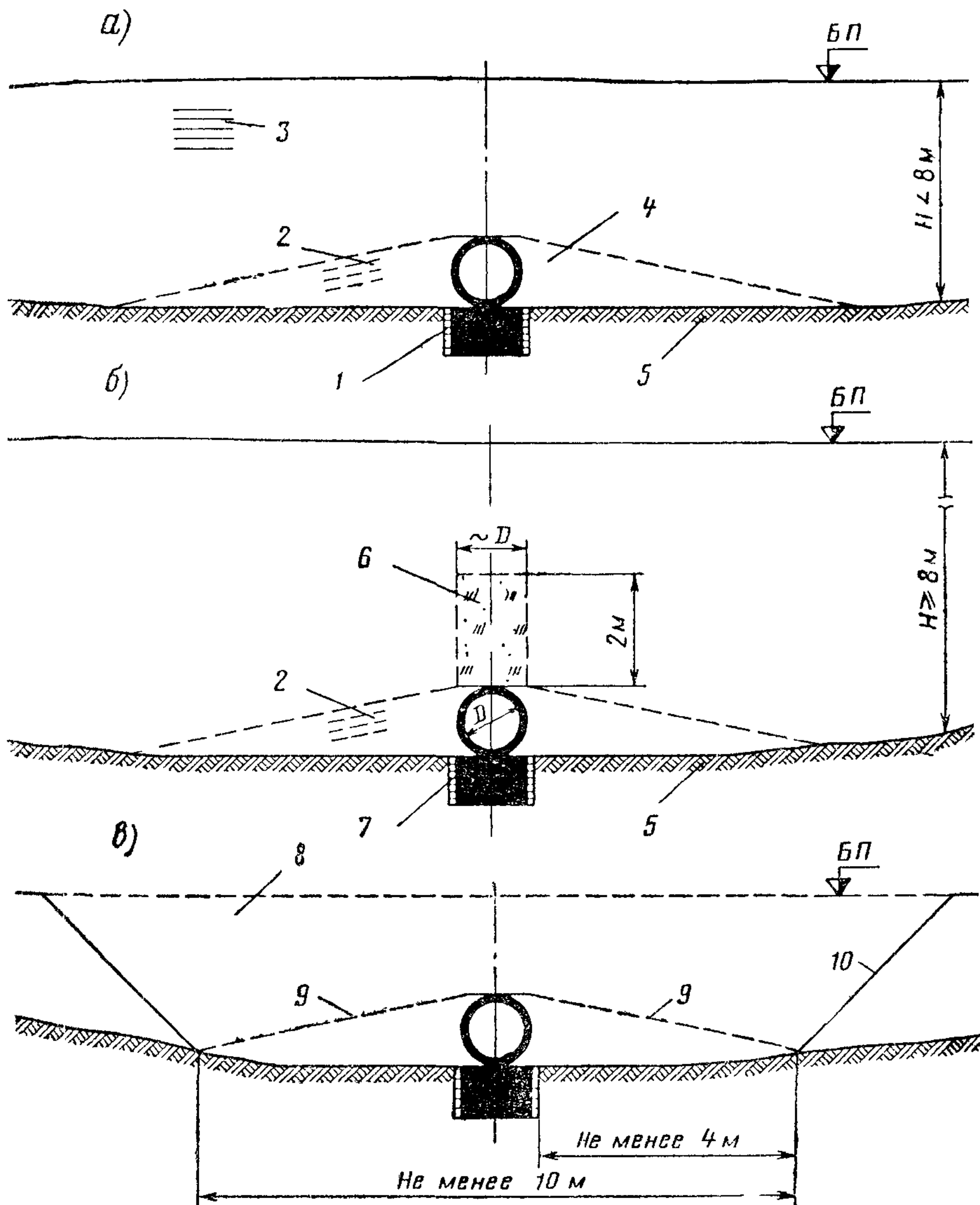
Рис. 2. Схемы возведения насыпей над трубами:
