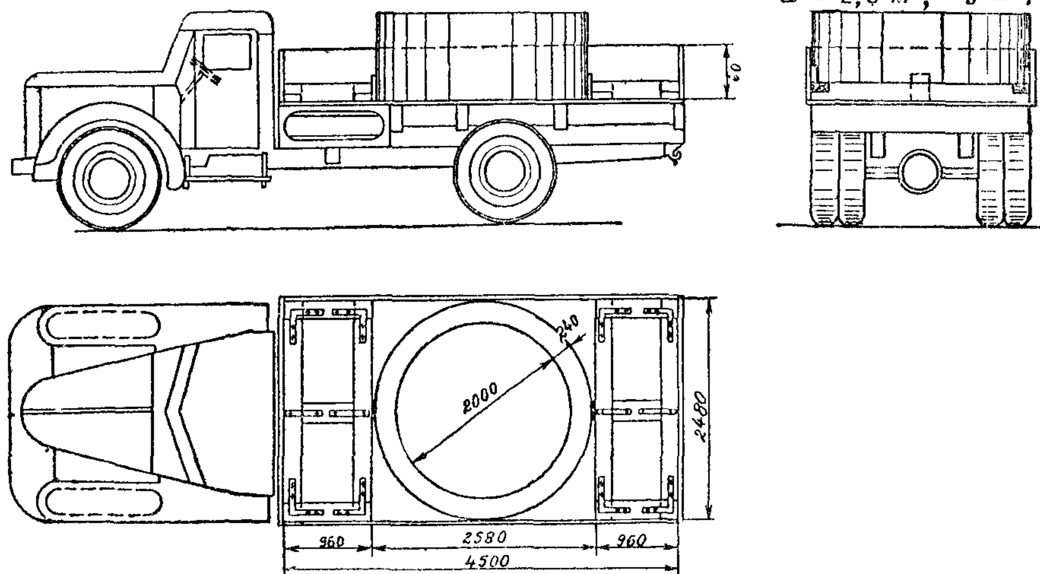
Рис. 2. Круглые звенья диаметром 2000 мм
