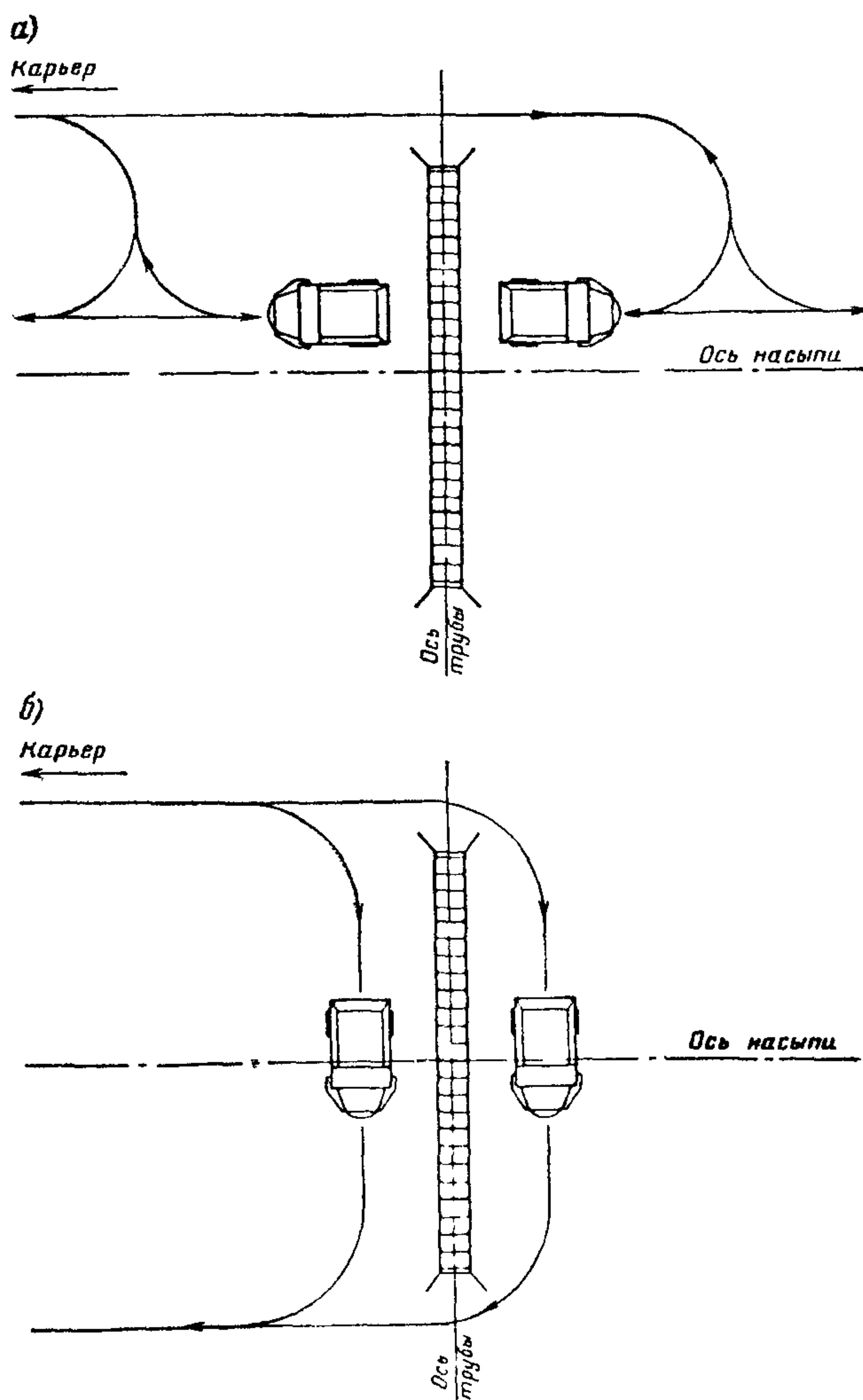
Рис. 3. Схемы движения самосвалов при засыпке труб
