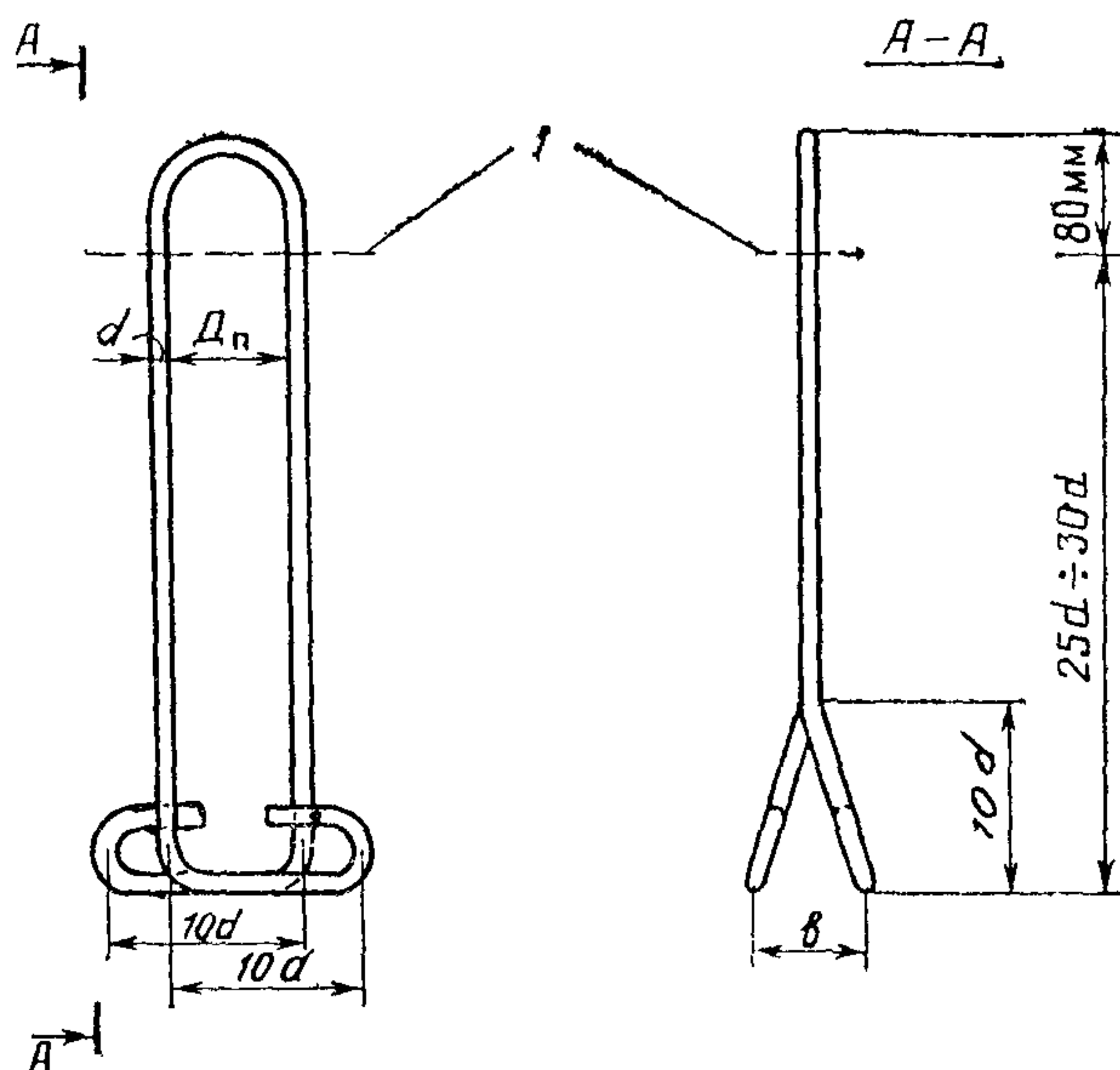
Рис. 1. Строповочная петля:
