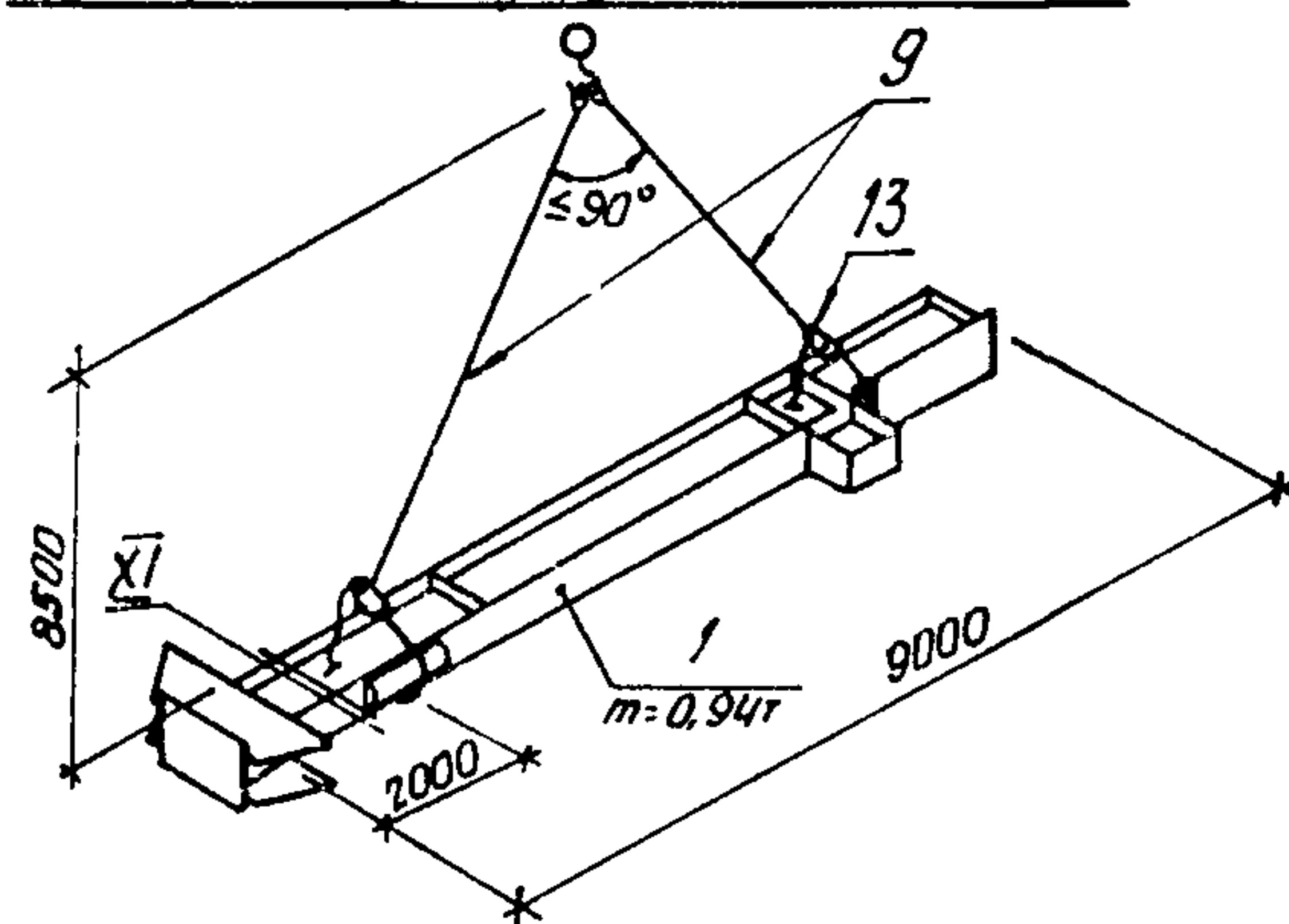
подкрановых балок
