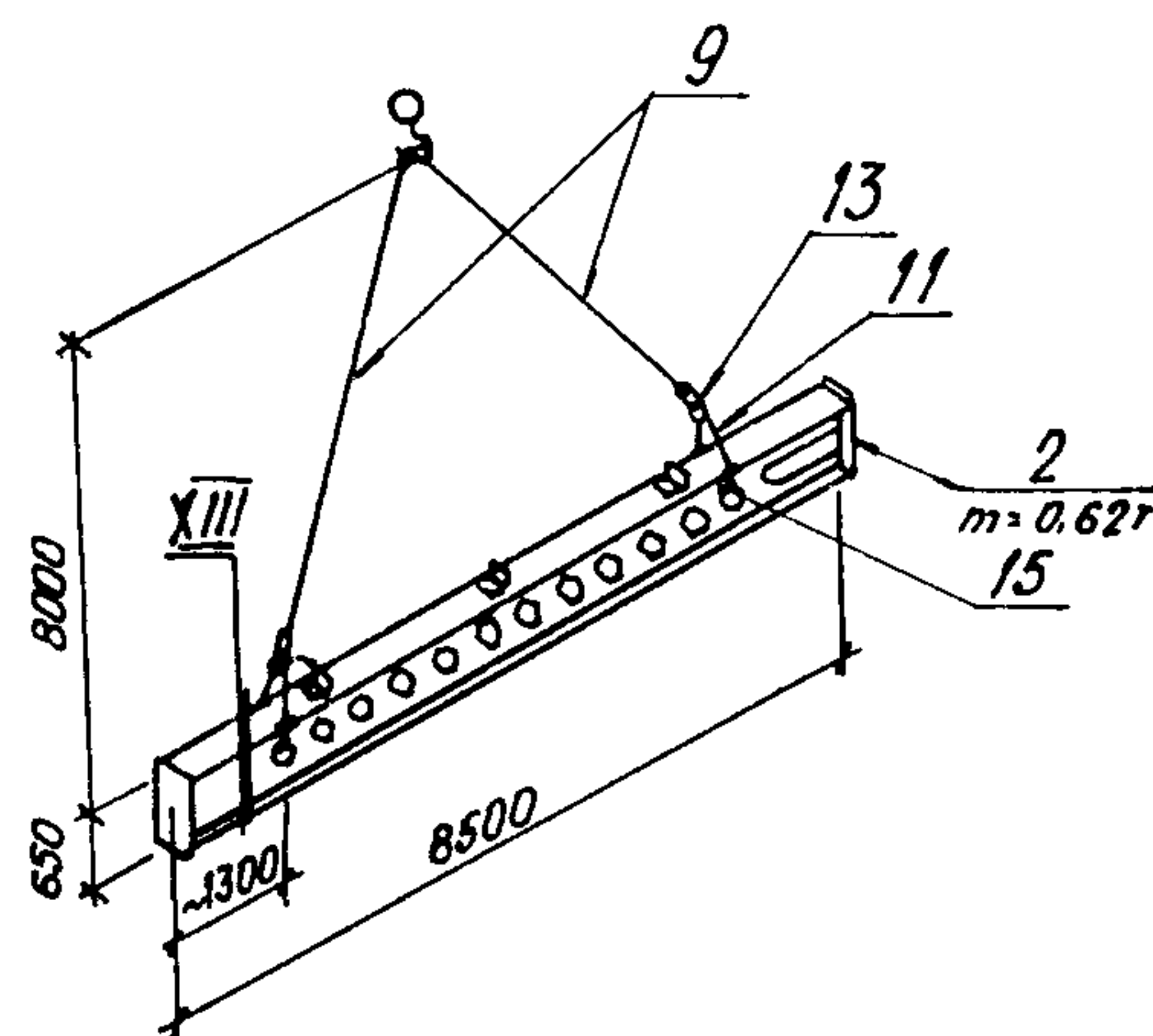
балок рамы при укрупнительной сборке
