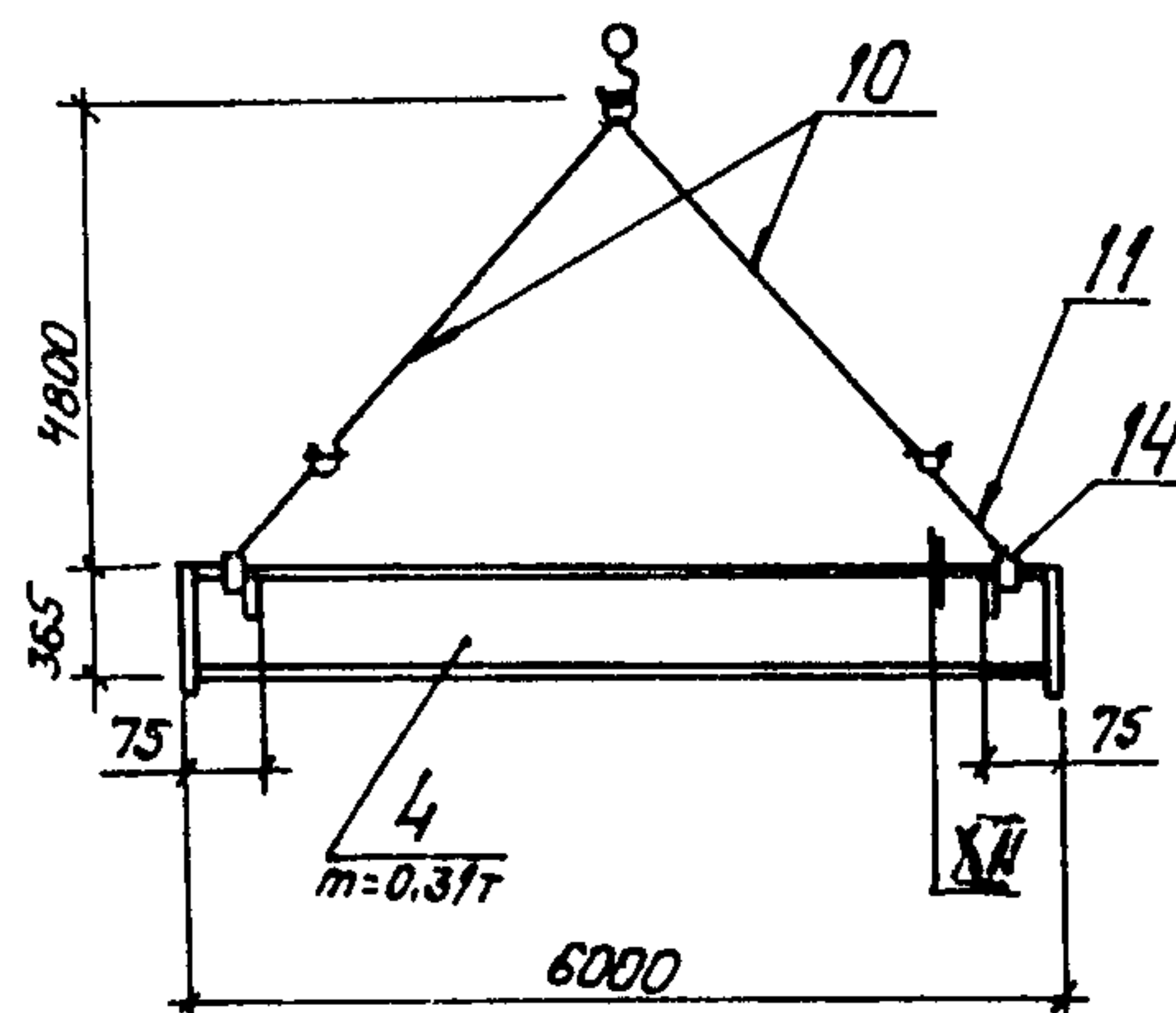
подкрановых балок
