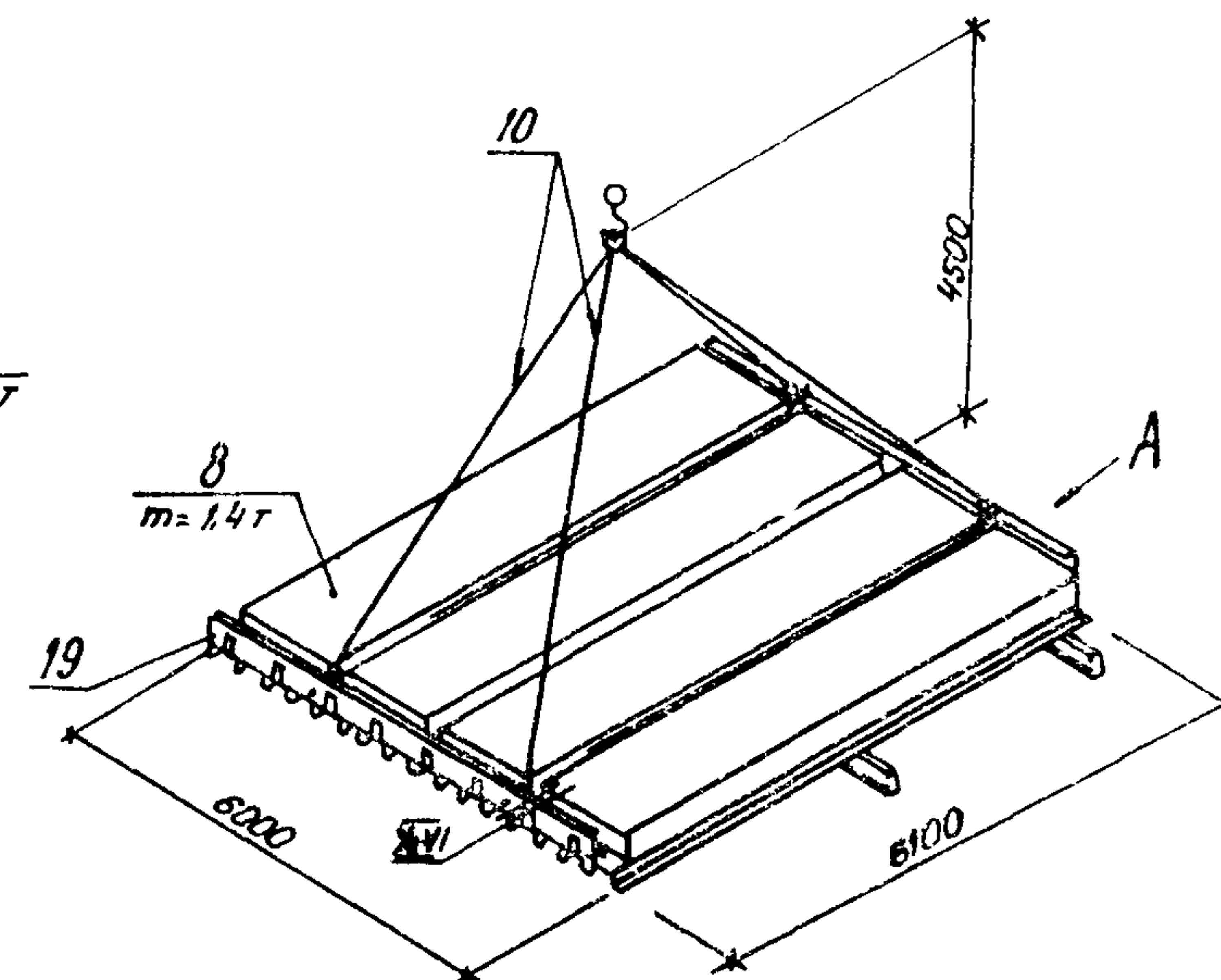
Вид по А
