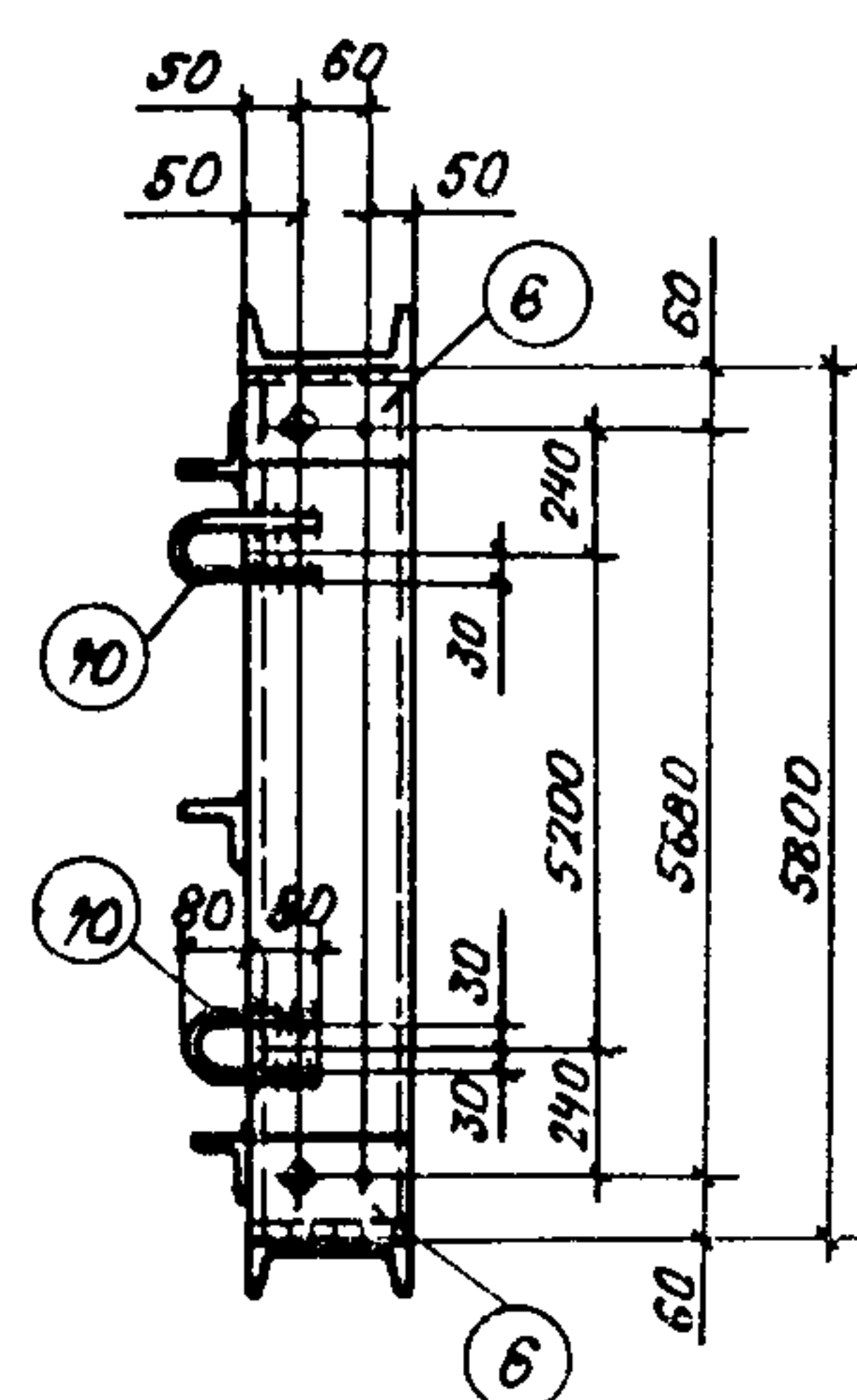
Элементы связи
