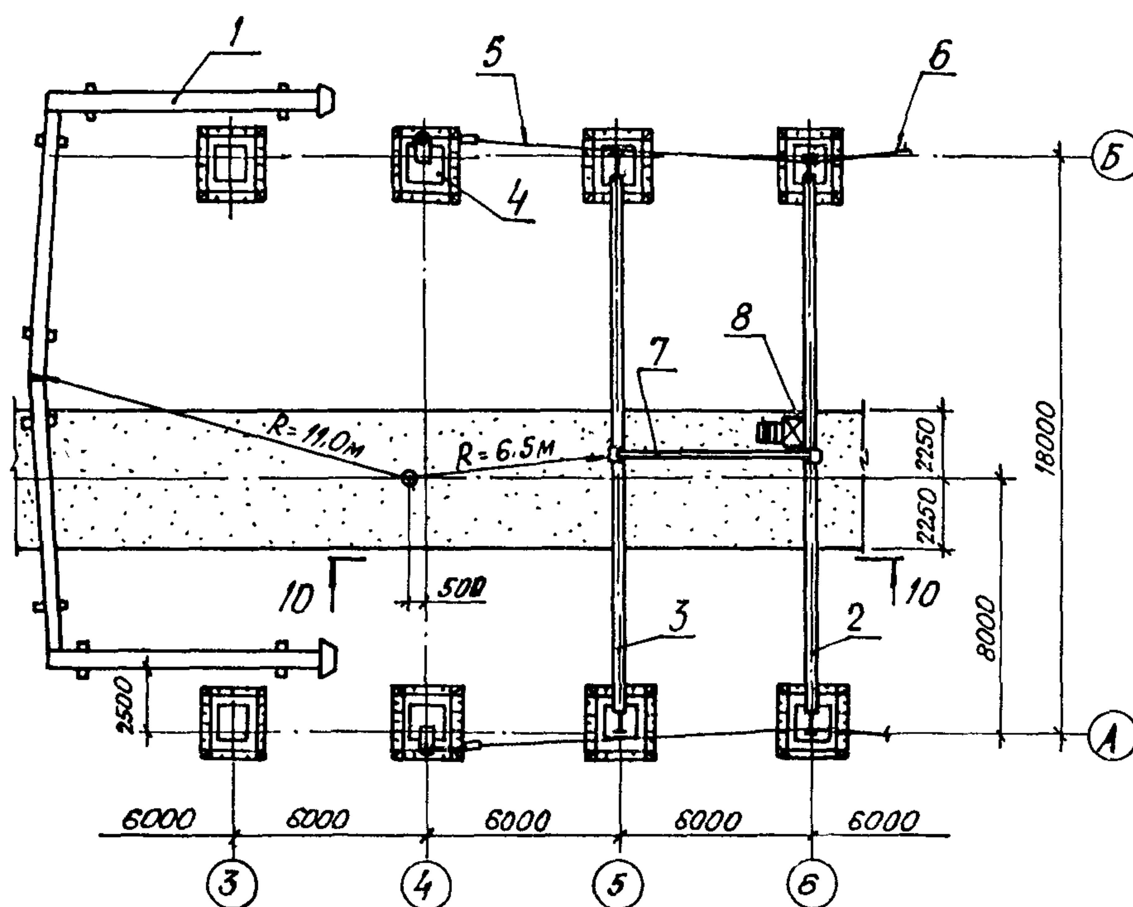
Схема монтажа рамы 2
