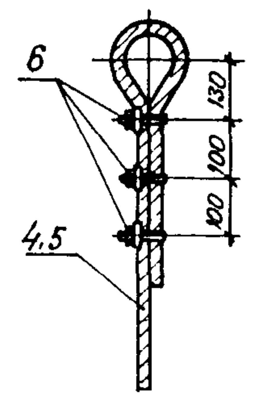
Хомут М-1
