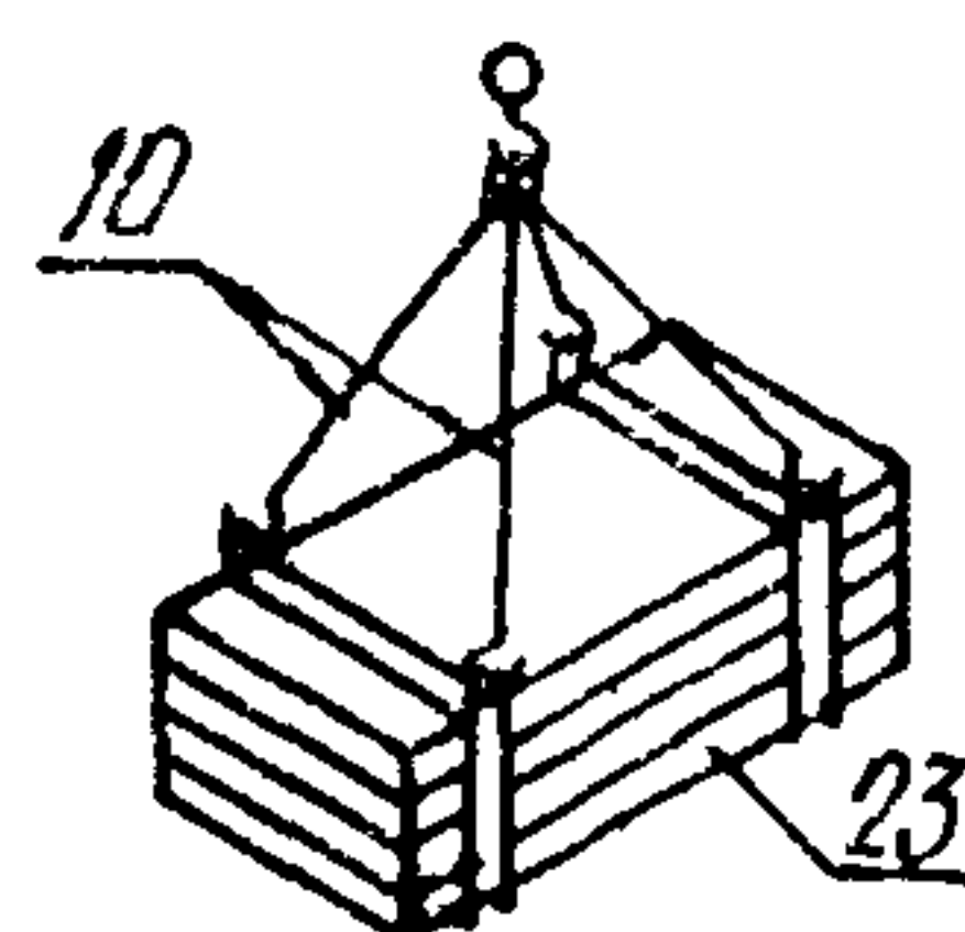
пакета панелей ПКМ-120
