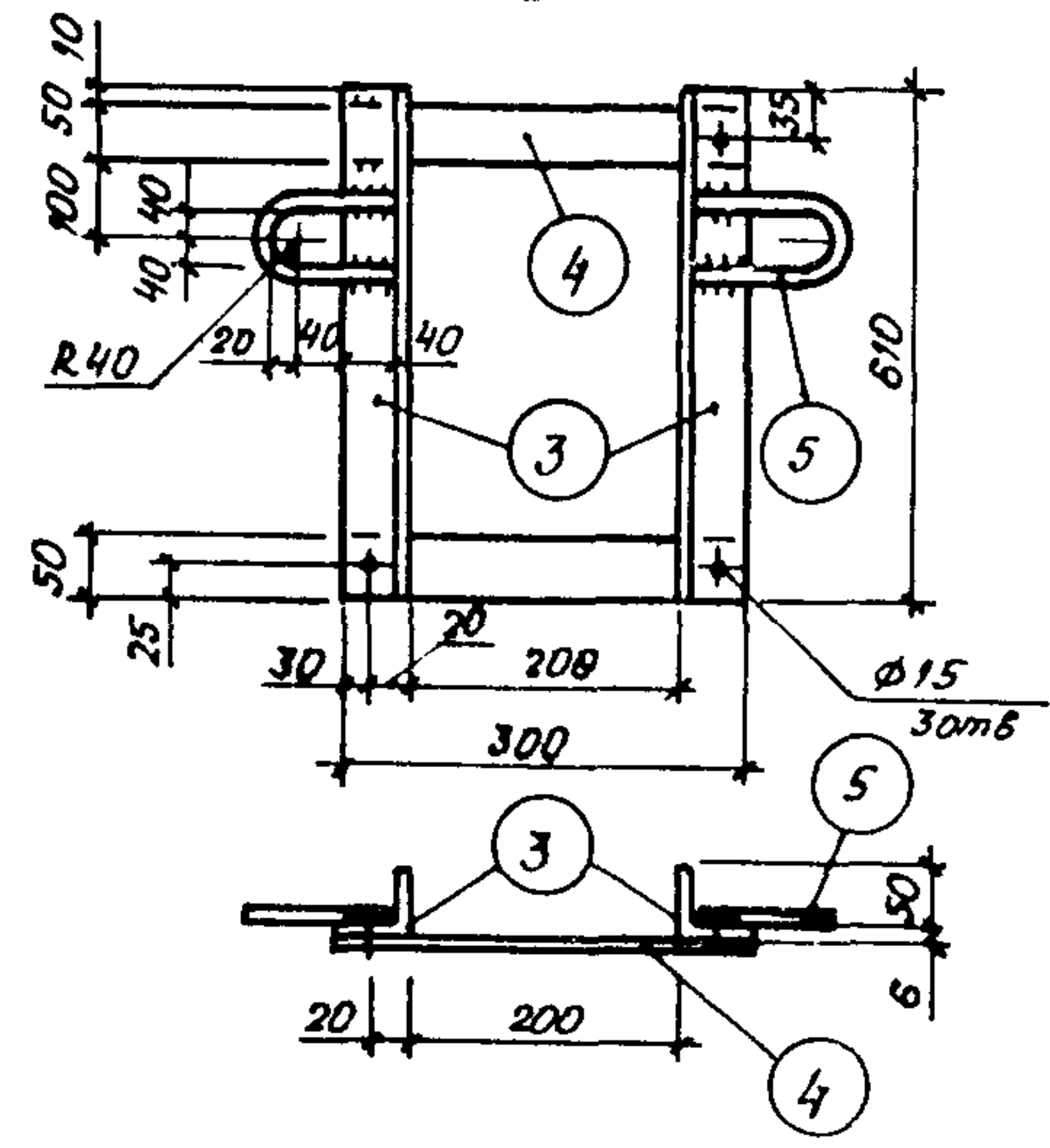
Хомут М-1
