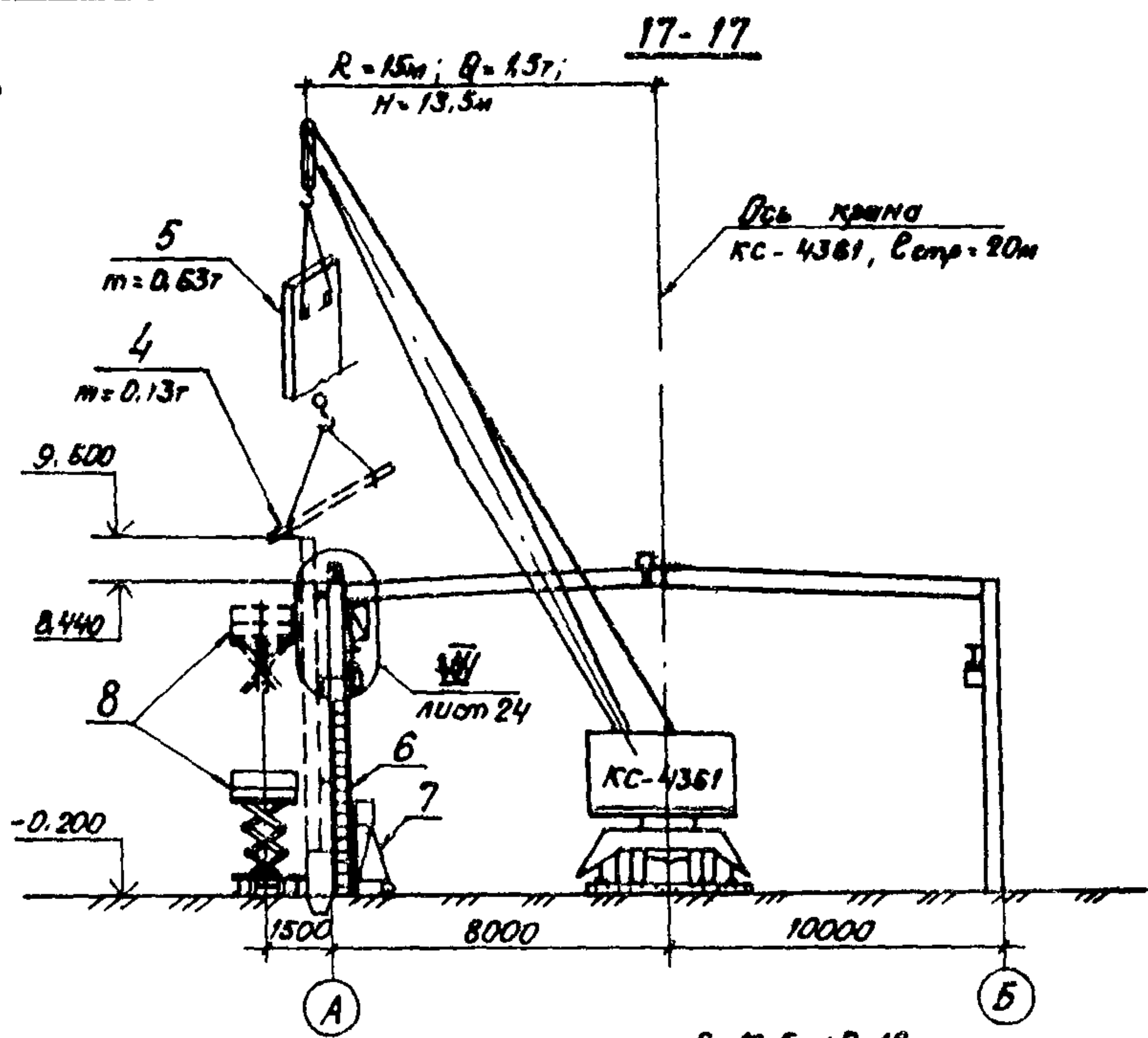
Схема монтажа элементов стенового ограждения (пролет 18м)
