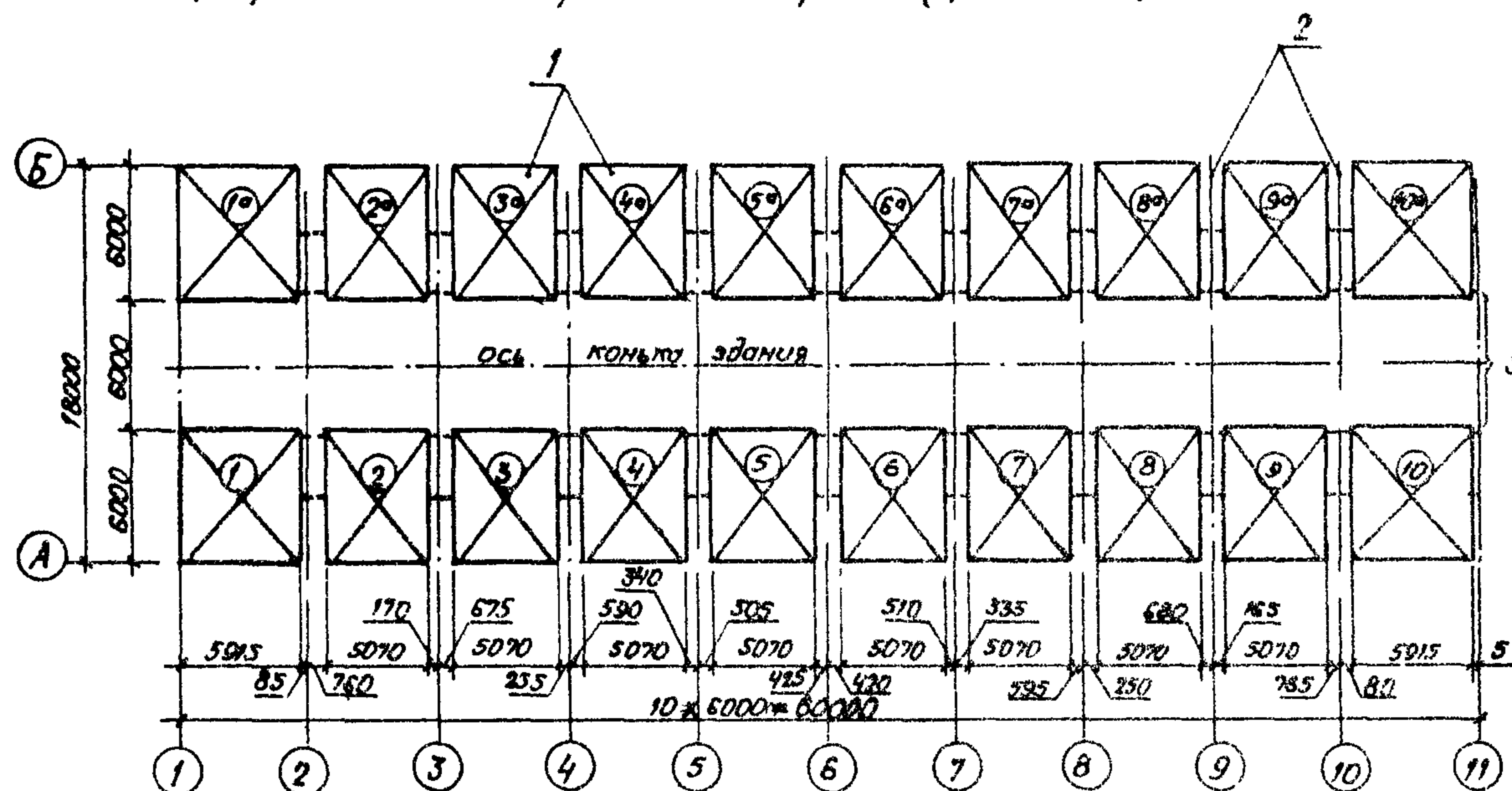
Маркировочная схема раскладки картин (пролет 18м)
