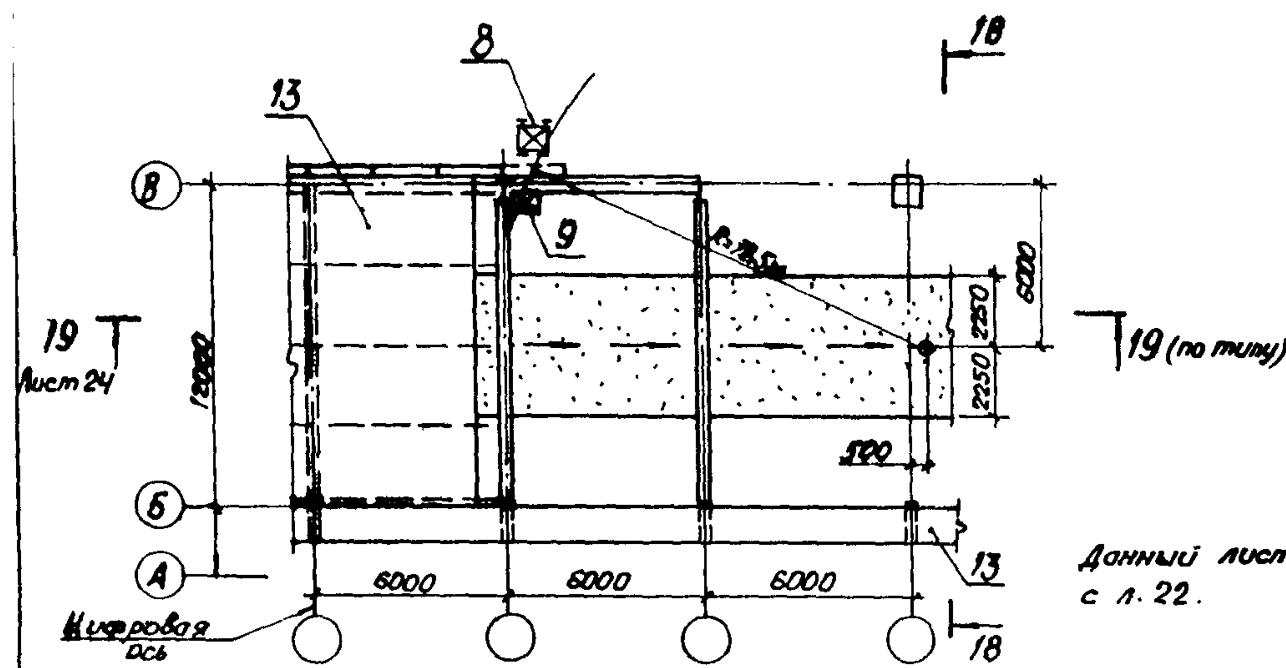
Схема монтажа элементов стенового ограждения (пролет 12м)
