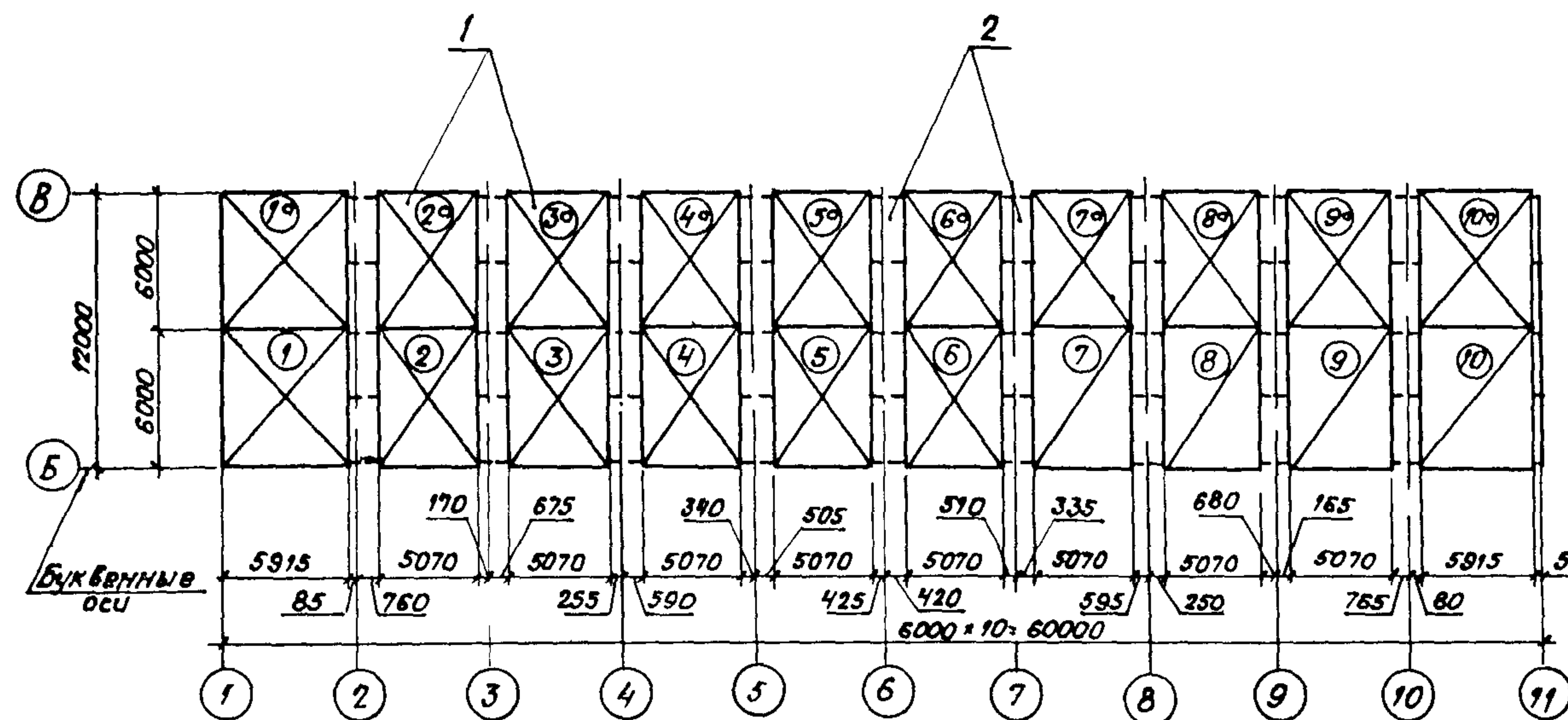
Маркировочная схема раскладки картин (пролет 12м)
