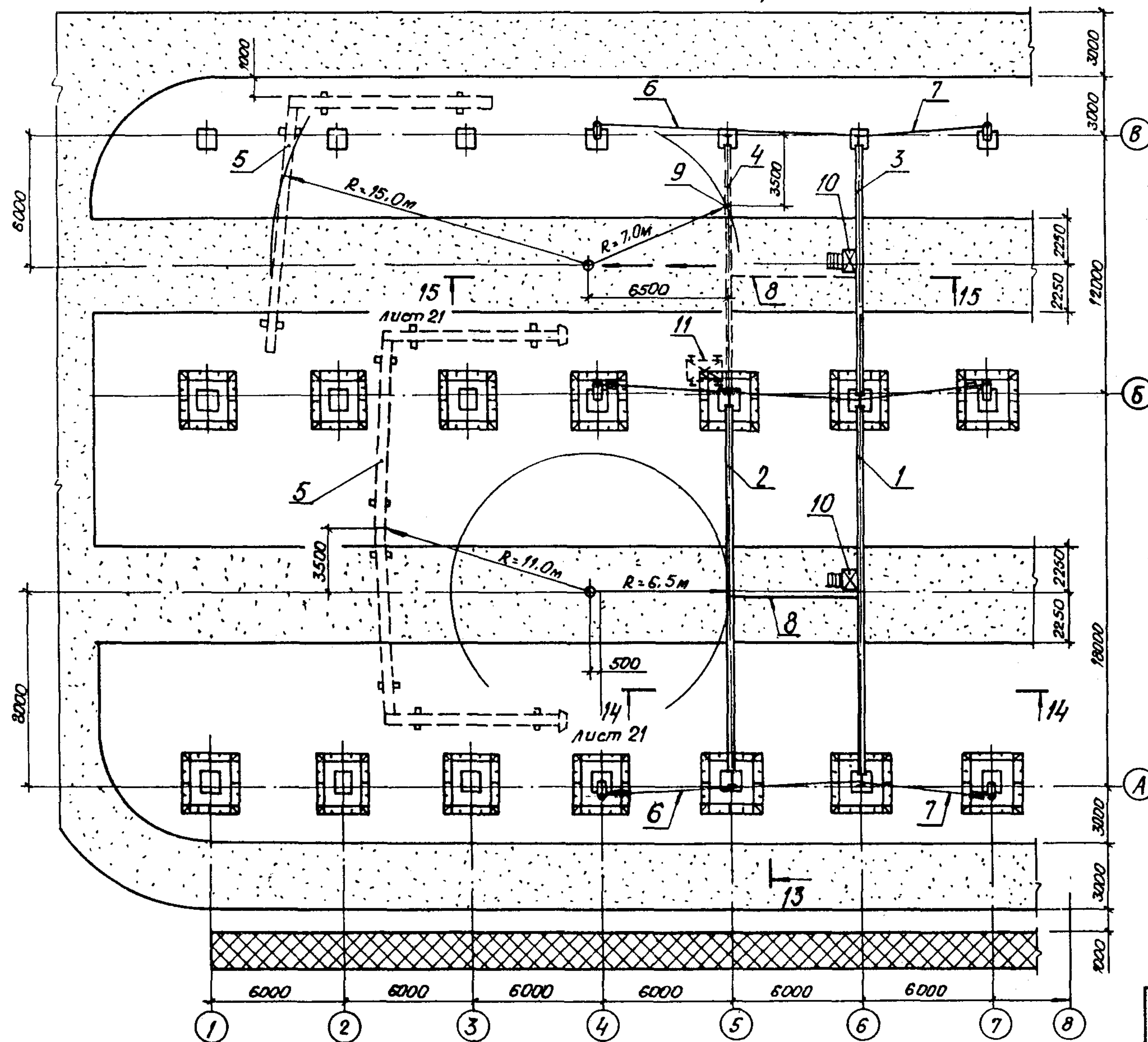
Схема монтажа второй рамы каркаса
