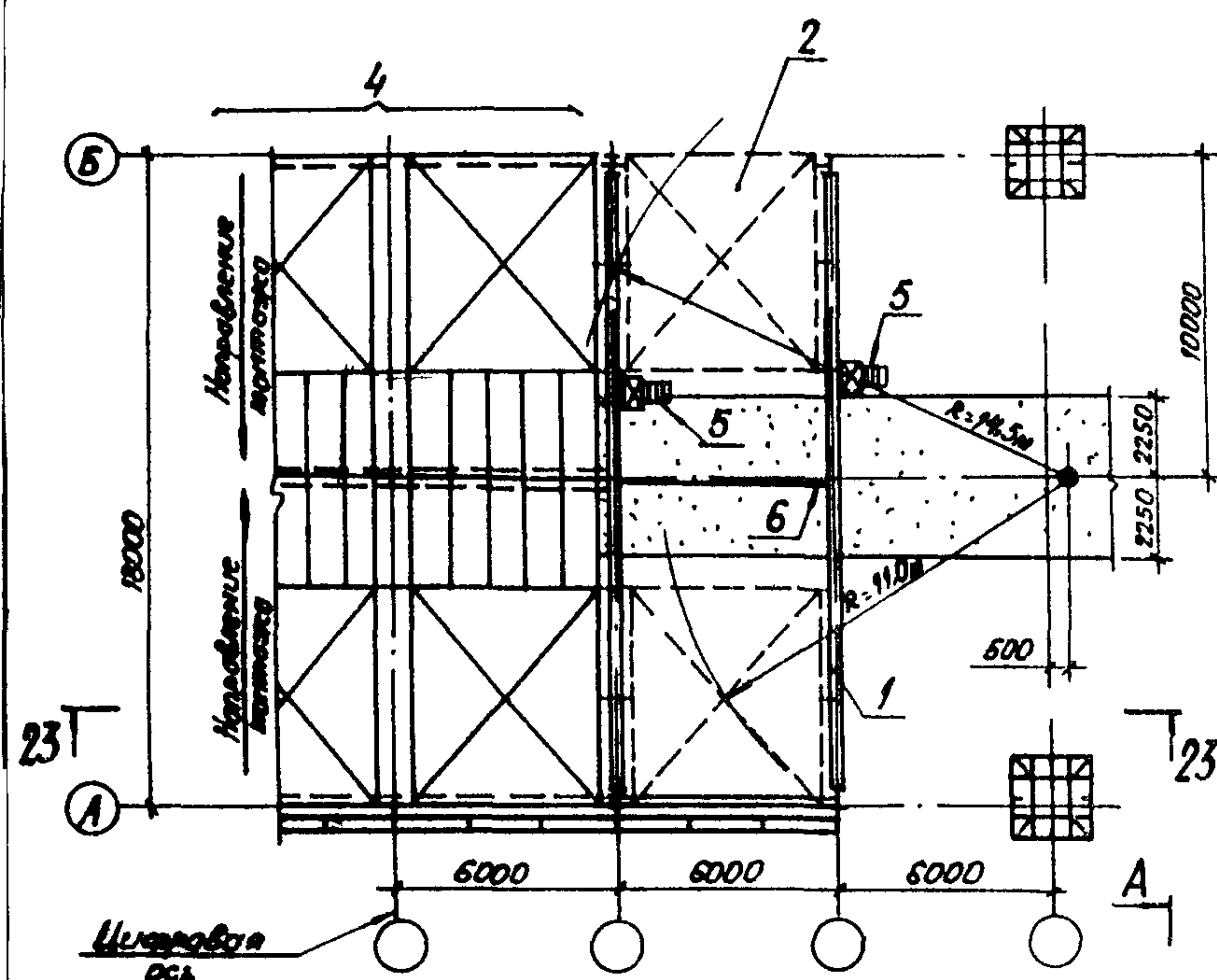
Схема монтажа покрытия ячейки (пролет 18м)
