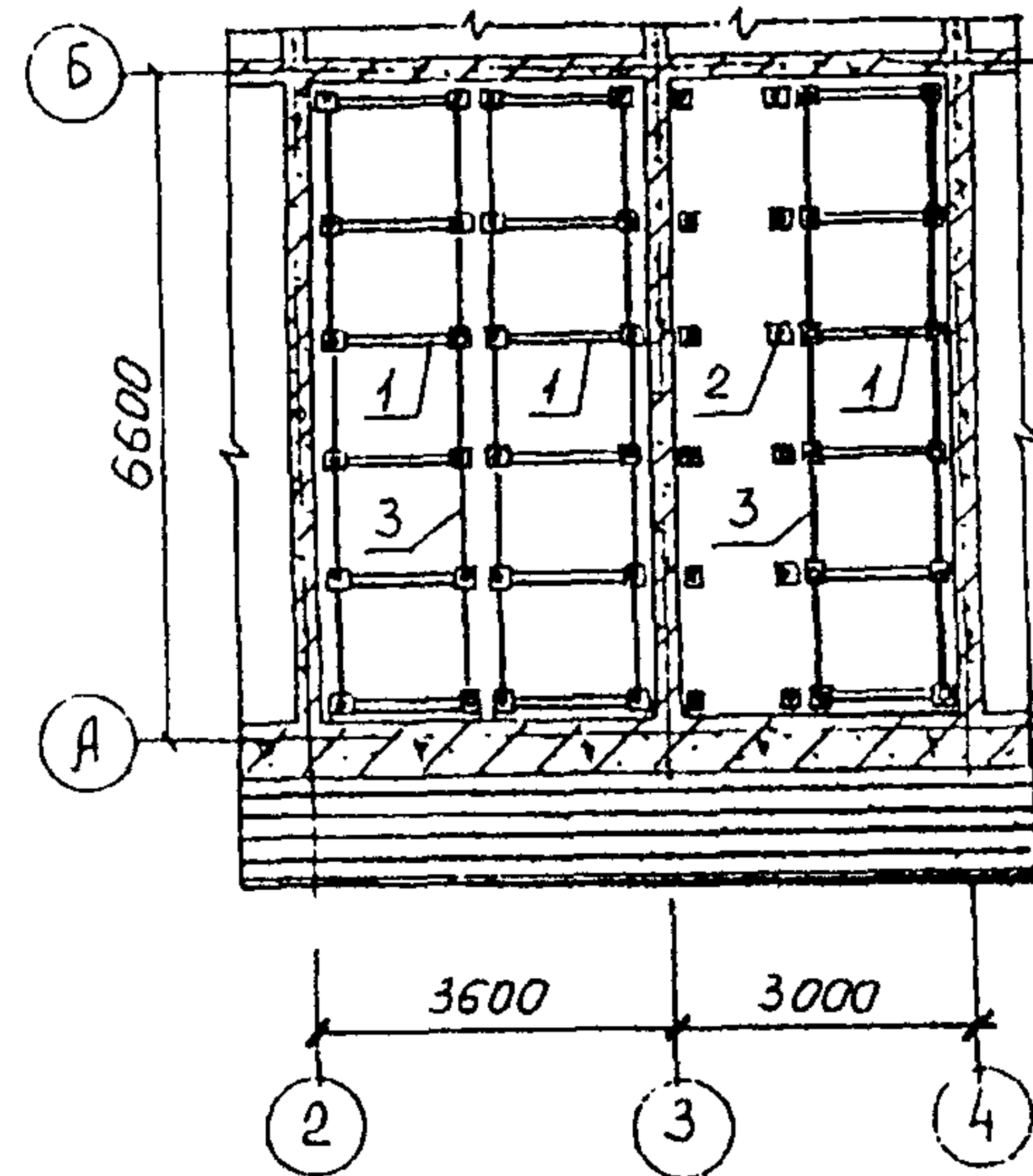
Установка рам, стоек и крестовин
