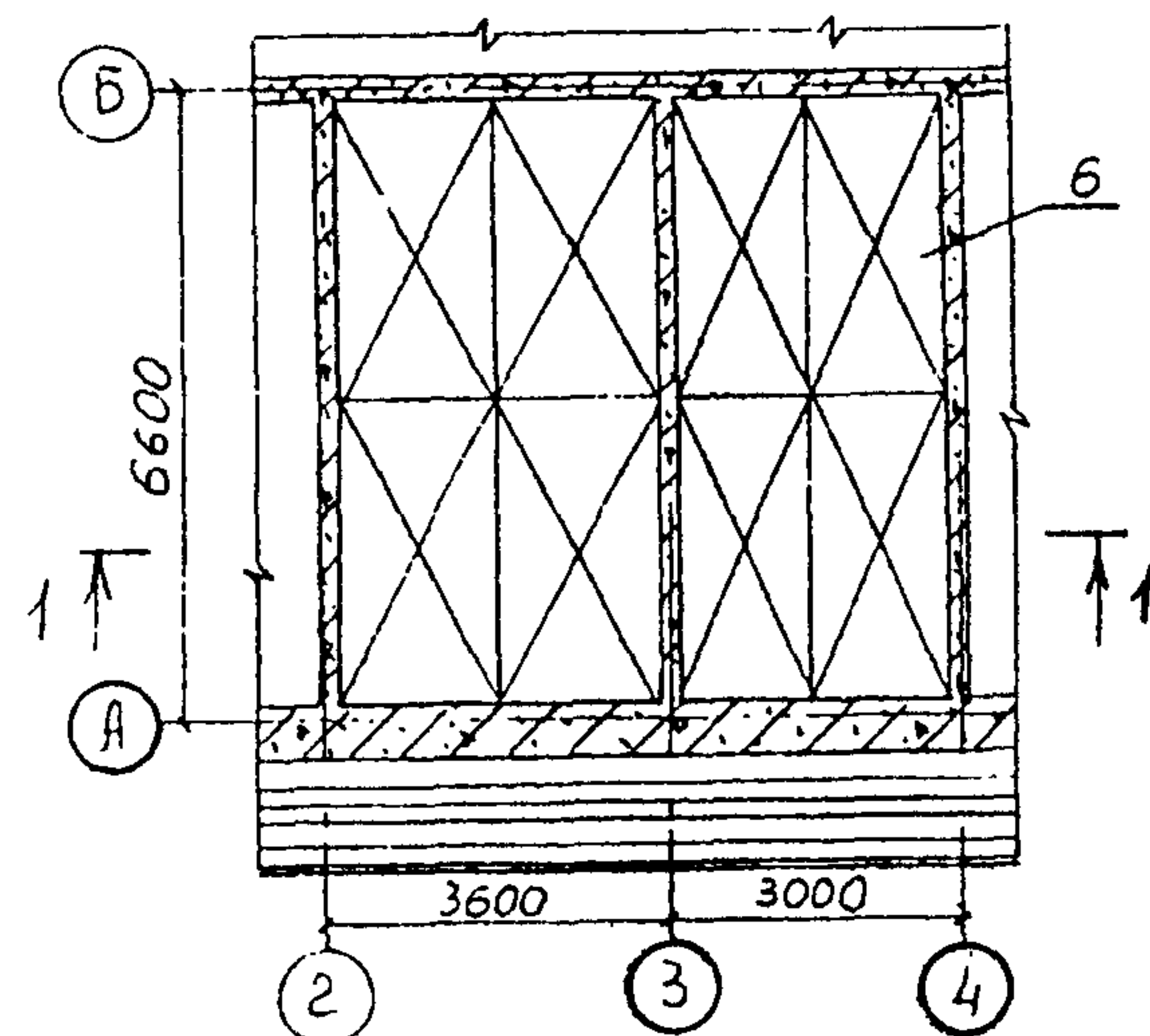
Раскладка листов фанеры
