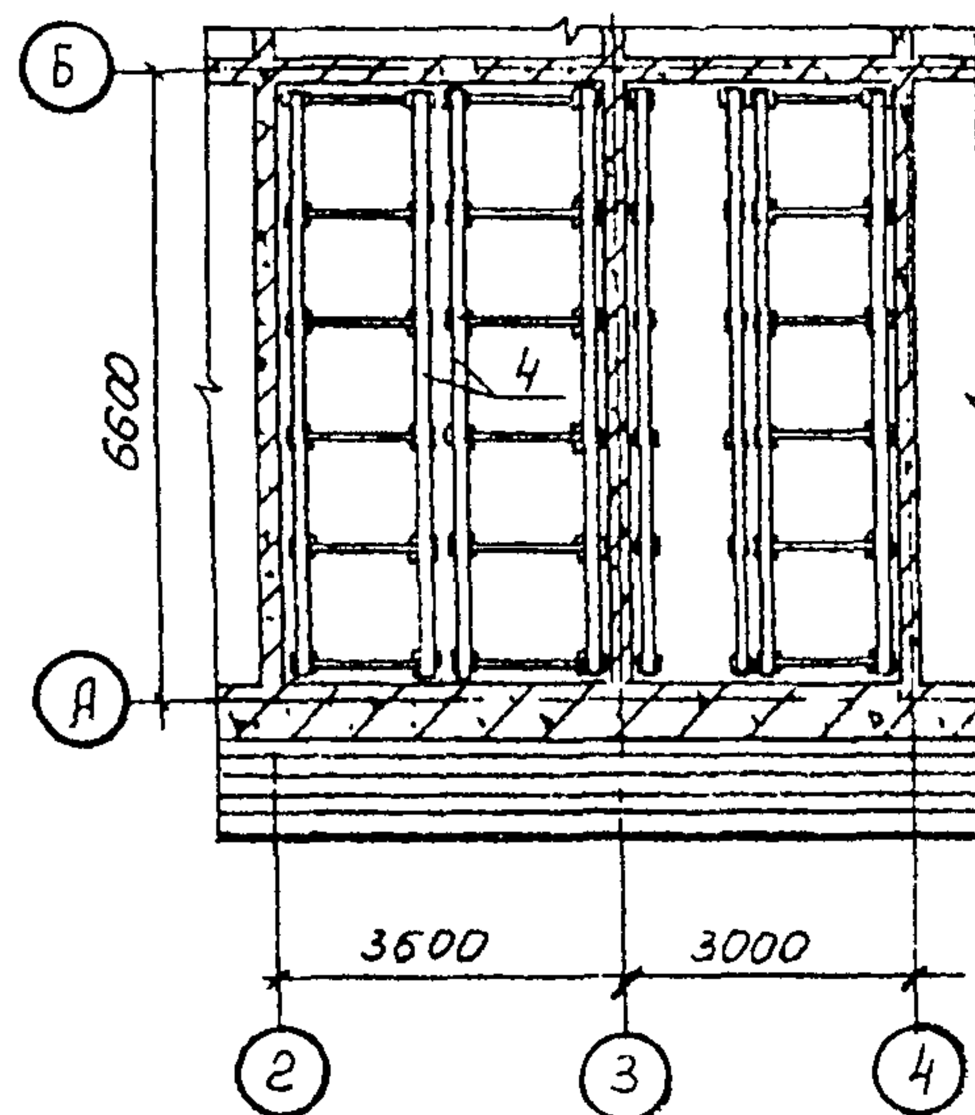
Установка продольных балок
