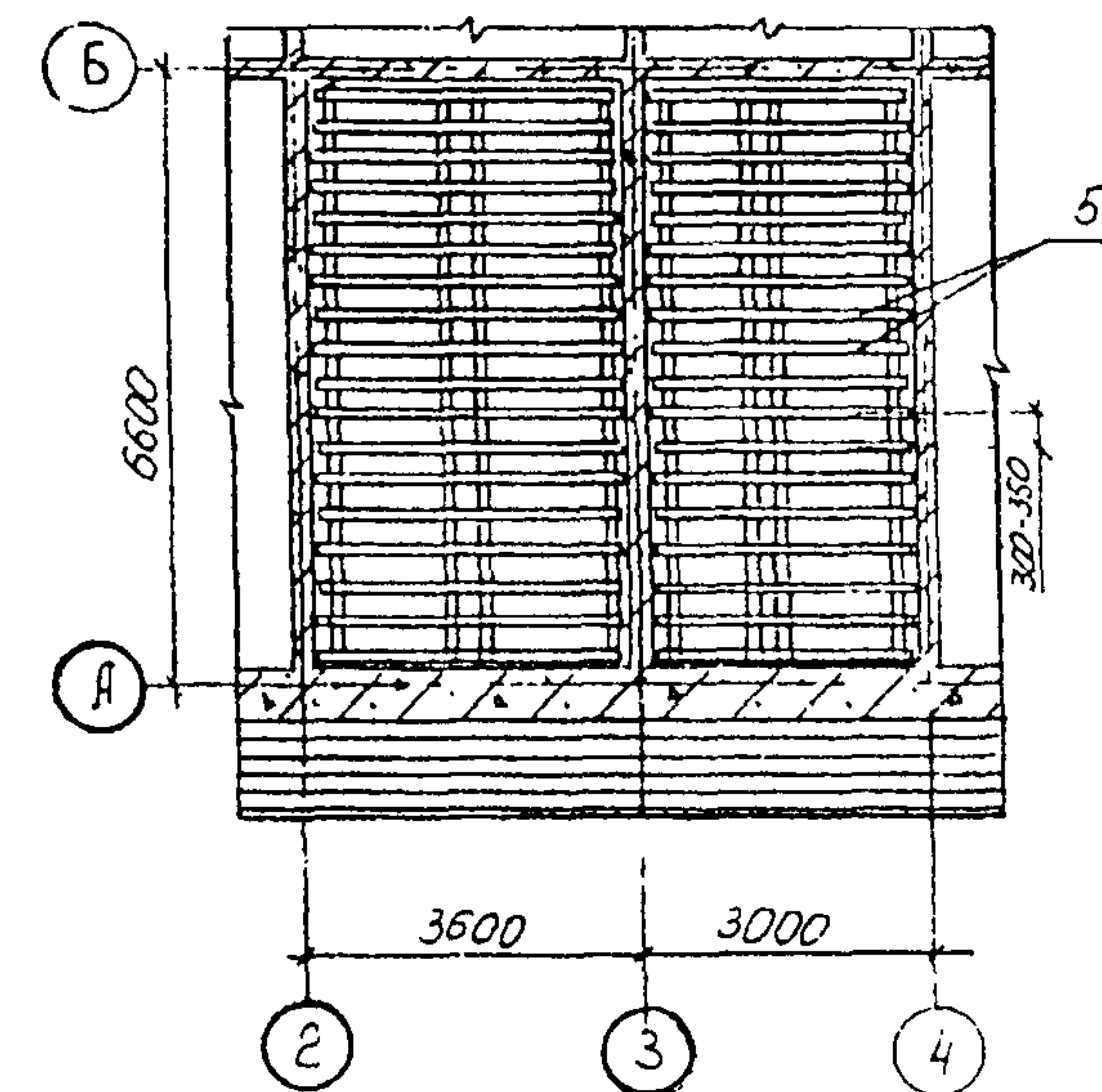
Установка поперечных балок
