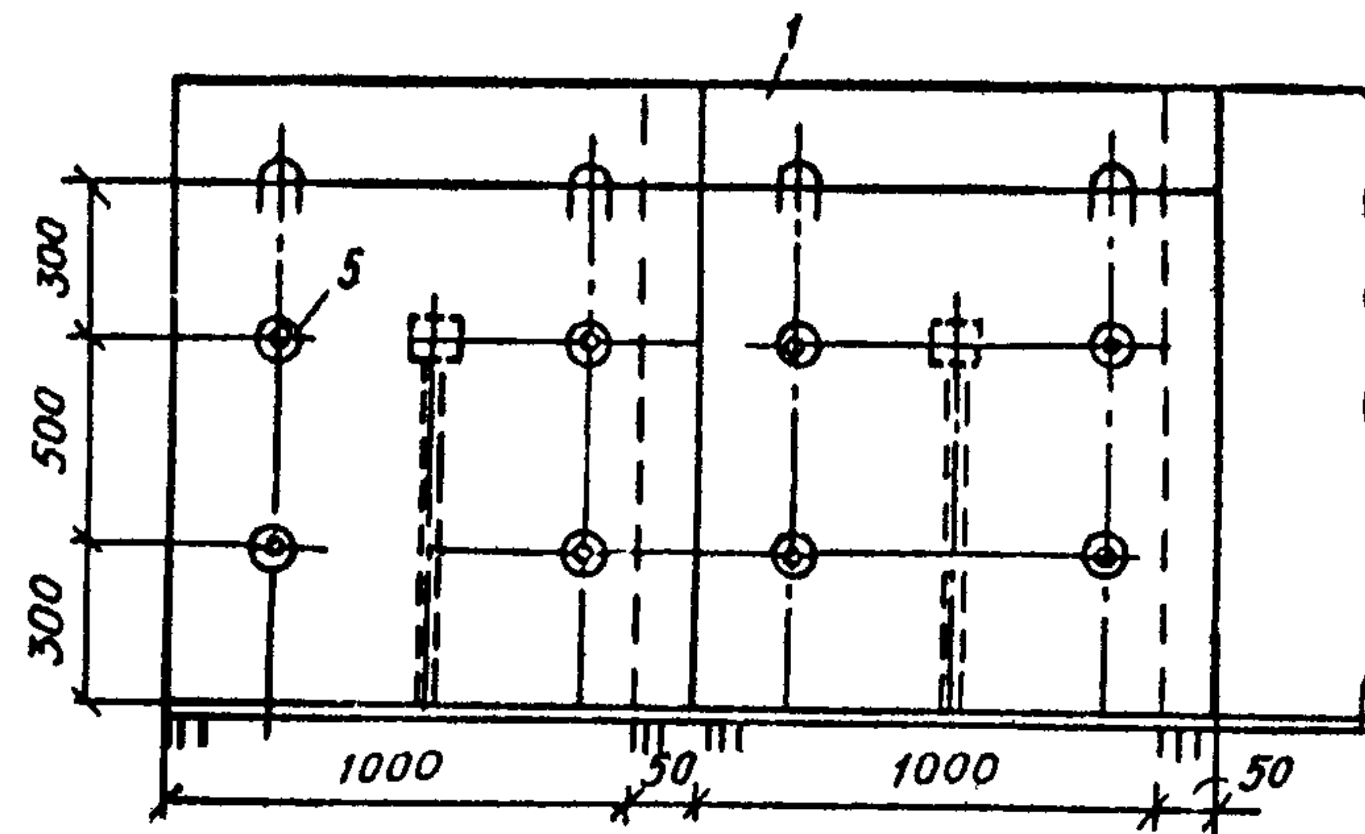
Схема сопряжения щитов-опалубок при их установке
