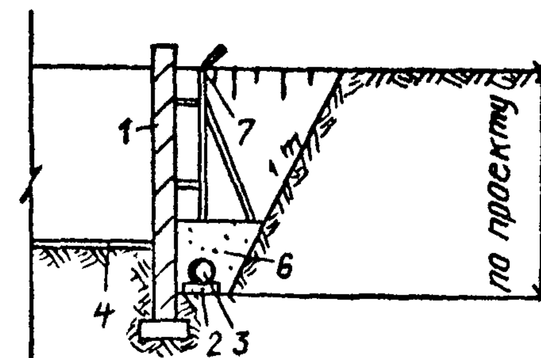
6. Демонтаж щита-опалубки
