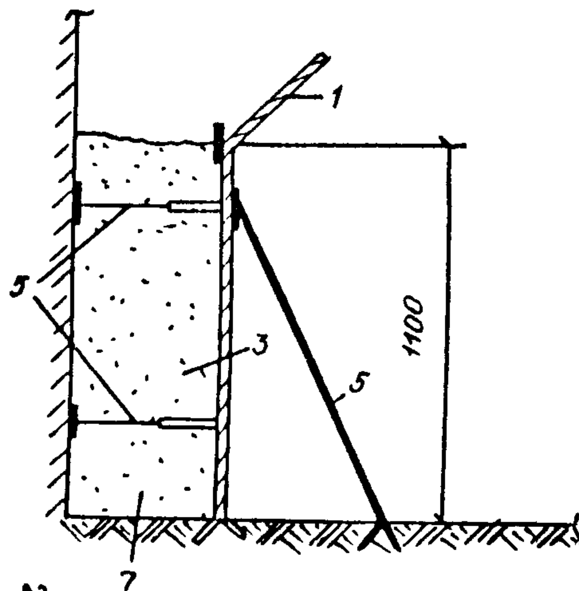
Схема сопряжения щитов-опалубок при их установке
