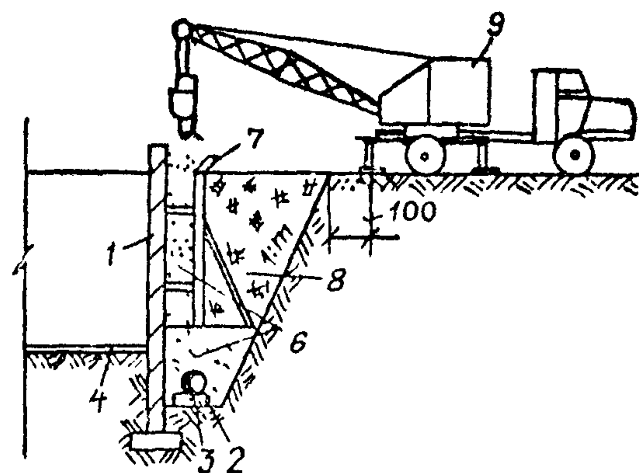
5. Устройство песчаной стены
