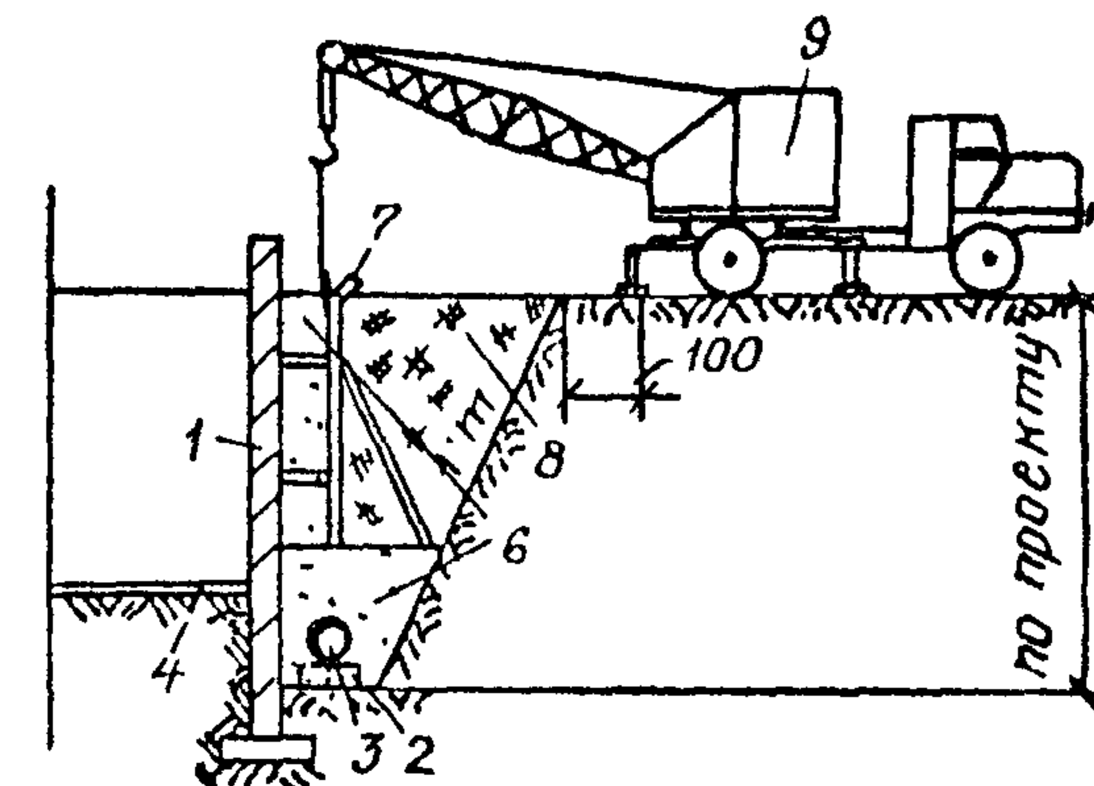
6. Демонтаж щита-опалубки
