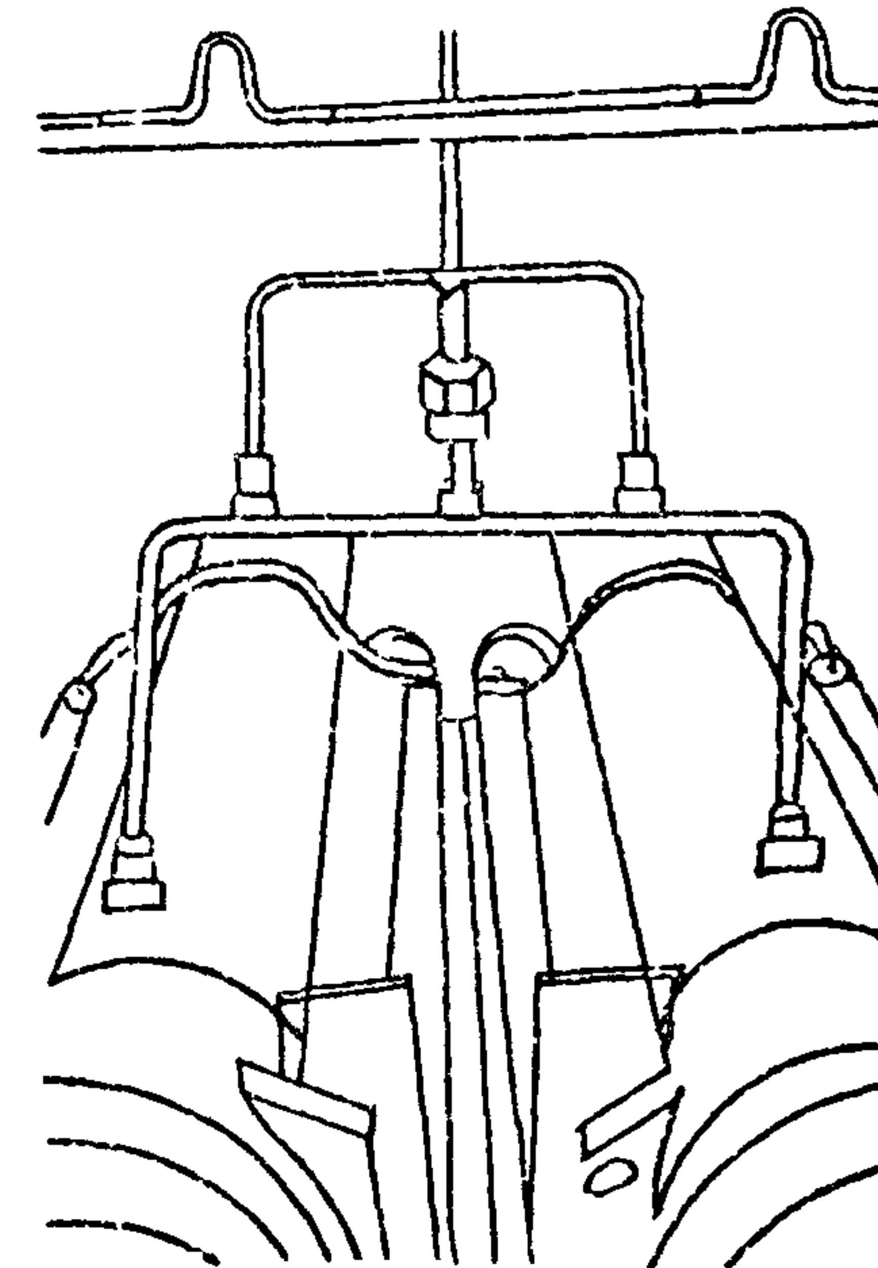
Гидродомкраты на раме (трест ГПР)
