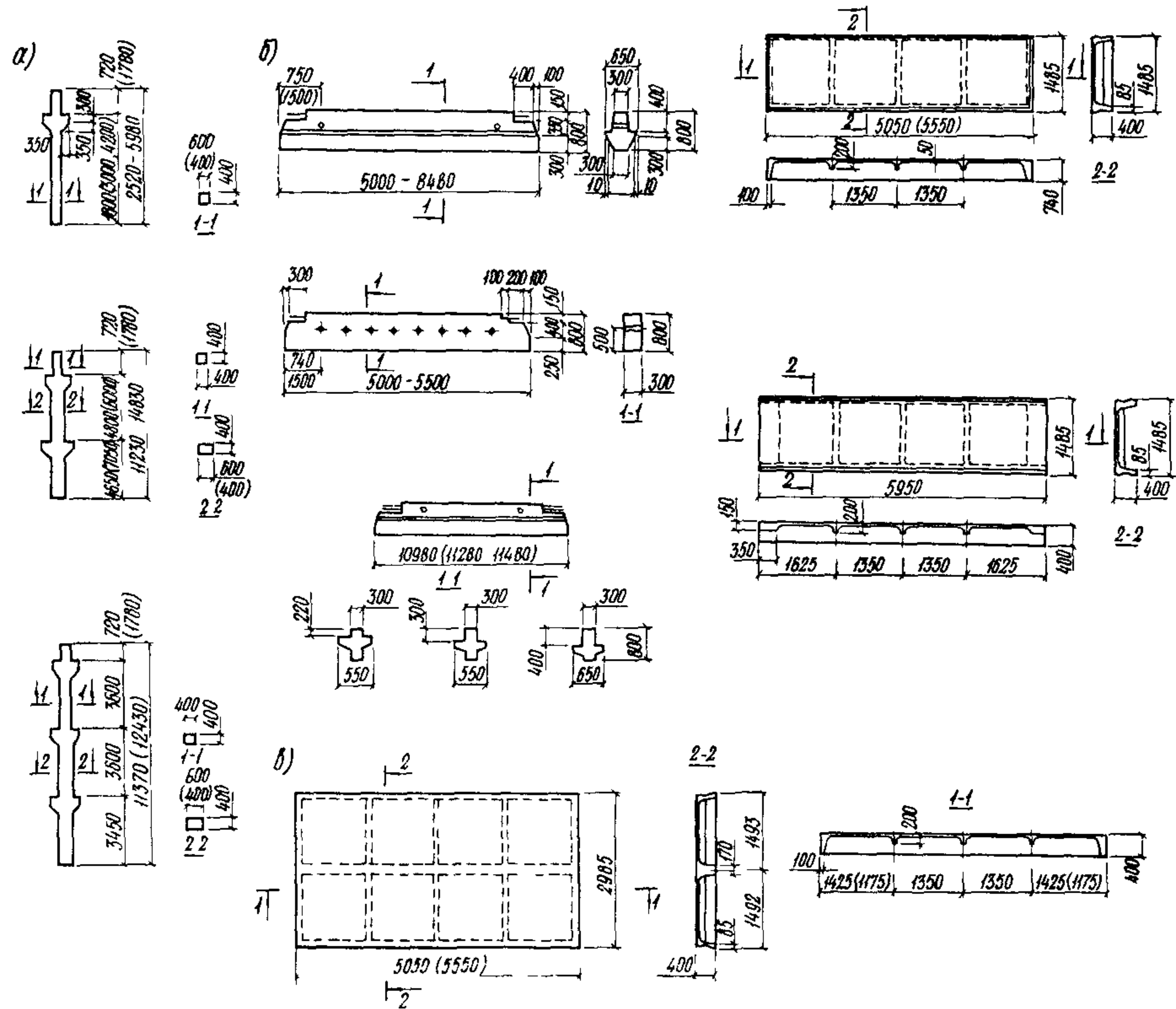
Рис. 2. Основные конструктивные элементы промышленных зданий серии ИИ 20/70, I.420-6, I-420-I2 а - колонны; б- ригели; в - плиты перекрытий
