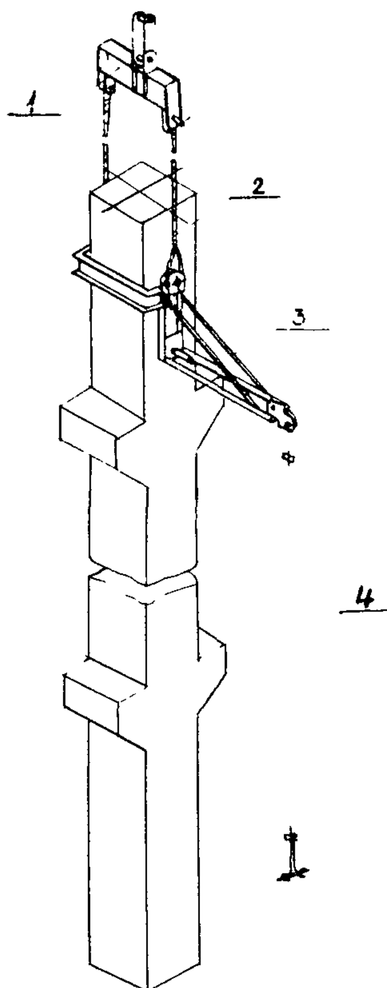
Рис. 5. Пальцевый захват для строповки колонн с отверстием
