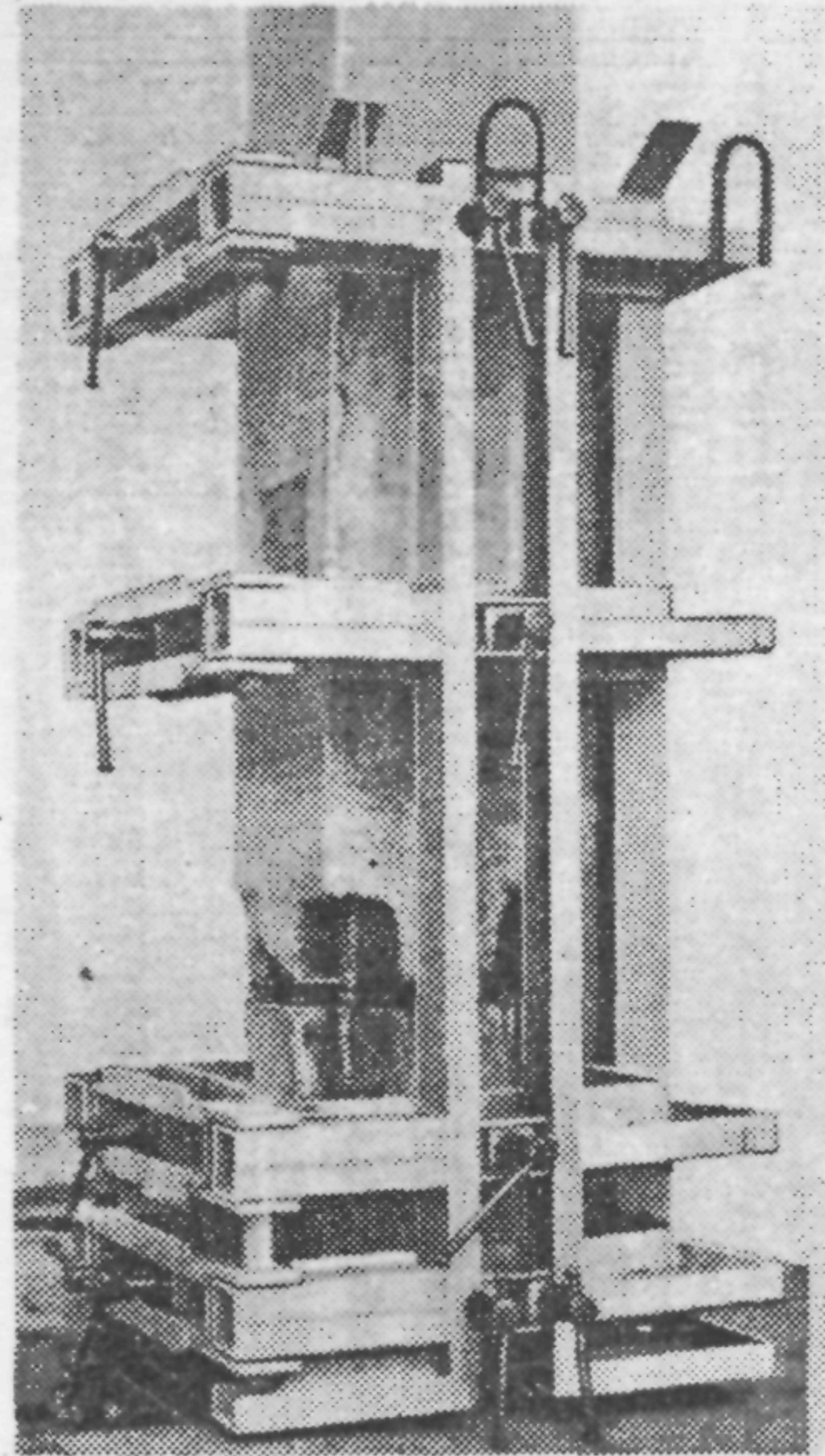
Рис. 7. Одиночный кондуктор для монтажа колонн связевого варианта каркаса серий ИИ-04, I.020-I
