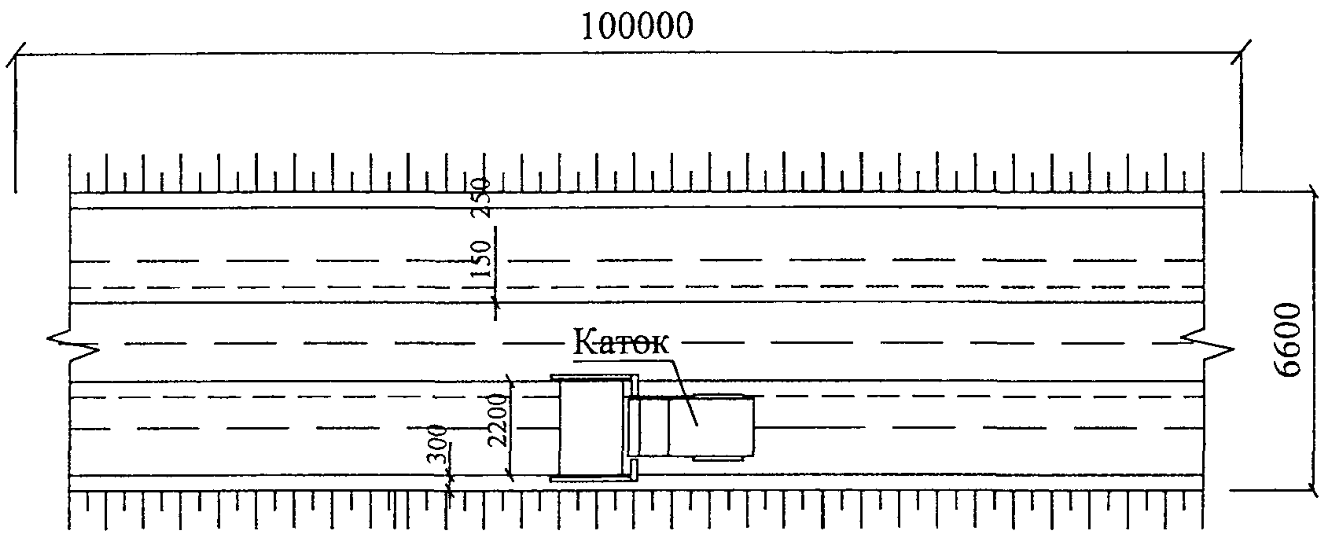
Рисунок 4 – Пример геометрии участка уплотнения для цифровых расчетов
