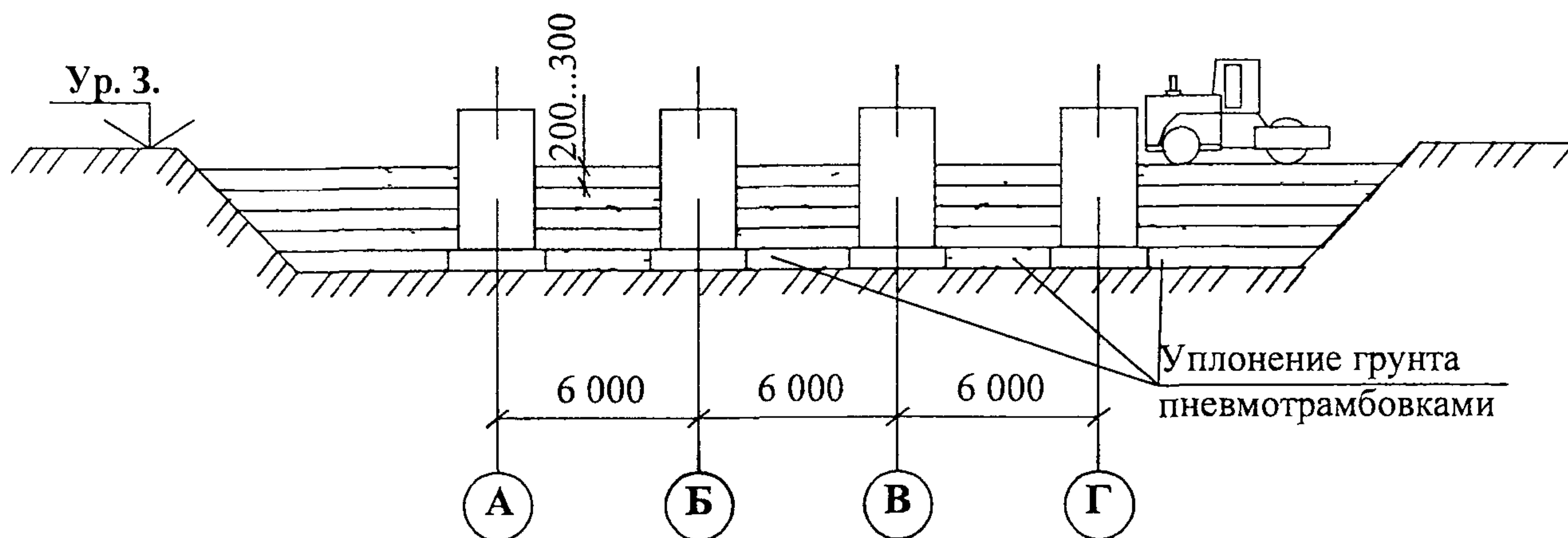
Рисунок 3- Схема послойного уплотнения грунта самоходными катками
