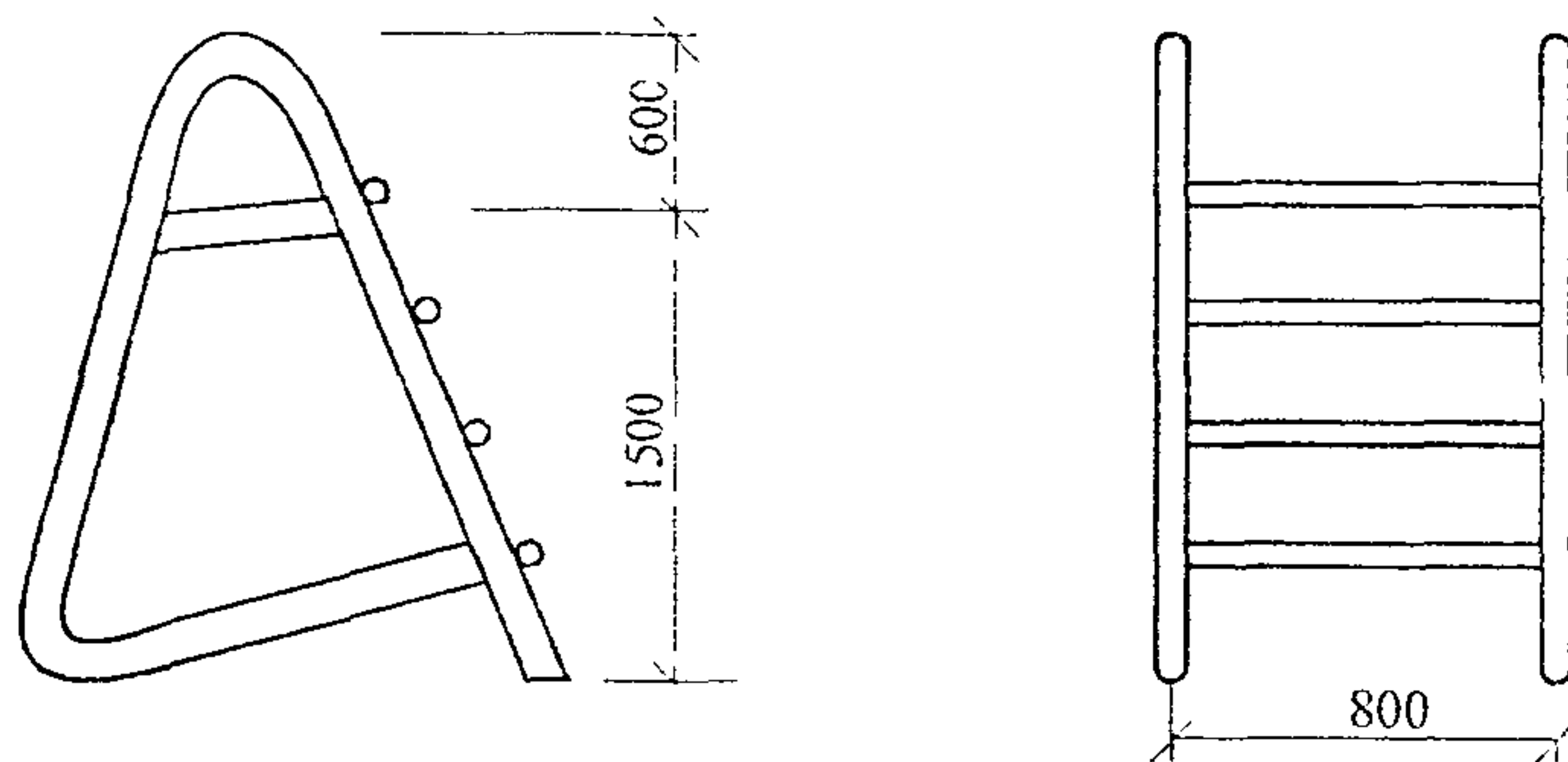
Рисунок 12 – Лестница-площадка
