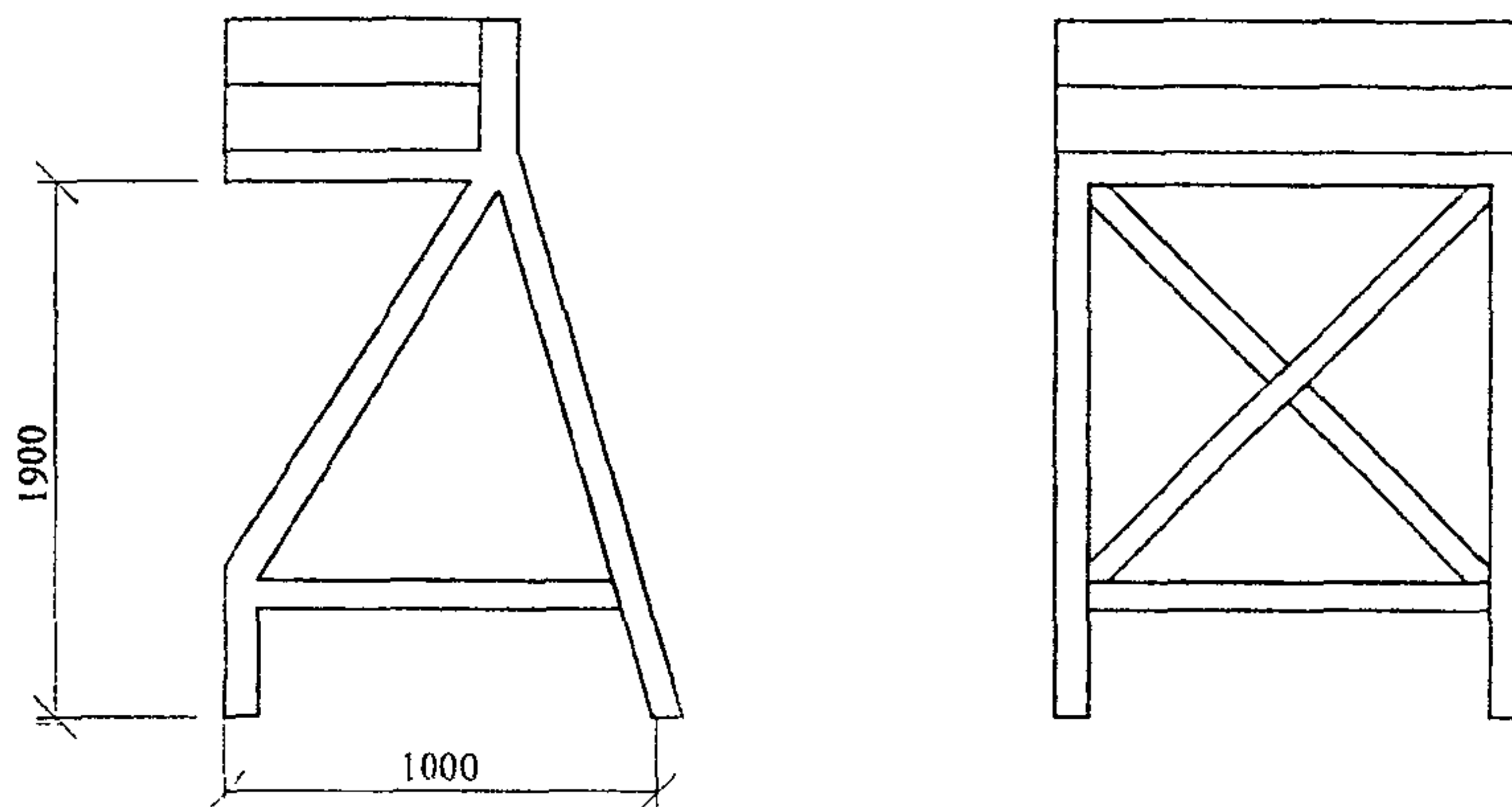
Рисунок 13 – Передвижная площадка Главкиевстрой
