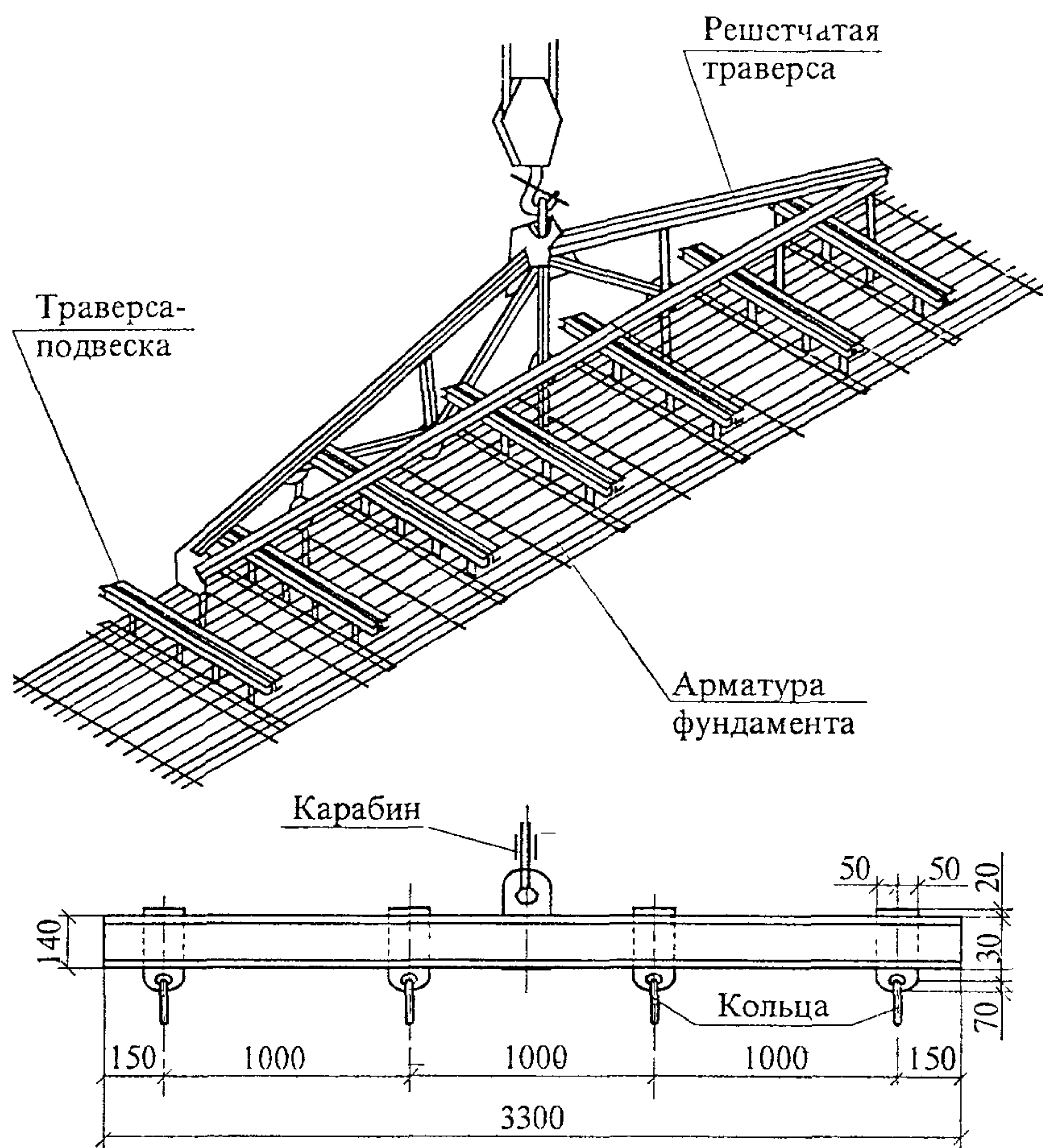
Траверса-подвеска
