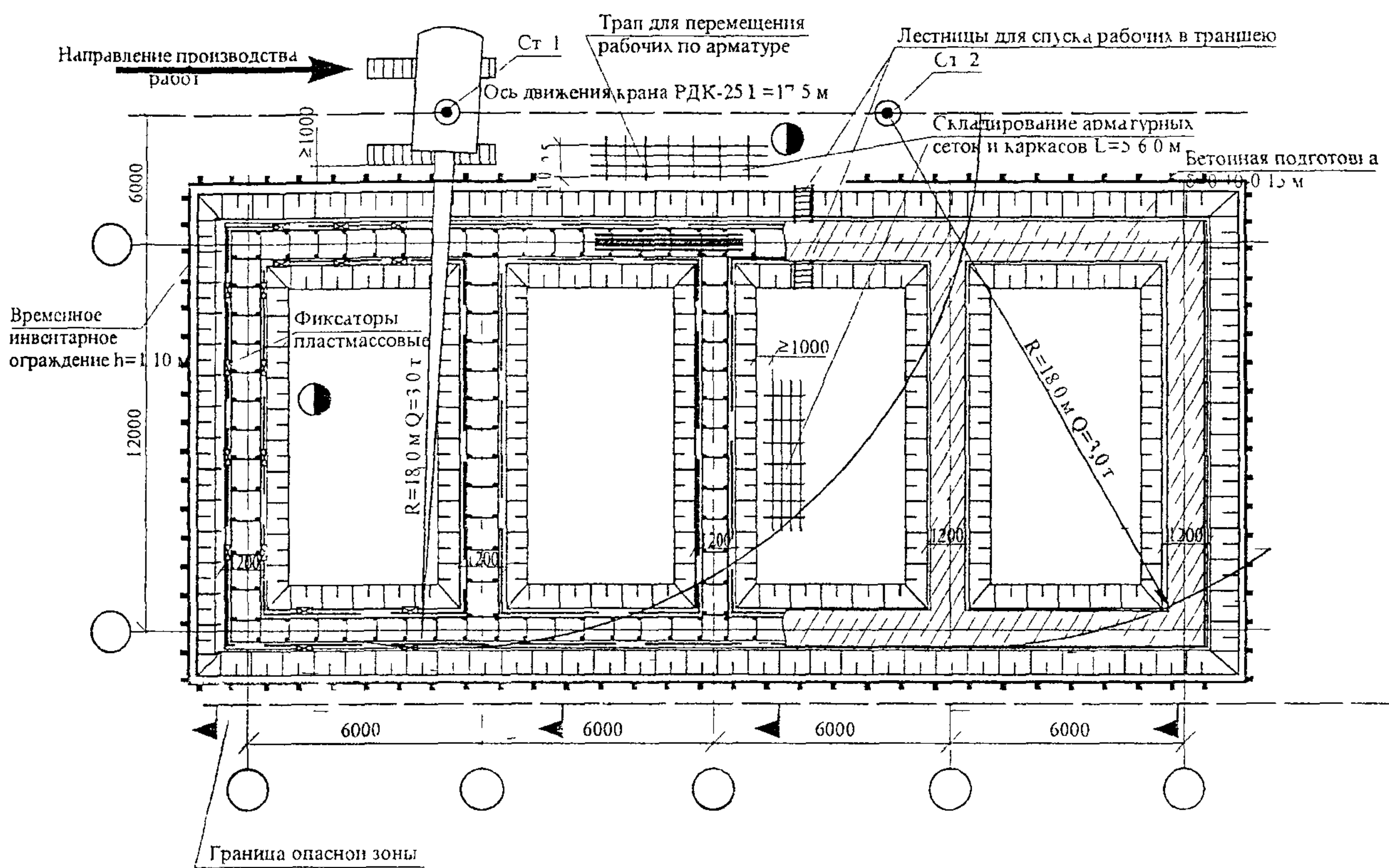
Рисунок 1 – Схема установки арматурных каркасов в ленточных фундаментах
