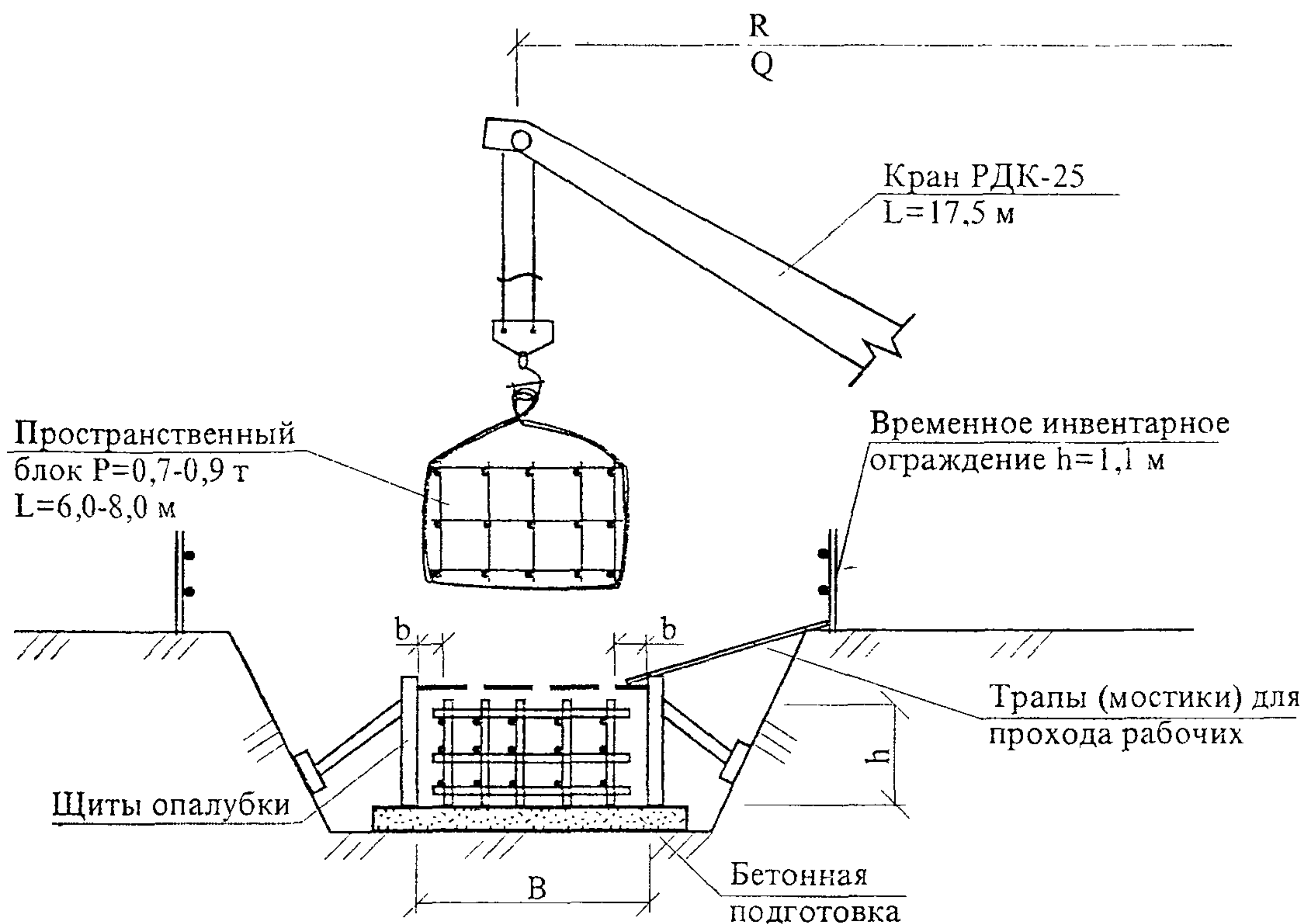
В – ширина фундамента (ростверка); h – высота каркаса; b – размер защитного слоя бетона Рисунок 3 – Схема монтажа пространственных арматурных блоков ленточного фундамента
