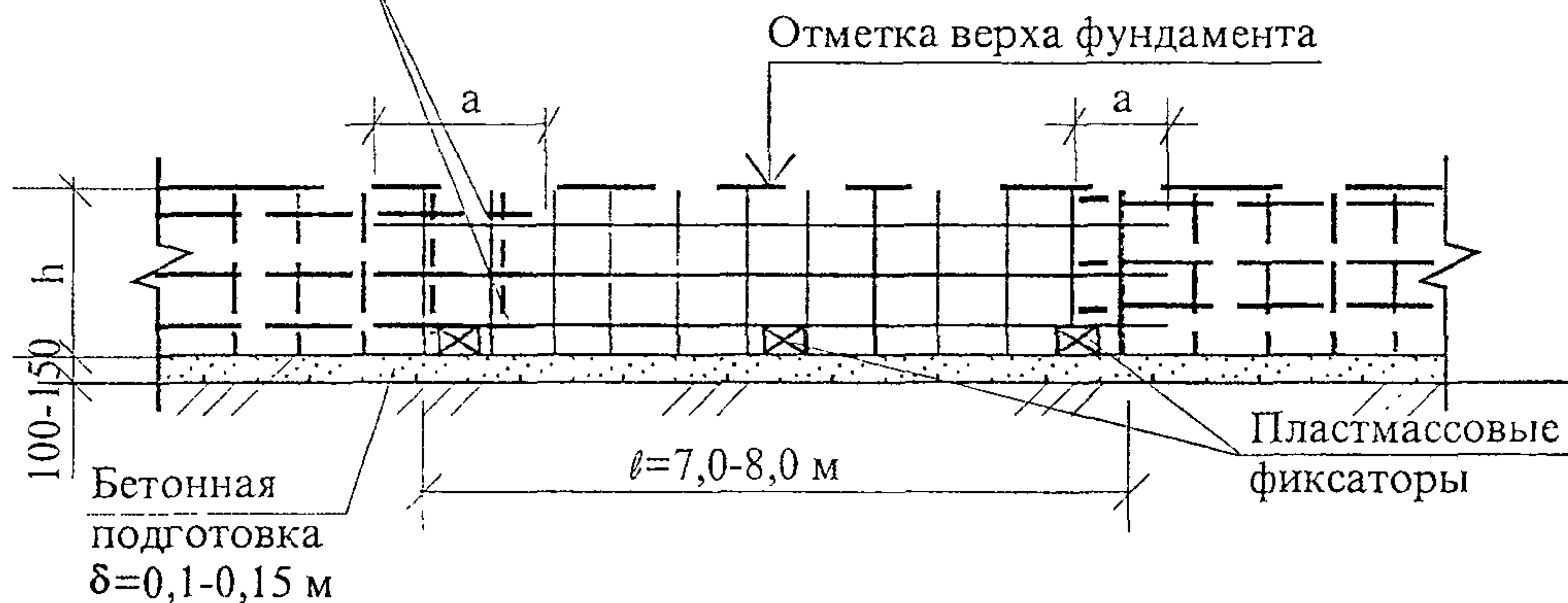
Рисунок 4 – Схема установки плоских каркасов
