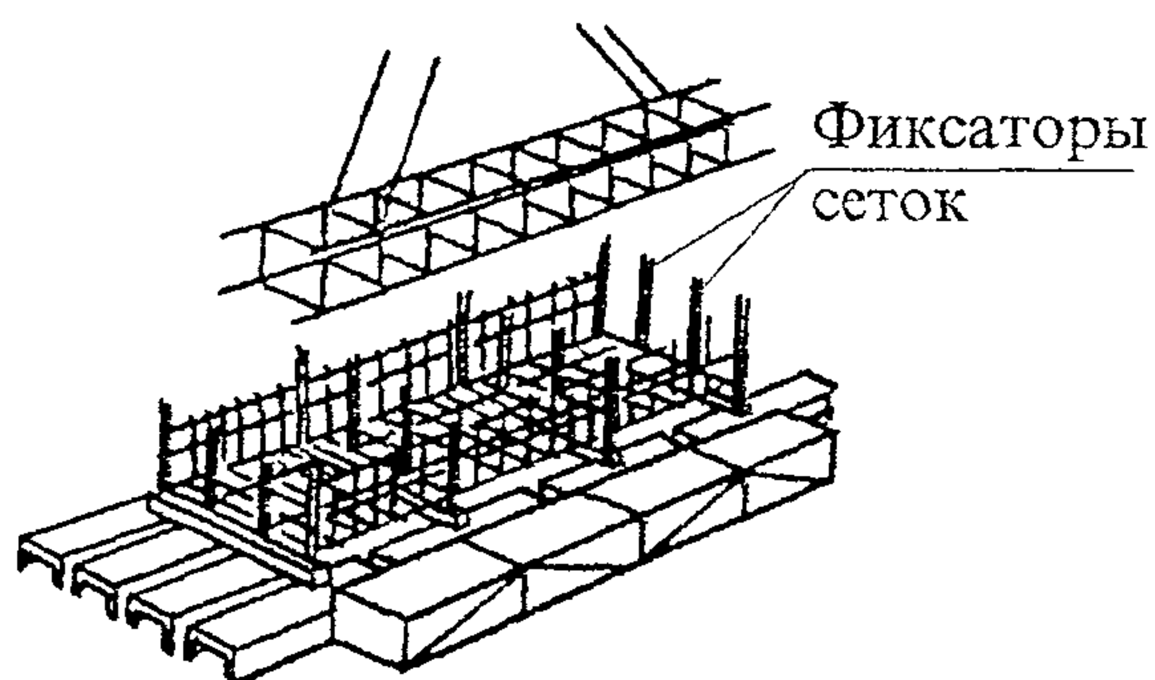
Рисунок 9 – Кондуктор-шаблон для сборки каркасов
