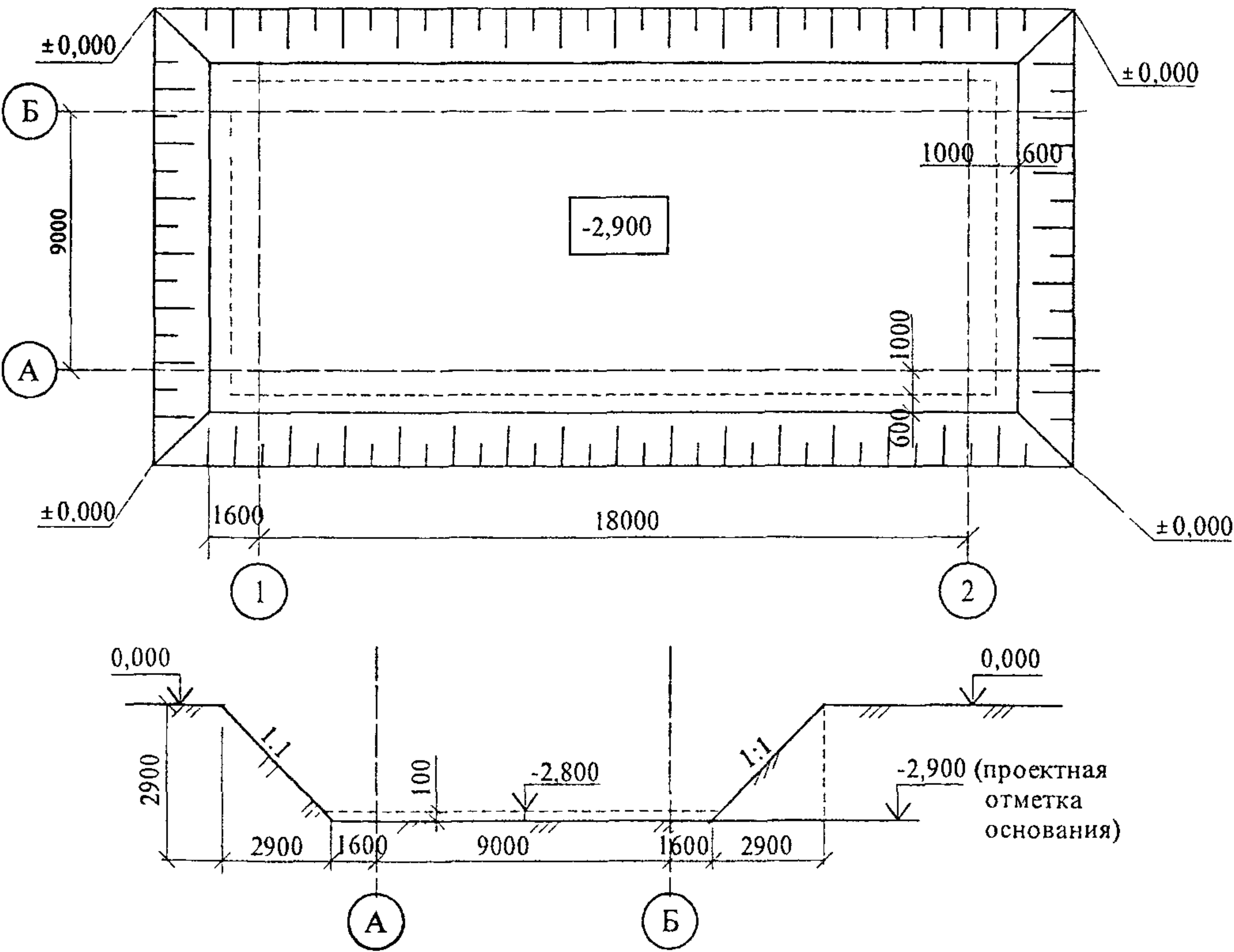
Рисунок 4 – Пример геометрии котлована для цифровых расчетов
