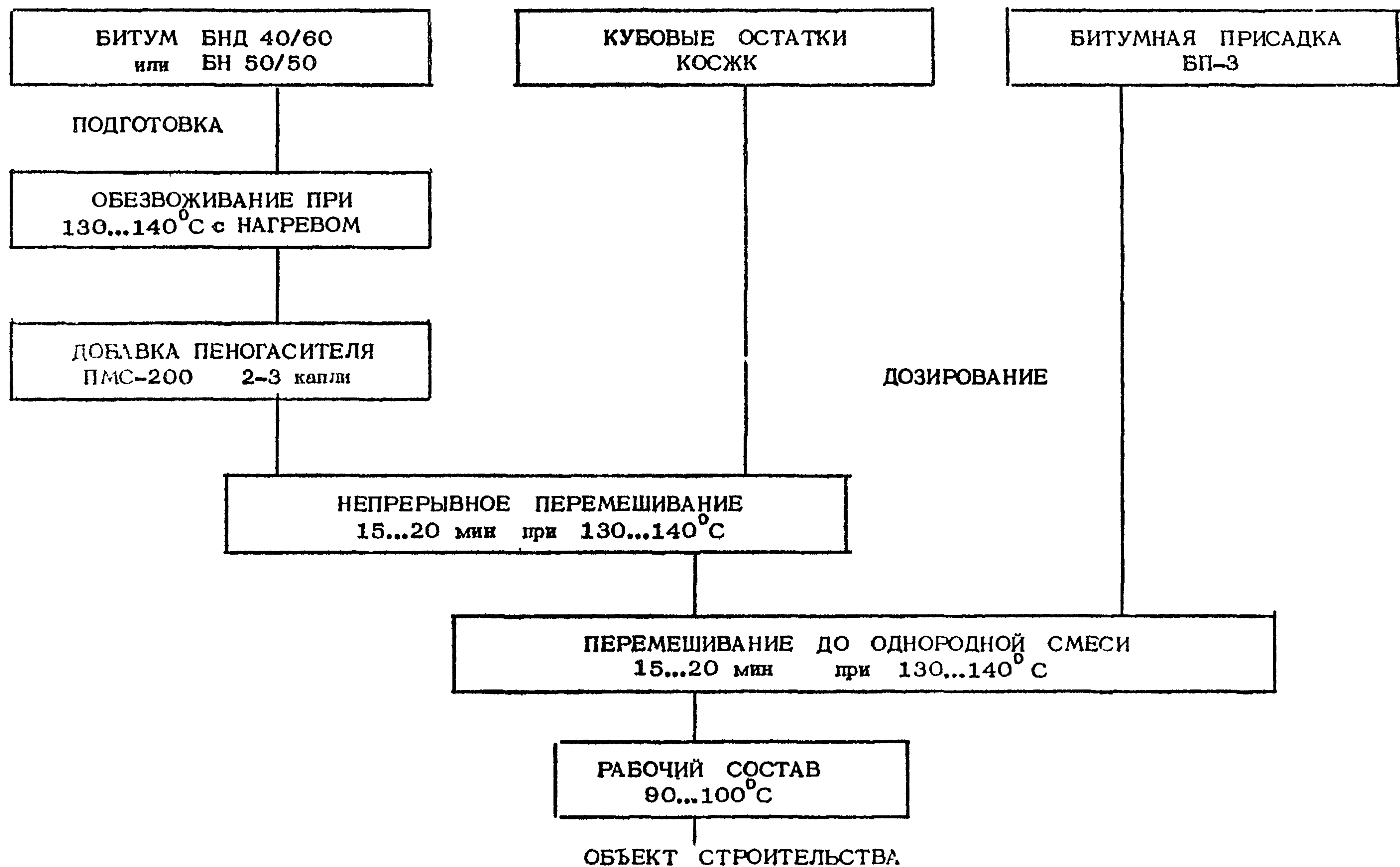
Рис. 1. Технологический процесс приготовления битумно-полимерной мастики
