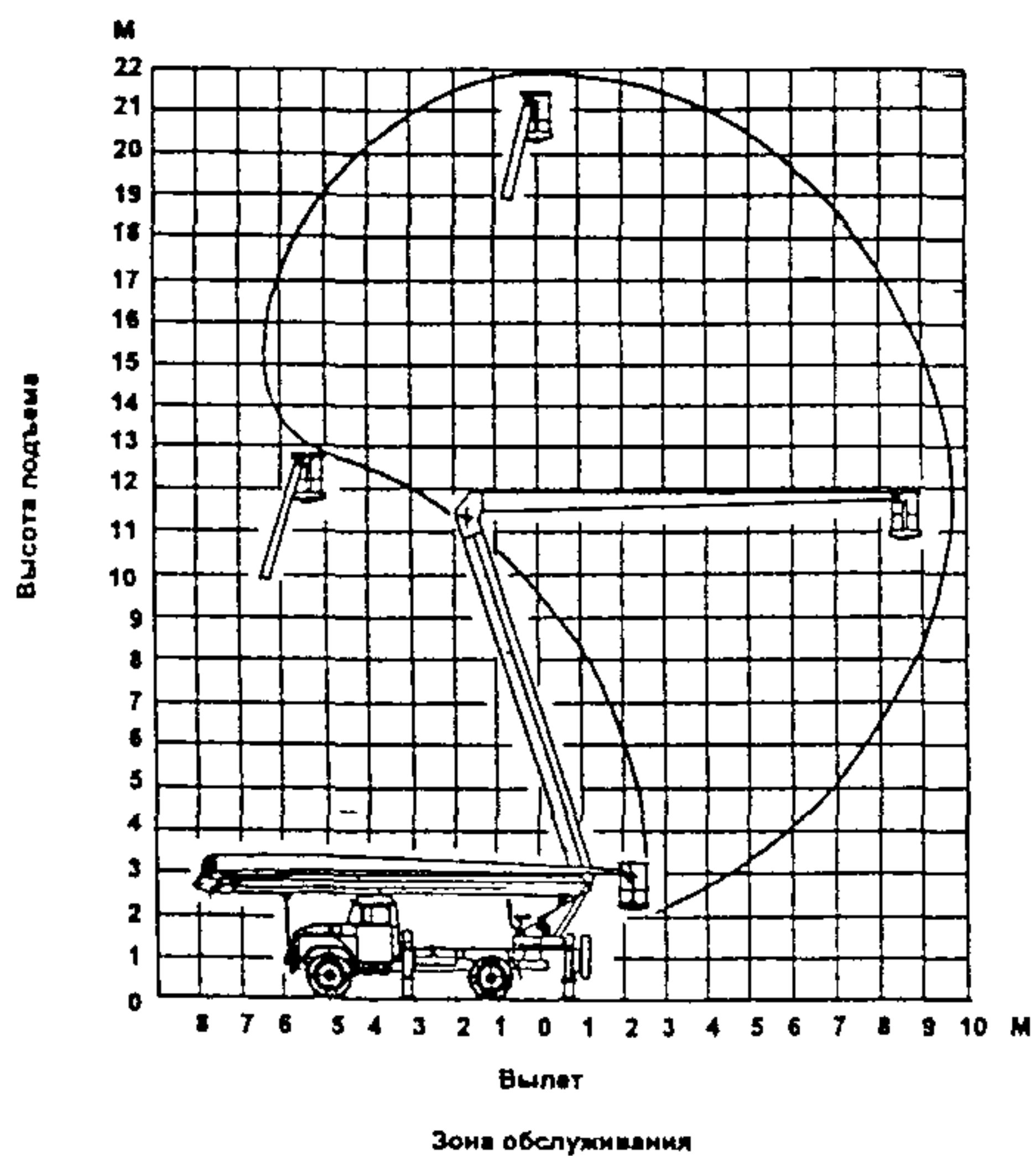
Рисунок 2 – Зоны обслуживания автомобильных подъемников
