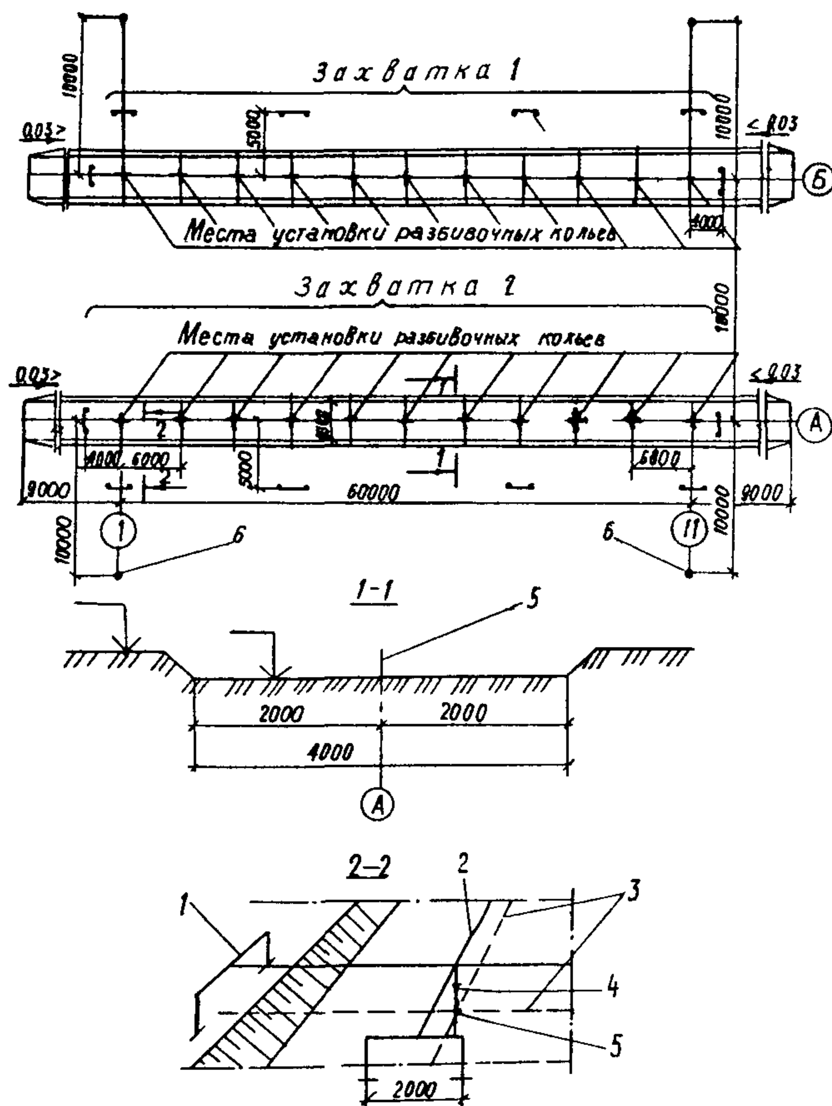
Рис. I. Схема расположения траншей и разбивочных колец:
