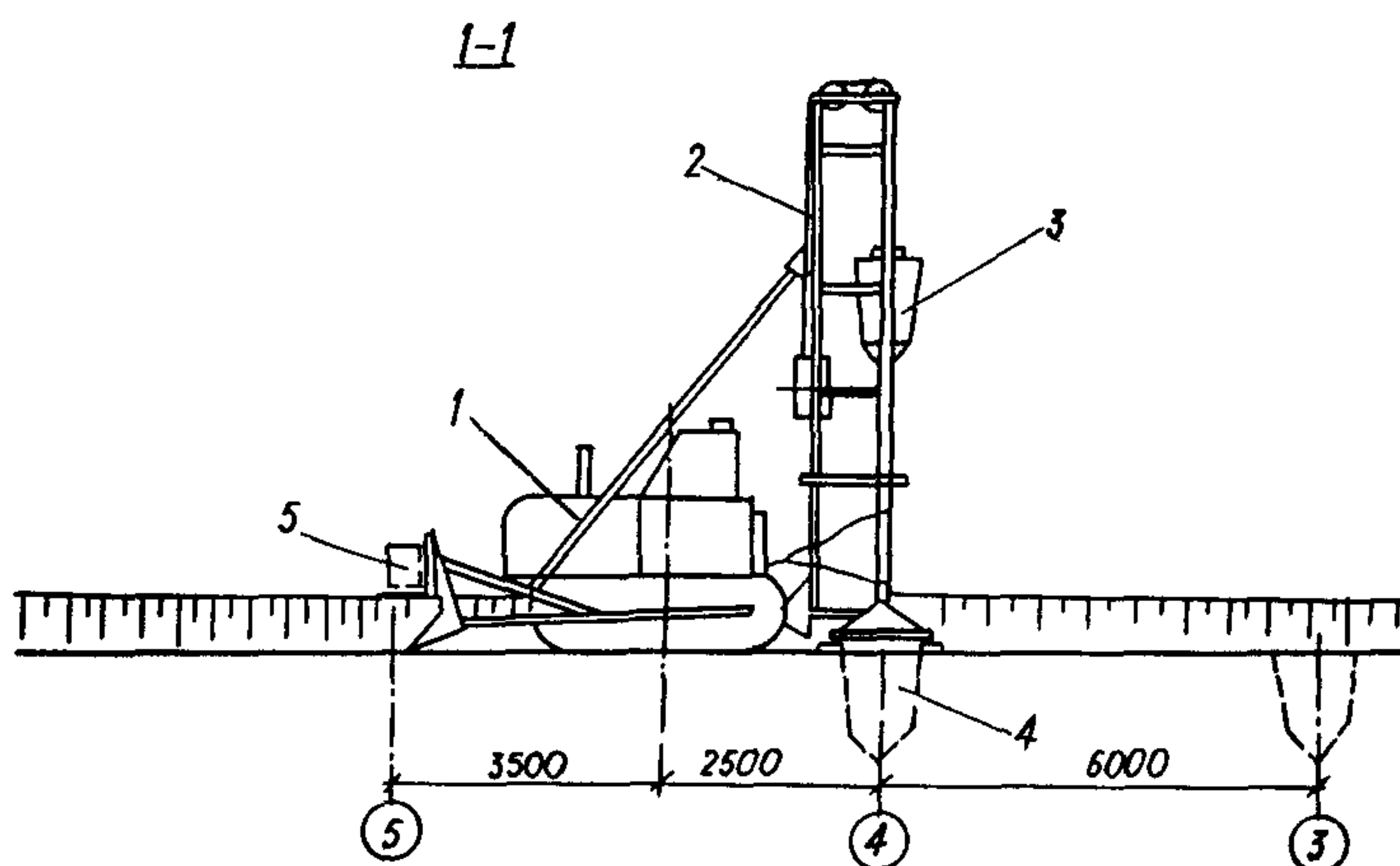
Рис.2. Схема устройства вытрамбованных котлованов: 1-бульдозер; 2-навесное оборудование; 3-трамбовка; 4-котлован; 5-противовес
