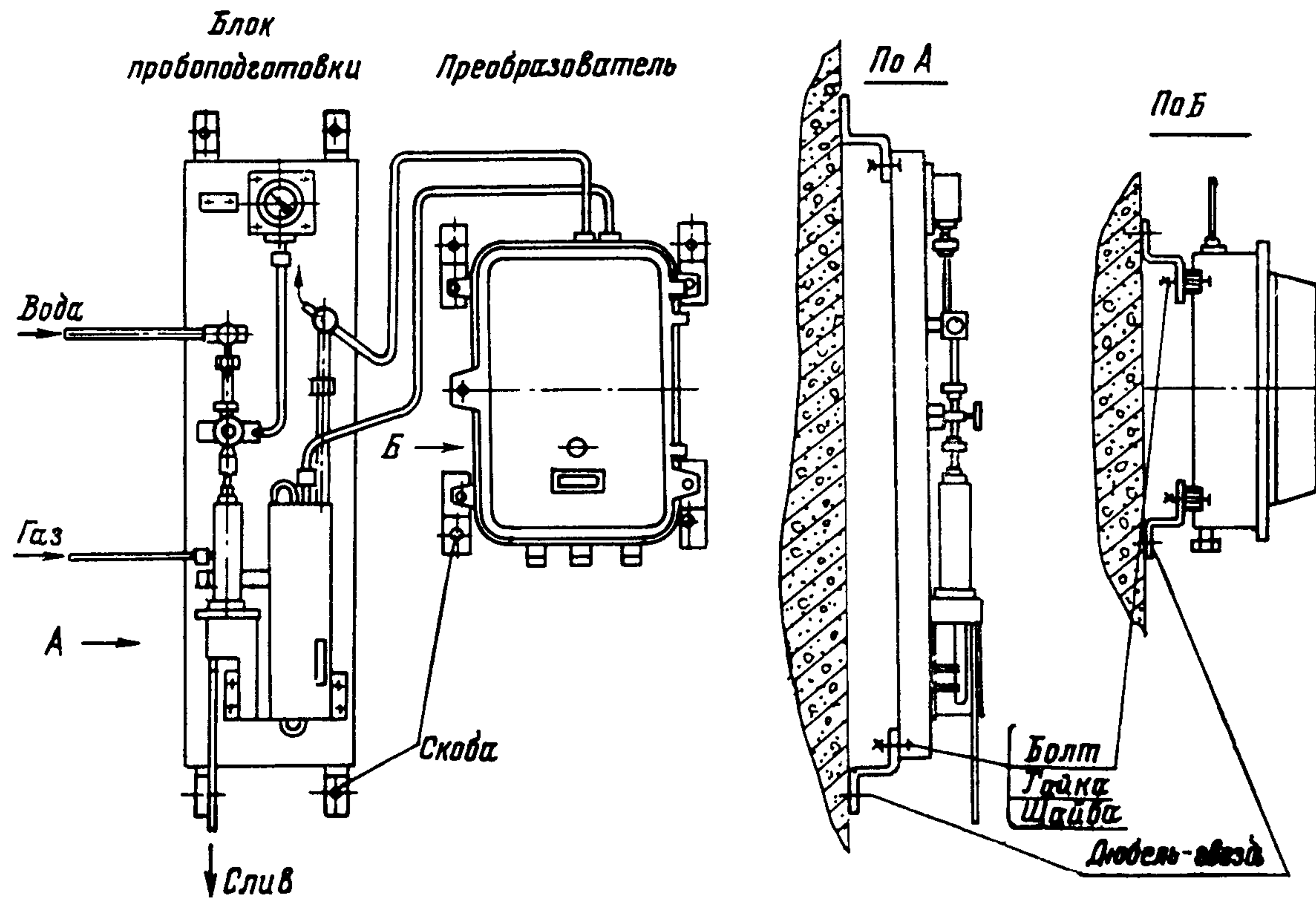
Рис. 1. Установка газоанализатора МН 5106-2 на стене
