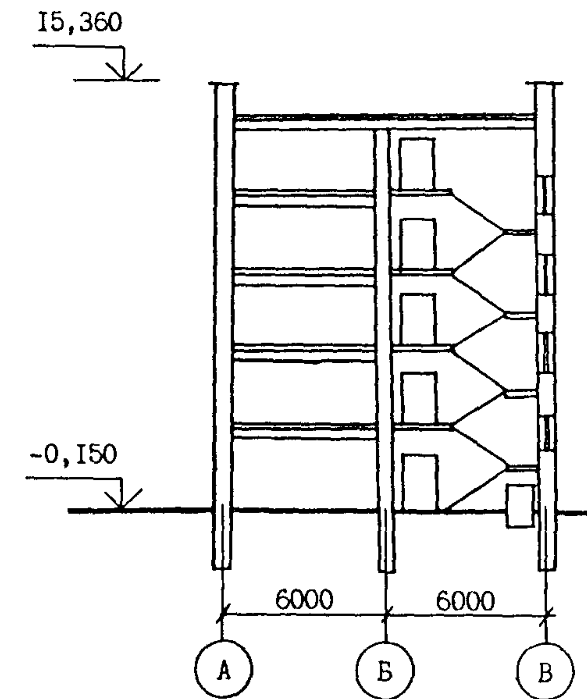
РАЗРЕЗ I-I
