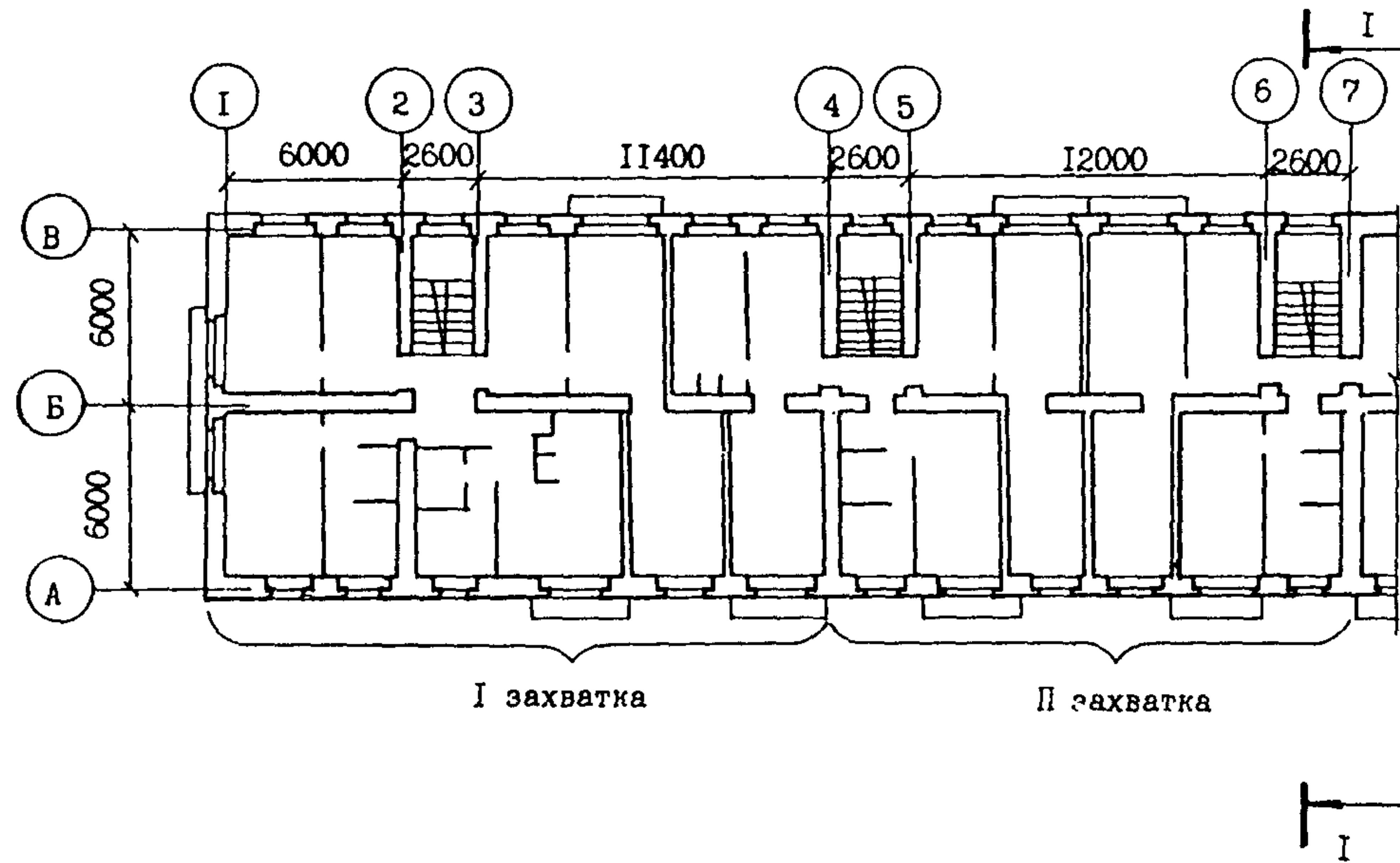
ПЛАН ЗДАНИЯ
