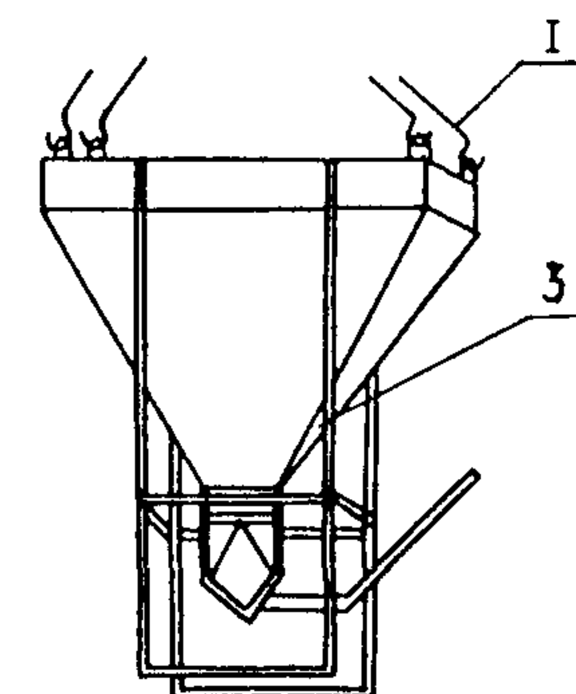
СТРОПОВКА БУНКЕРА С РАСТВОРОМ
