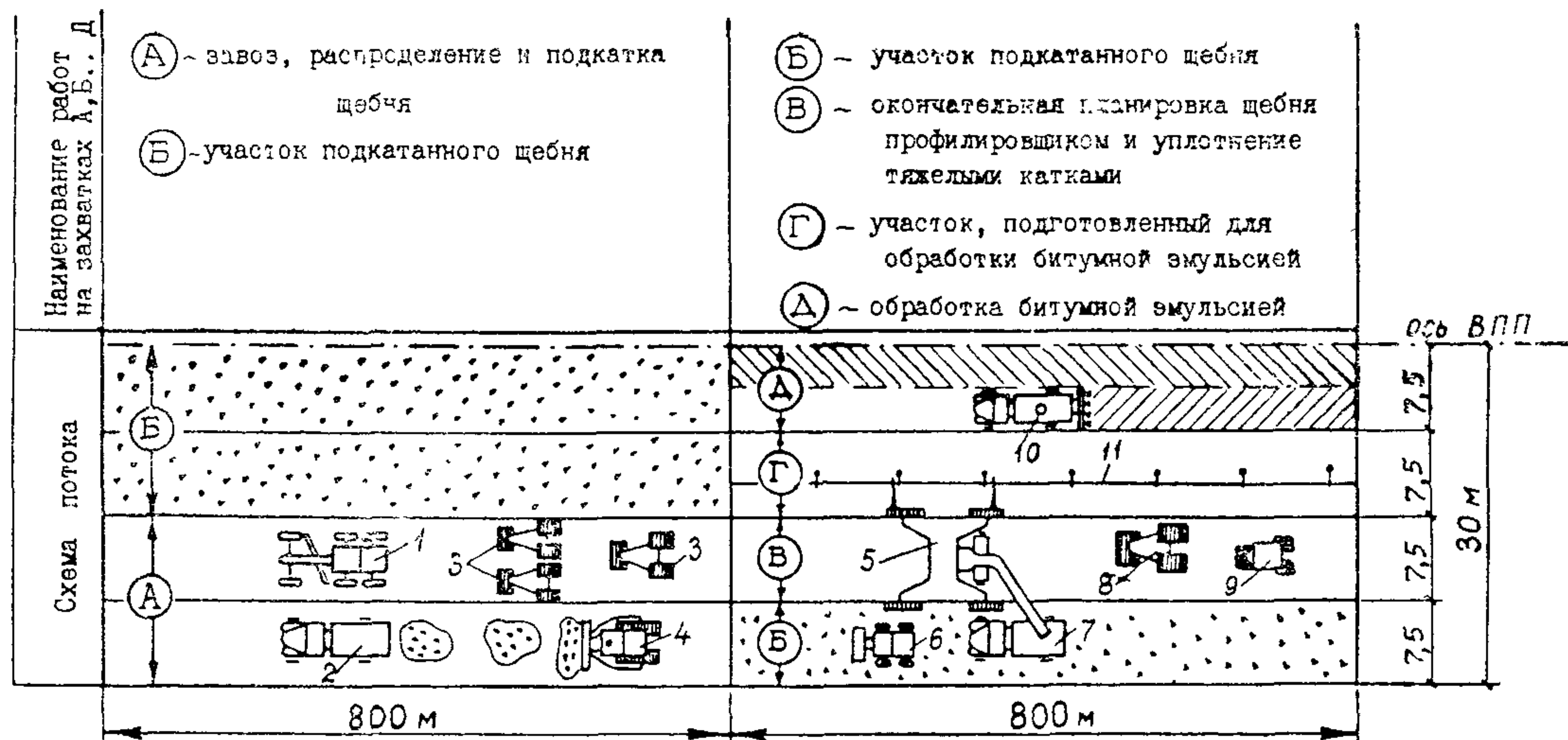
Рис. 2. Схема организации работ по устройству щебеночного основания: 1—автогрейдер Д-395; 2—автомобиль-самосвал со щебнем; 3—легкие моторные катки Д-552; 4—бульдозер Д-493А; 5—профилировщик ТS-425 или ДС-97; 6—ковшовый погрузчик ТО-18; 7—автомобиль-самосвал, 8—тяжелый моторный каток Д-553; 9—каток на пневматических шинах Д-627А; 10—автогудронатор Д-640А, 11—копирная струна
