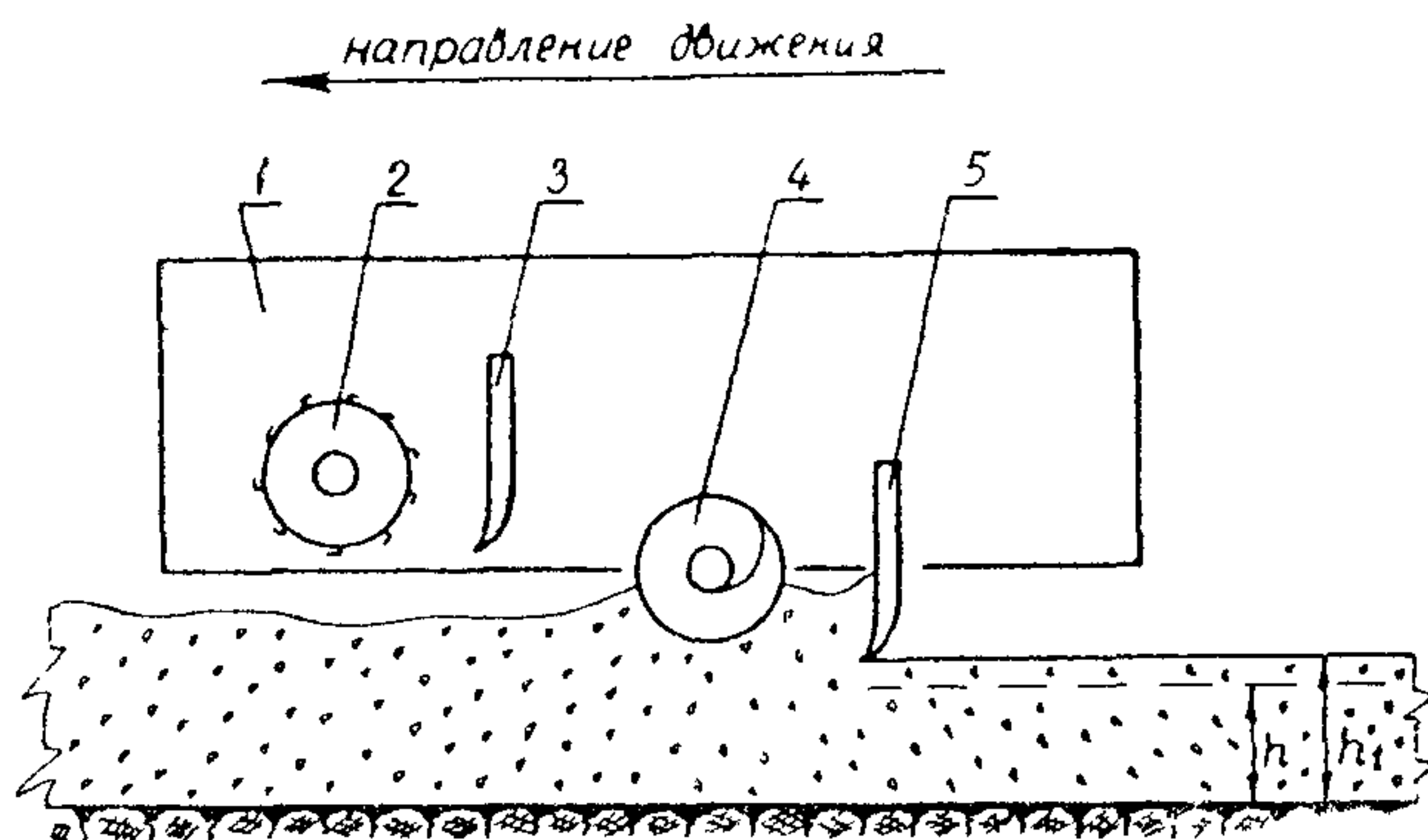
Рис. 3. Положение рабочих органов профилировщика при планировке щебня:
