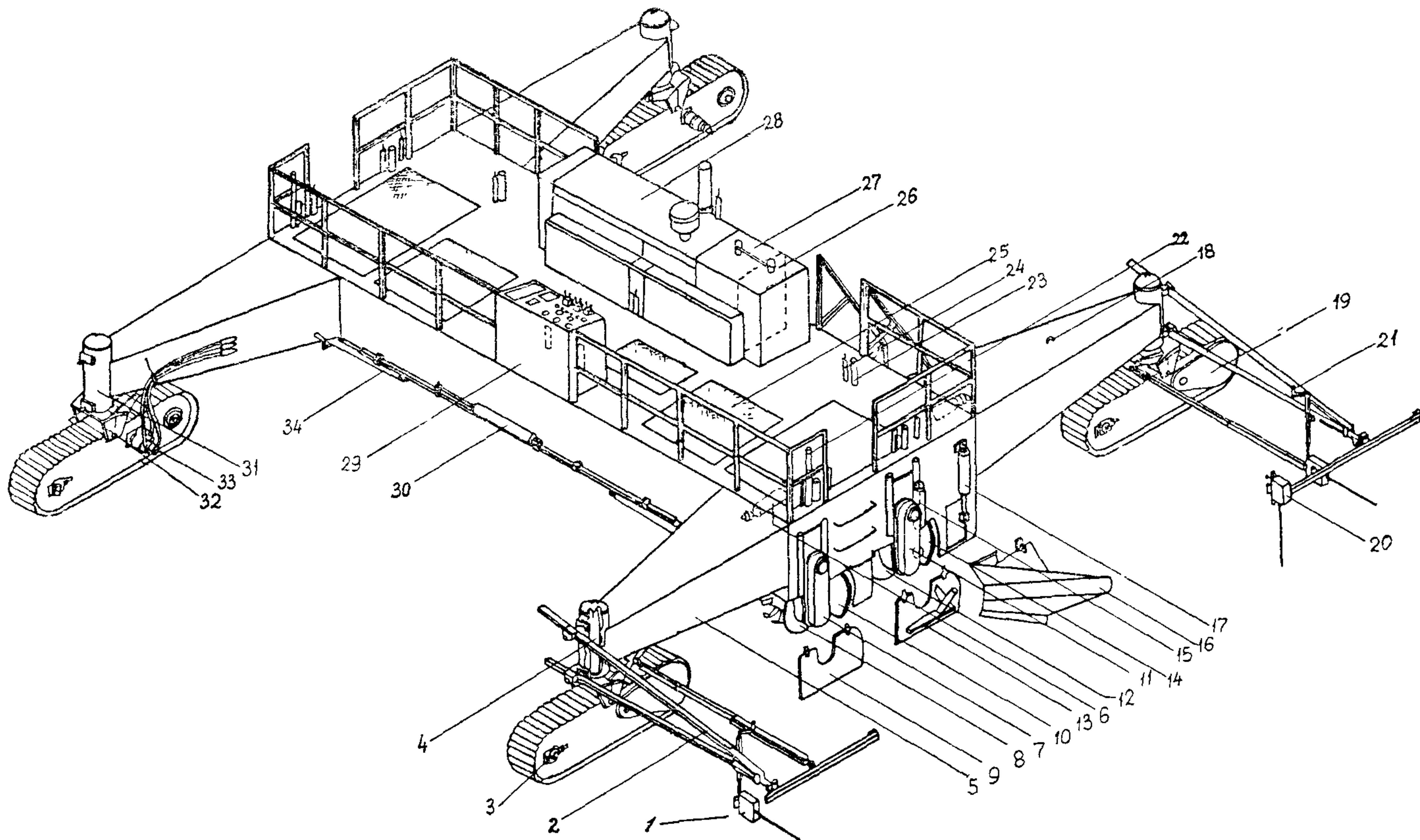
Рис. 1. Основные части профилировщика TS-425:
