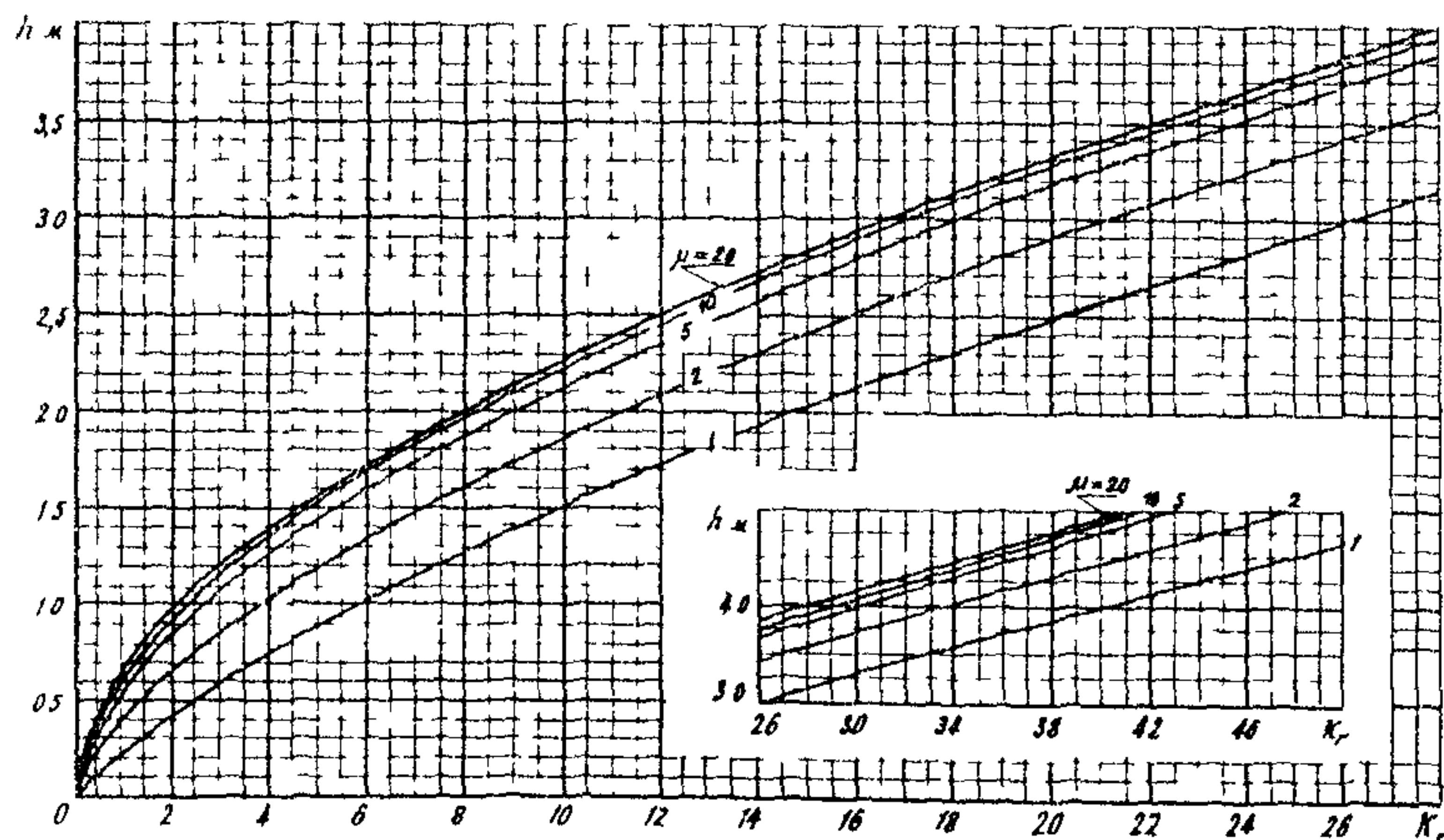
Рис.2. Графики для определения глубины протаивания земляного полотна
