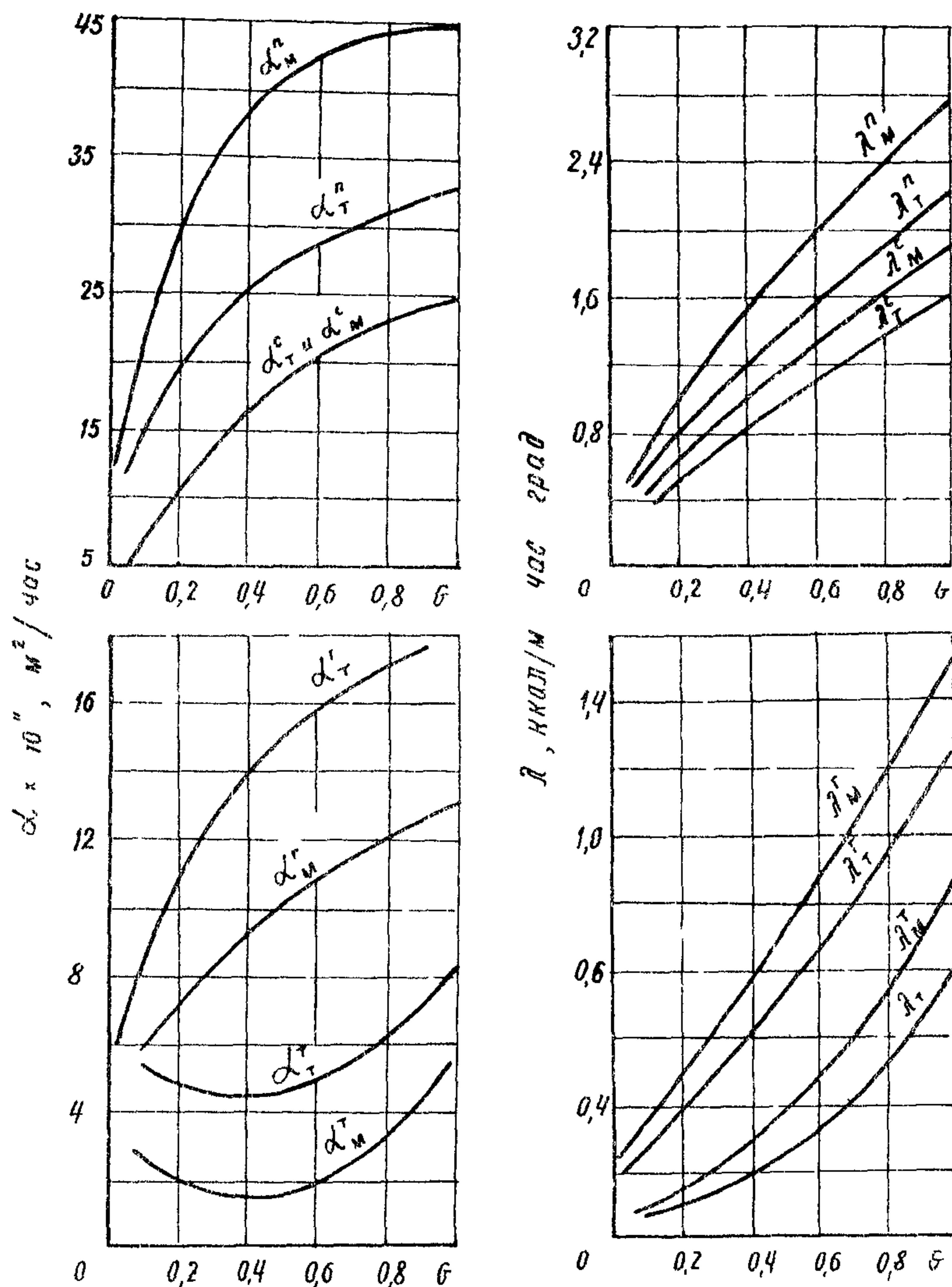
Рис.1. Графики для определения коэффициентов темпера - туро ( \alpha ) - и теплопроводности ( \lambda ) грунтов. Индек - сы вверху означают: П-пески, С-супеси, Г-суглинки и глины, Т-торфы. Индексы внизу: Т-талые, М-мерзлые. Средние значения объемной теплоемкости грунтов определяют по формуле C_{об} = \frac{\lambda}{\alpha}
