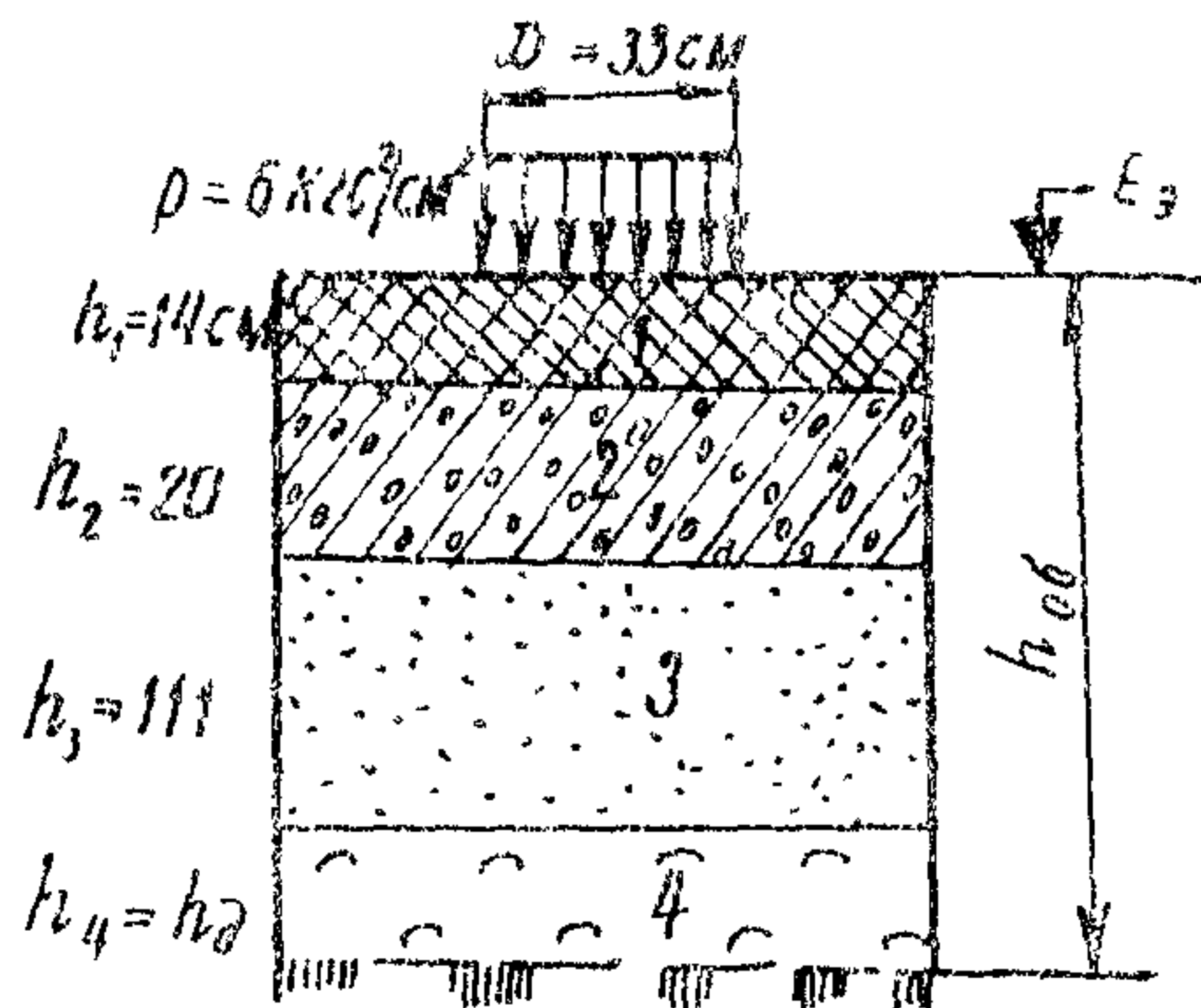
Схема дорожной конструкции для определения E_{обш}
