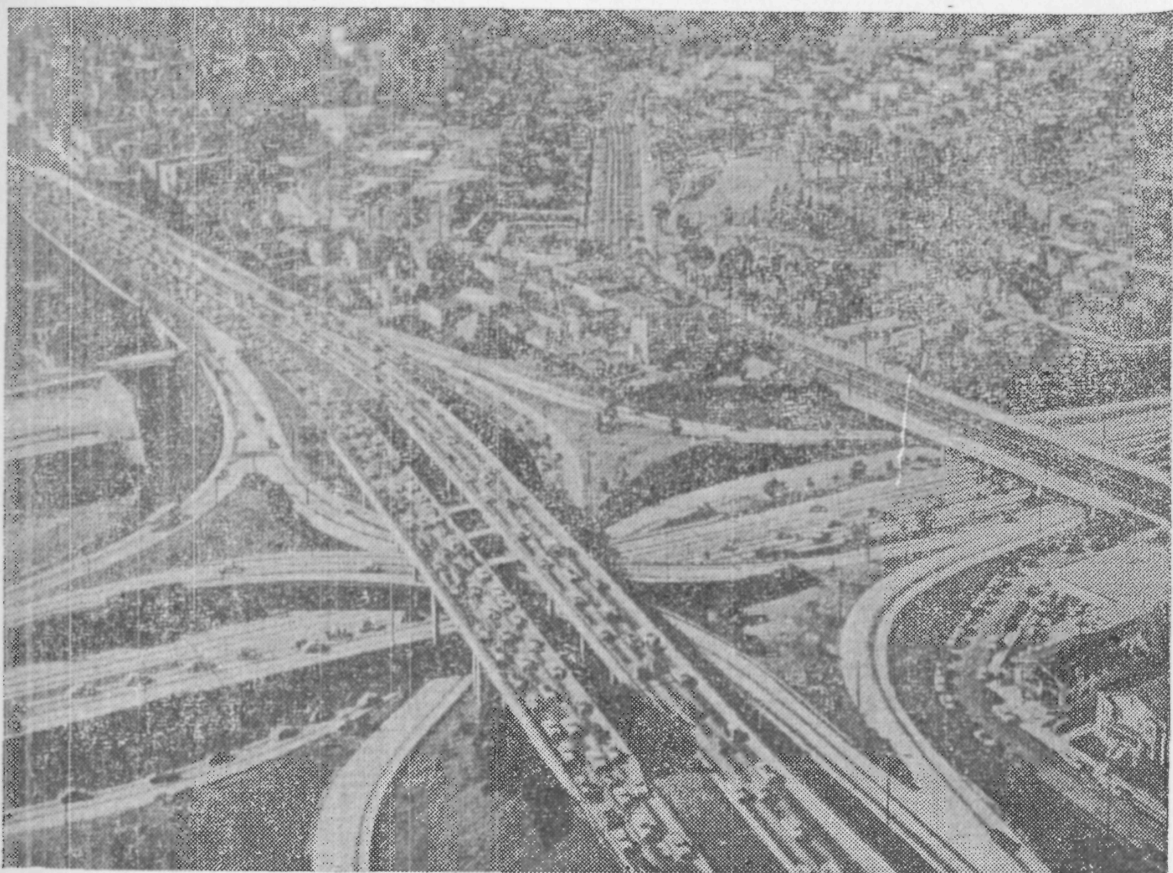
Рис. 10. Пересечение левоповоротного типа в четырех ярусах
