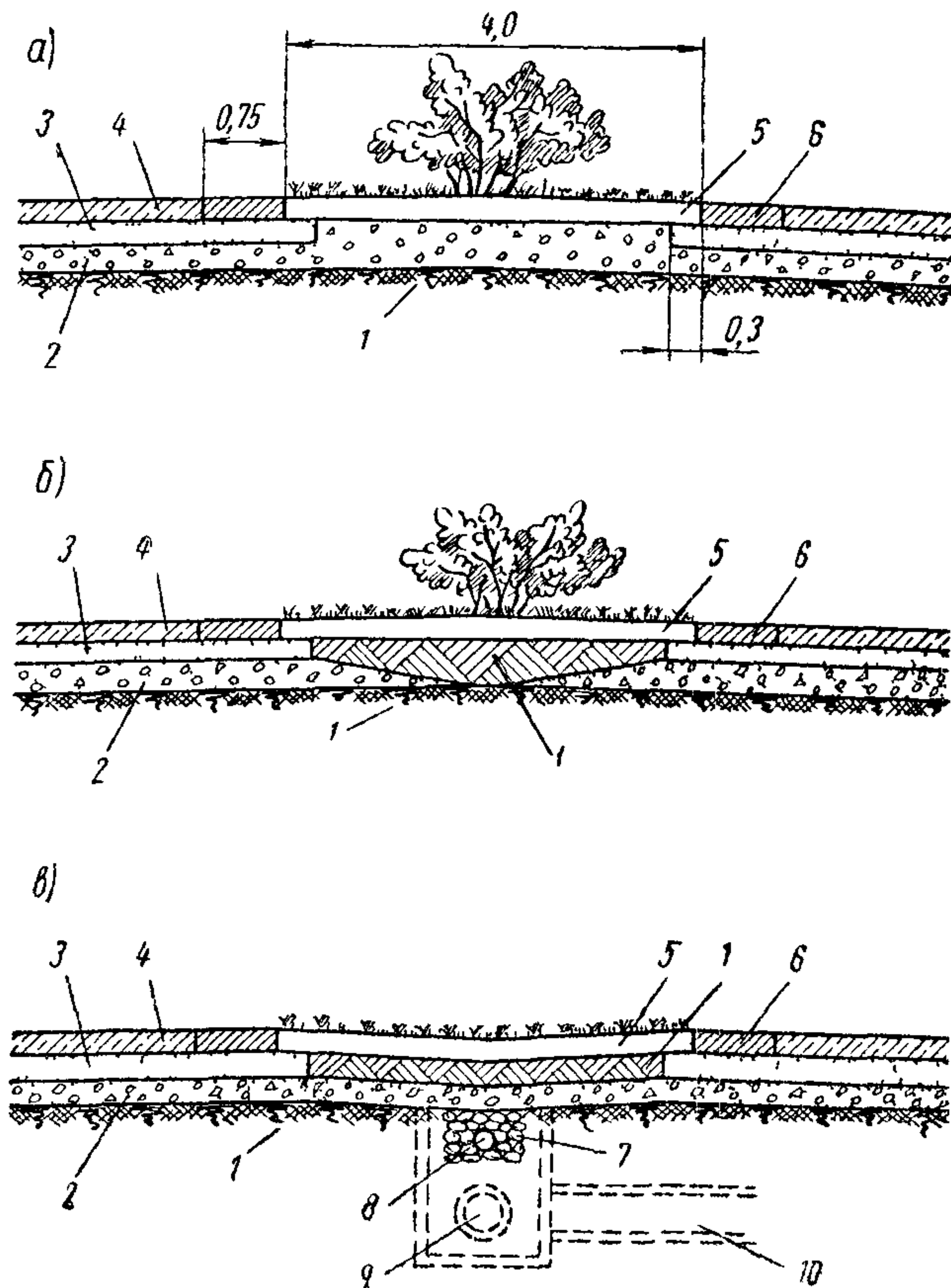
Рис 6 Конструкция разделительной полосы и схема водоотвода
