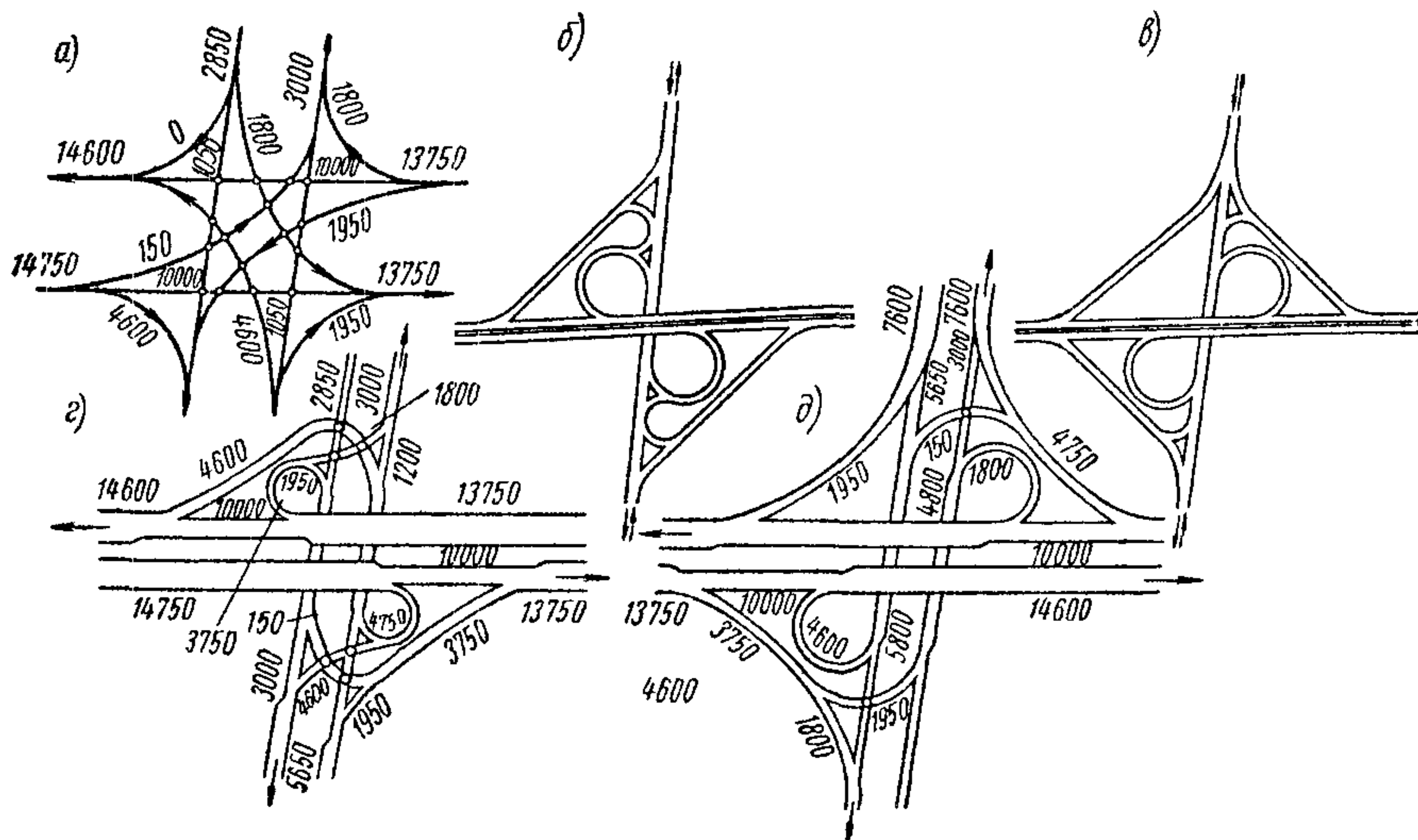
Рис 12 Варианты пересечения по типу неполного клеверного листа: а—схема интенсивности движения в разных направлениях, б—первый вариант пересечения, в—второй вариант пересечения, г—эпюра интенсивности движения по первому варианту, д—то же, по второму варианту пересечения
