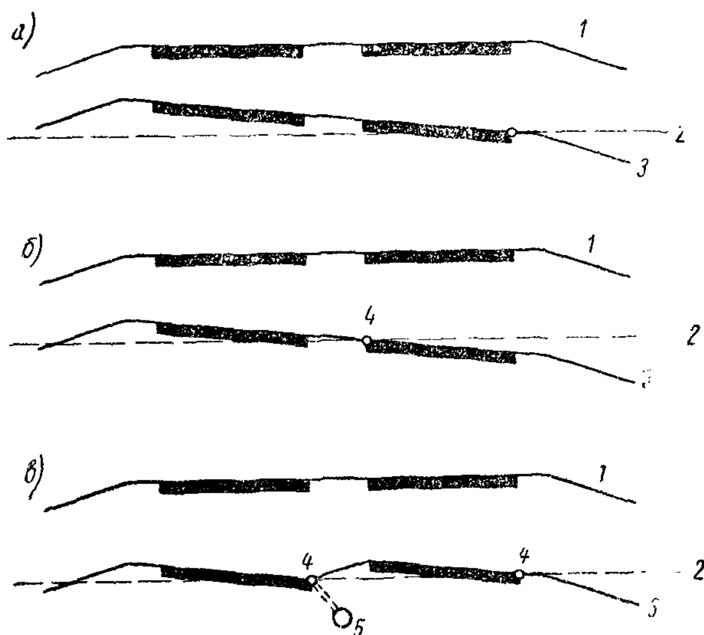
Рис. 3. Конструкция поперечного профиля автомагистрали при устройстве виража:
