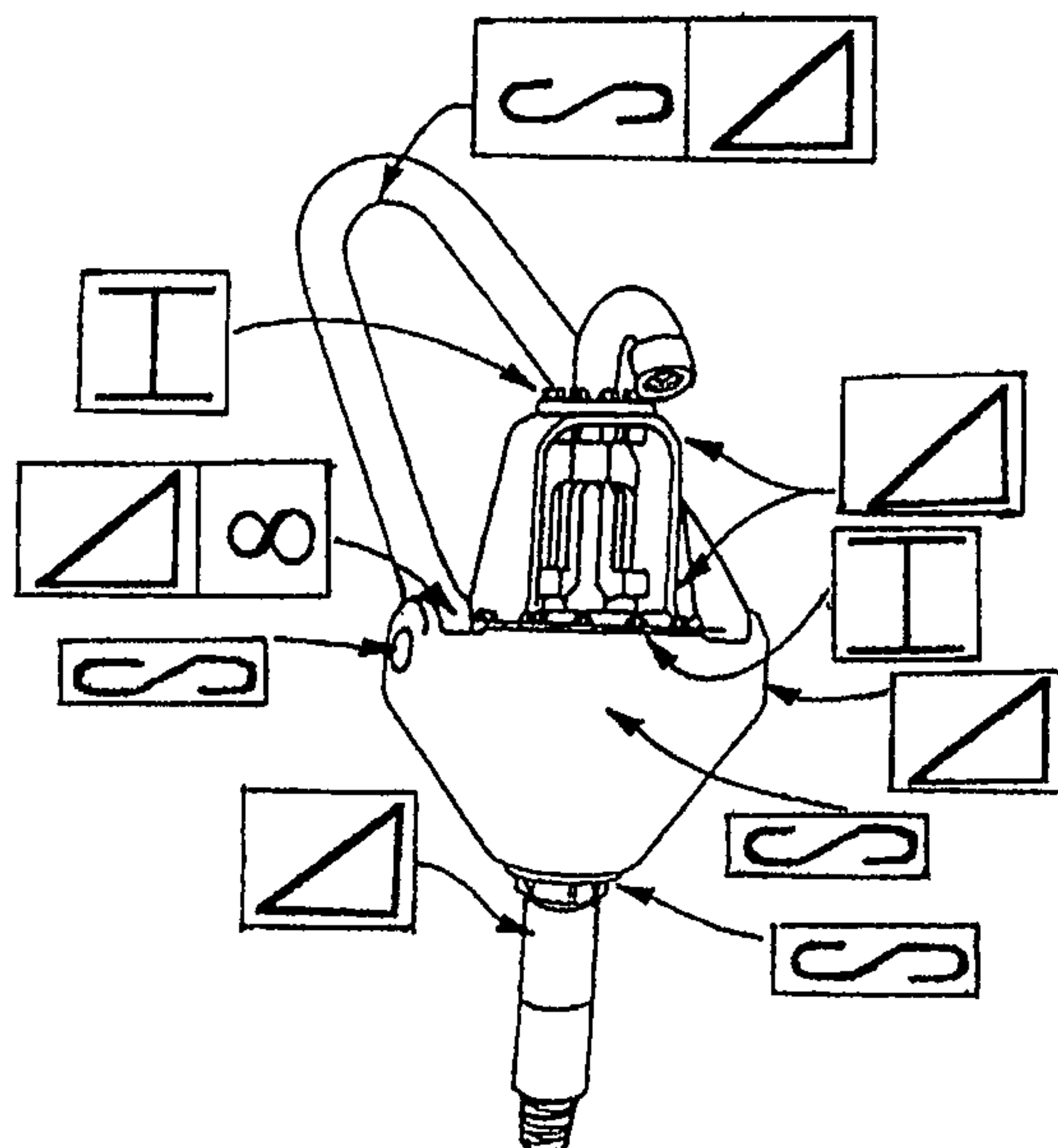
Рис. 5.7. Вертлюг
