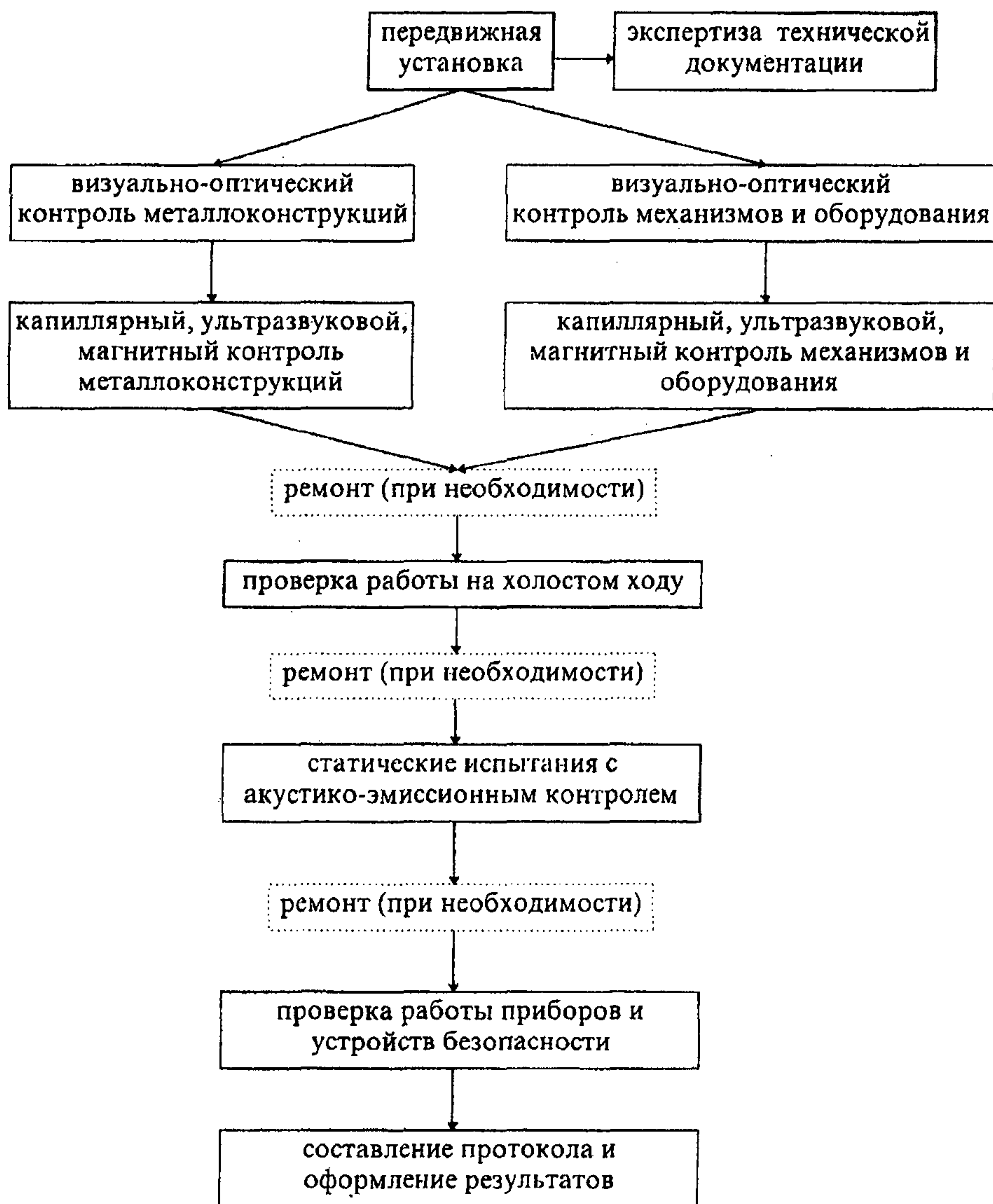
Рис. 2.1. Порядок технического диагностирования передвижных установок
