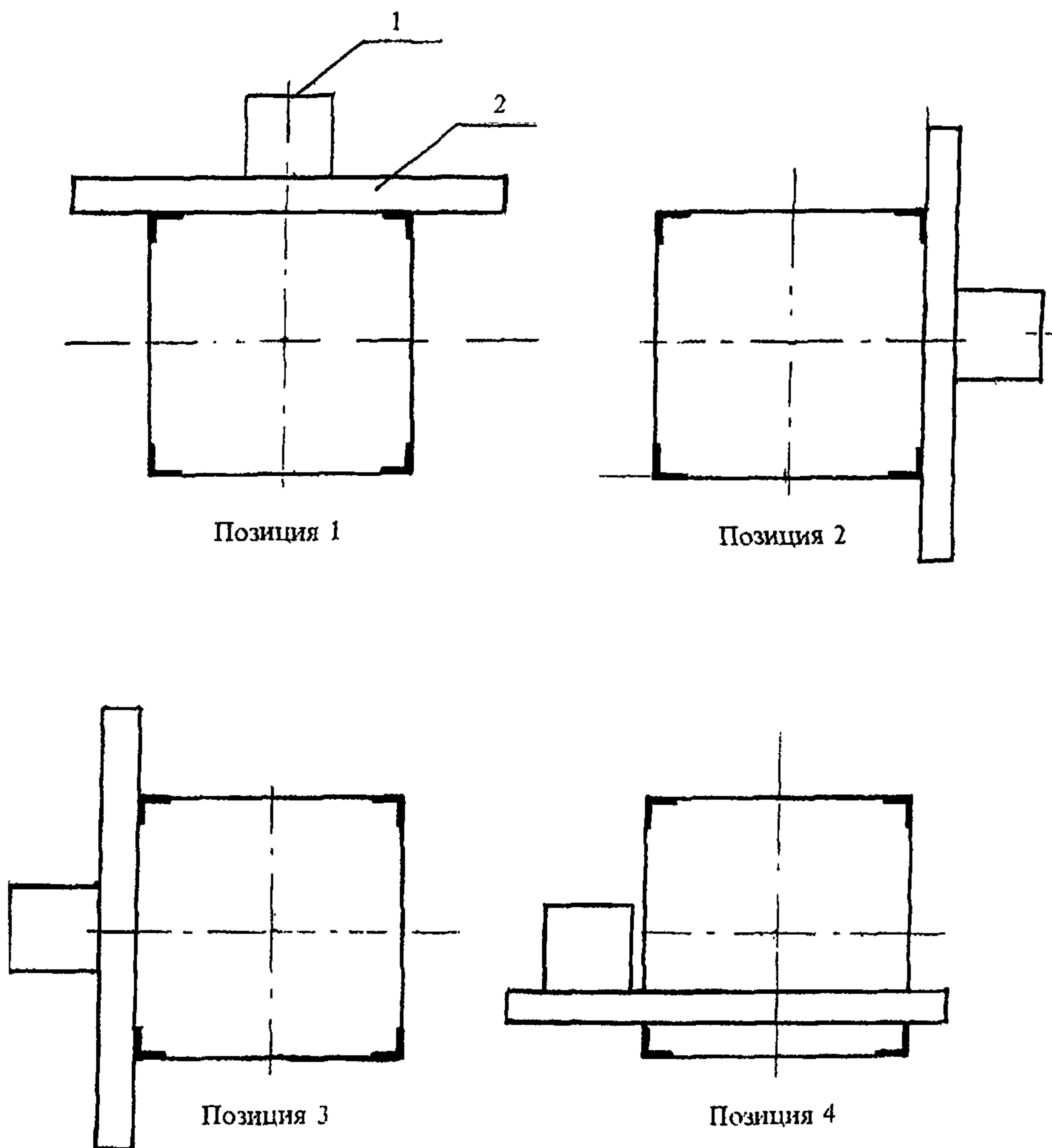
Рис. 8.2: 1 — оптический квадрант; 2 — поверочная линейка
