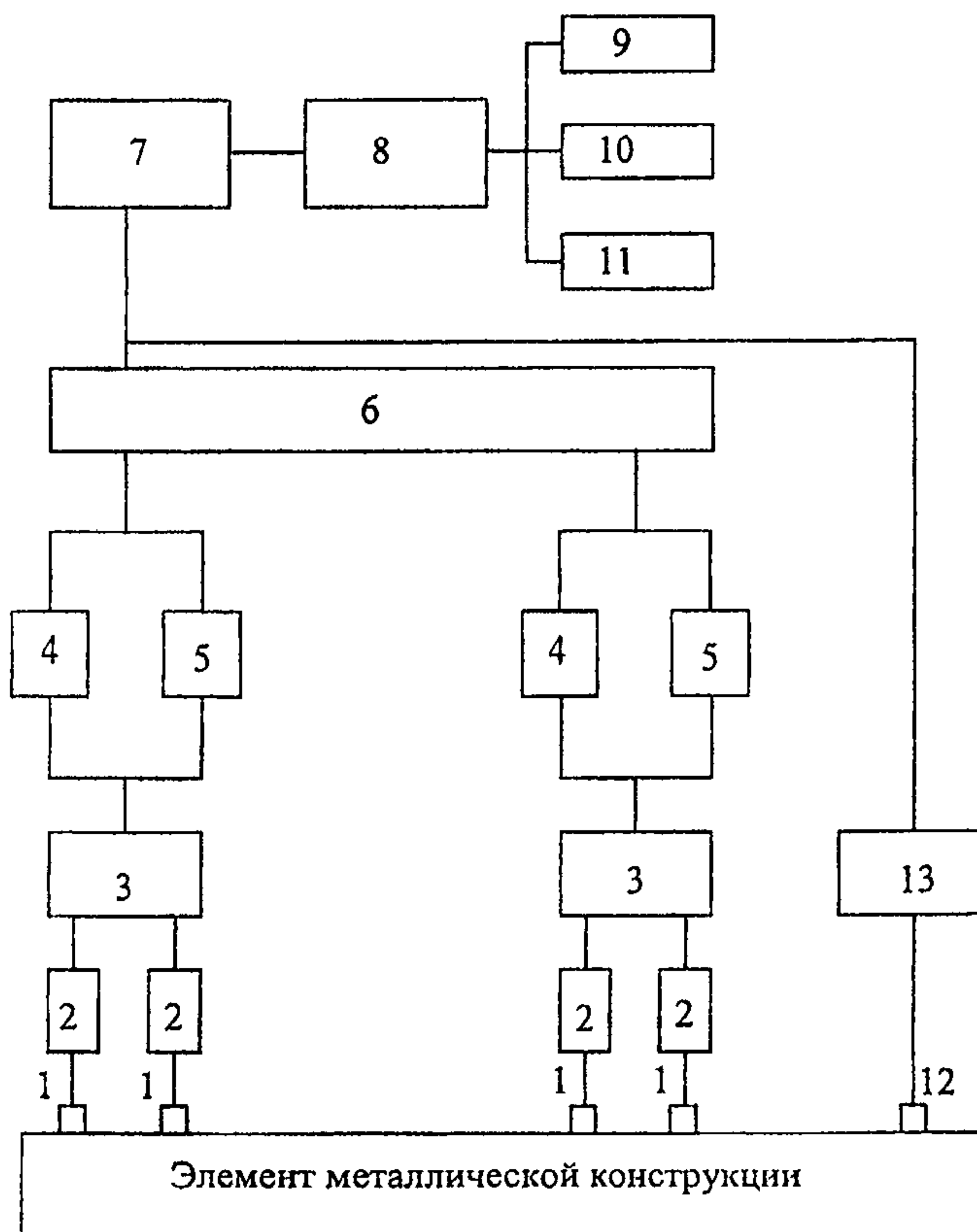
Рис. 6.2.1. Структурная схема АЭ диагностического комплекса:
