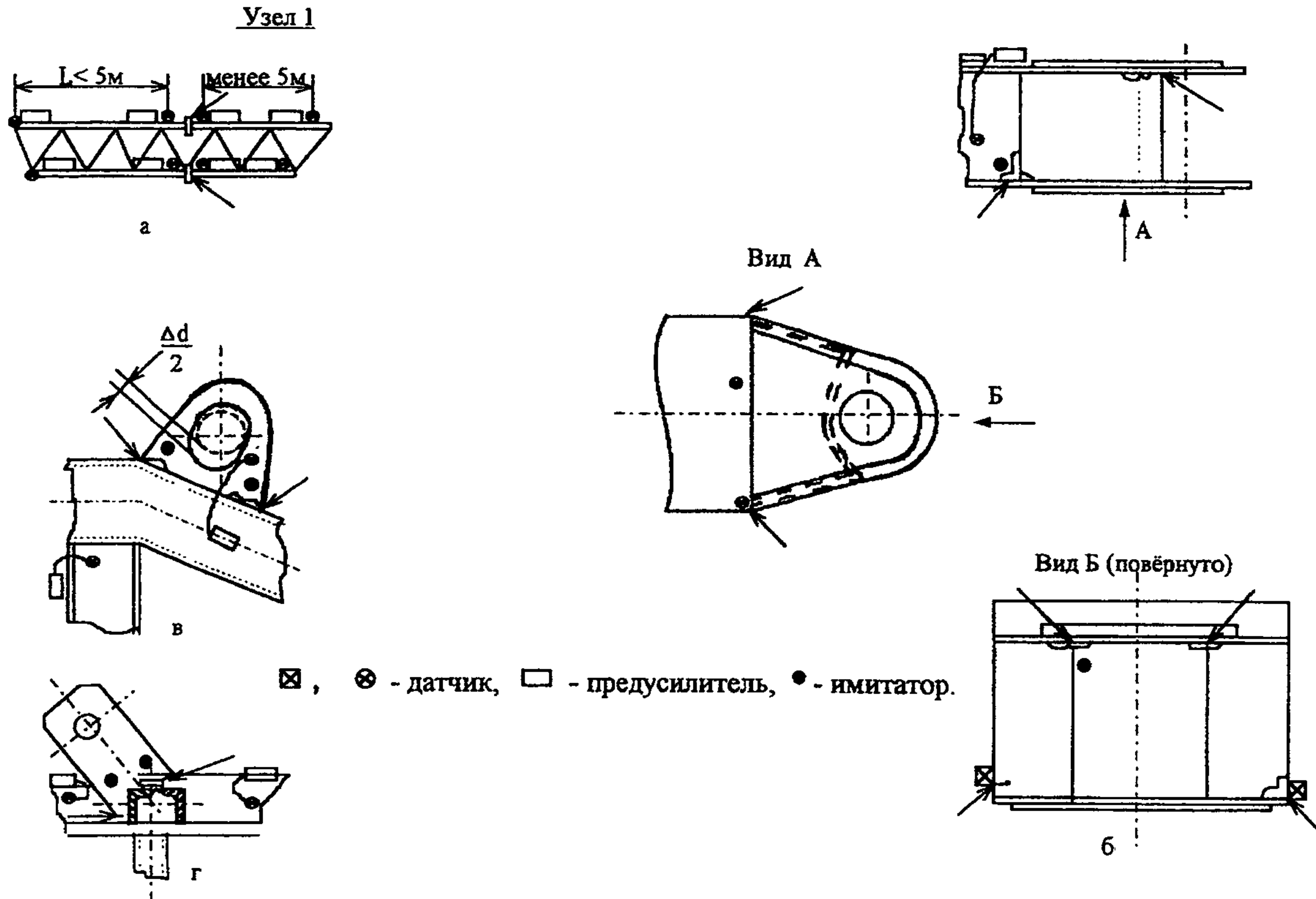
Рис. 6.5.1. Примеры установки АЭ-датчиков и предусилителей на конструкции подъемника: а — мачта; б — рама шасси; в, г — узлы конструкции
