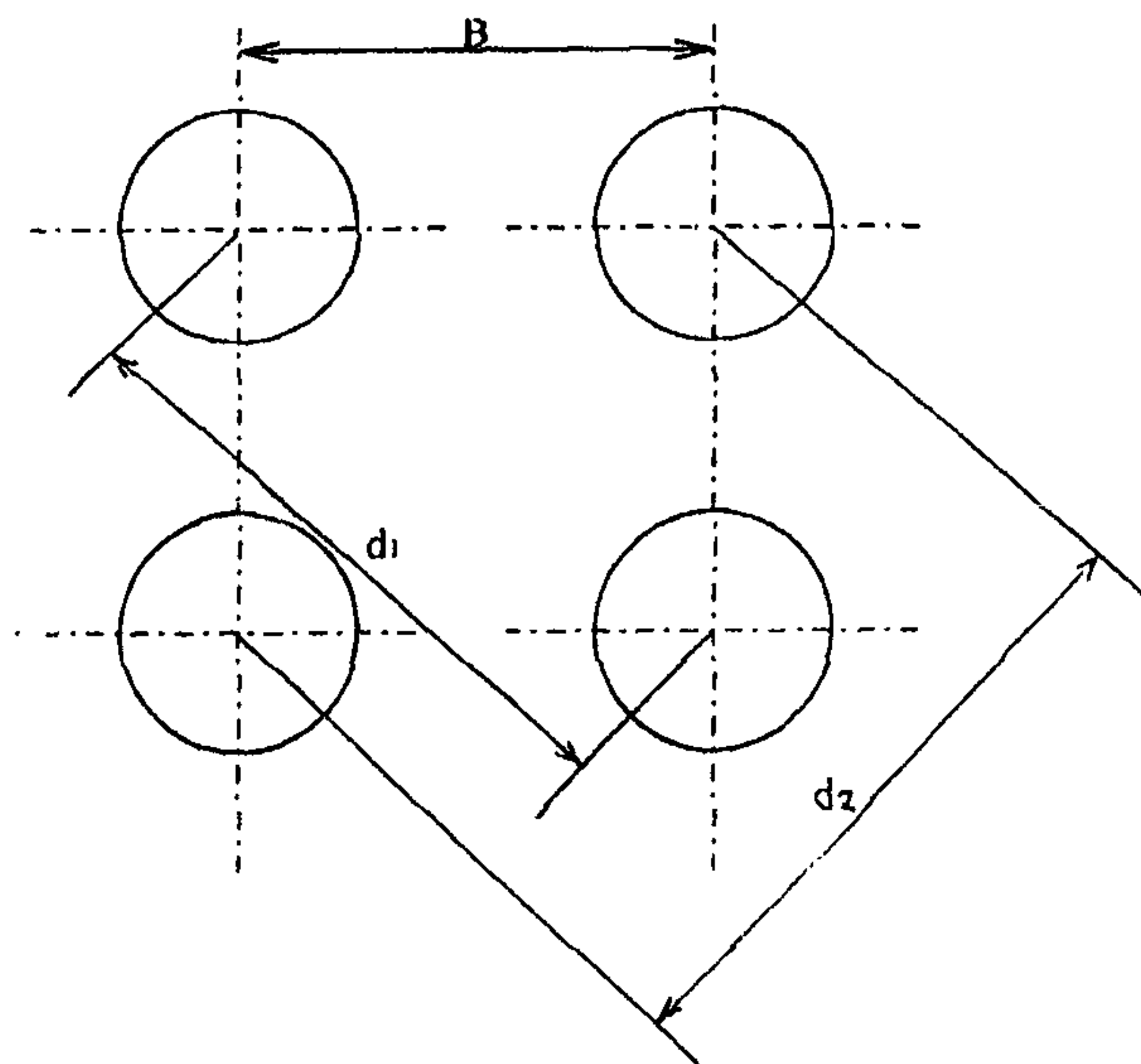
Рис. 1. Поперечное сечение мачты
