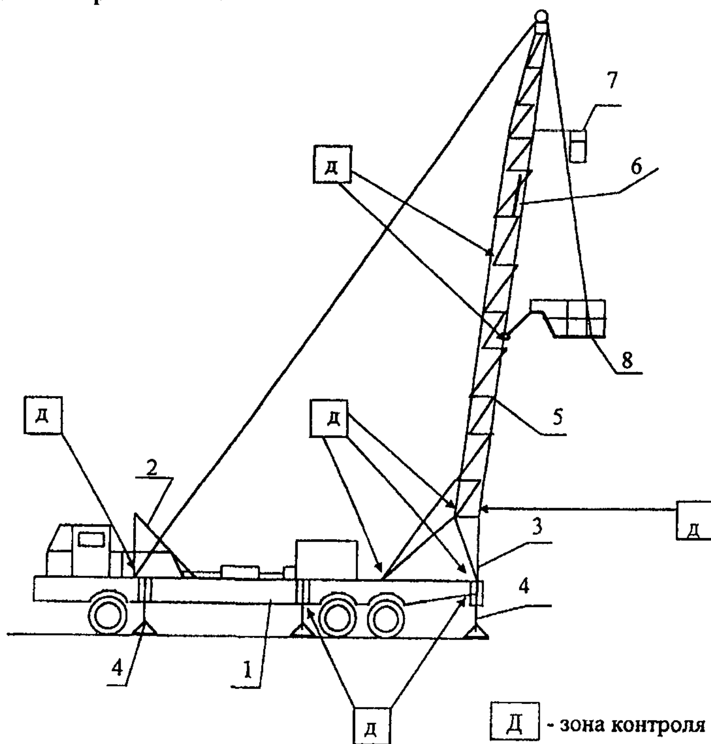
Рис. 6.3.1. Подъемник для капитального и текущего ремонта скважин:
