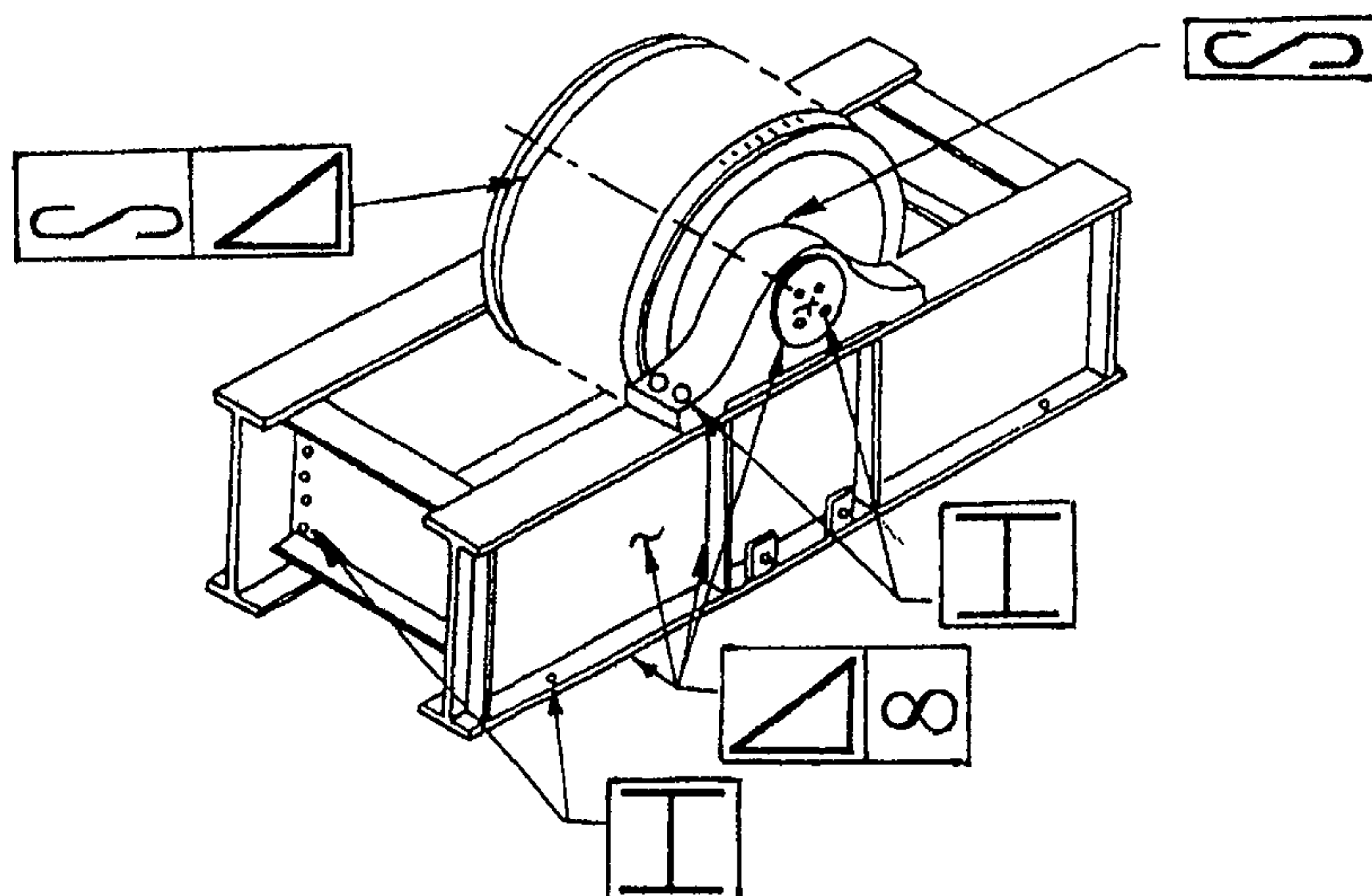
Рис. 5.3. Кронблок
