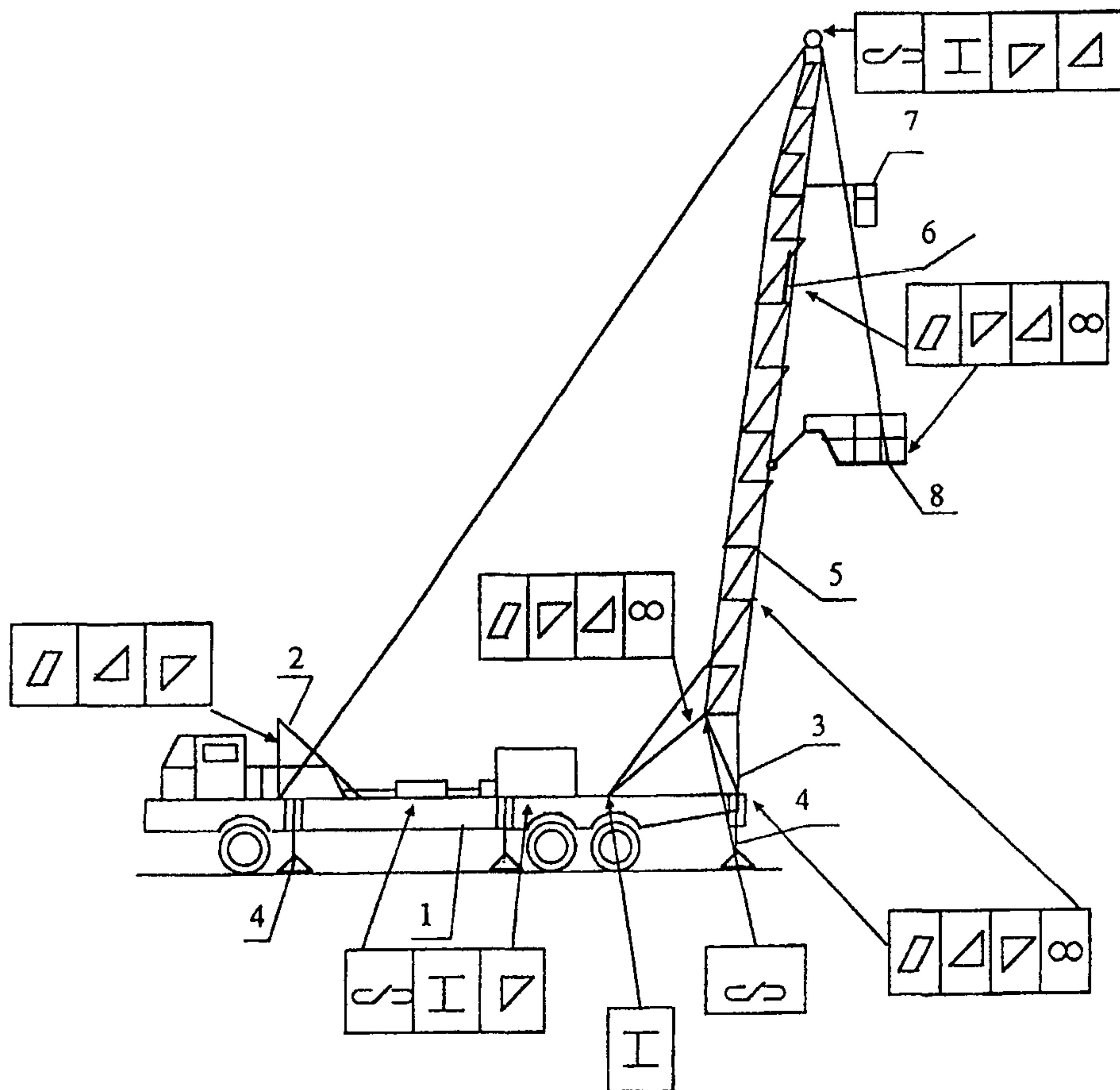
Рис. 5.2. Подъемник для капитального и текущего ремонта скважин:
