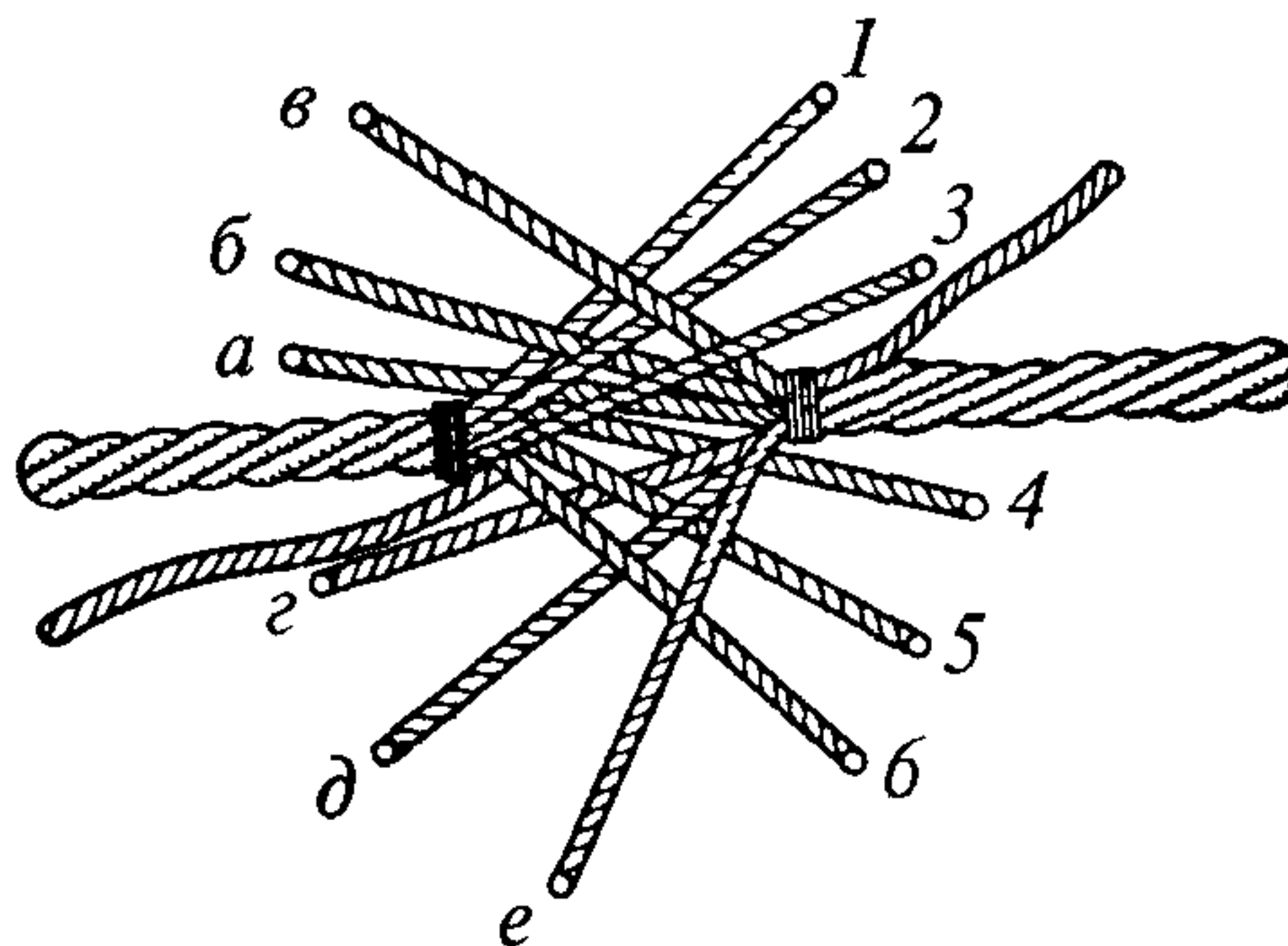
Рис. 48. Чередование прядей при счалке канатов
