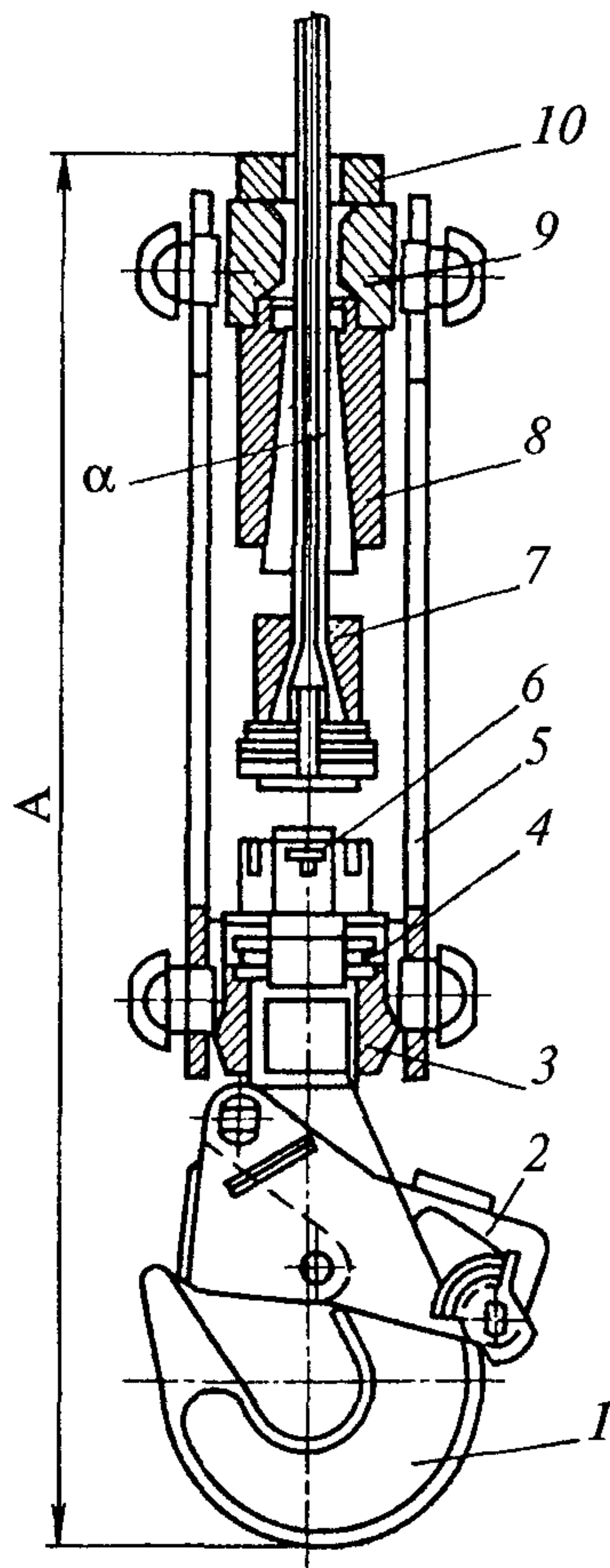
Рис. 33. Устройство прицепное типа УПЗ
