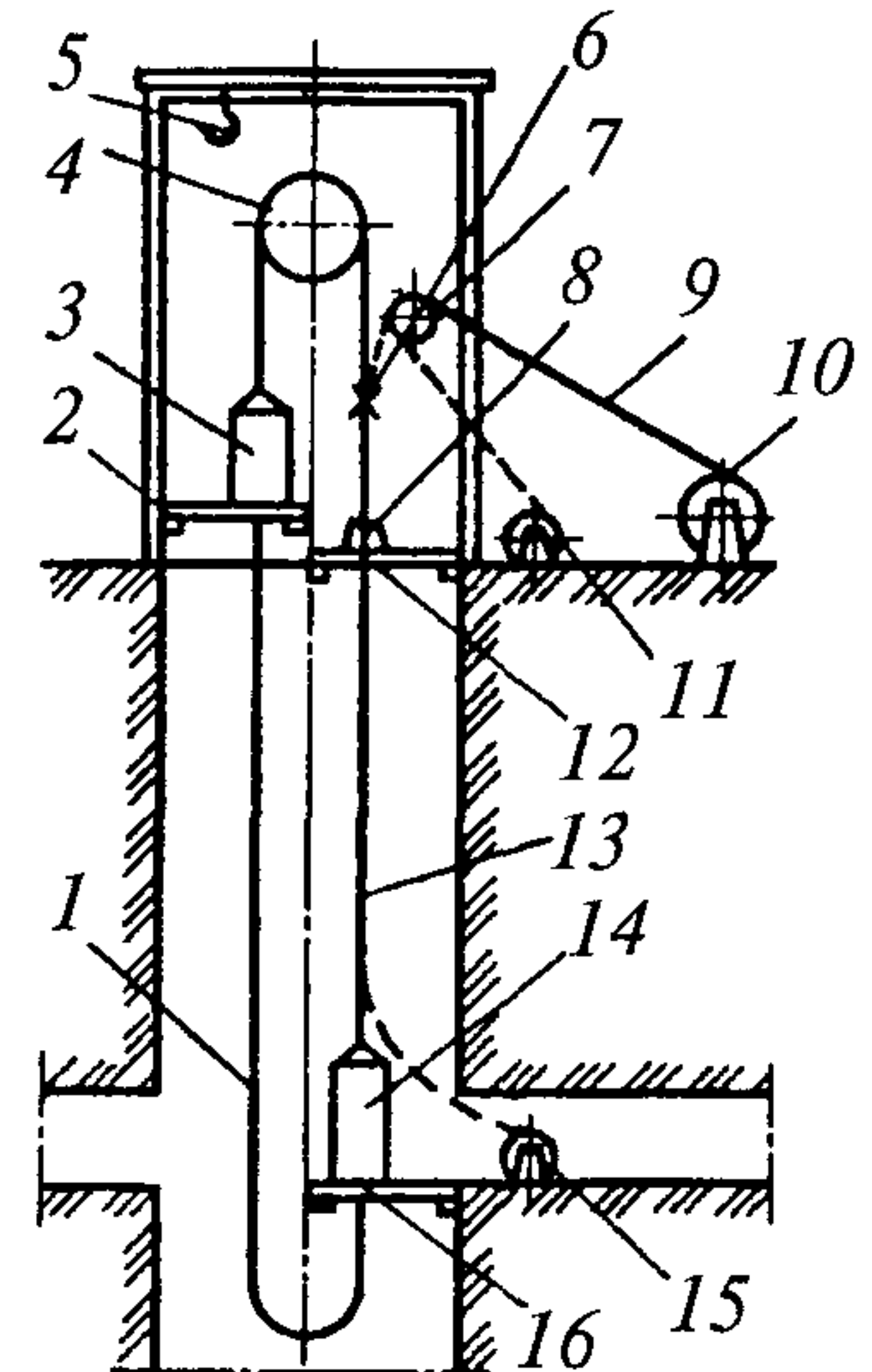
Рис. 22. Схема замены головного каната на многоканатной подъемной машине
