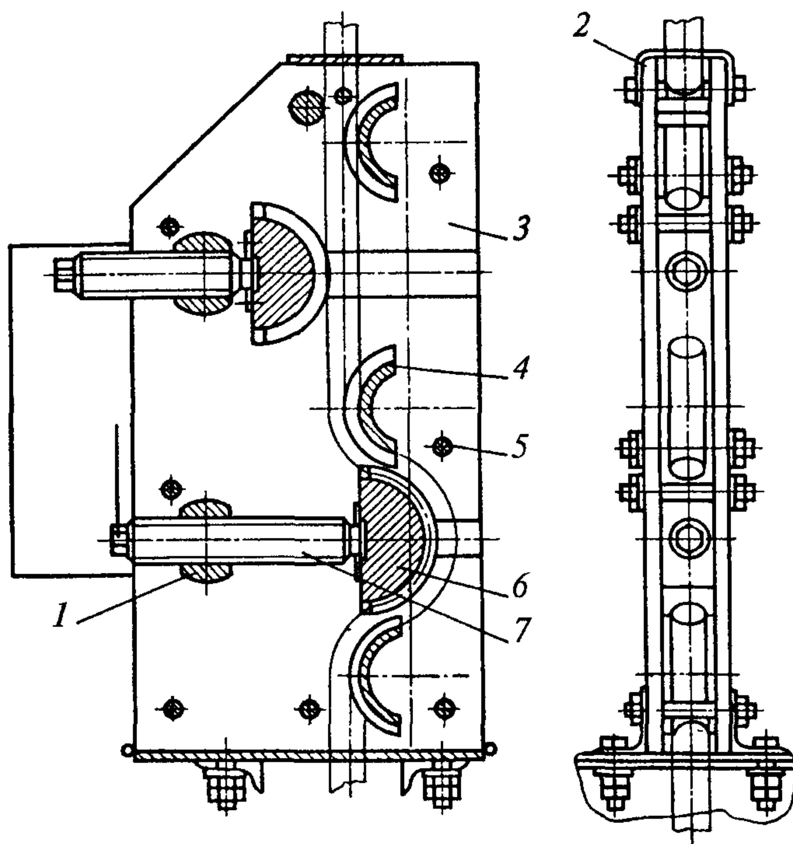
Рис. 38. Амортизатор
