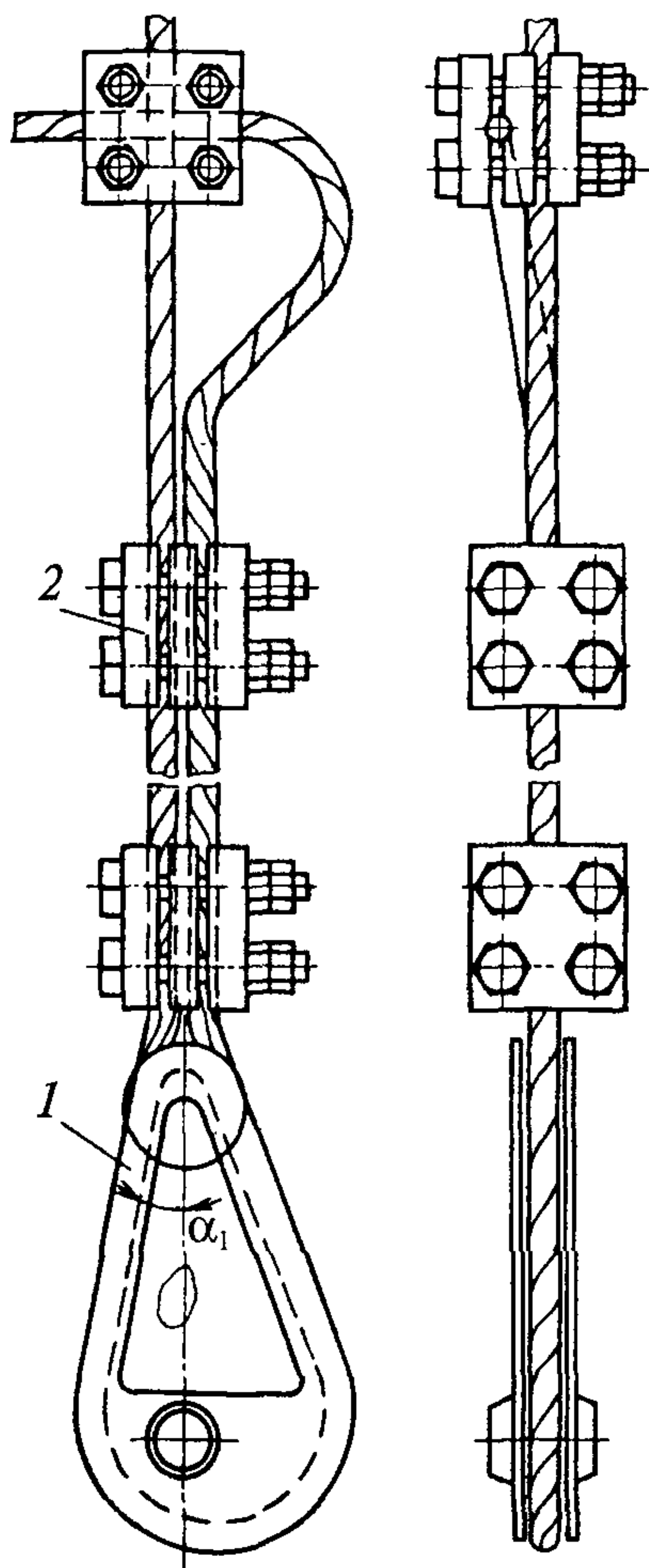
Рис. 31. Грушевидный несимметричный коуш с зажимами конструкции МакННН
