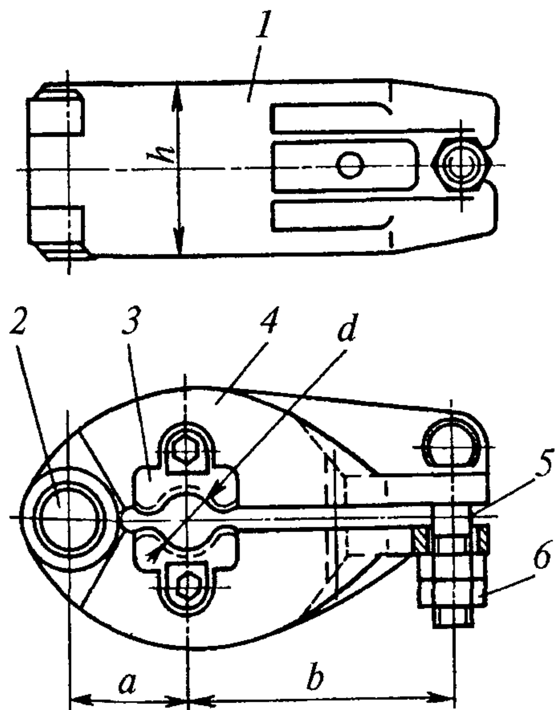
Рис. 11. Быстроразъемный грушевидный зажим
