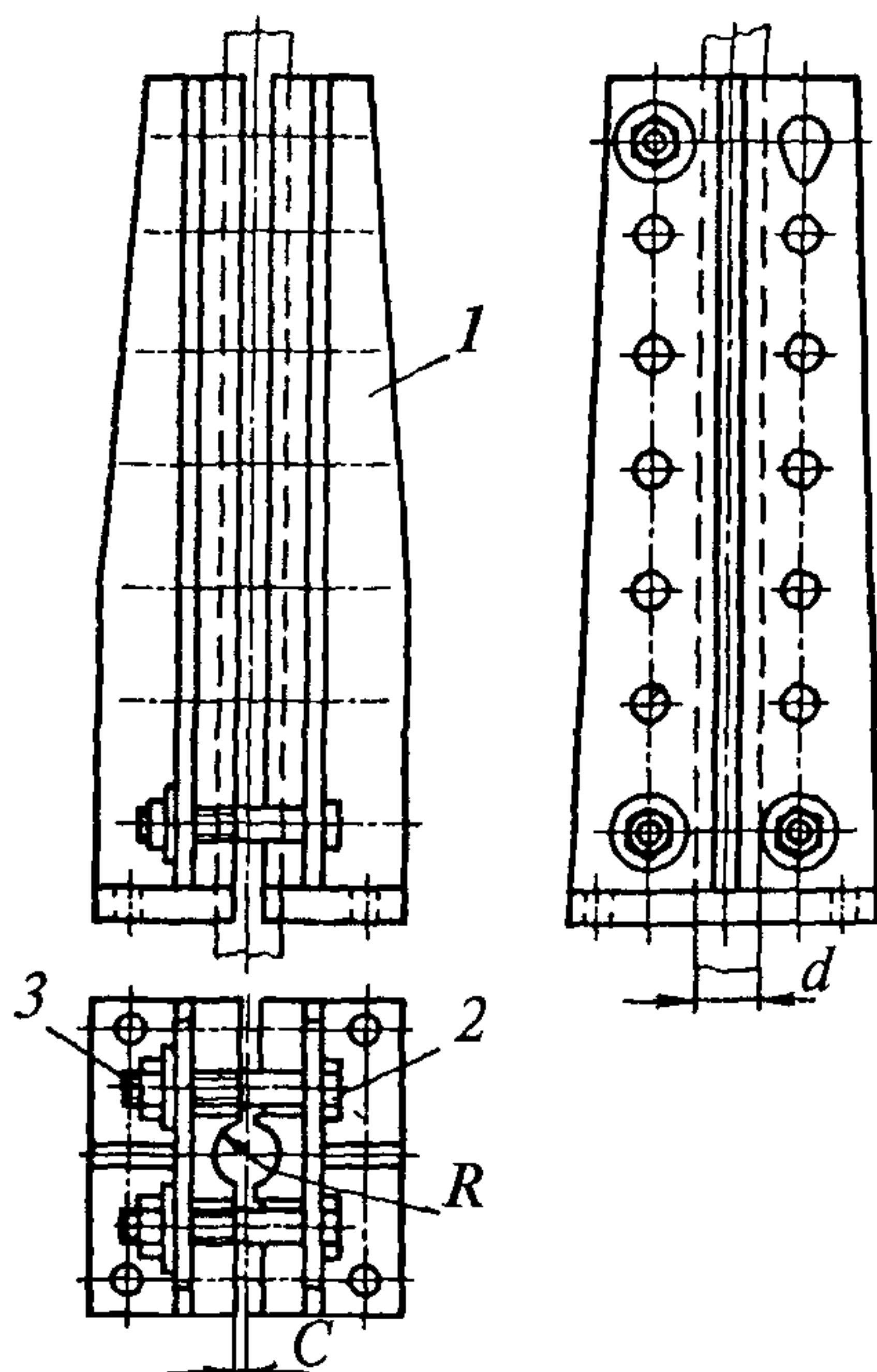
Рис. 10. Многоболтовой зажим для крепления канатов
