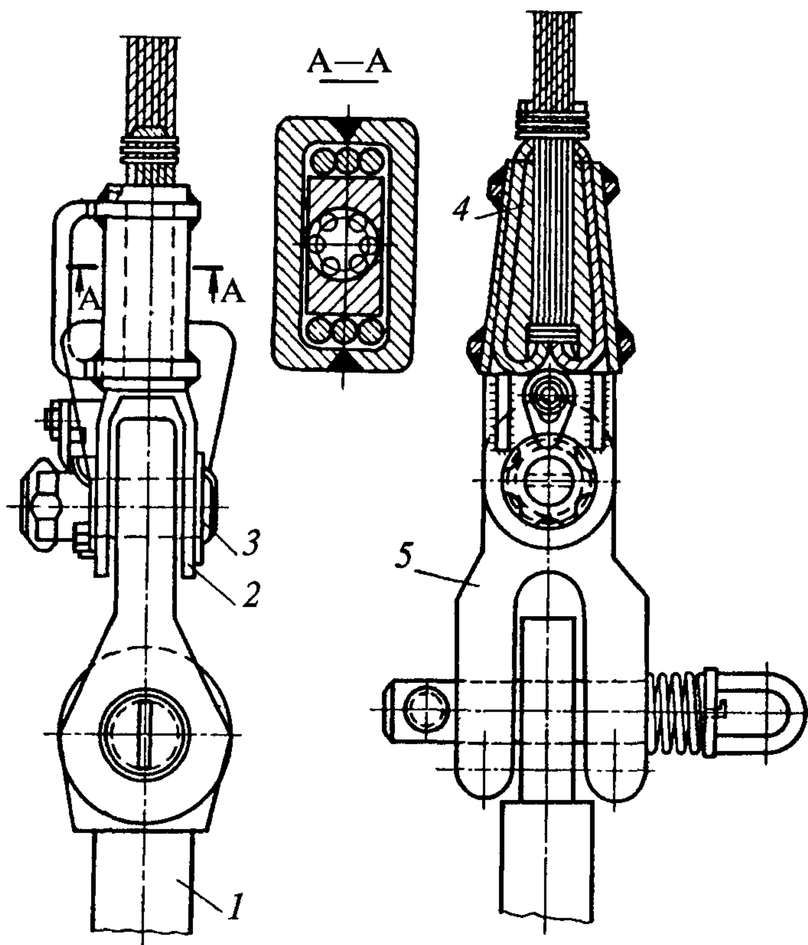
Рис. 35. Устройство прицепное МПЛ-1
