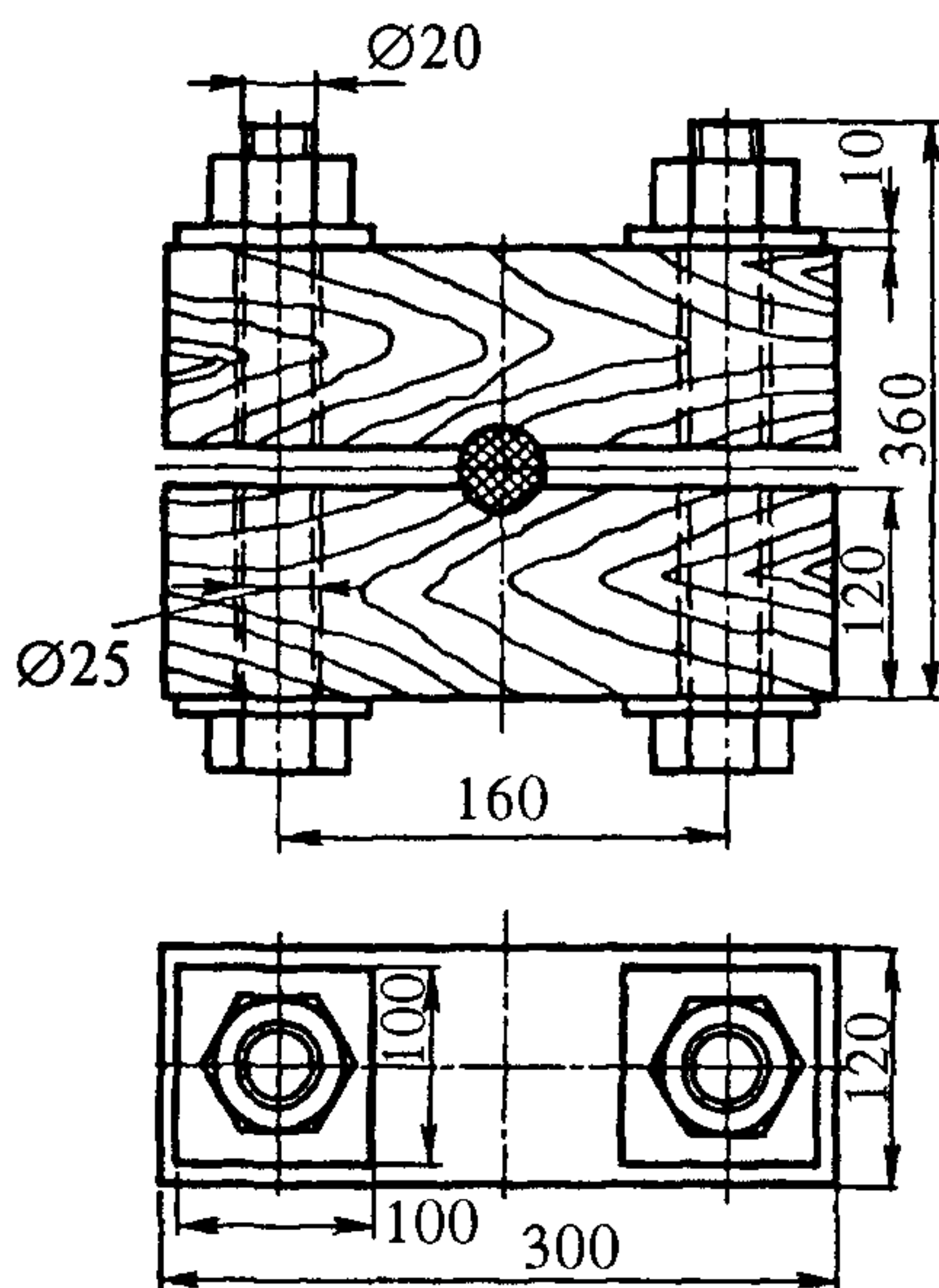
Рис. 12. Деревянный зажим для крепления канатов
