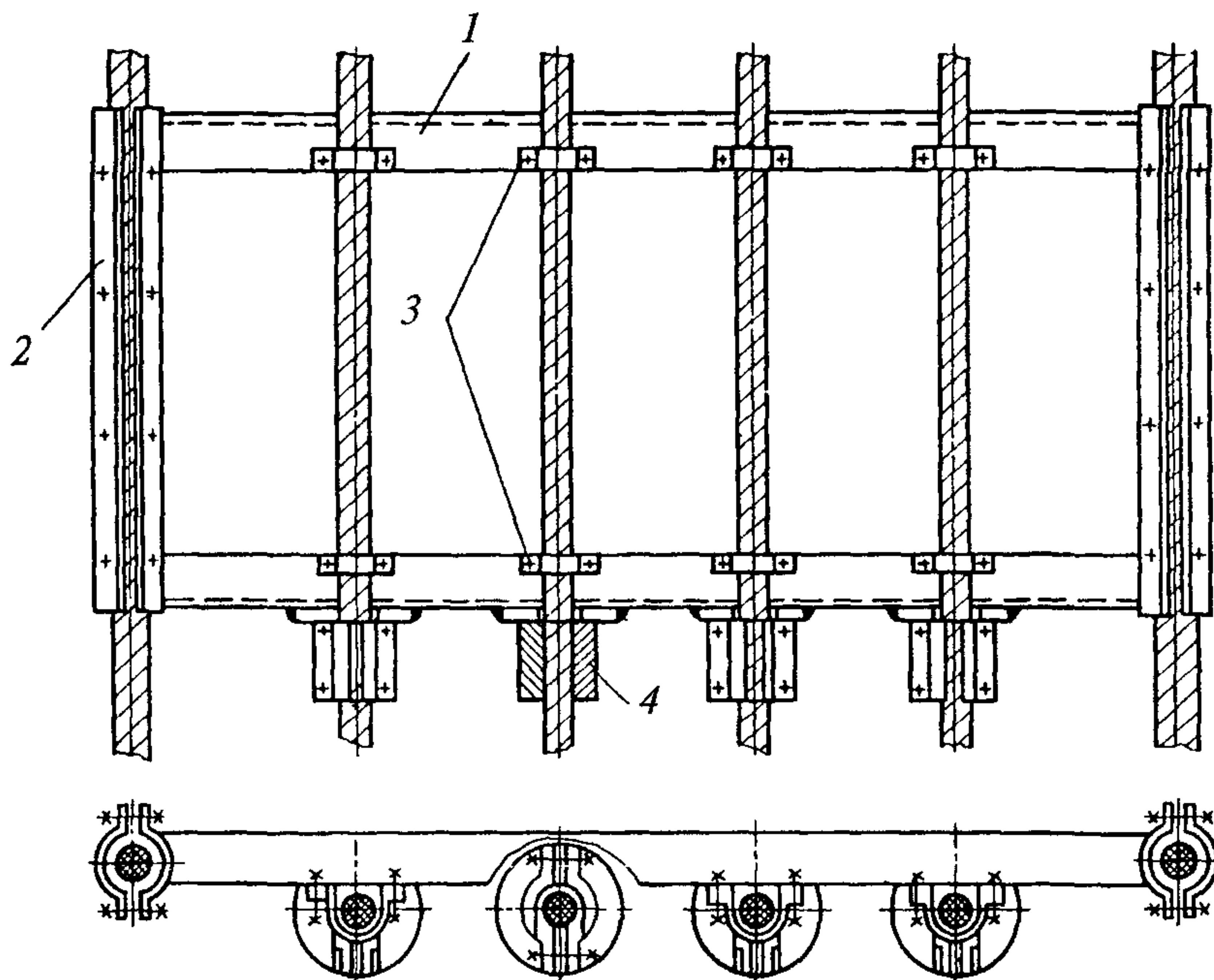
Рис. 13. Направляющая рамка головных канатов
