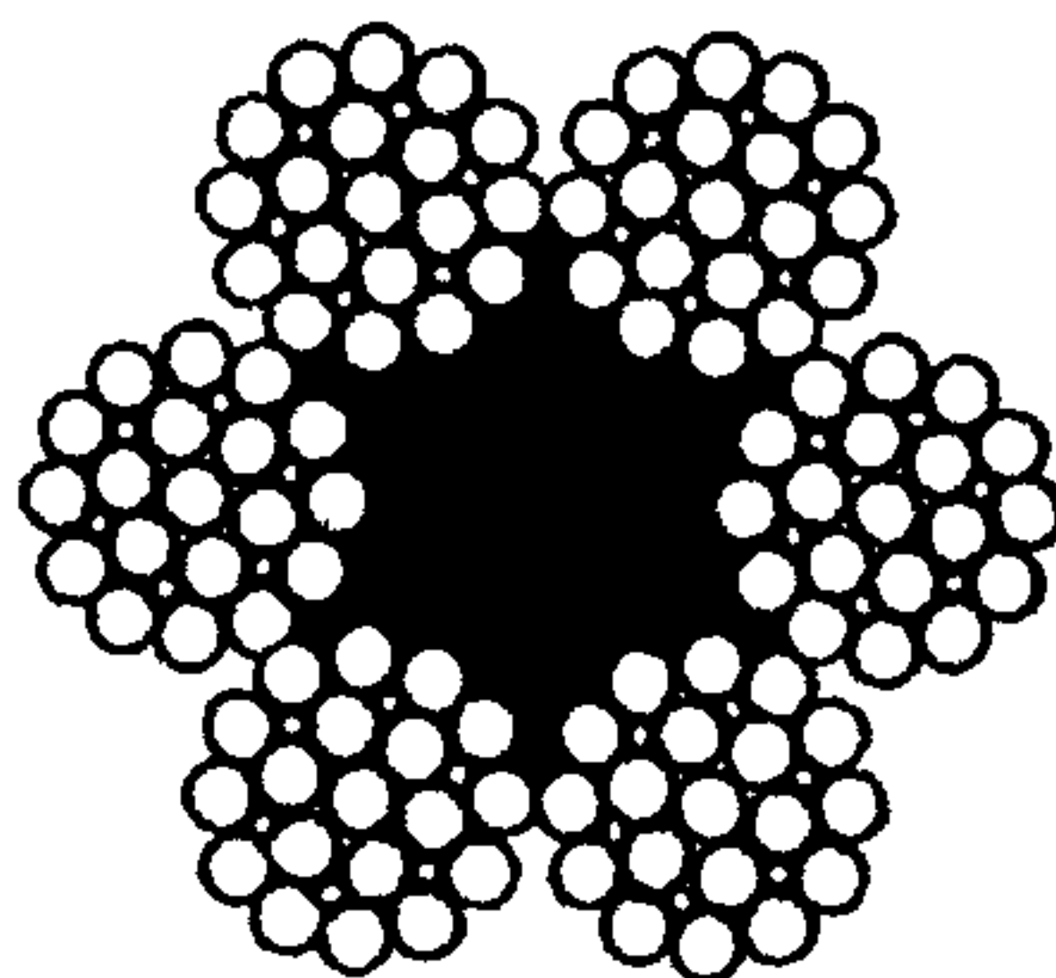
Рис. 5. Амортизационные канаты по ГОСТ 7665–80
