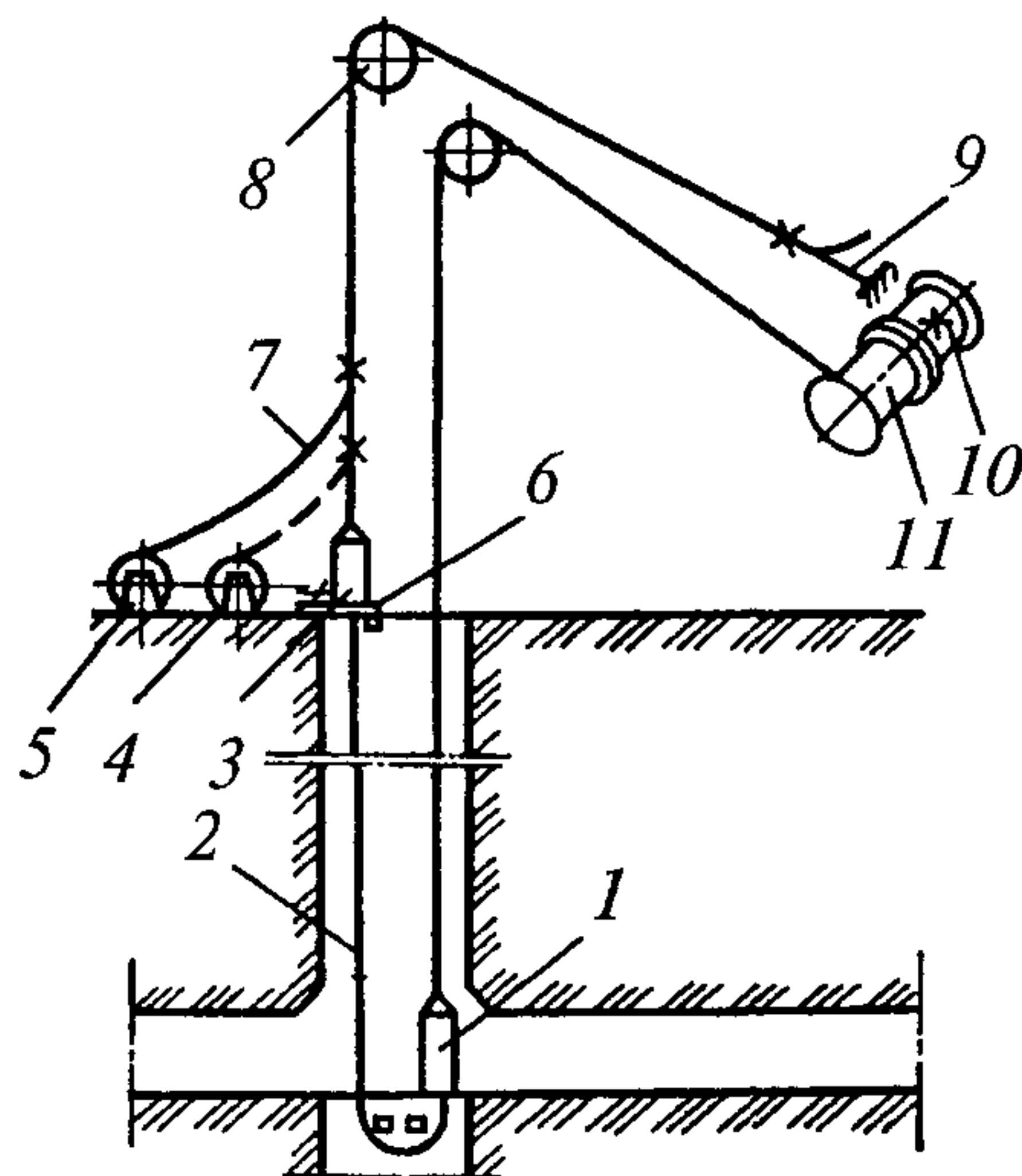
Рис. 16. Схема замены головного каната на двухбарабанной машине
