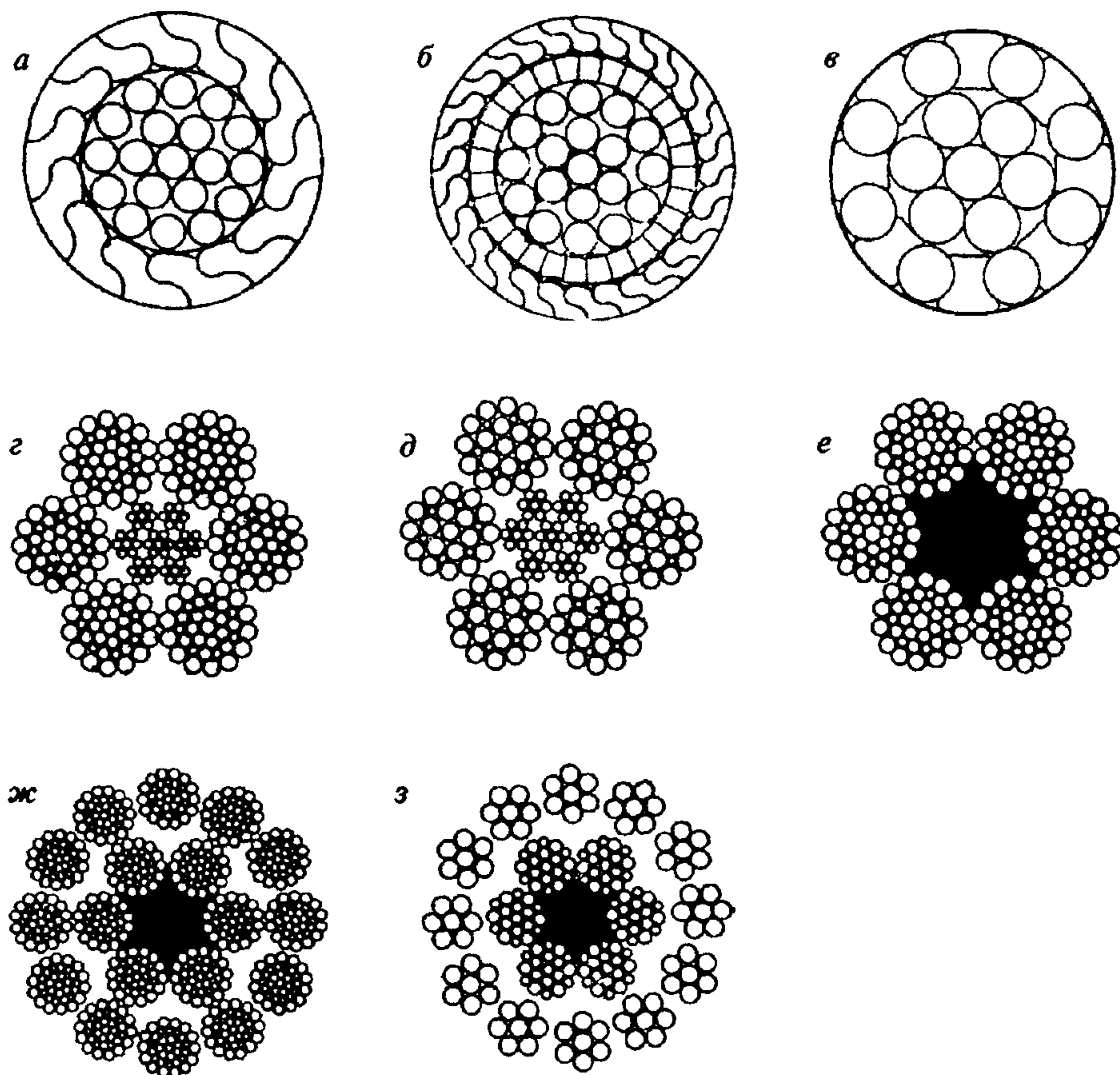
Рис. 6. Канаты проводниковые эксплуатационных и проходческих подъемов:
