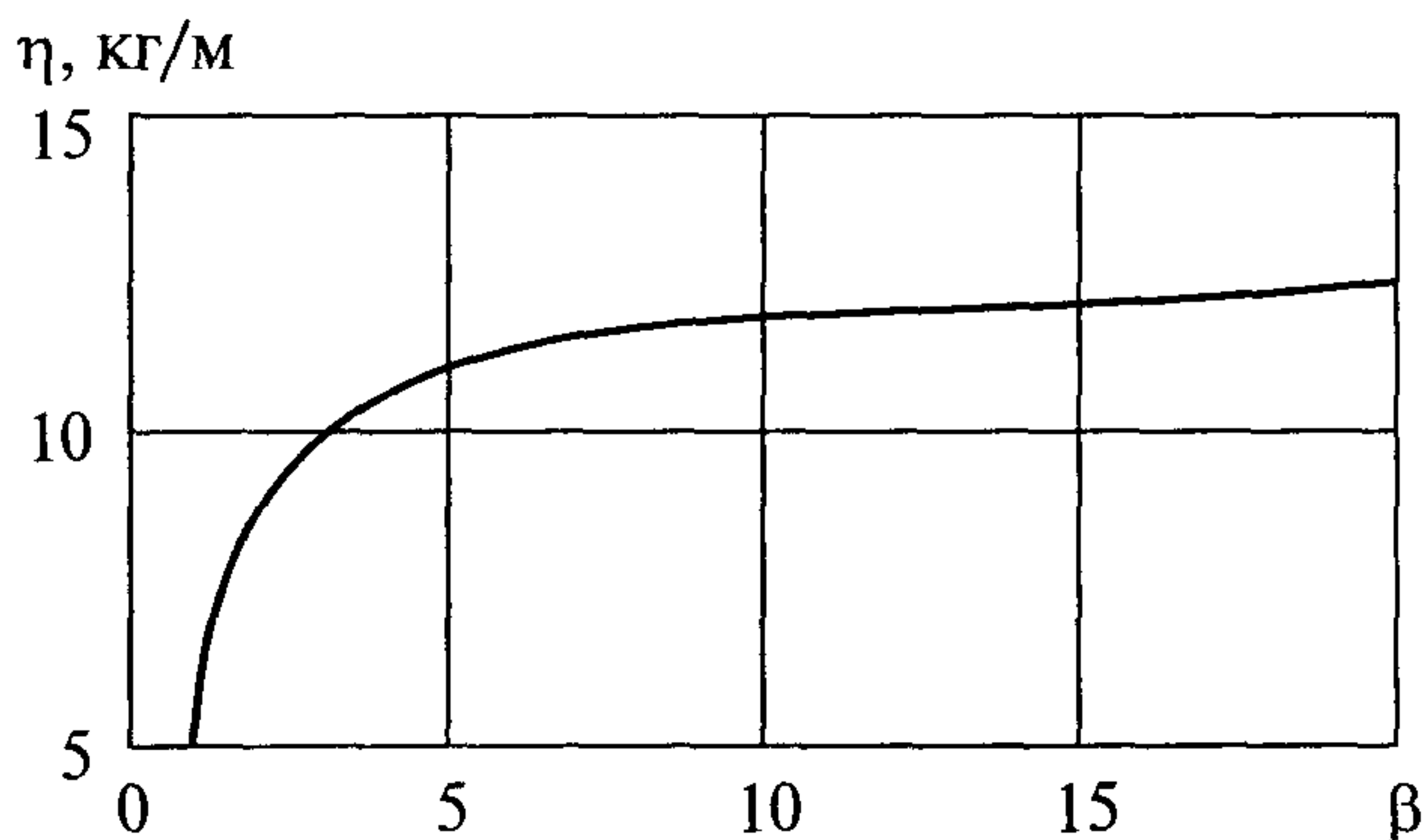
Рис. 7. Зависимости для расчета канатных проводников
