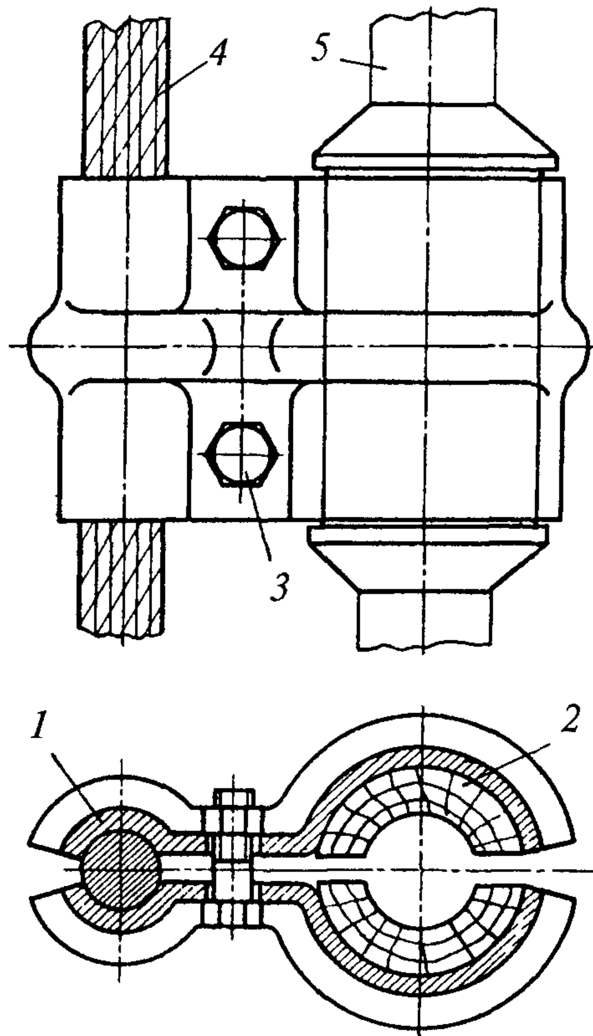
Рис. 44. Устройство для подвески кабеля
