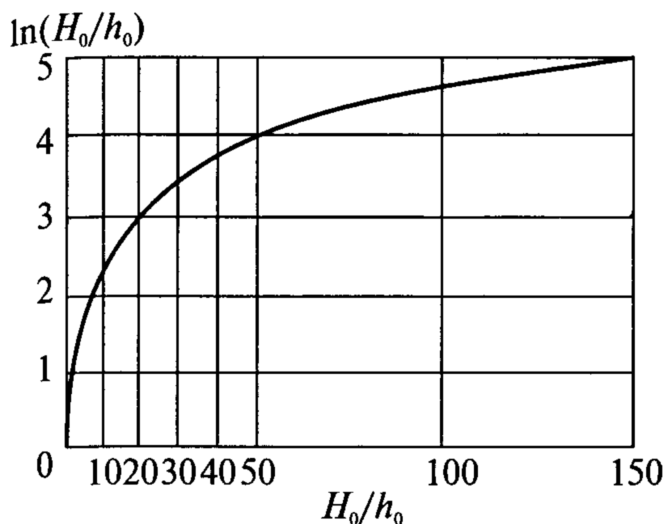
Рис. 50. График значений коэффициента \ln\left(\frac{H_0}{h_0}\right)
