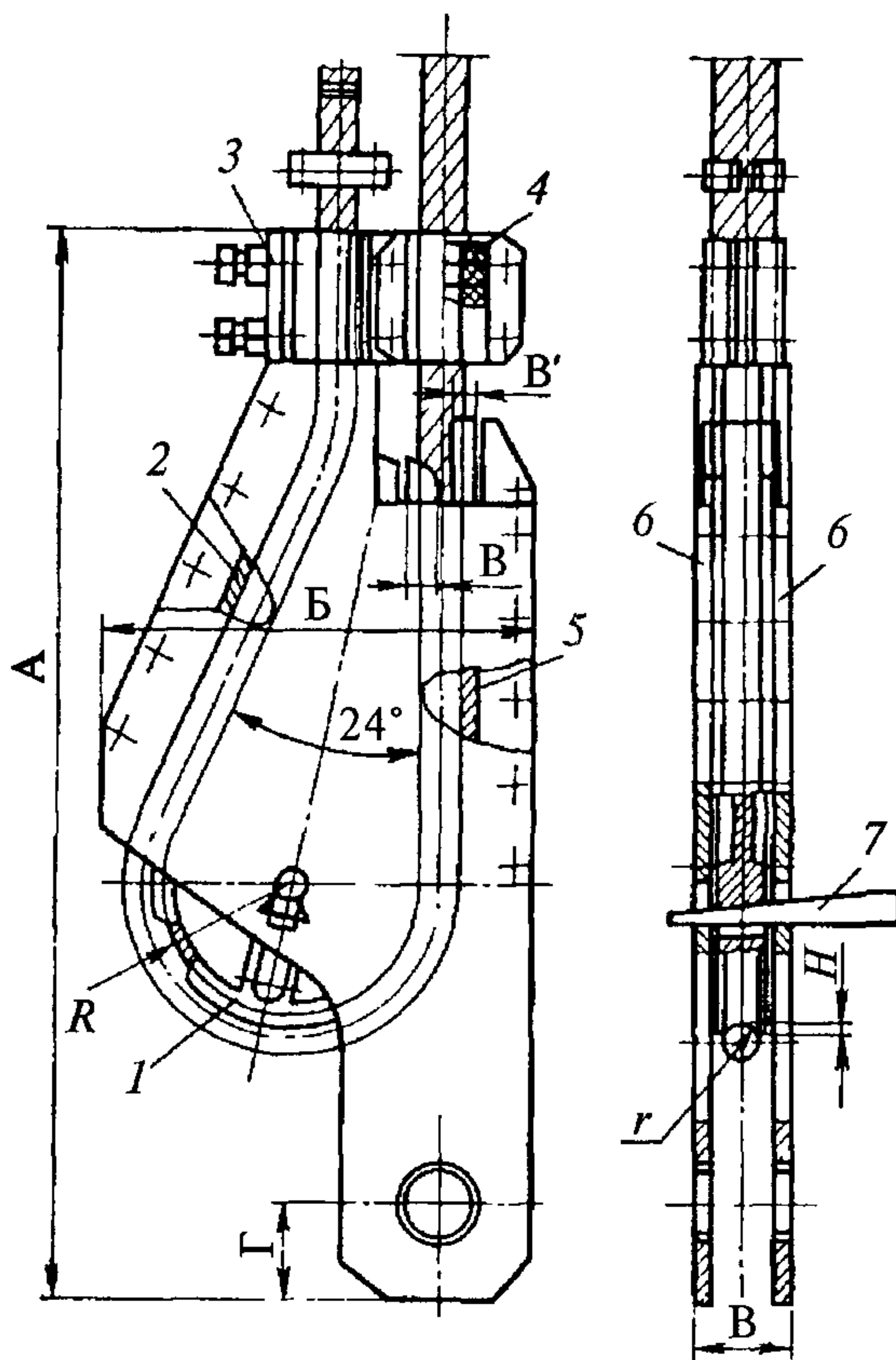
Рис. 28. Устройство прицепное типа КД
