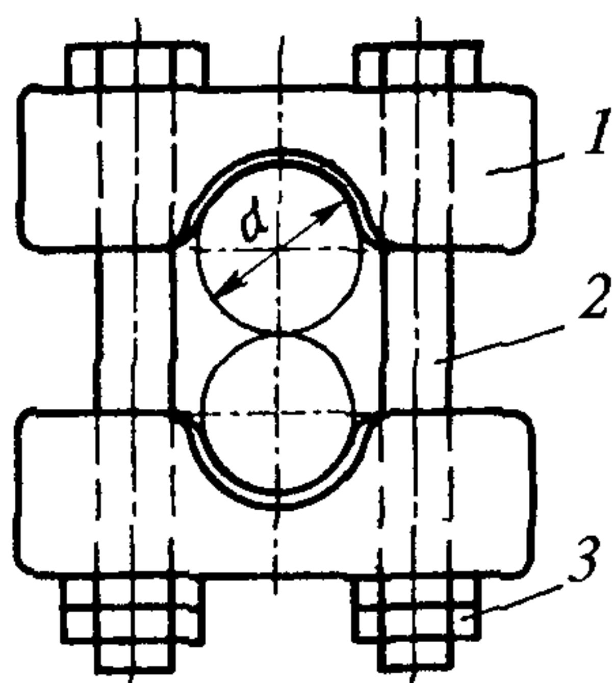
Рис. 8. Четырехболтовой зажим для соединения канатов
