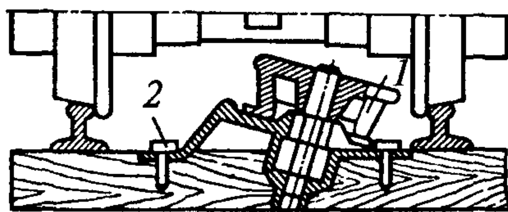
Рис. 53. Отклоняющий цилиндрический ролик 1 с креплением 2
