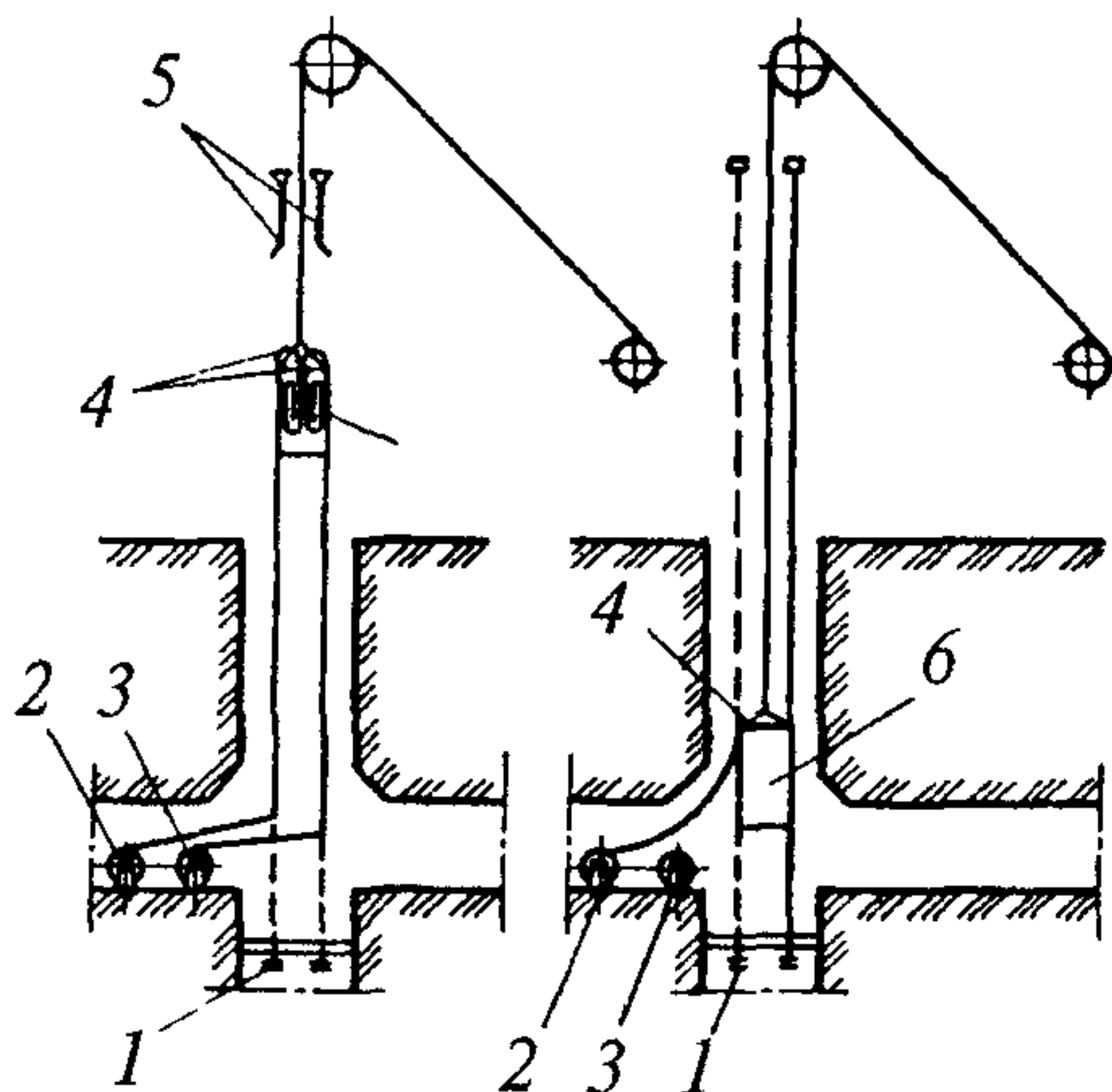
Рис. 25. Схема первоначальной навески и замены тормозного каната
