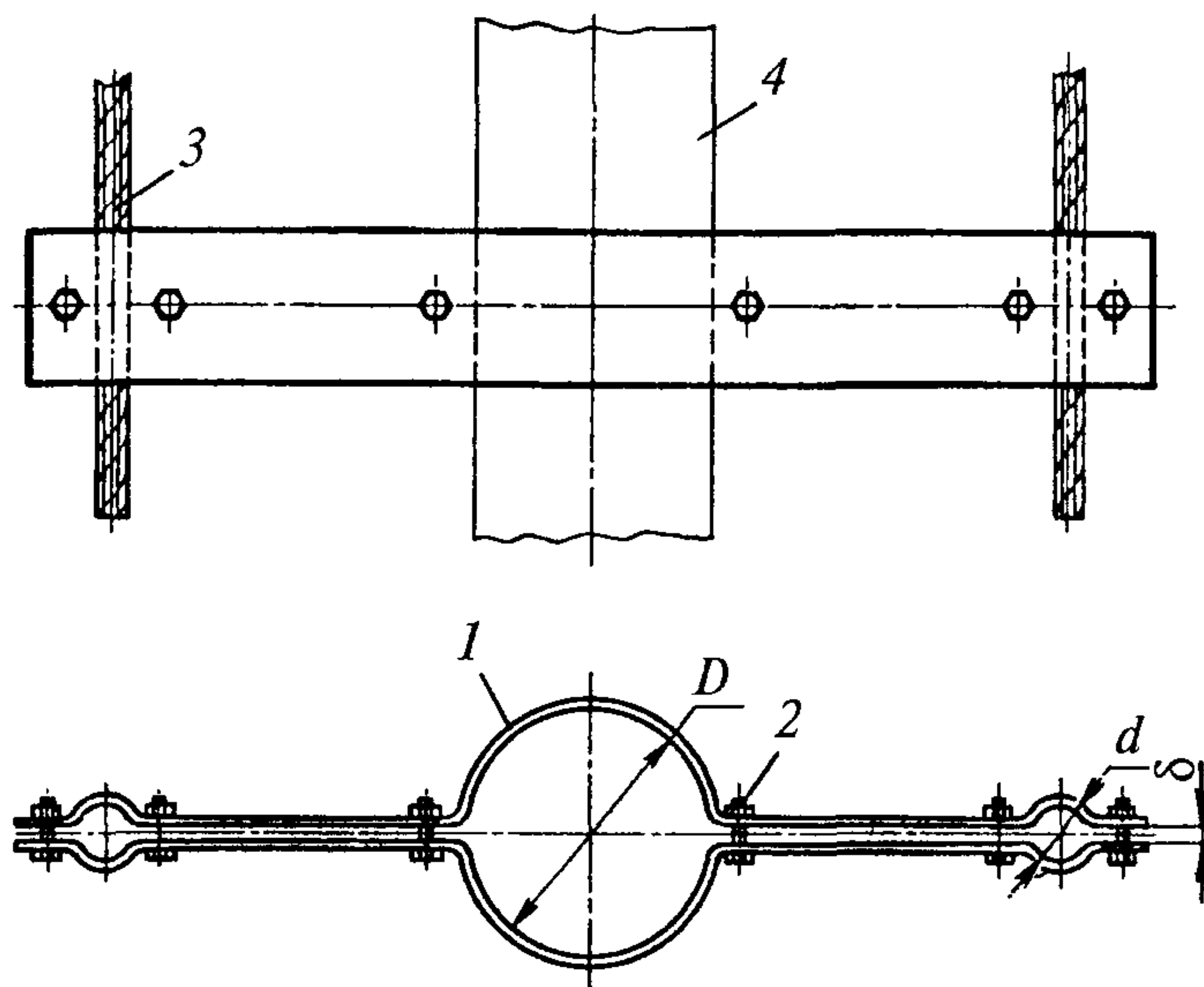
Рис. 45. Устройство для подвески трубопровода
