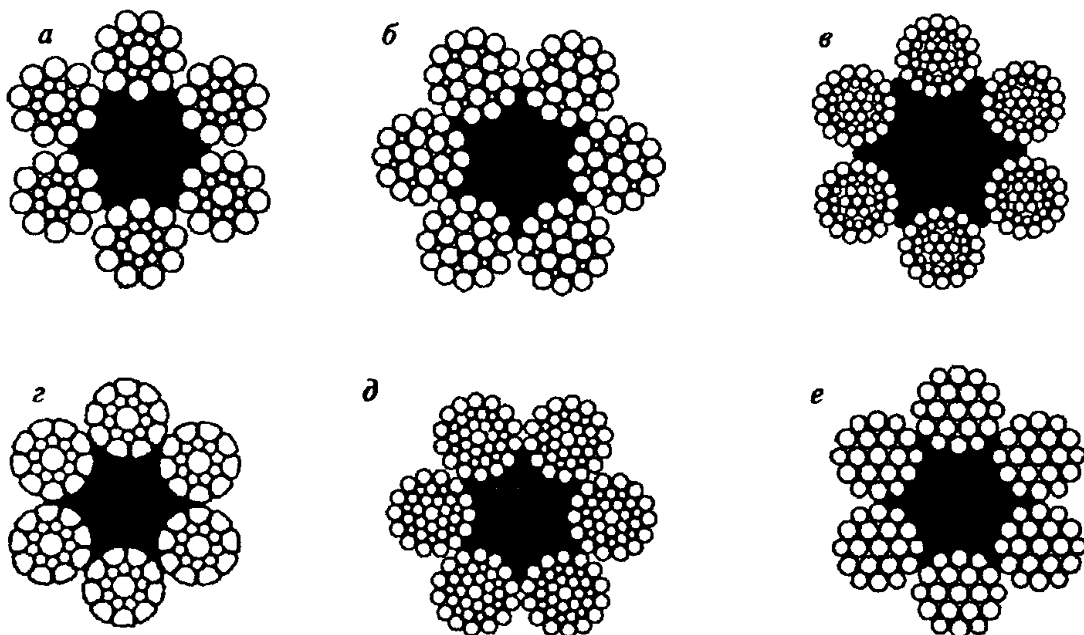
Рис. 2. Канаты подъемные для наклонных стволов: a — по ГОСТ 3077–80; б — по ГОСТ 7665–80; в — по ГОСТ 3079–80; г — канаты из пластически обжатых прядей ПК; д — по ТУ 14-4-1444–87-Б, ГОСТ 7668–80; е — по ГОСТ 2688–80
