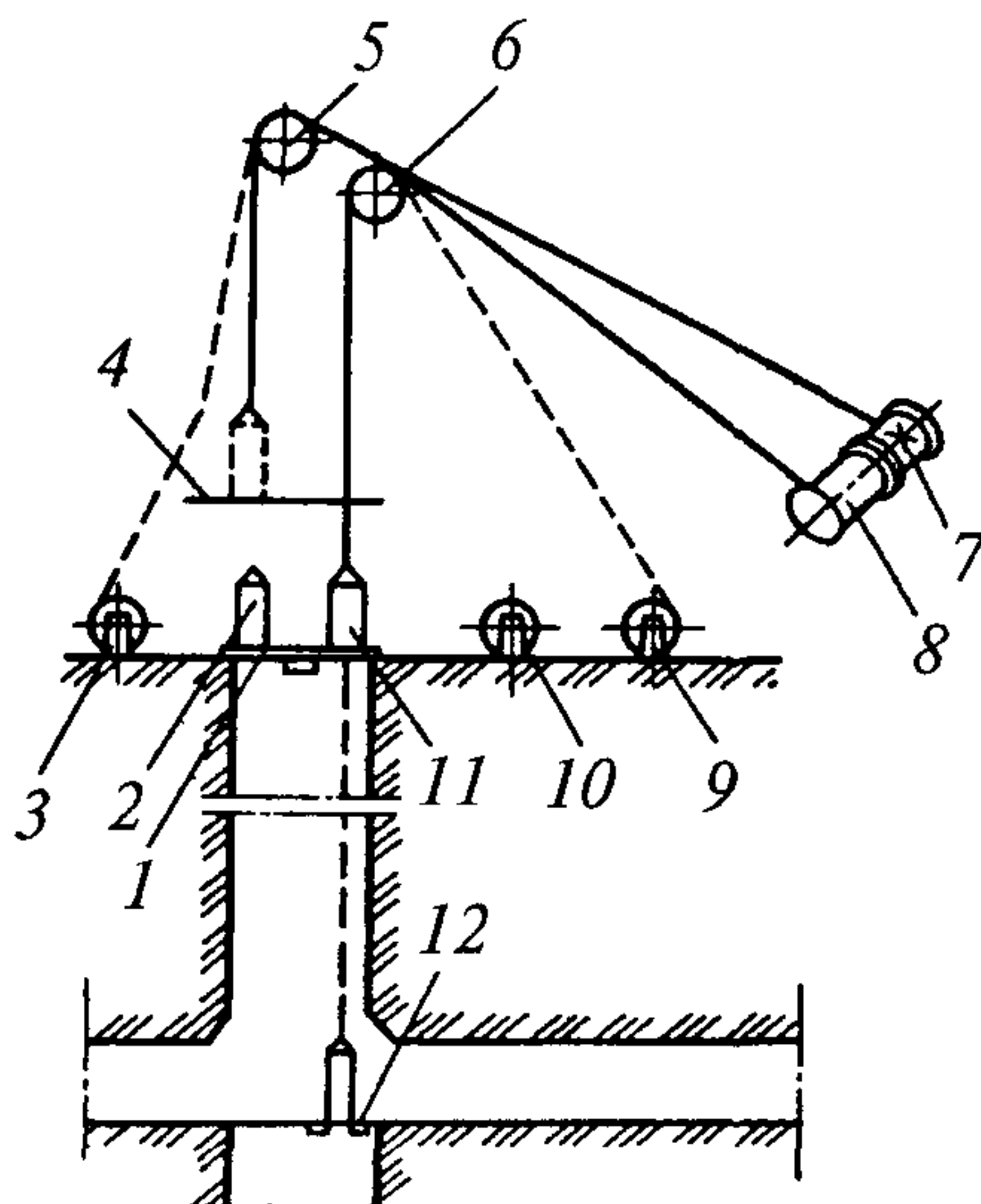
Рис. 15. Схема первоначальной навески на двухбарабанной машине
