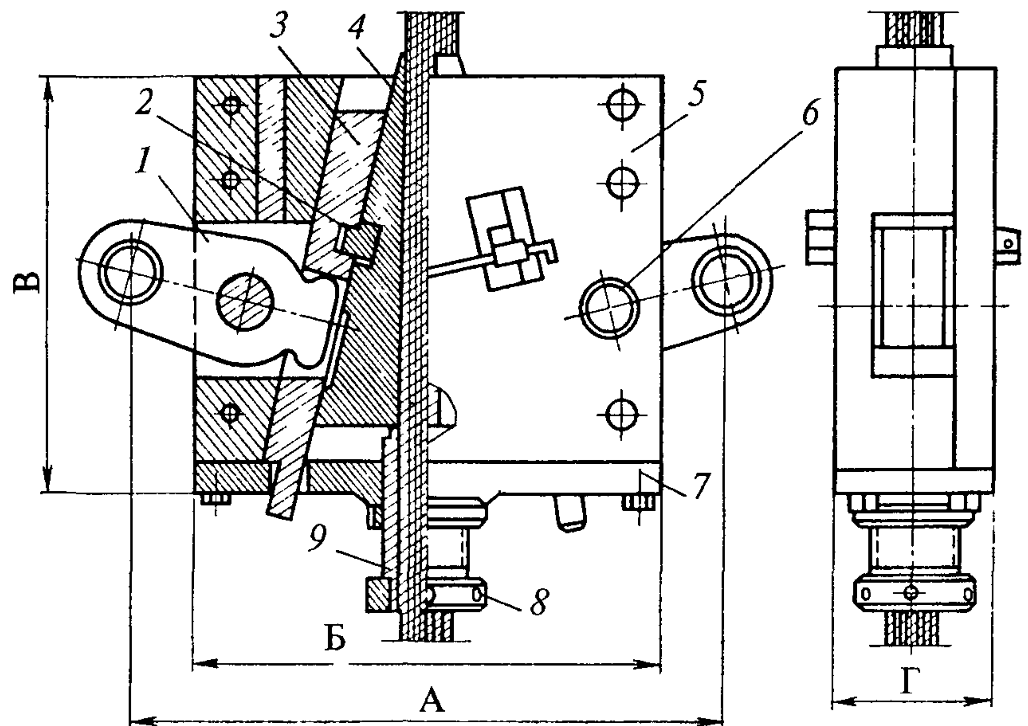
Рис. 30. Клиновые коуши типов КРГ, ККП
