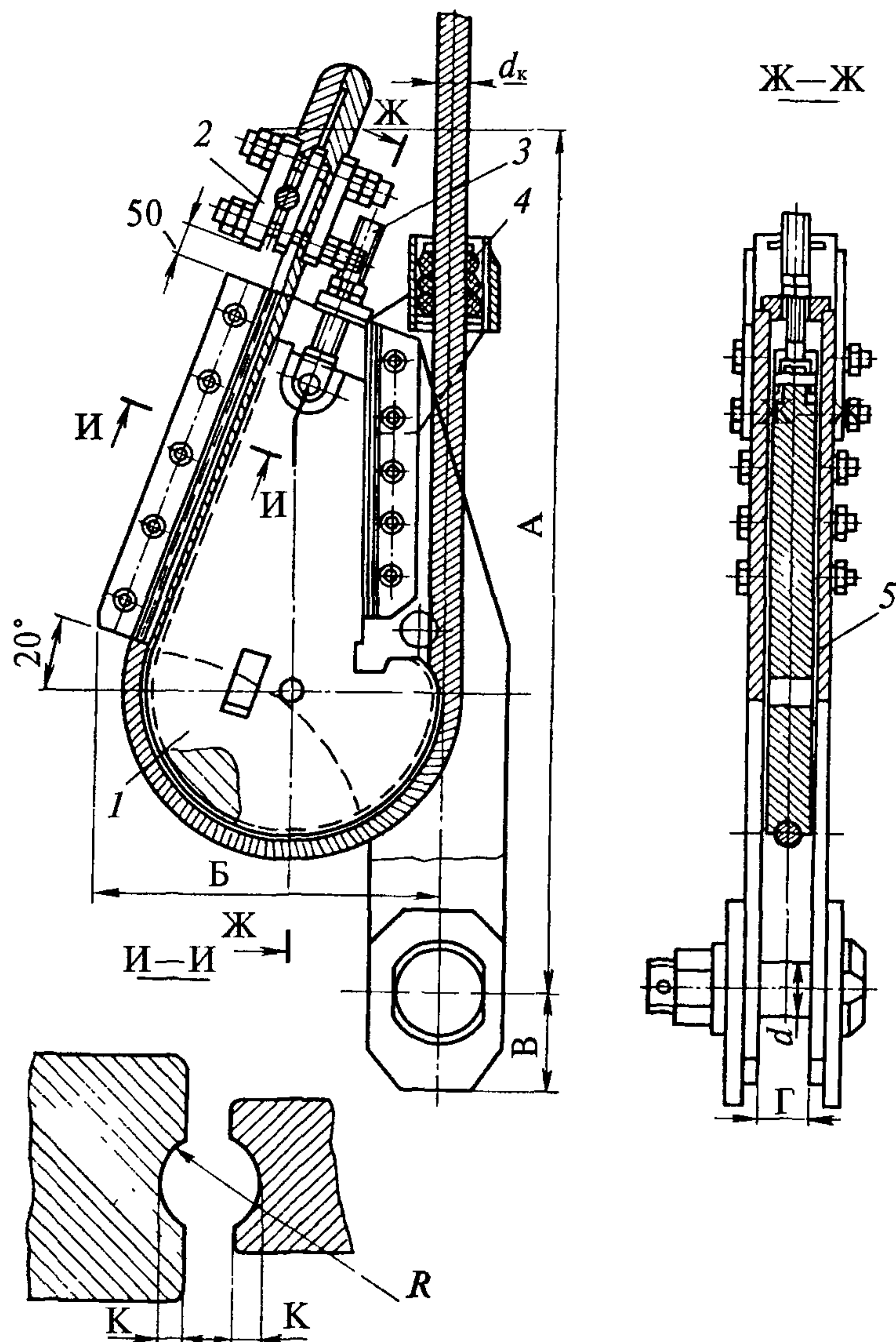
Рис. 29. Устройство прицепное тела ККБ
