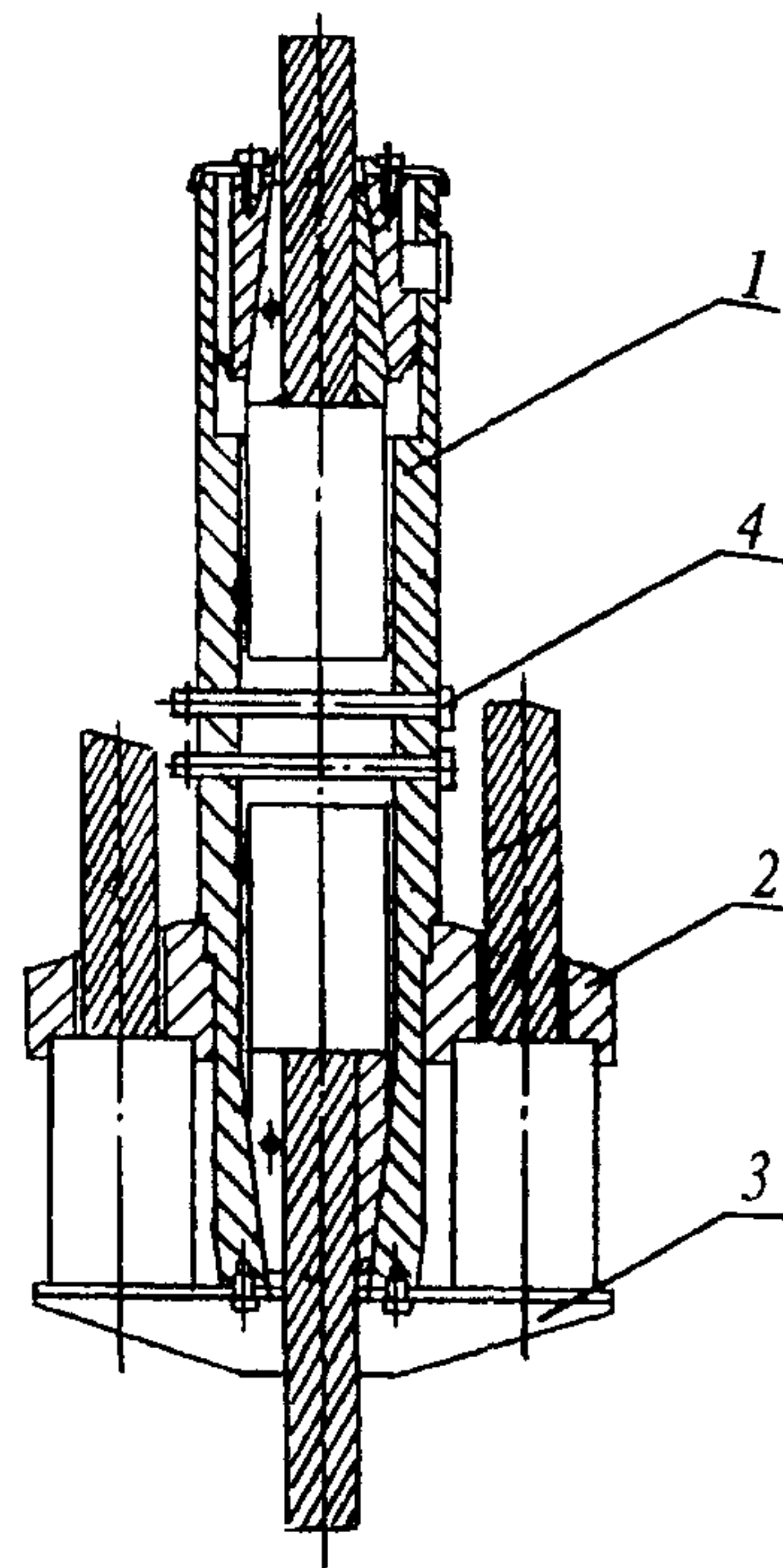
Рис. 40. Трехручьевая соединительная муфта
