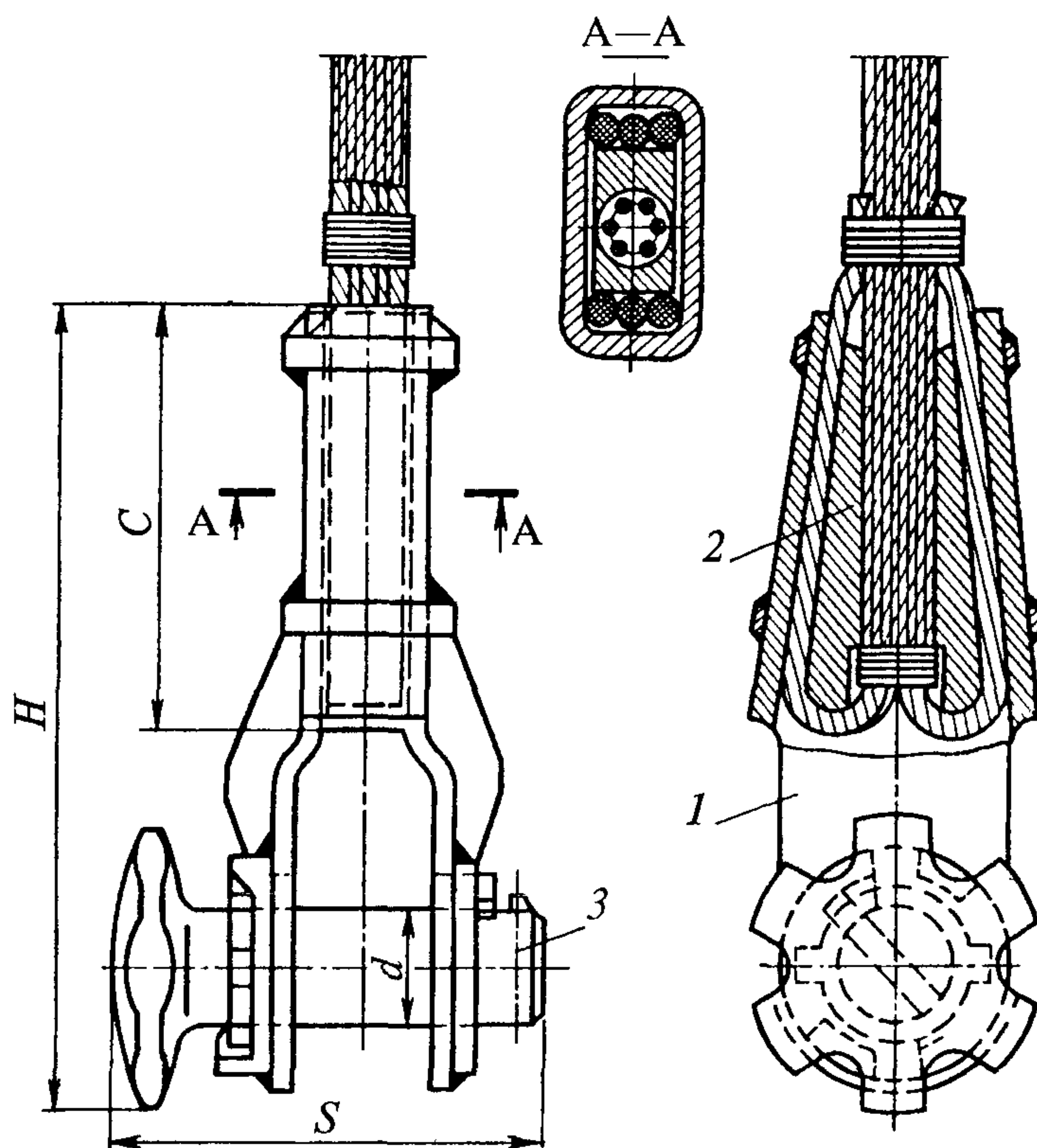
Рис. 34. Устройство прицепное типа МП
