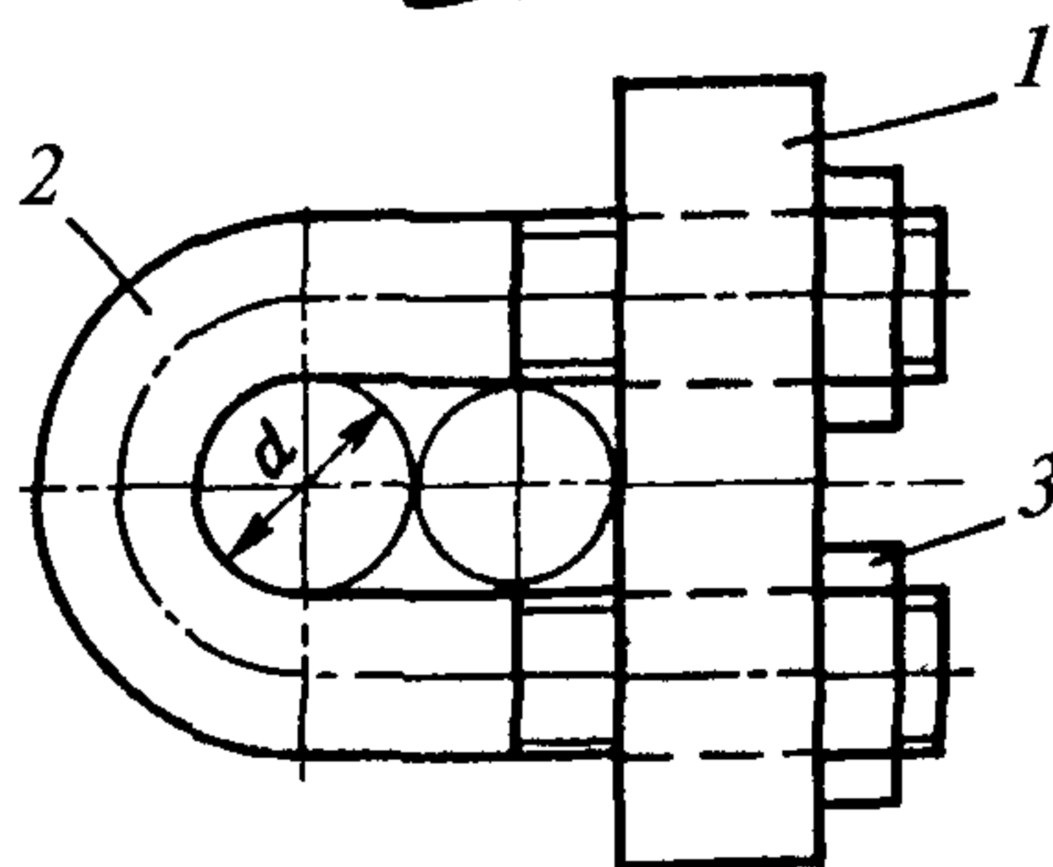
Рис. 9. U-образный зажим для соединения канатов
