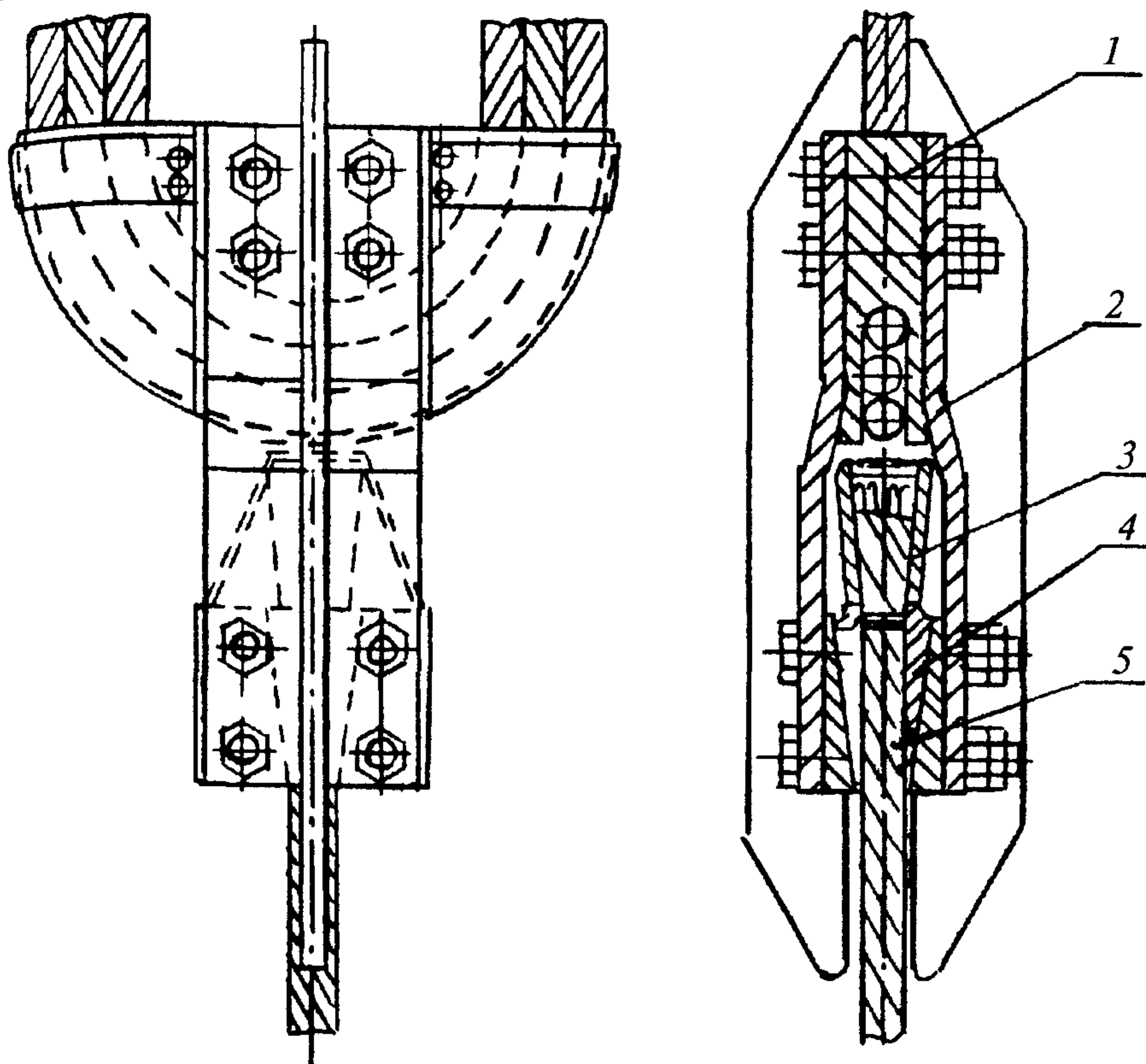
Рис. 41. Блочная соединительная муфта
