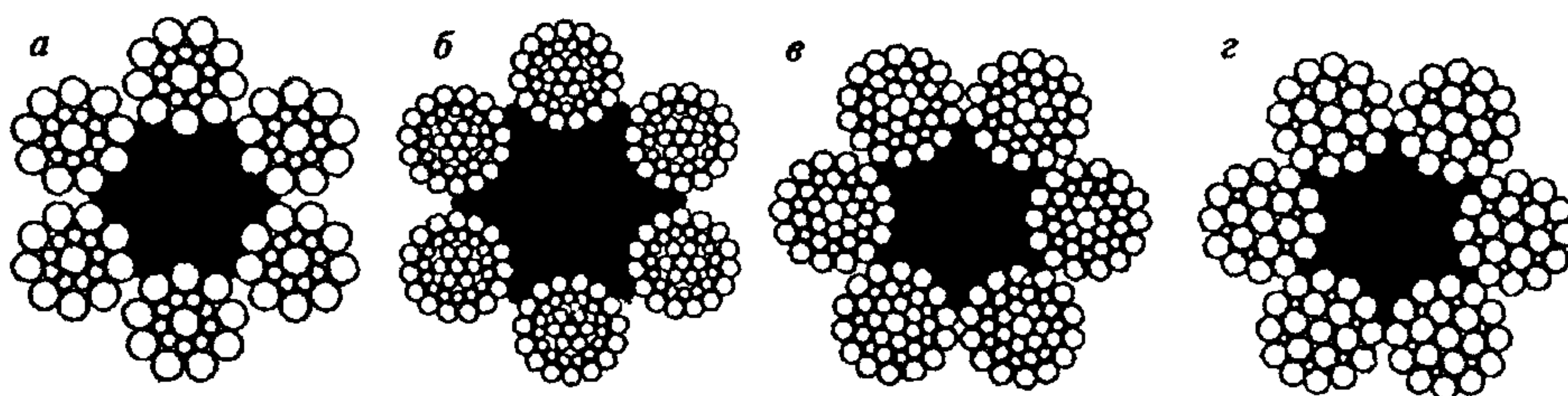
Рис. 4. Тормозные канаты:
