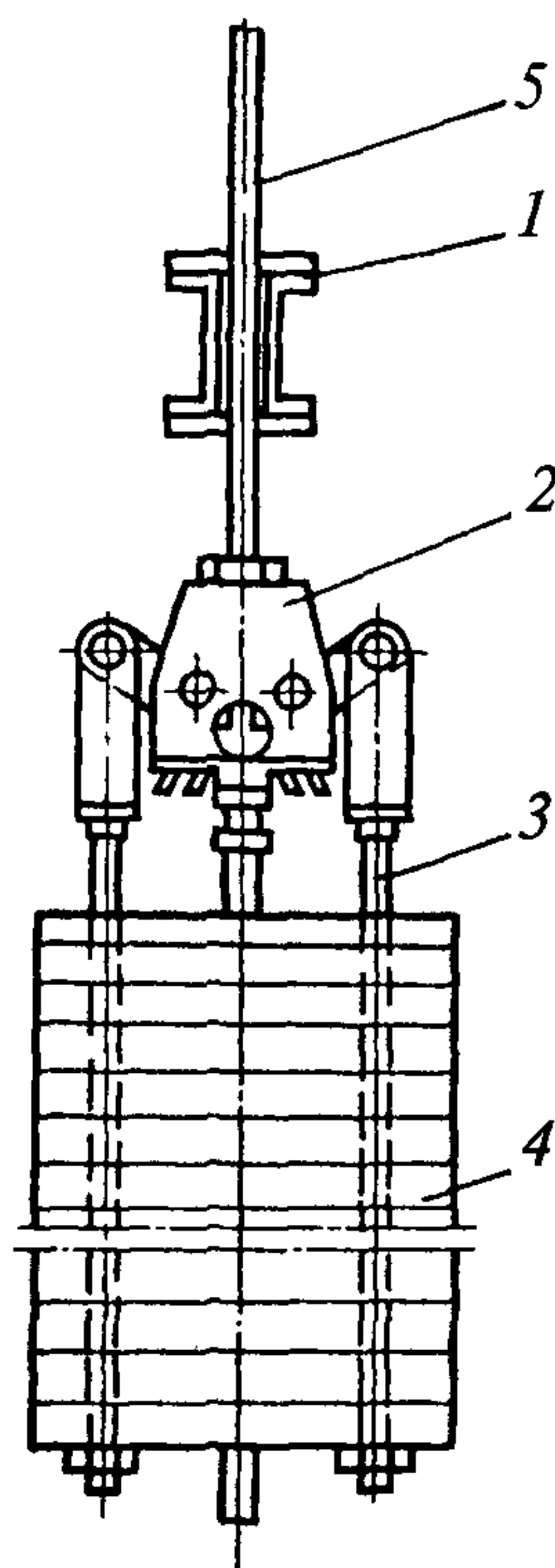
Рис. 42. Крепление грузов для натяжения проводниковых канатов в зумпфе
