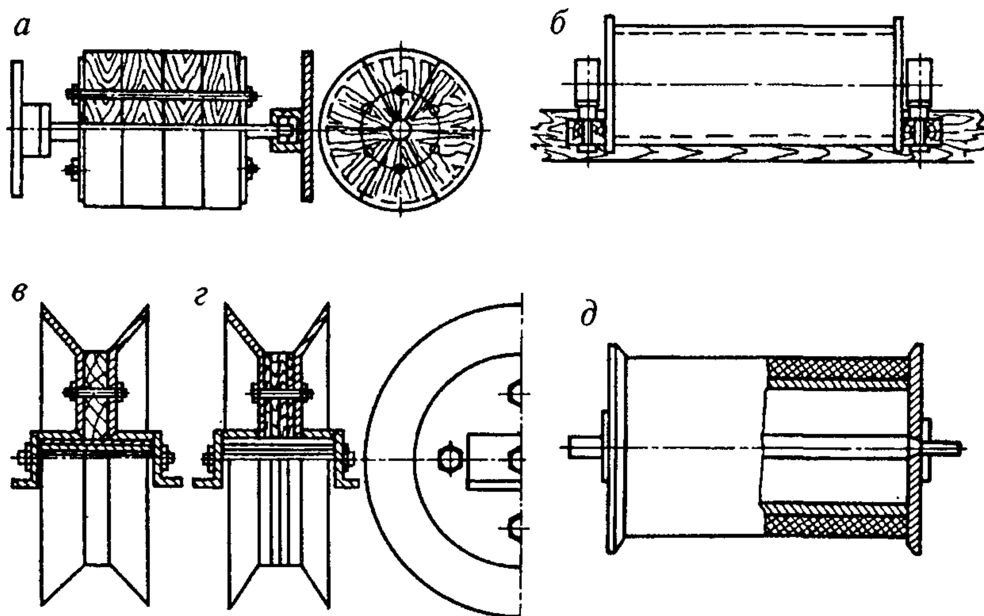
Рис. 51. Путьевые ролики:
