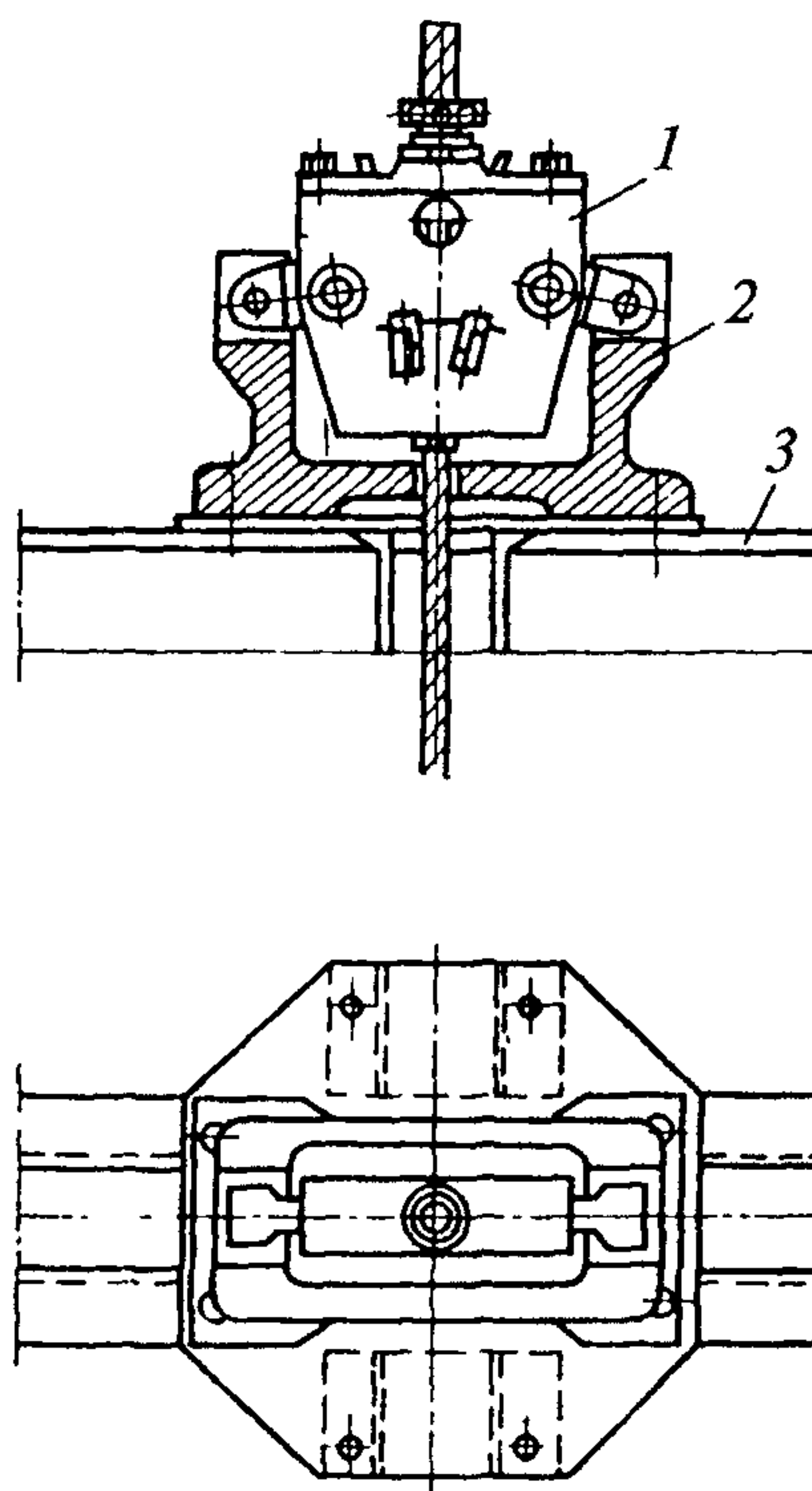
Рис. 43. Крепление проводникового каната на копре
