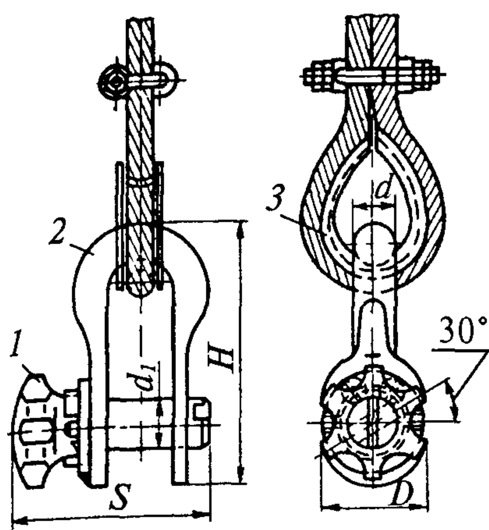
Рис. 36. Устройство прицепное типа ПС
