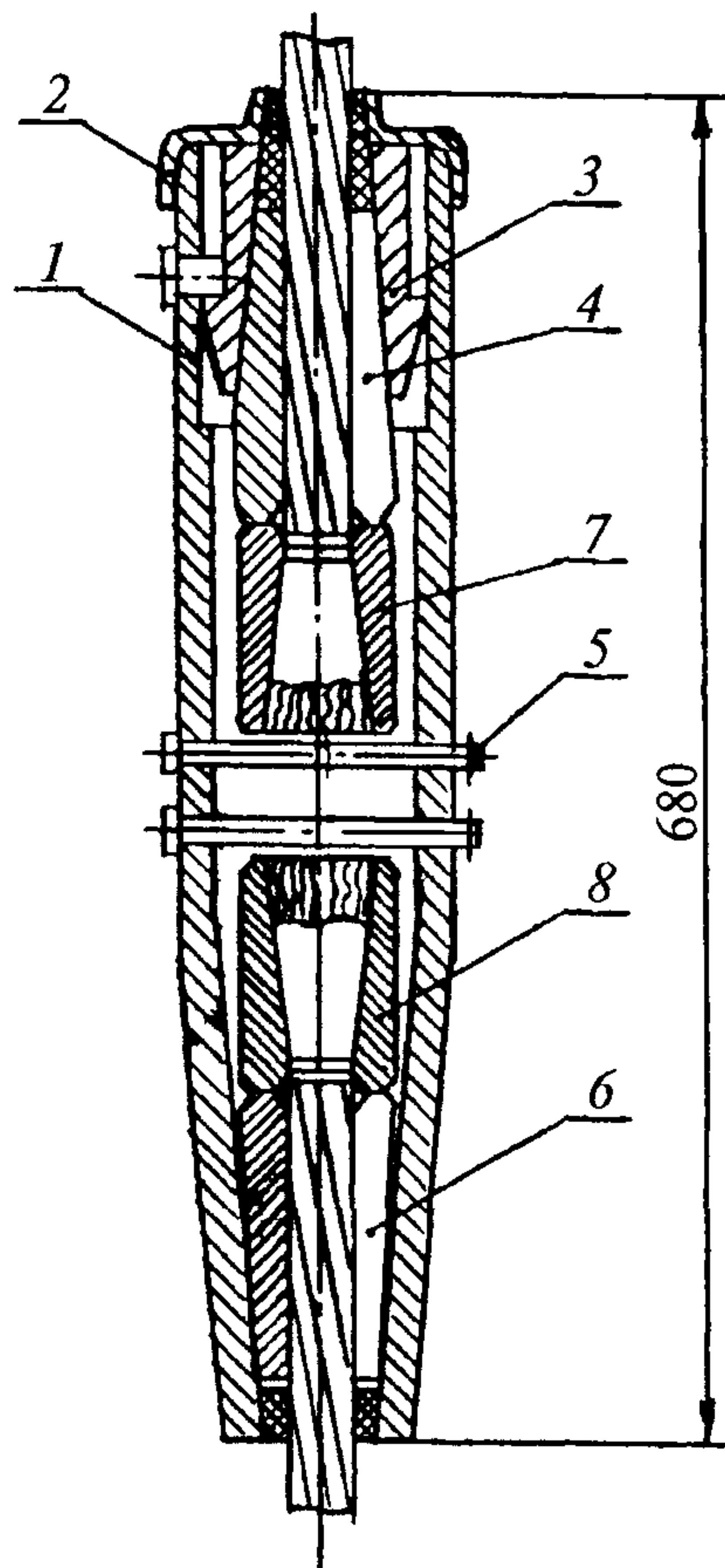
Рис. 39. Одноручьевая соединительная муфта
