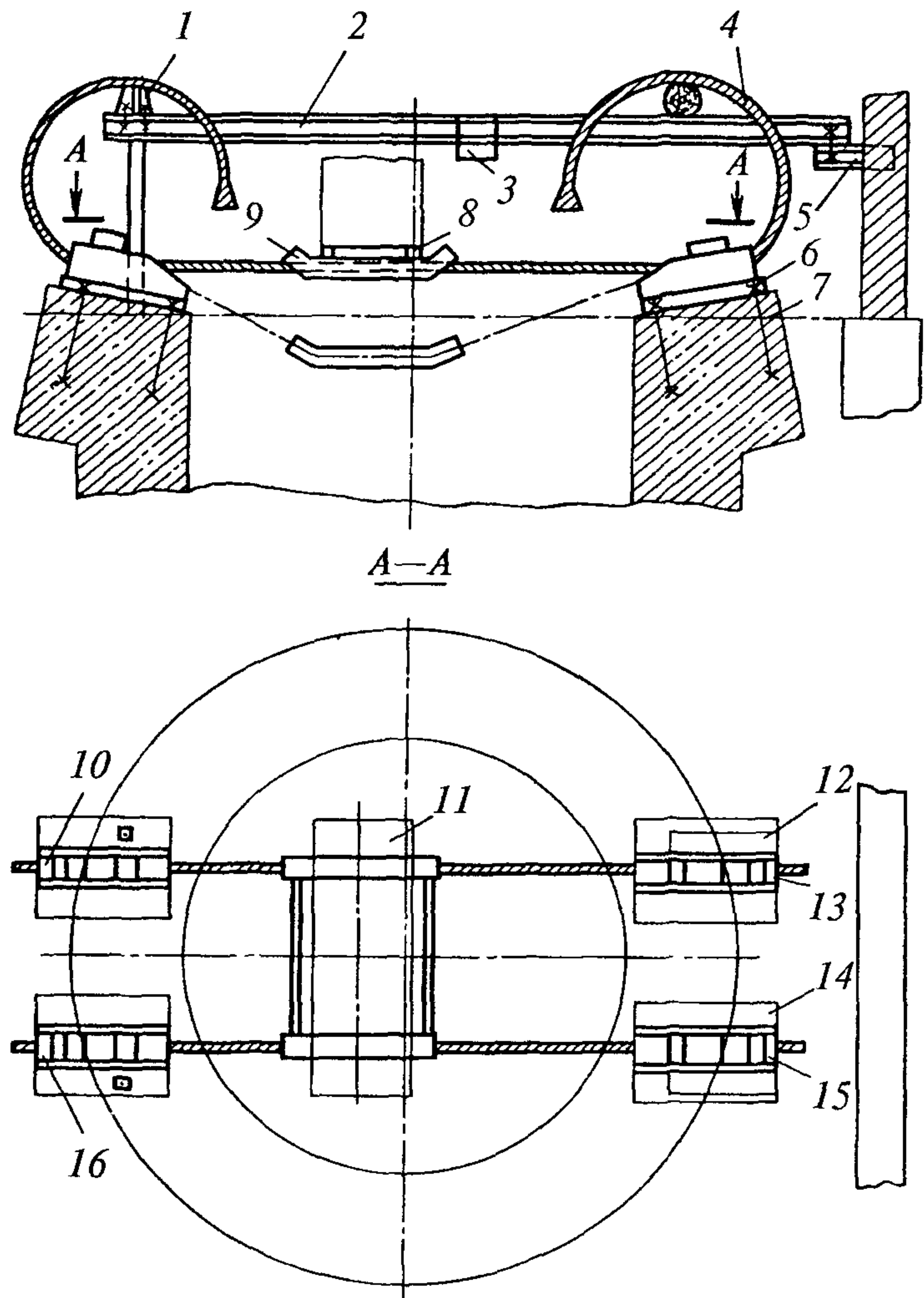
Рис. 14. Гибкое перекрытие для испытания парашютов
