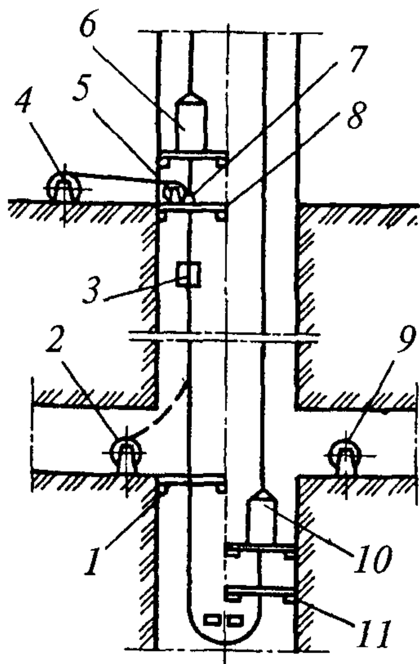
Рис. 24. Схема первоначальной навески и замены уравновешивающего каната
