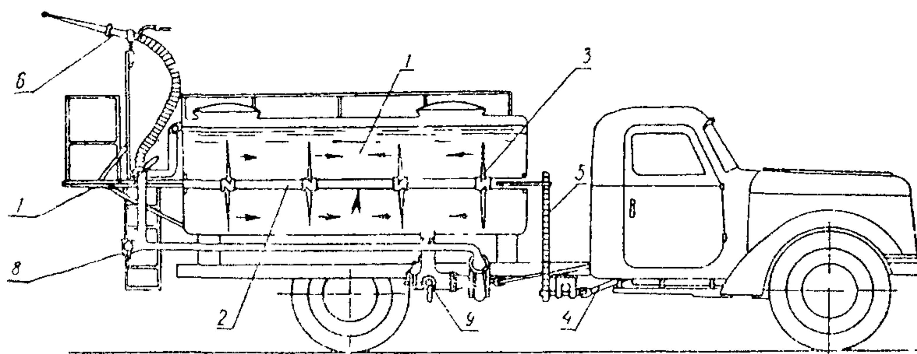
Рис. 1. Схема гидросеялки ДЭ-16:
