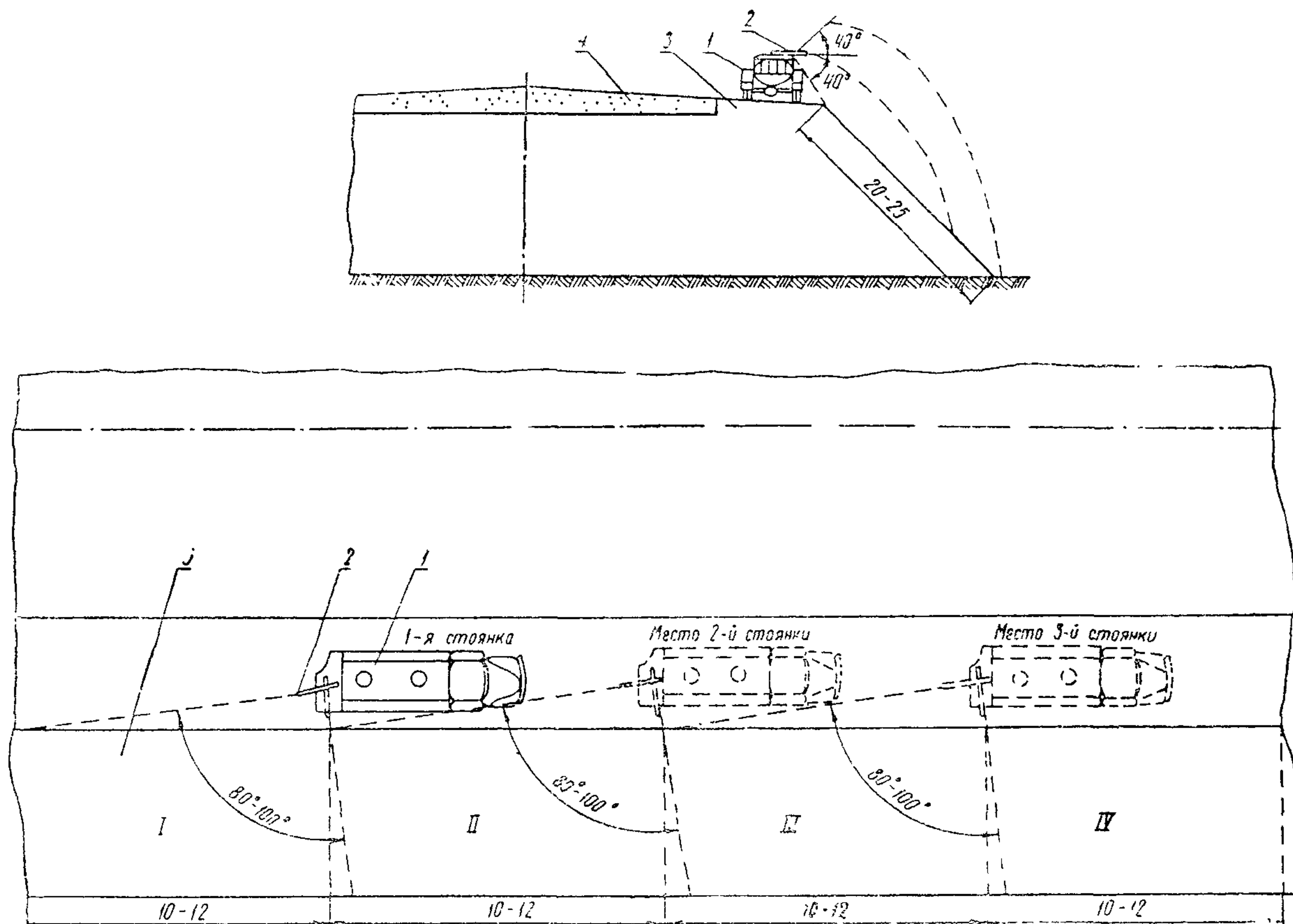
Рис. 2. Технологическая схема по укреплению откосов земляного полотна гидропосевом многолетних трав: 1—гидросеялка ДЭ-16, 2—гидрометатель; 3—обочина; 4—покрытие; 5—укрепленный участок откоса; I, II, III, IV—участки, обрабатываемые с одной стоянки
