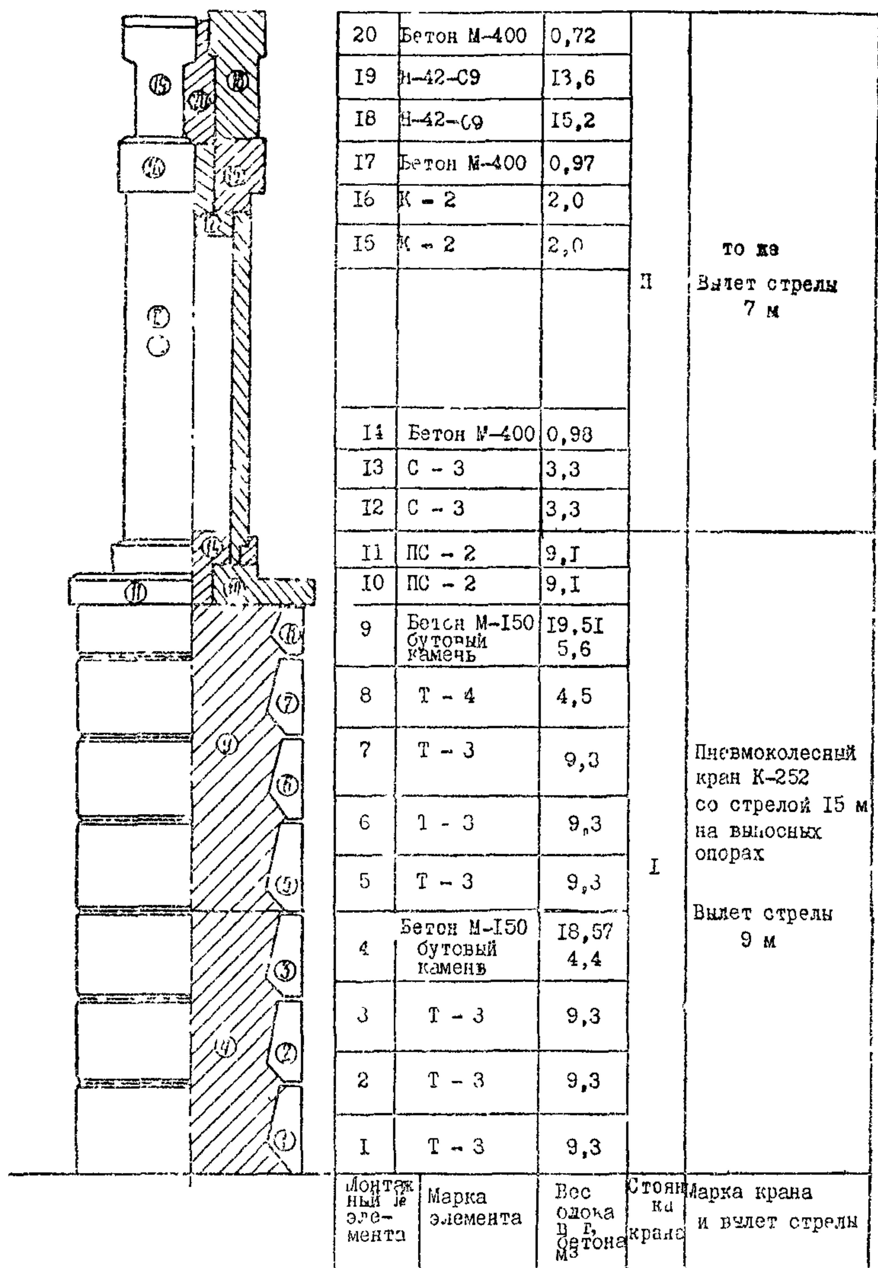
Рис 4 Технологическая схема последовательности монтажа опоры при монолитном заполнении ядра
