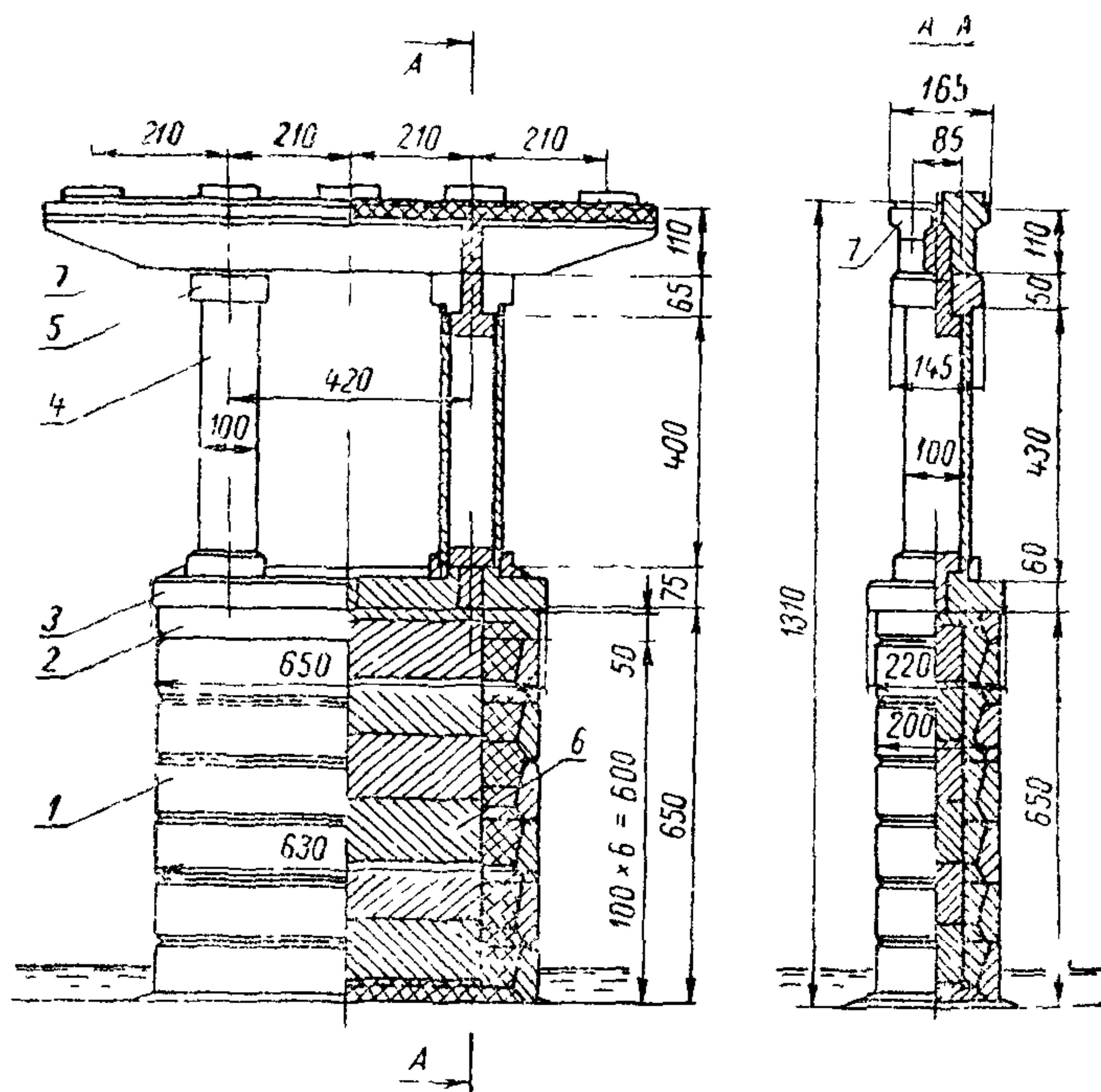
Рис. 1. Общий вид опоры:
