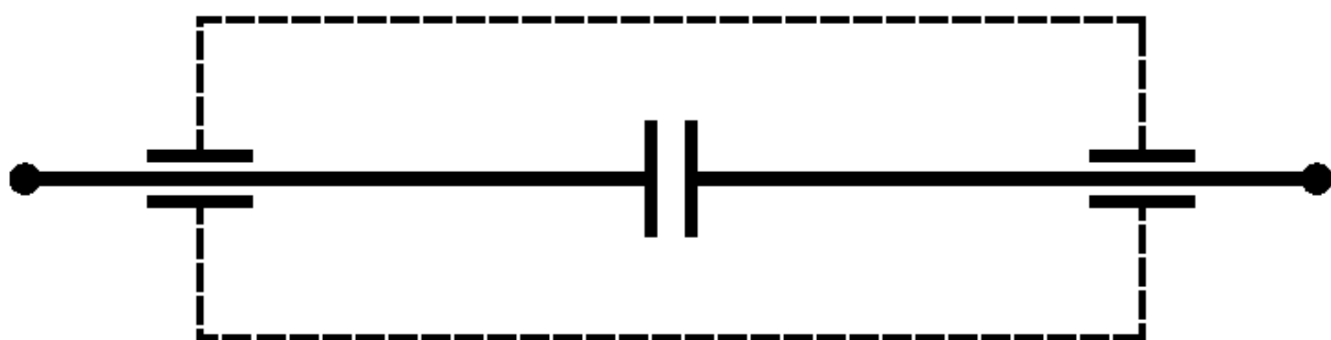
Рисунок 1 — Конденсатор с двумя выводами
