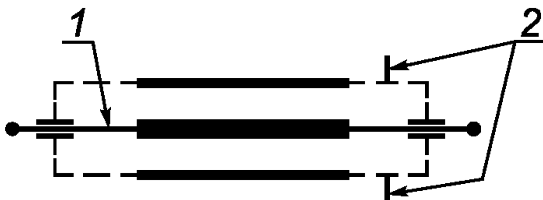
1 — центральный токоведущий проводник; 2 — круглый монтажный заземленный фланец Рисунок 3 — Проходной конденсатор (коаксиальный)
