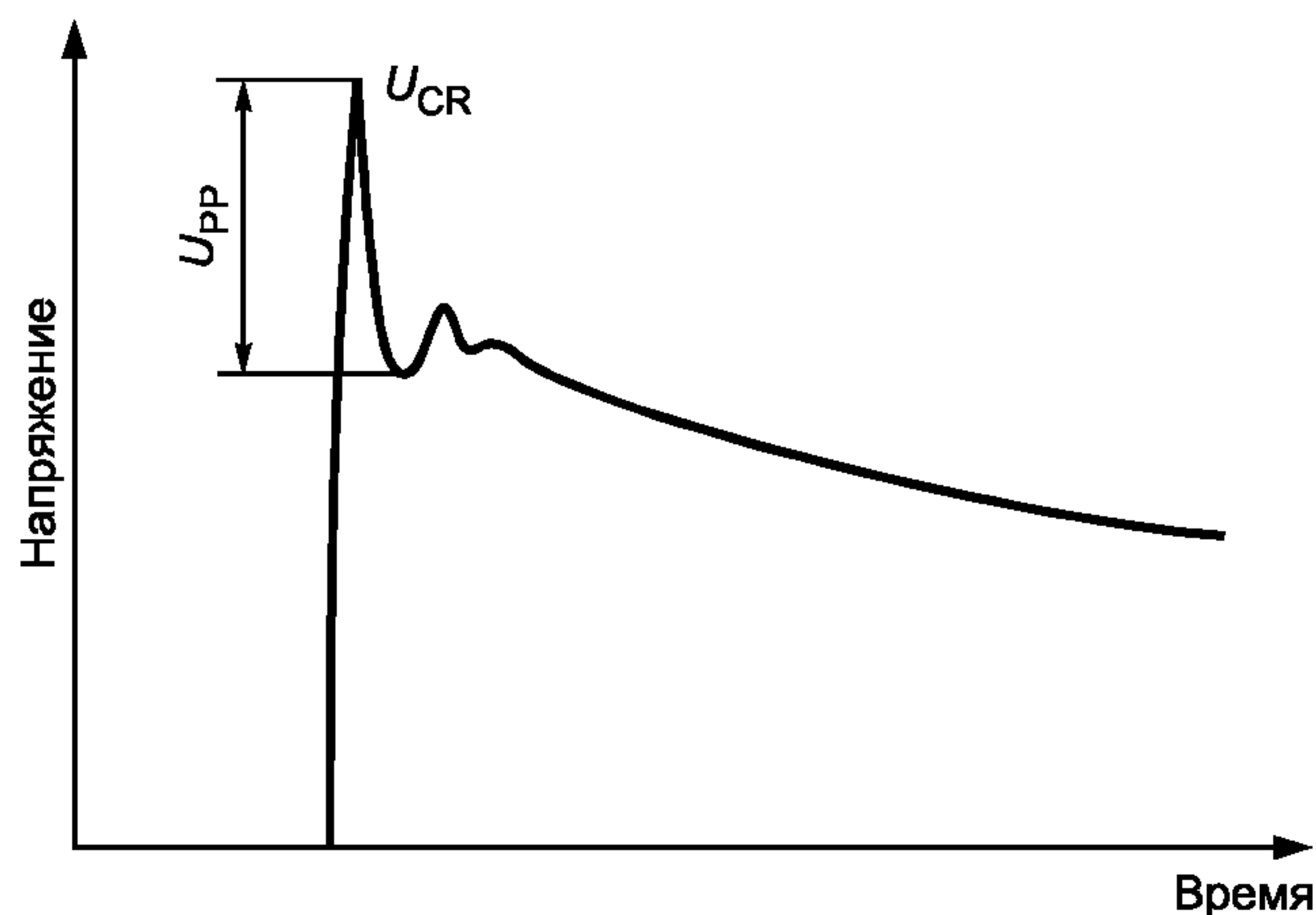
Рисунок 6 — Форма импульса
