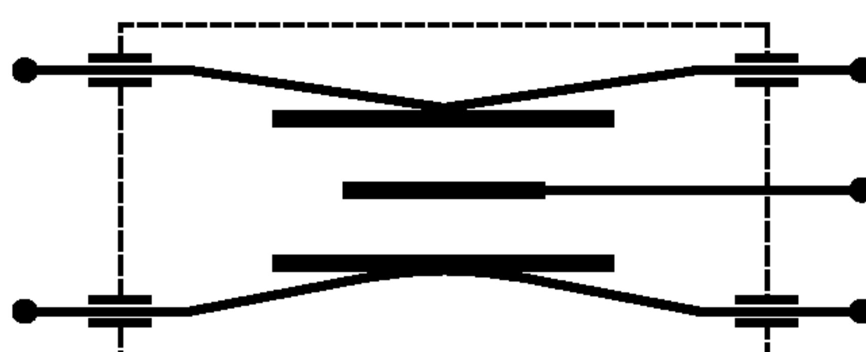
Рисунок 4d — Многосекционный проходной конденсатор
