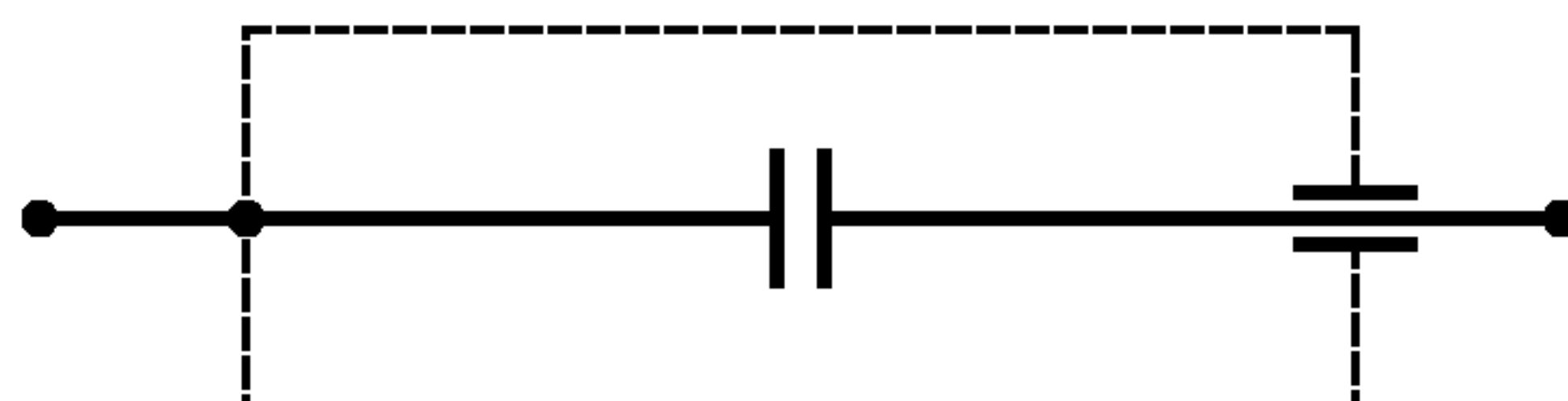
Рисунок 5а — Односекционный шунтирующий конденсатор
