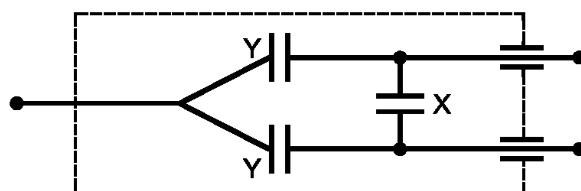
Рисунок 5b — Шунтирующий конденсатор, соединенный по схеме треугольника
