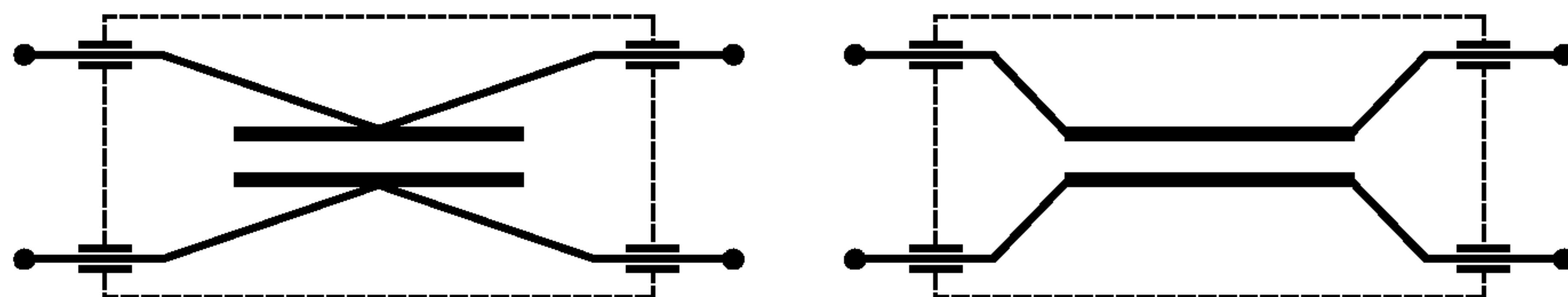
Рисунок 4а — Проходной конденсатор для симметричного включения в цепь (некоаксиальный)
