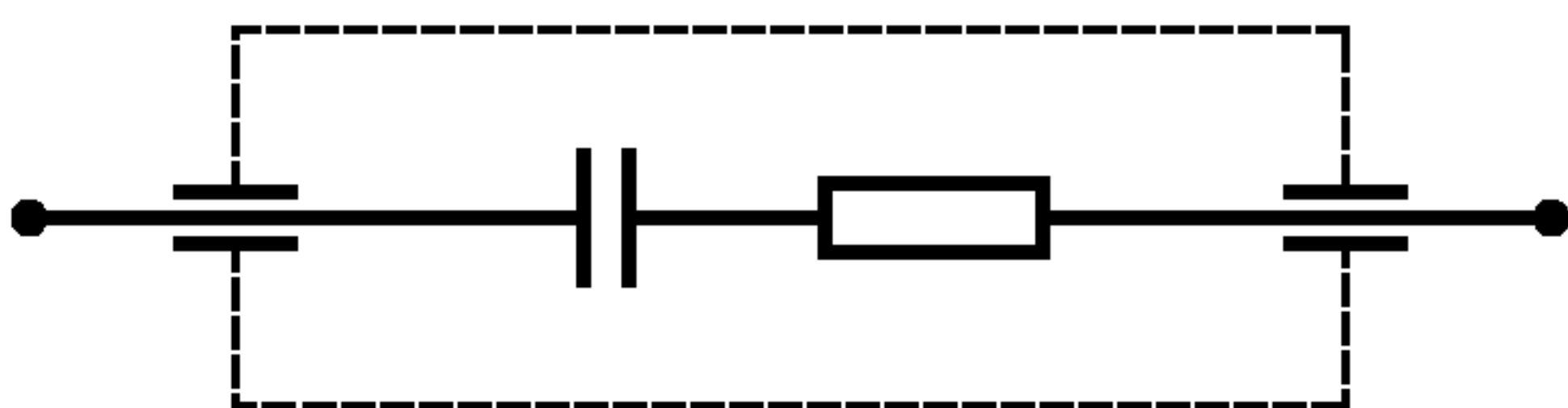
Рисунок 2 — RC-сборка
