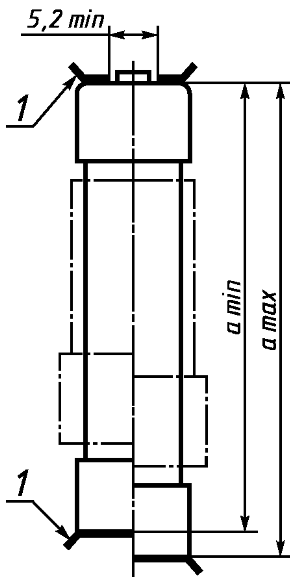
Контакты на торцевых поверхностях плавких вставок
