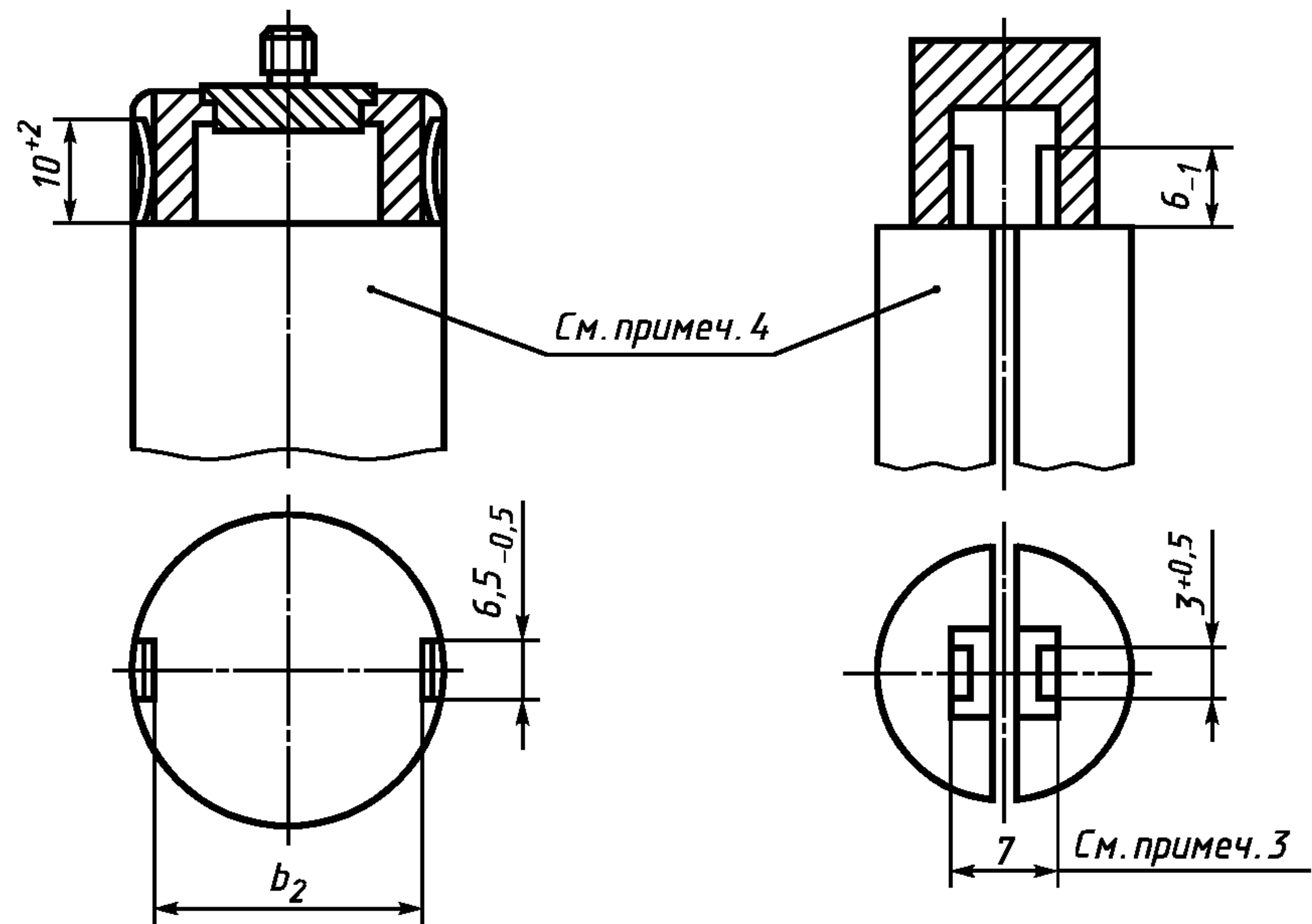
Рабочая головка ключа
