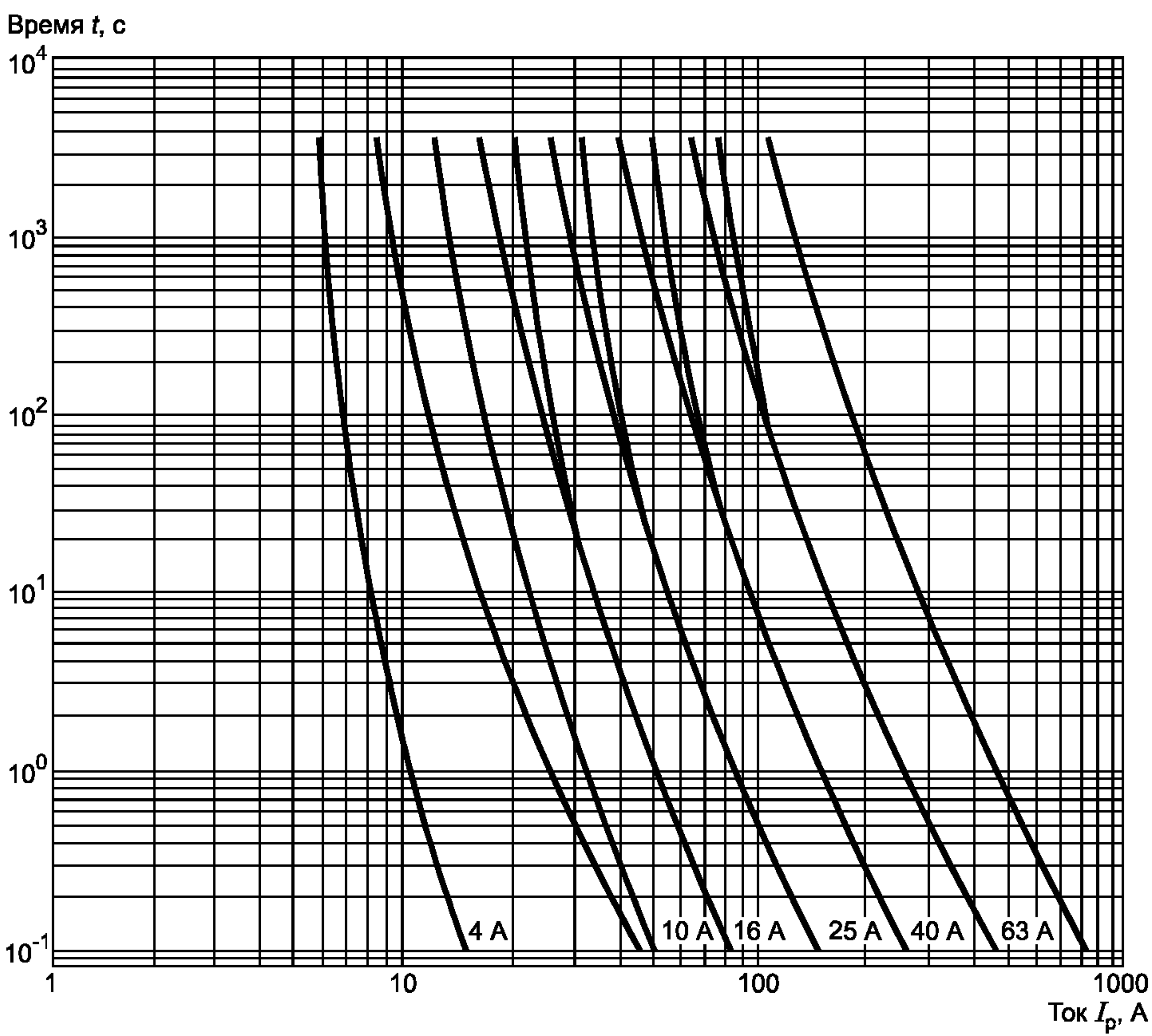
Рисунок 25b — Времятоковые зоны
