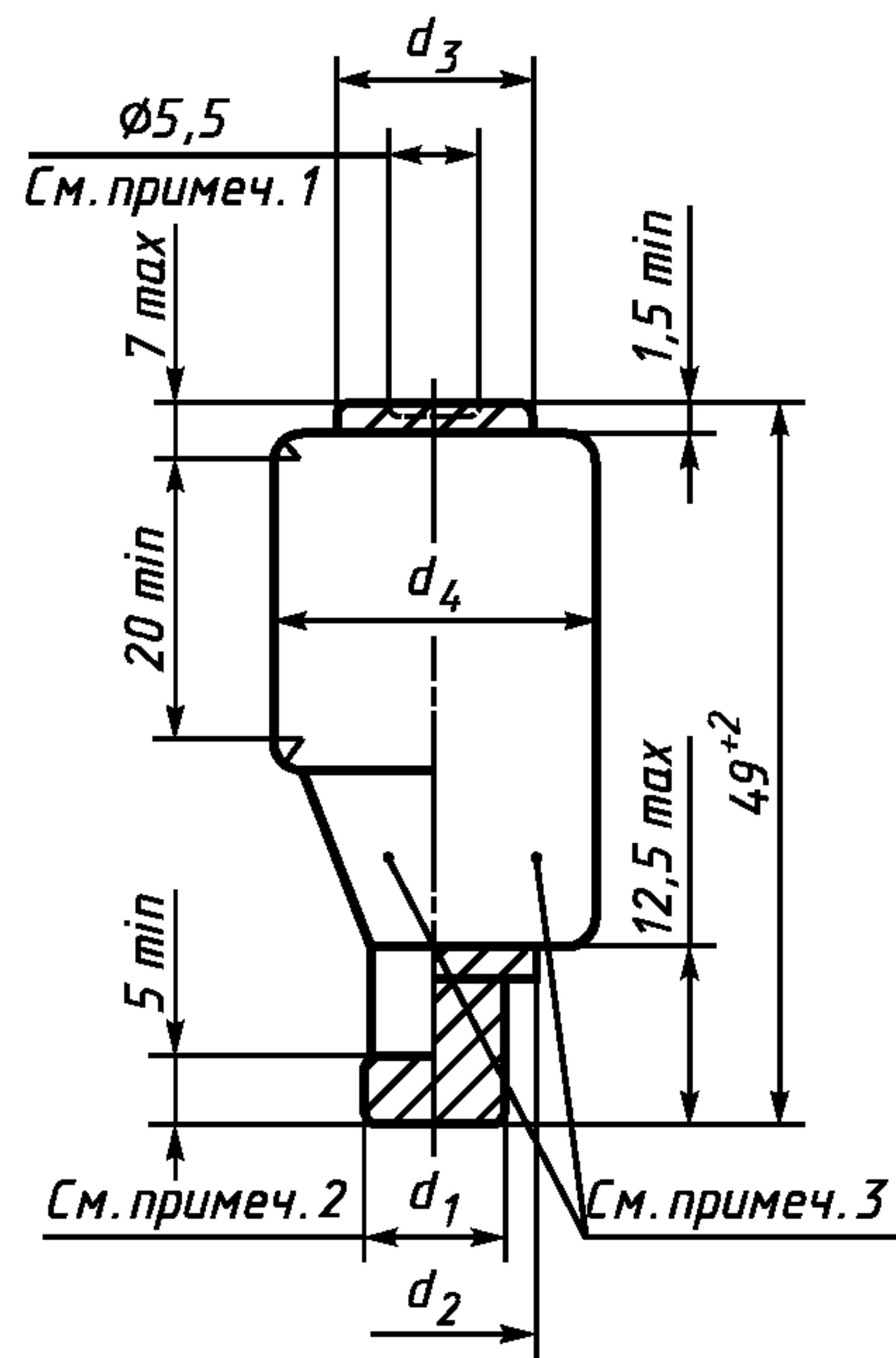
Типоразмеры DII; DIII
