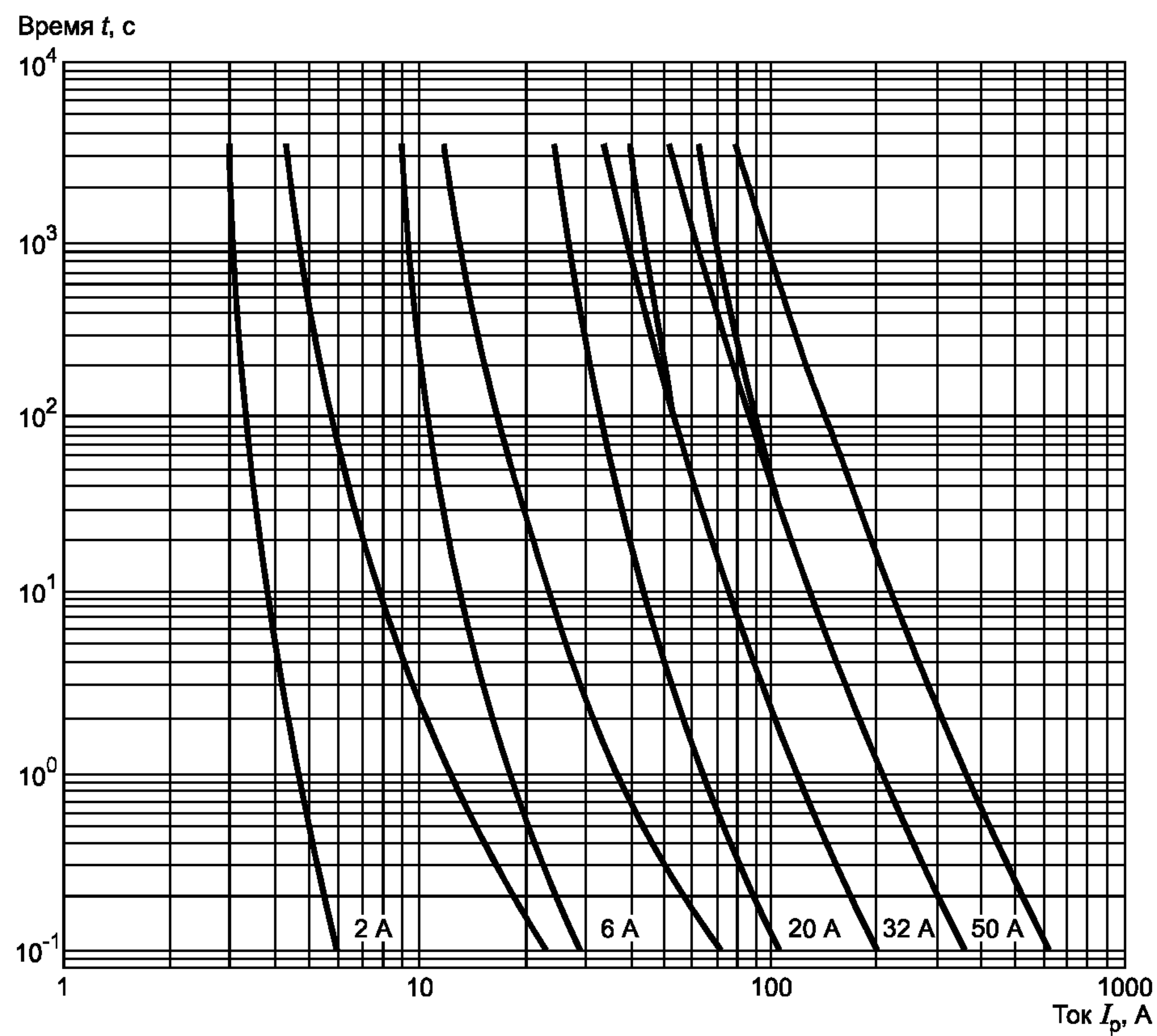
Рисунок 25а — Времятоковые зоны
