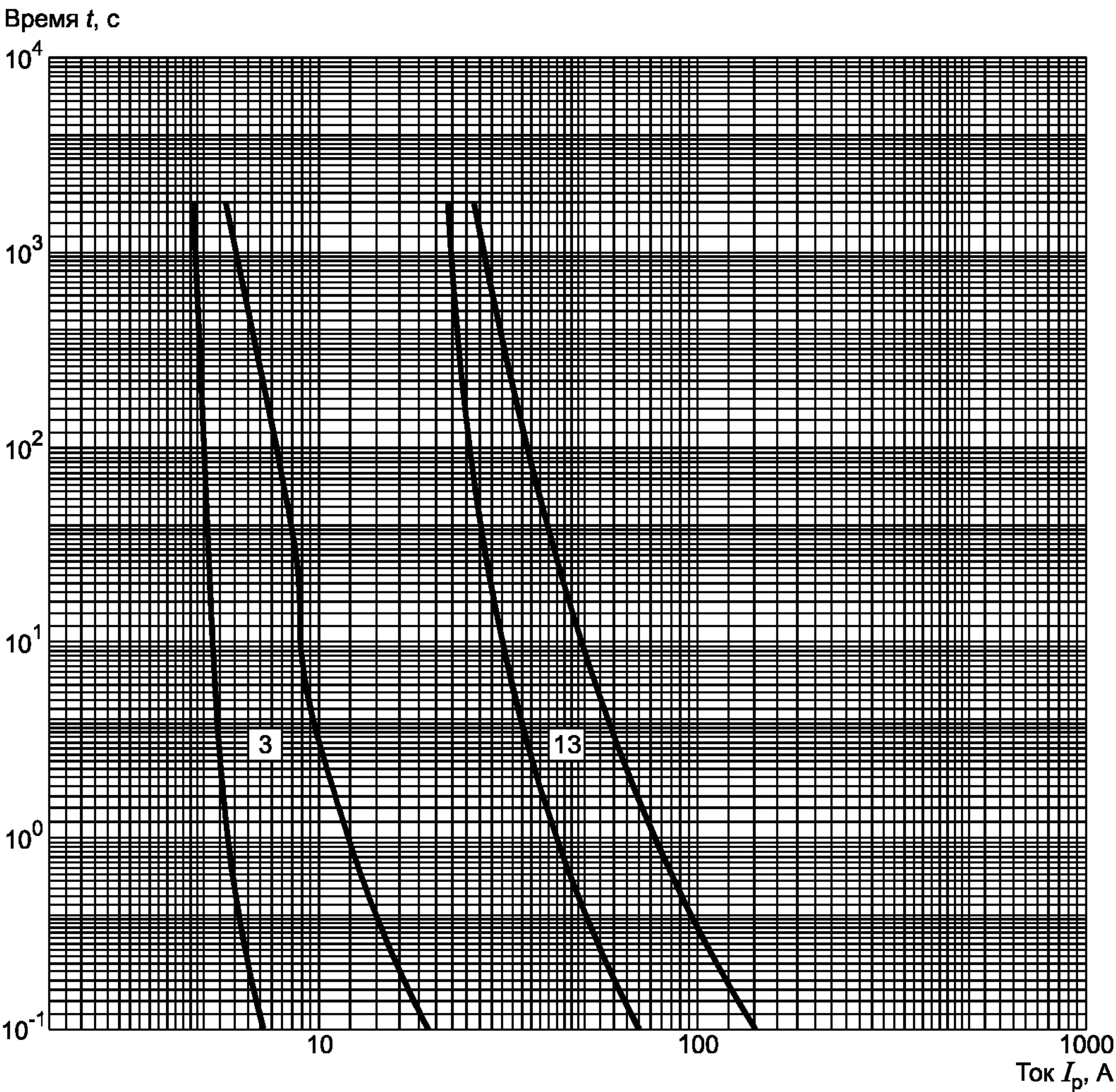
Рисунок 34 — Времятоковые зоны для плавких вставок типа gG
