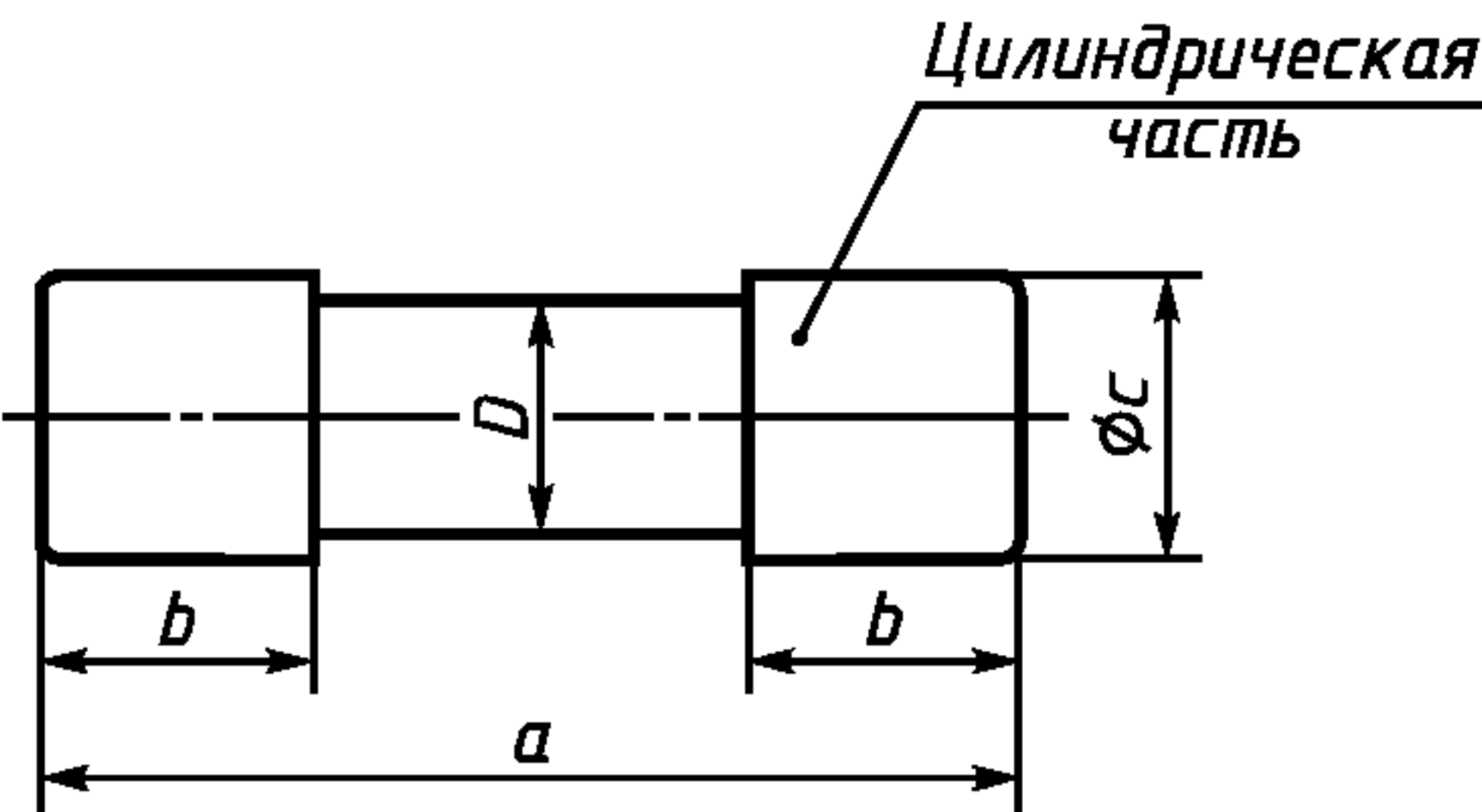
Рисунок не определяет конструкцию, а предназначен только для указания размеров.
