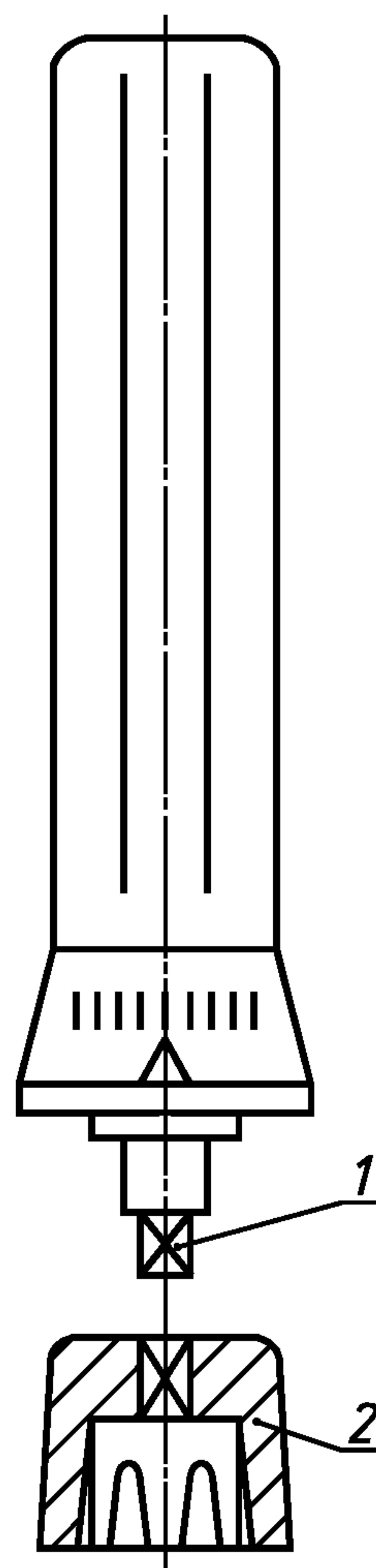
1 — соединительный элемент (квадрат); 2 — переходник (для держателя плавкого предохранителя)
