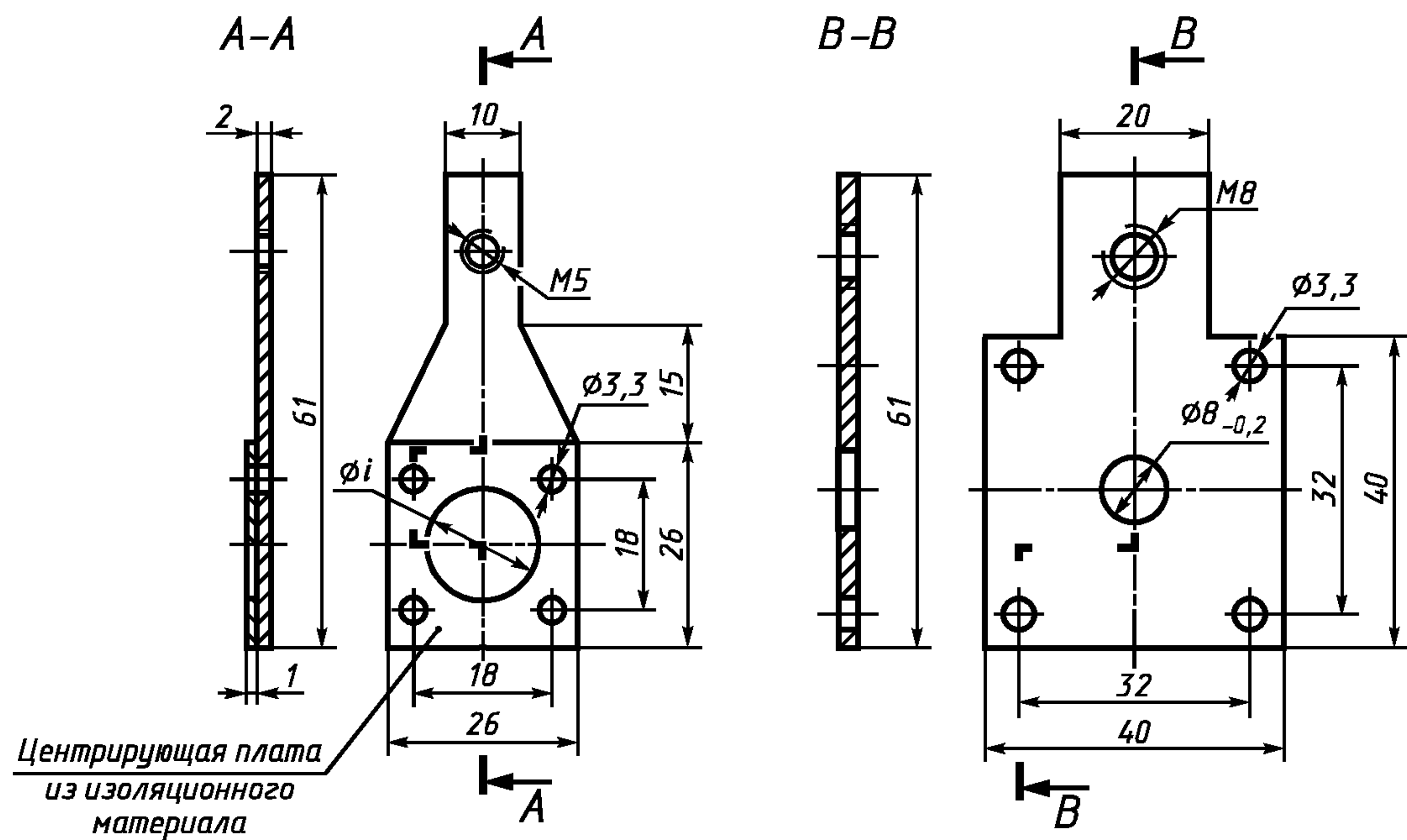
Типоразмеры D01—D03, DII, DIII
