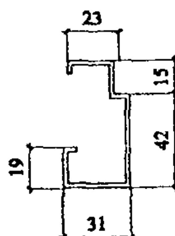
Горизонтальный опорный профиль
