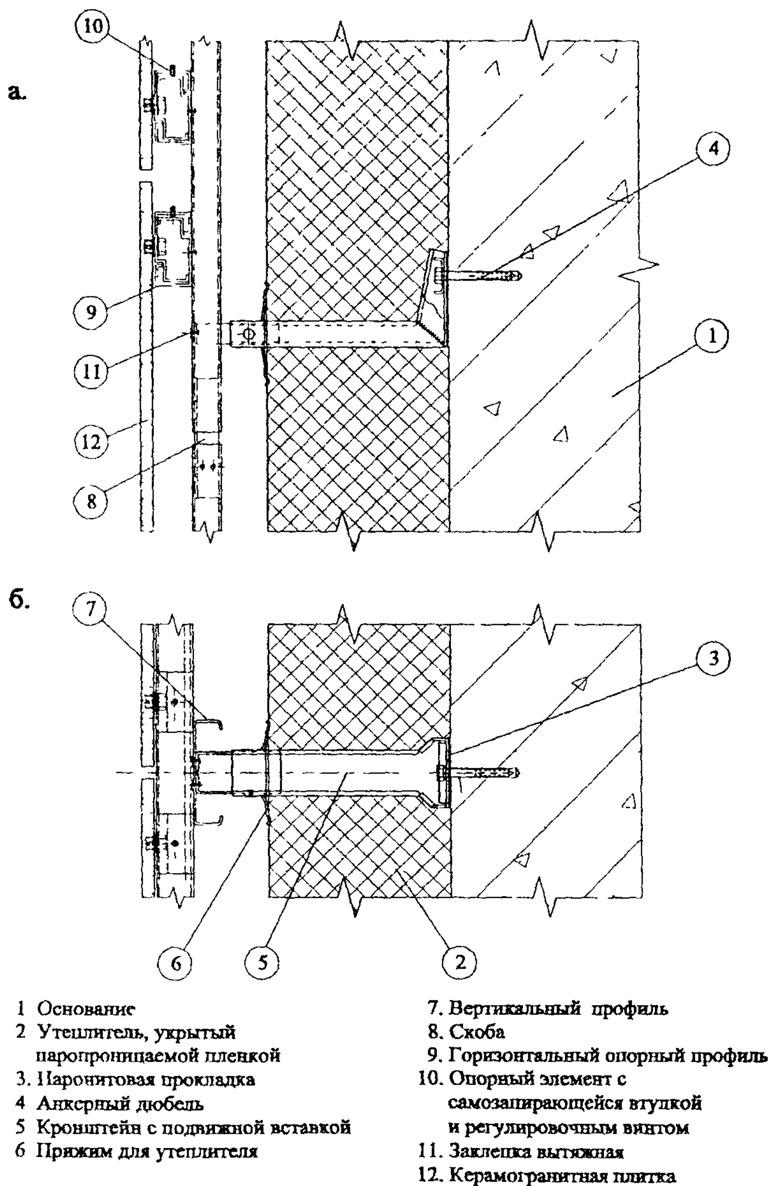
Рис. 3 11 Фасадная система "Диат" СД-02
