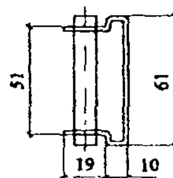
Салазки со штифтом
