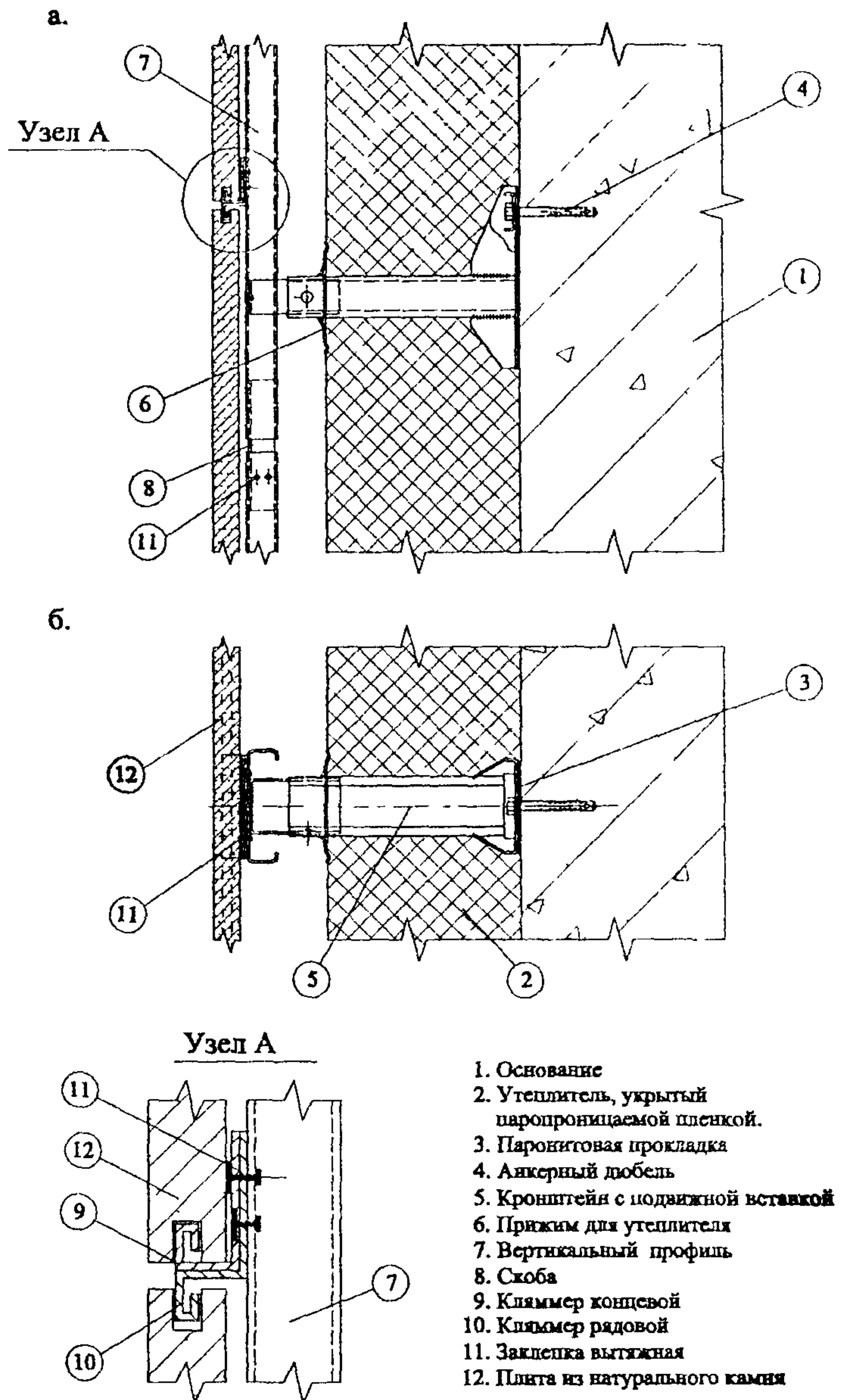
Рис. 3.16. Фасадная система "Диаг" СД-05
