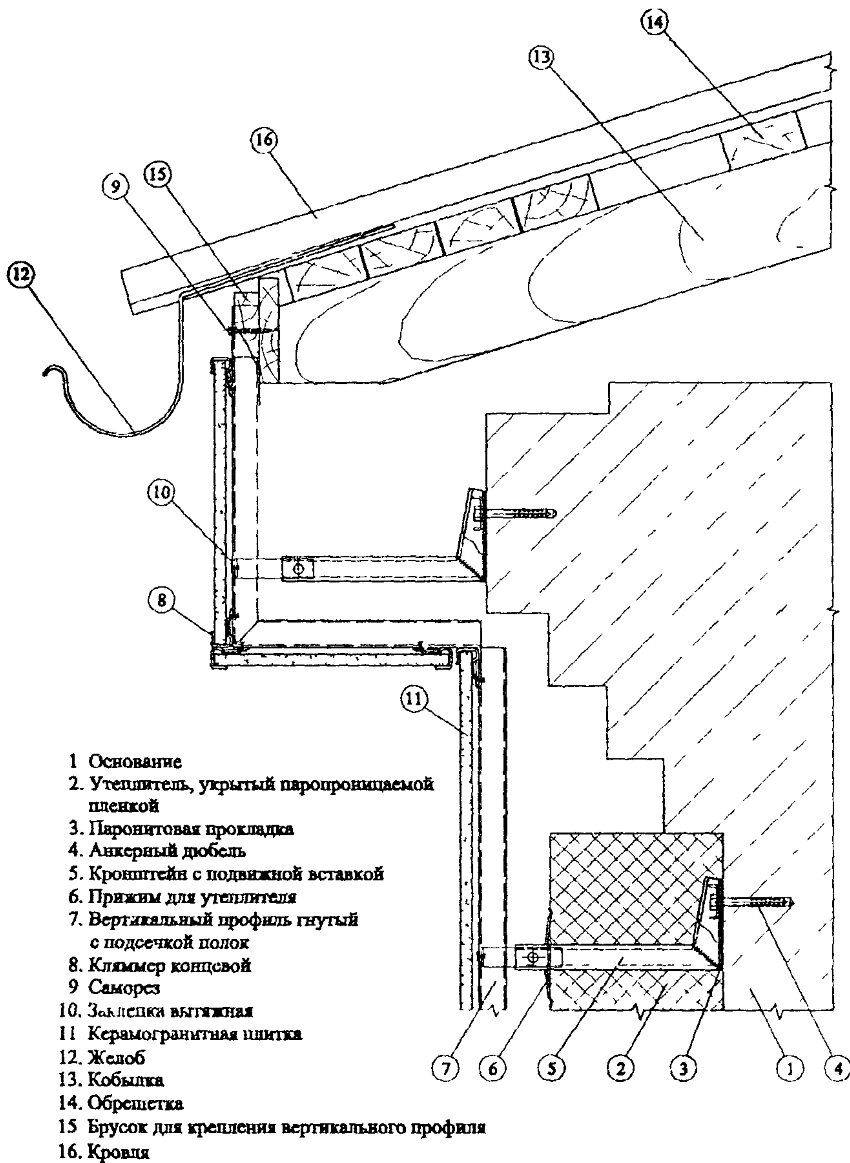
Рис. 3.28. Фасадная система "Диаг" СД-01 у карниза
