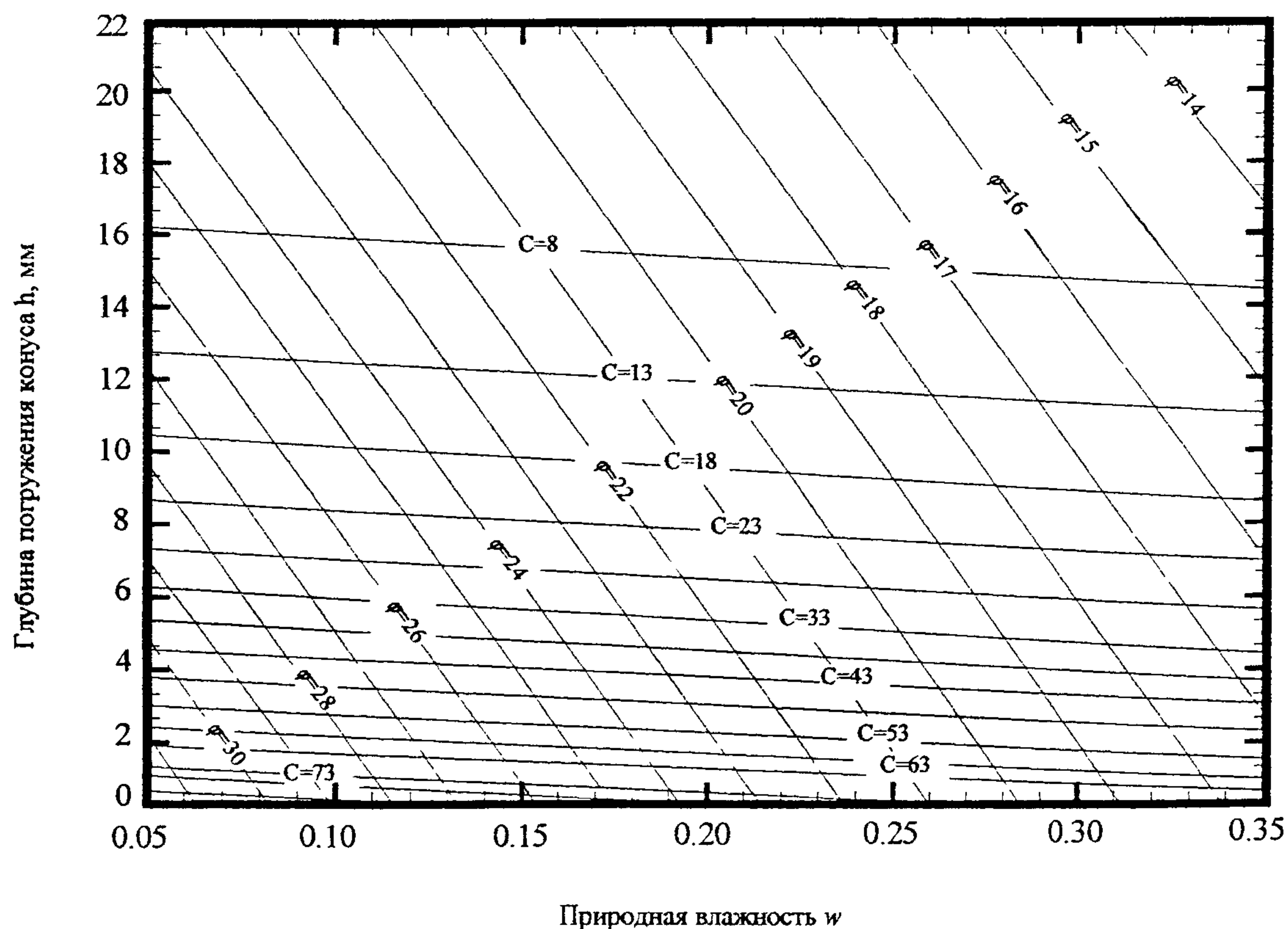
Рисунок Е.7 – Номограмма для определения удельного сцепления c , кПа, и угла внутреннего трения \varphi , град., ледниковых (моренных) глинистых грунтов
