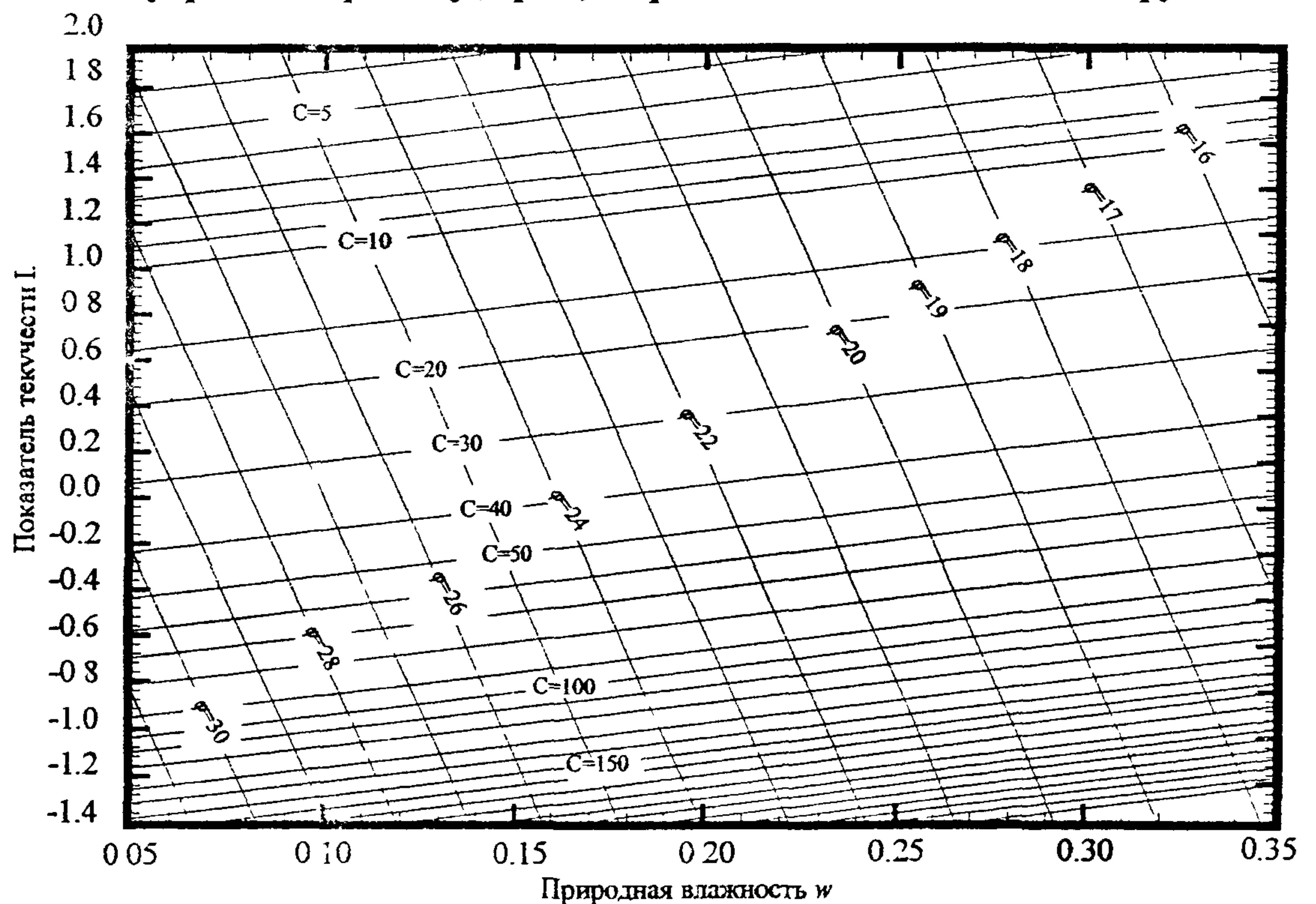
Рисунок Е.2 – Номограмма для определения сцепления c_n , кПа и угла внутреннего трения \varphi_n , град., ледниковых (моренных) глинистых грунтов
