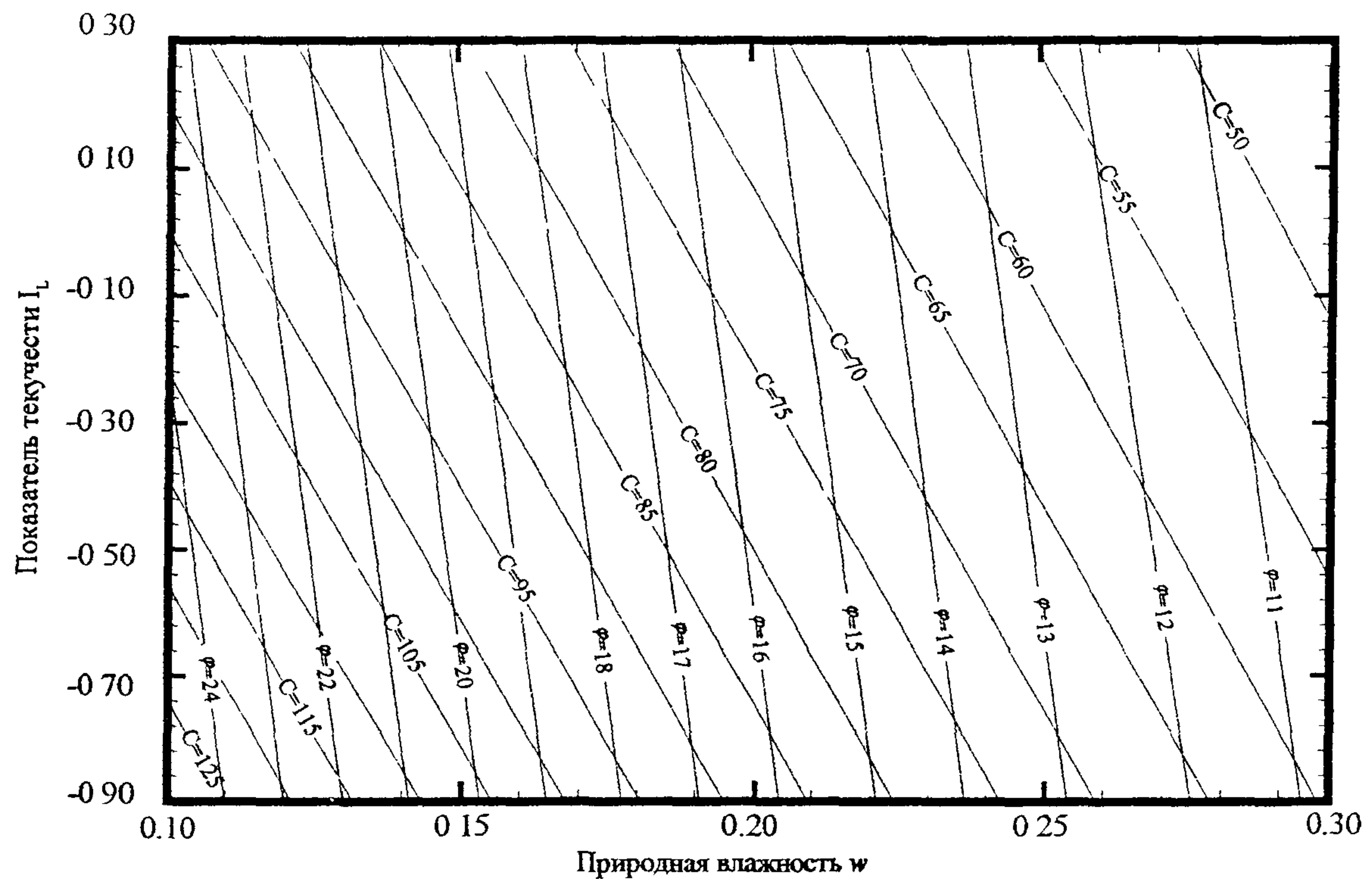
Рисунок Е.3 – Номограмма для определения сцепления c , кПа, и угла внутреннего трения \varphi , град., нижнекембрийских глинистых грунтов
