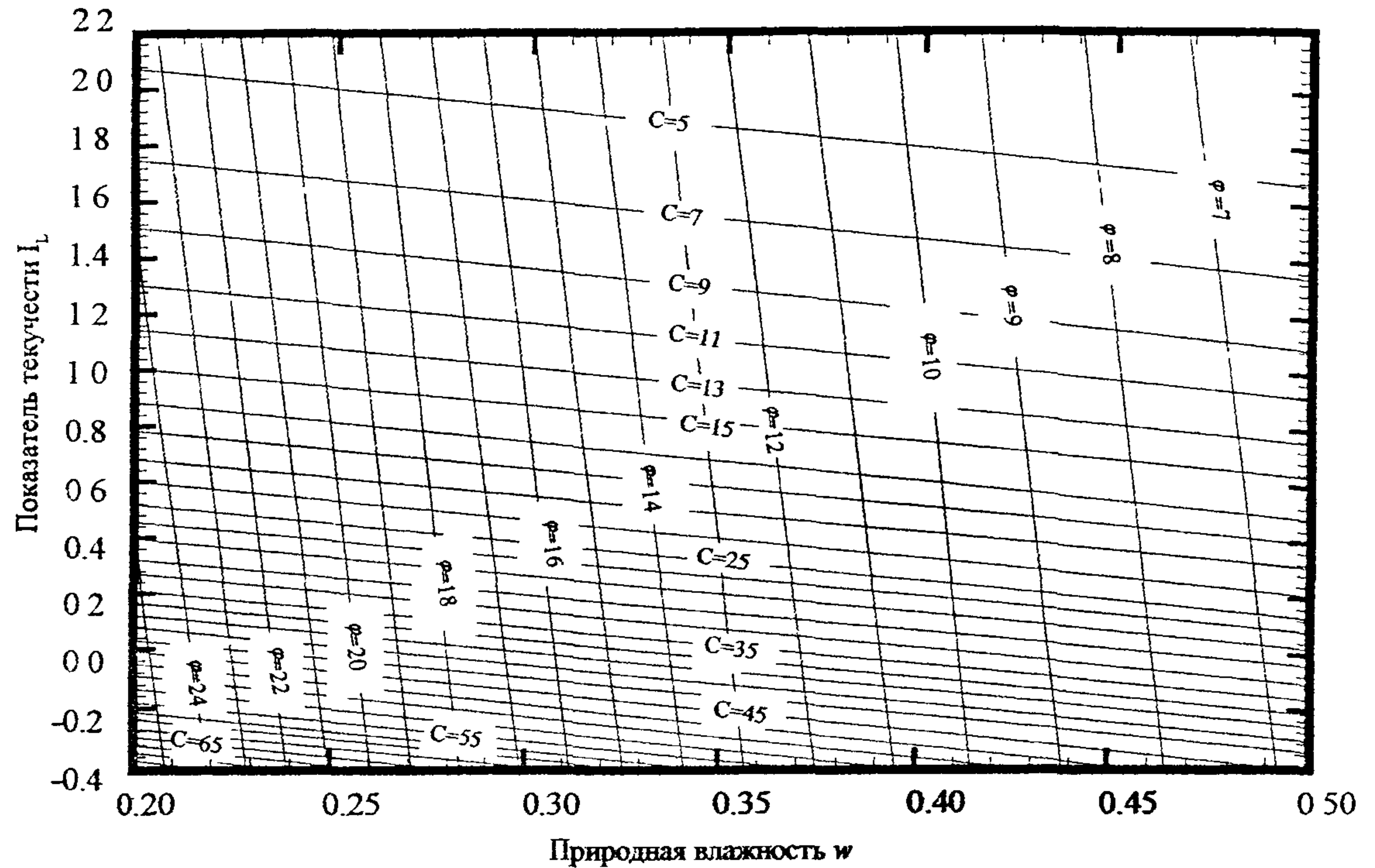
Рисунок Е.1 – Номограмма для определения удельного сцепления c_n , кПа и угла внутреннего трения \varphi_n , град., озерно-ледниковых глинистых грунтов
