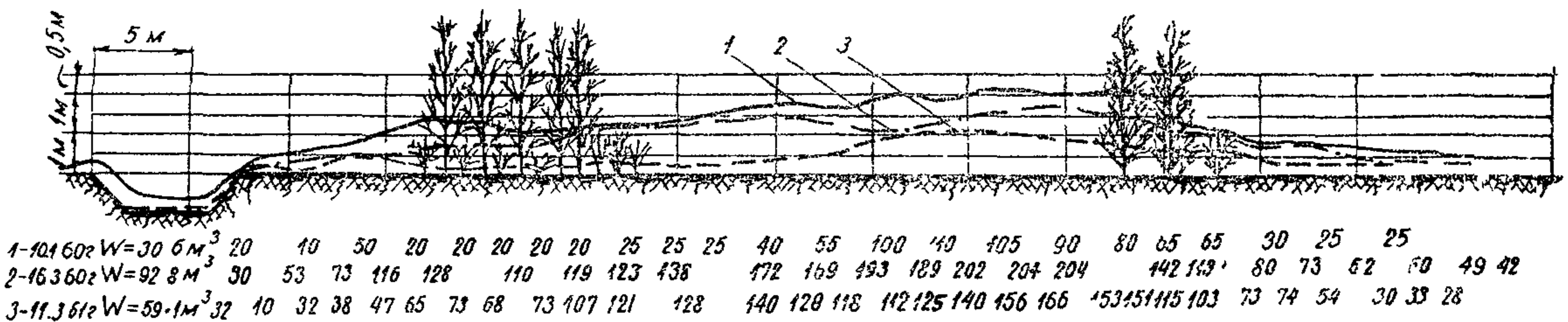
Рис. 6. Эффективность 3-рядной дополнительной полосы, усиливающей производственную 12-рядную полосу (Москва-Куйбышев, км 602-900)
