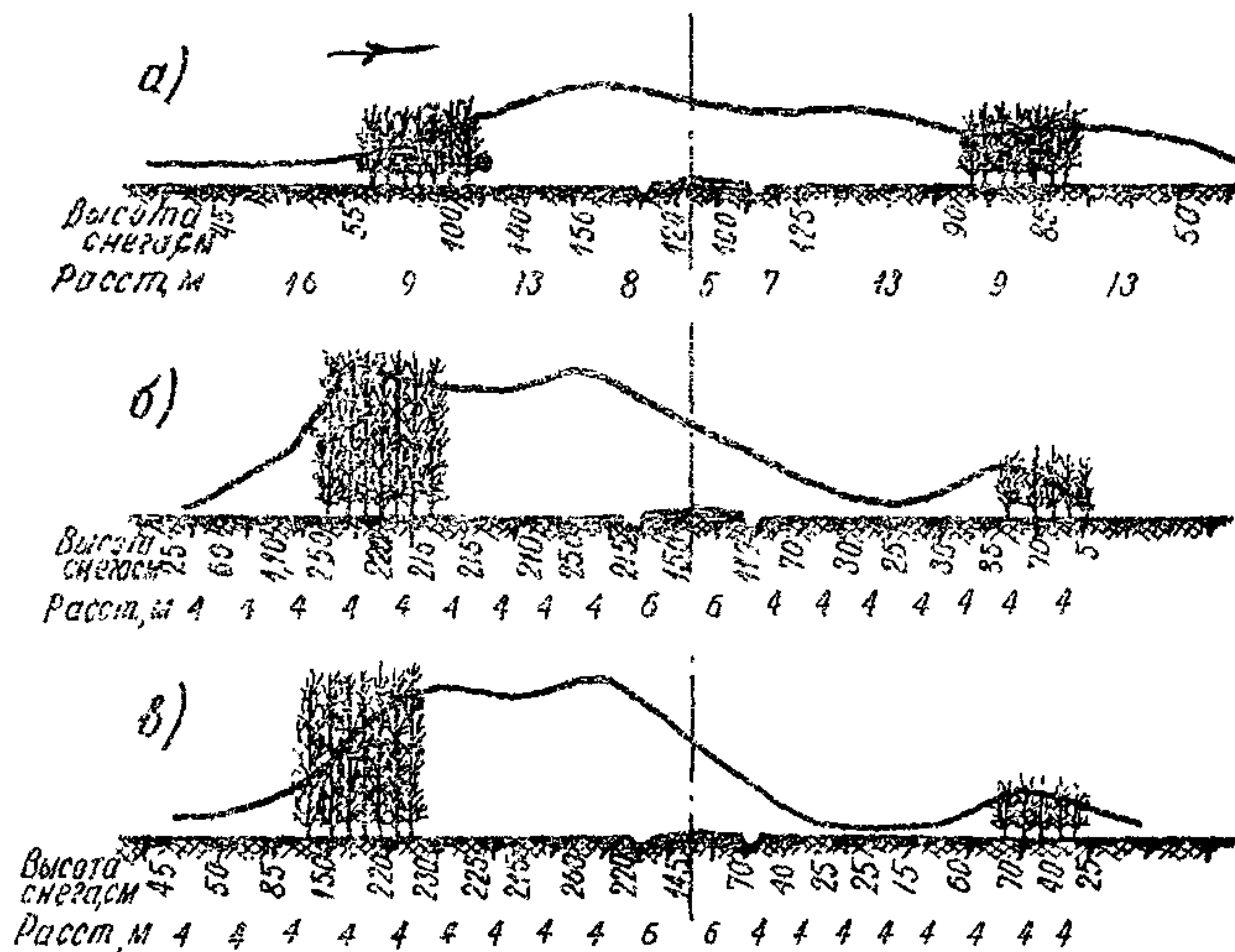
Рис. I. Снежные заносы при близком размещении снегозадерживающих полос к дороге Москва-Харьков. Стрелка показывает направление ветра
