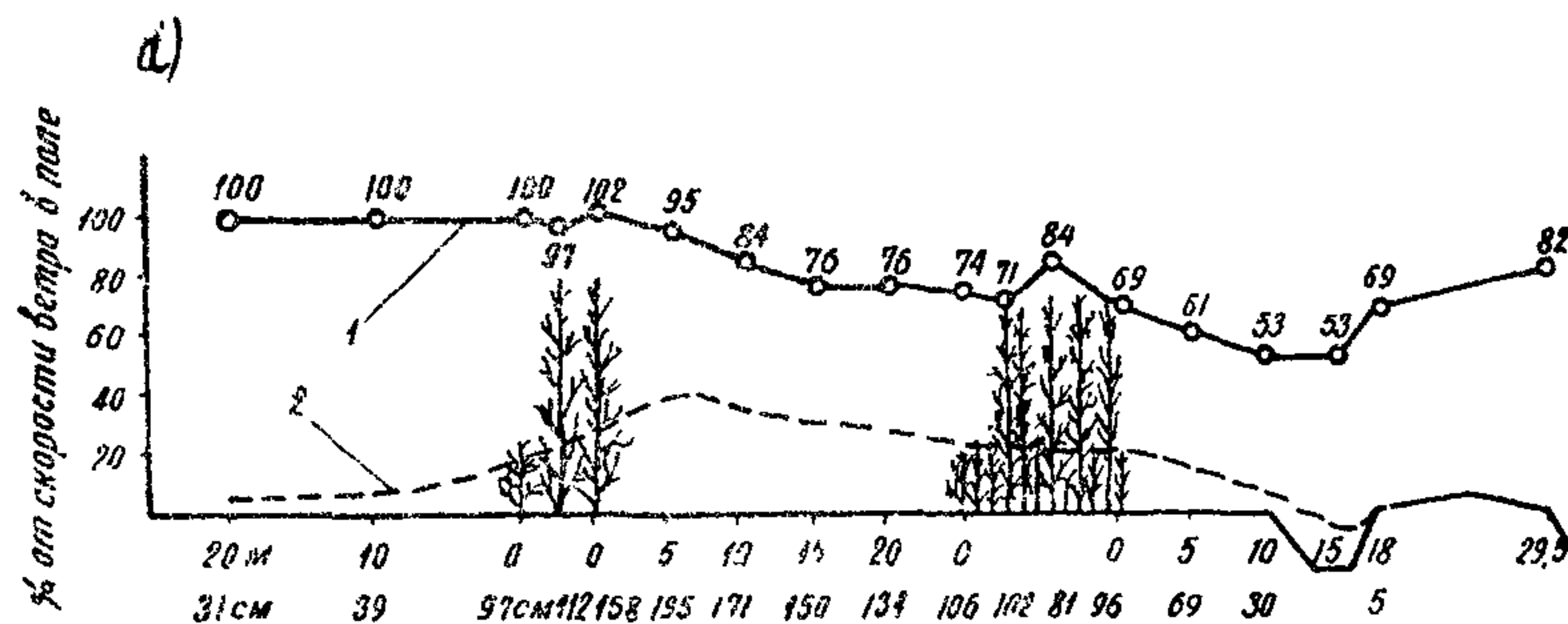
Рис. 5. Скорость ветра у дополнительной 43-рядной опытной полосы (слева) при перпендикулярном (а) и косом (б) направлениях ветра. 1- скорость ветра на высоте 14 см; 2- снегоотложение
