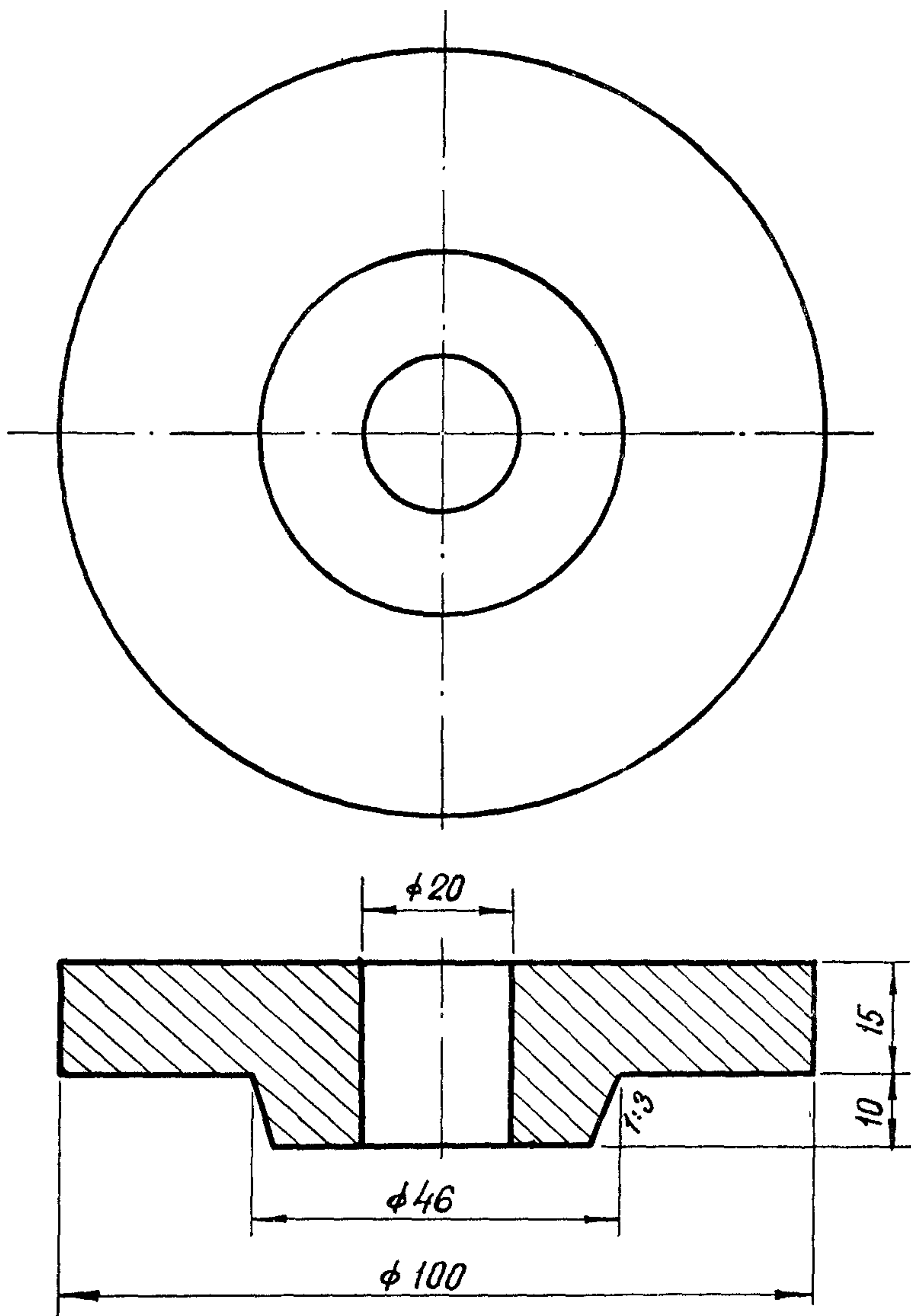
Рис. 4. Поданкерная шайба для плит ПАГ-Х1У (материал Ст.-3)
