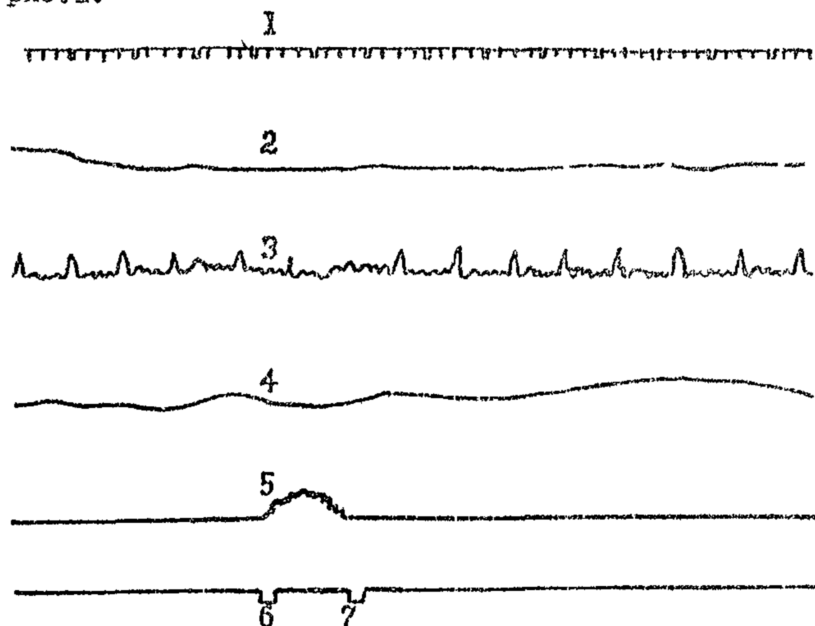
Рис. I. Психофизиологические показатели водителя и режимы движения на участке смены полосы движения: 1— путь; 2— скорость; 3— ЭКГ; 4— КГР; 5— поперечное ускорение; 6 и 7— соответственно начало и конец маневрирования автомобиля
