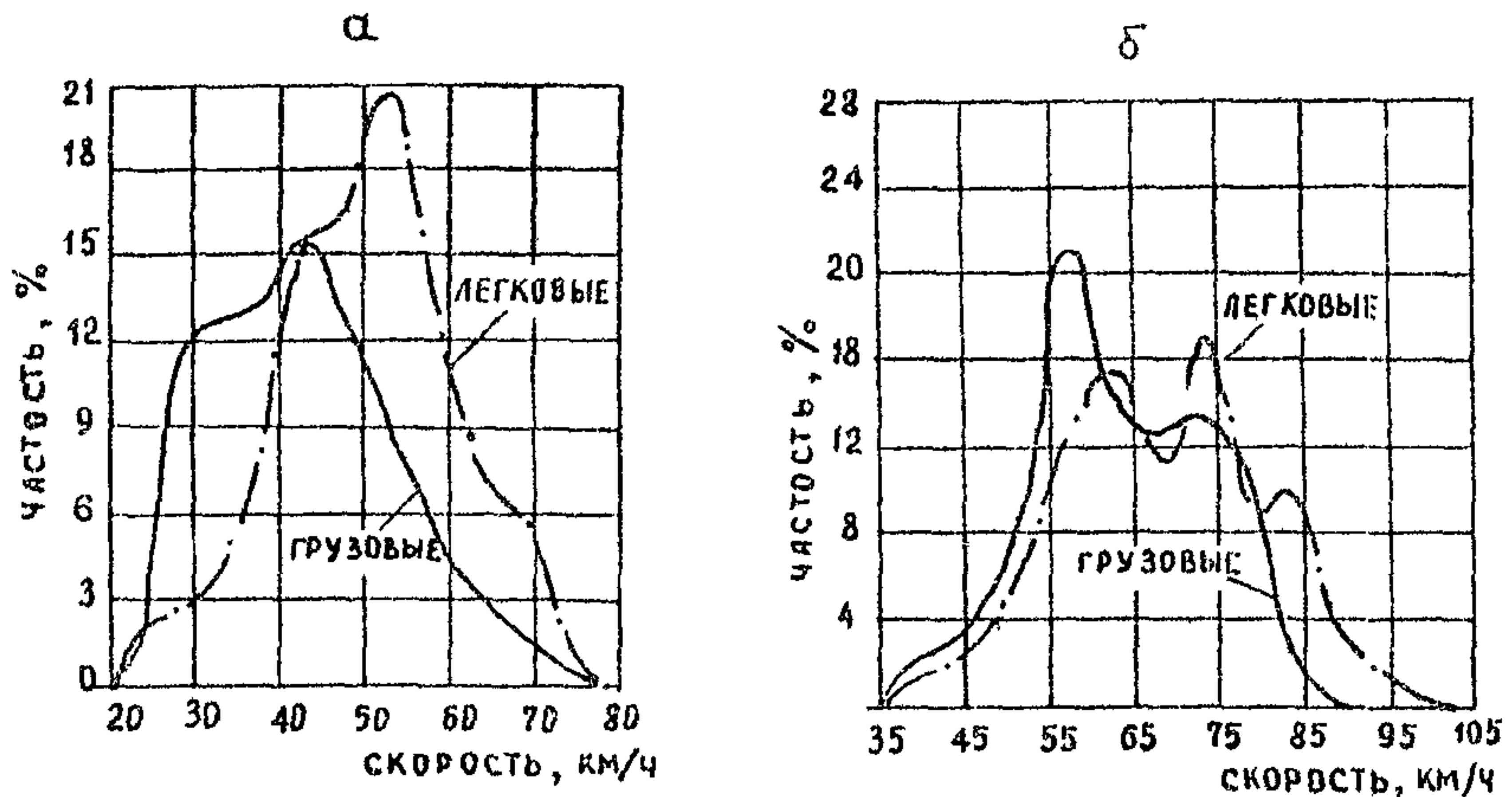
Рис.3. Распределение скоростей движения автомобилей в зимнее время: а – снежный накат; б – чистое асфальтобетонное покрытие
