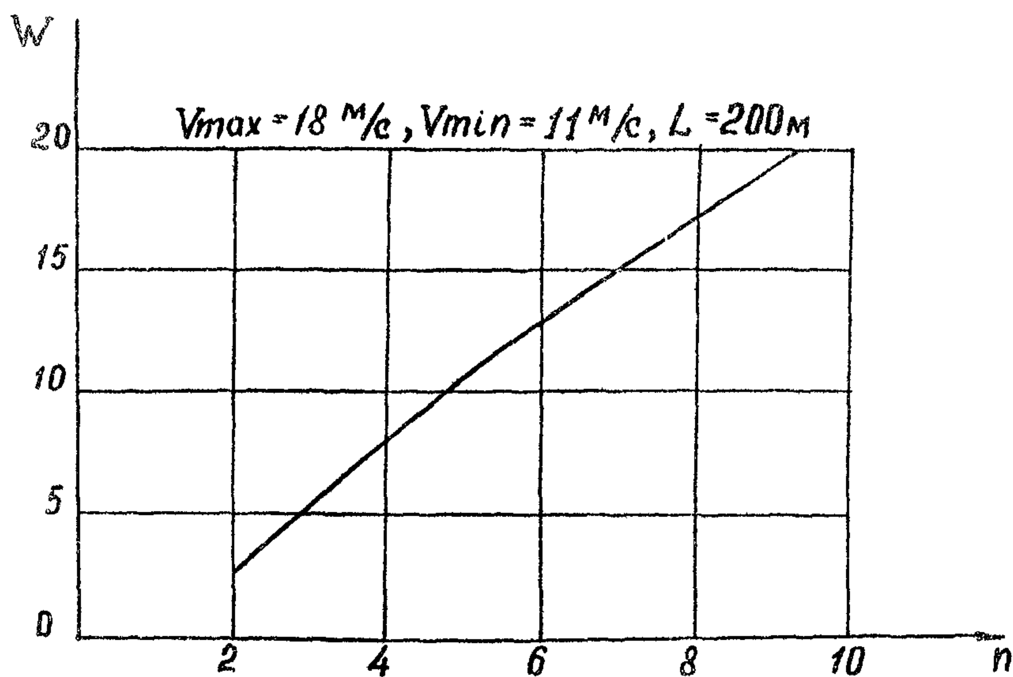
Рис.2. Зависимость средней длительности группы от количества автомобилей
