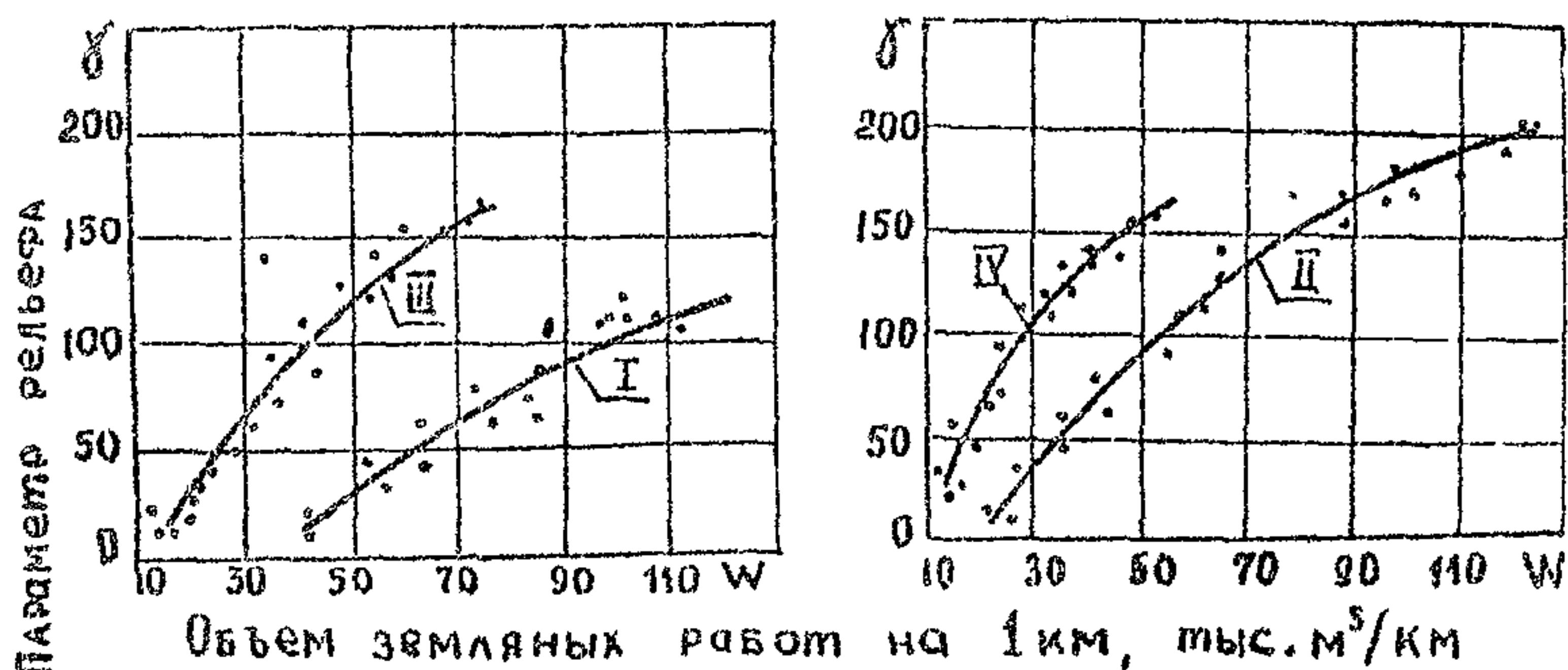
Рис.1. Зависимость W = f(\gamma) для I, II, III, IV -технических категорий дороги
