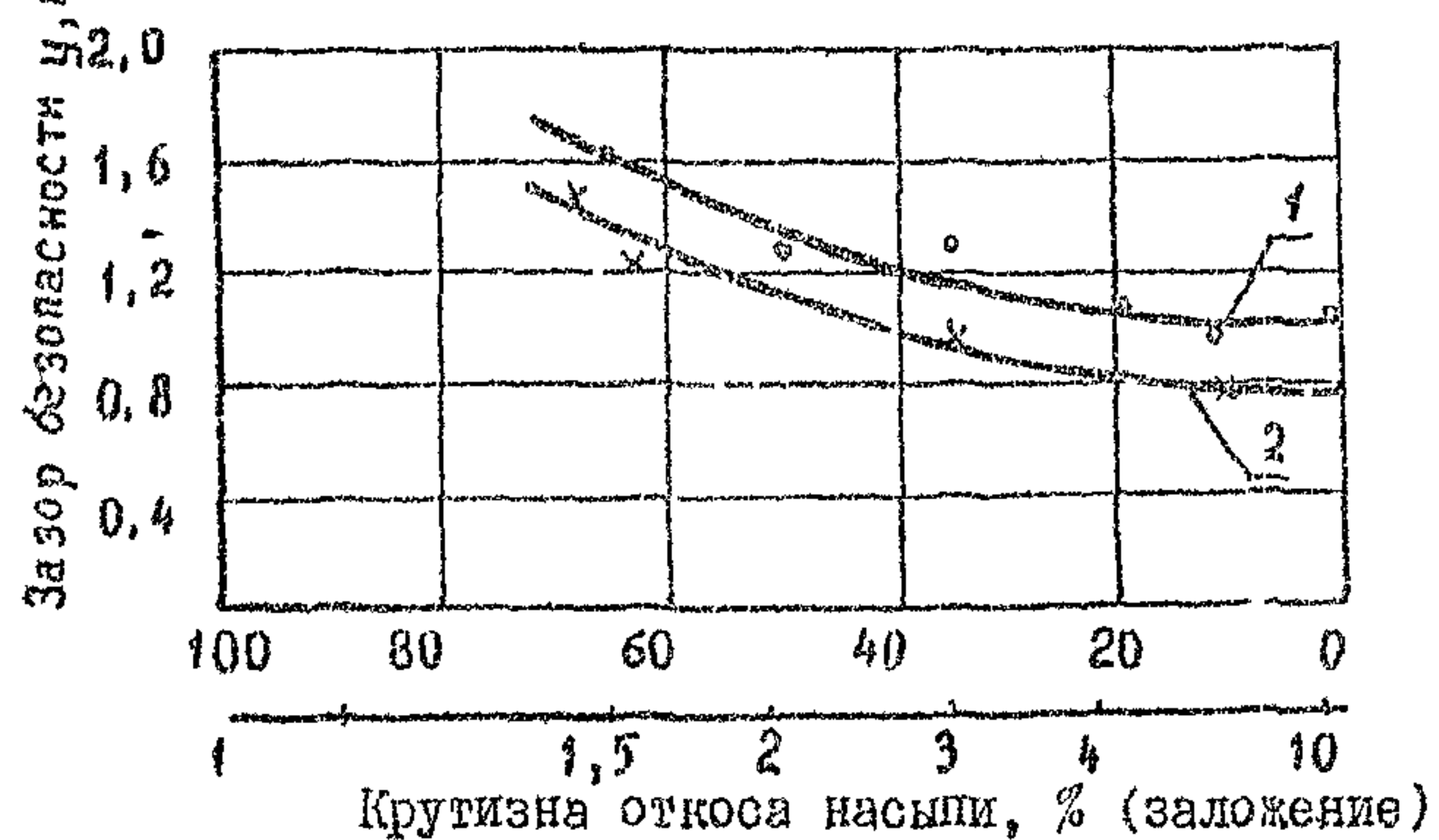
Рис.1. Зависимость зазора безопасности y от крутизны откоса насыпи при движении: 1 — на спуск; 2 — на подъем
