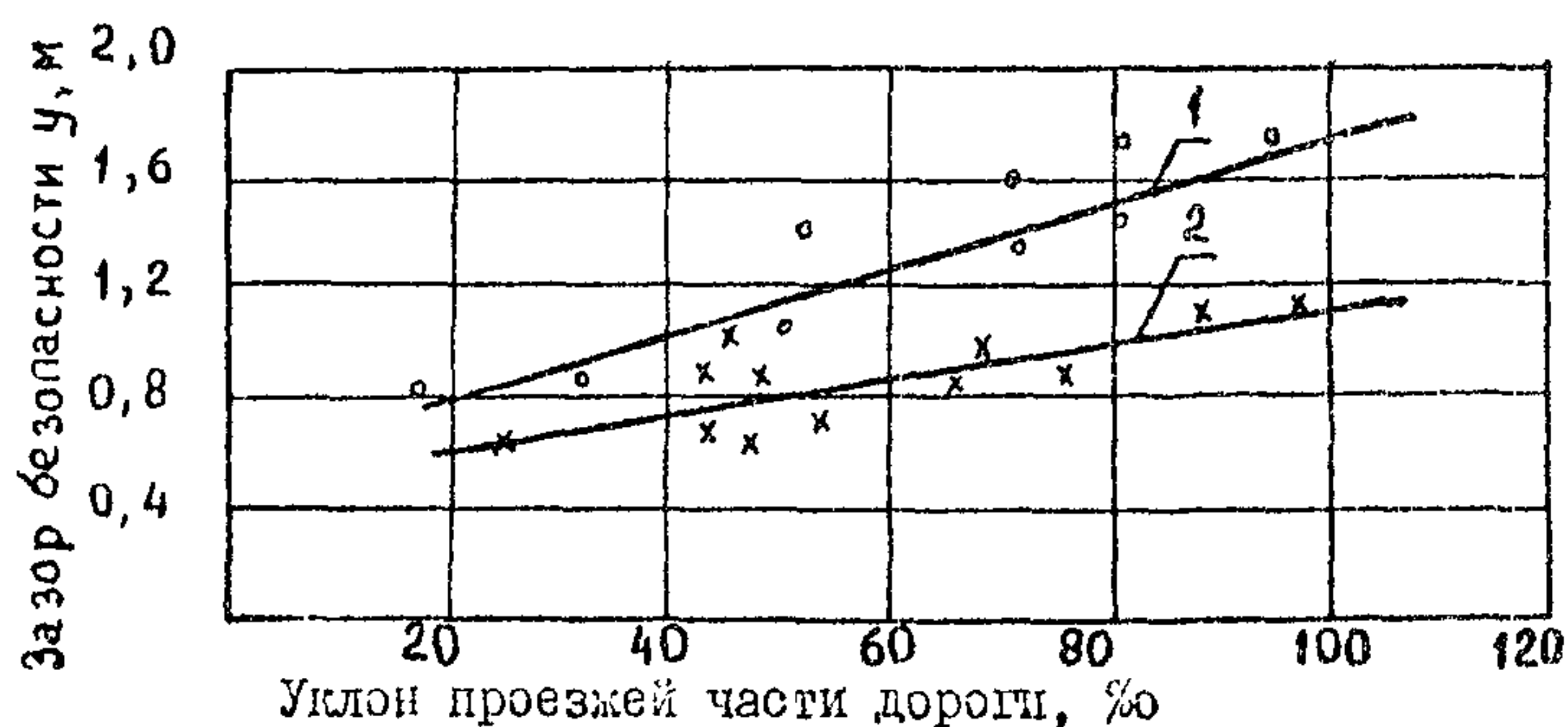
Рис.3. Зависимость зазора безопасности y от продольного уклона проезжей части дороги при движении: 1- на спуск; 2- на подъем
