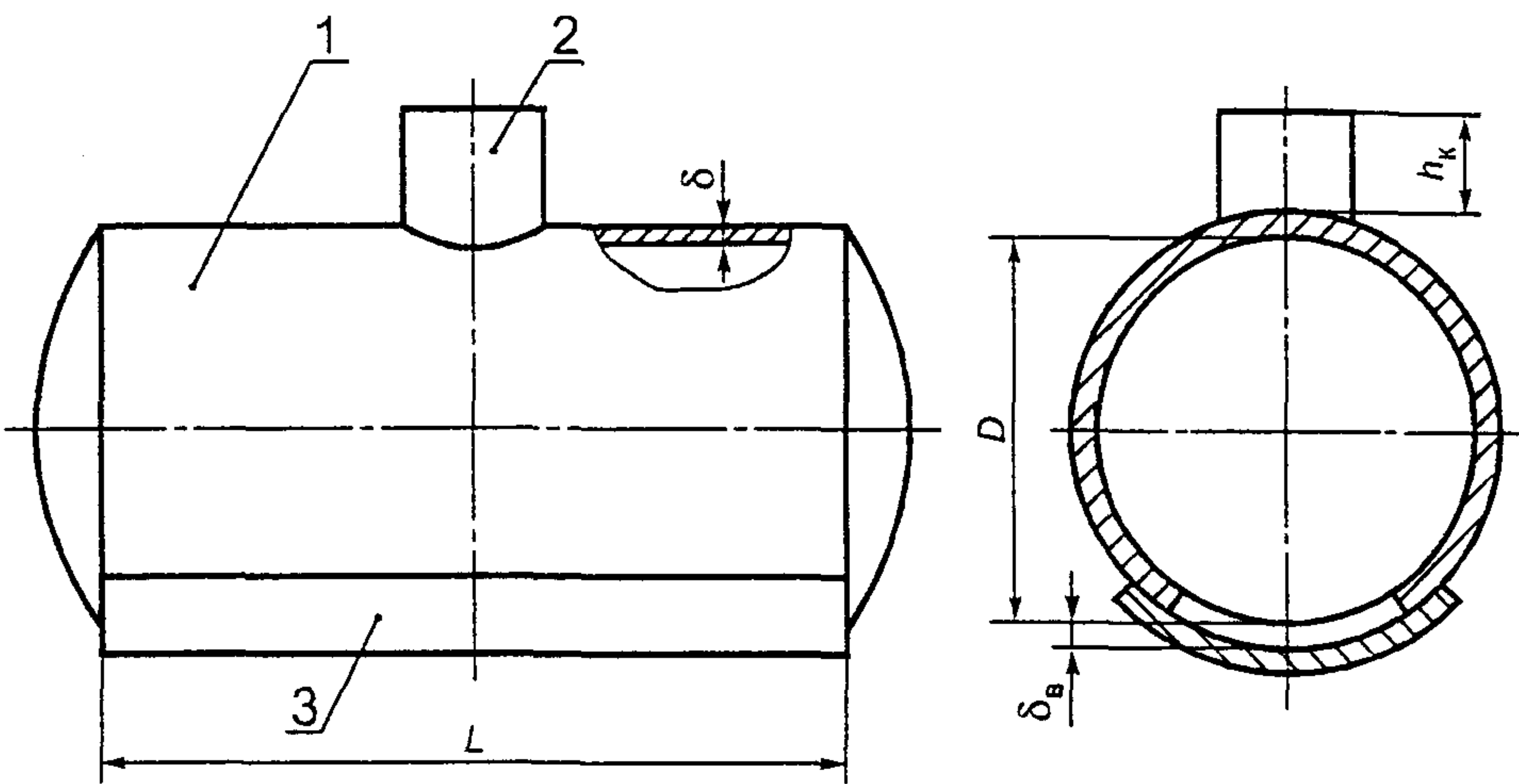
1 — котел цистерны; 2 — колпак; 3 — ванночка
