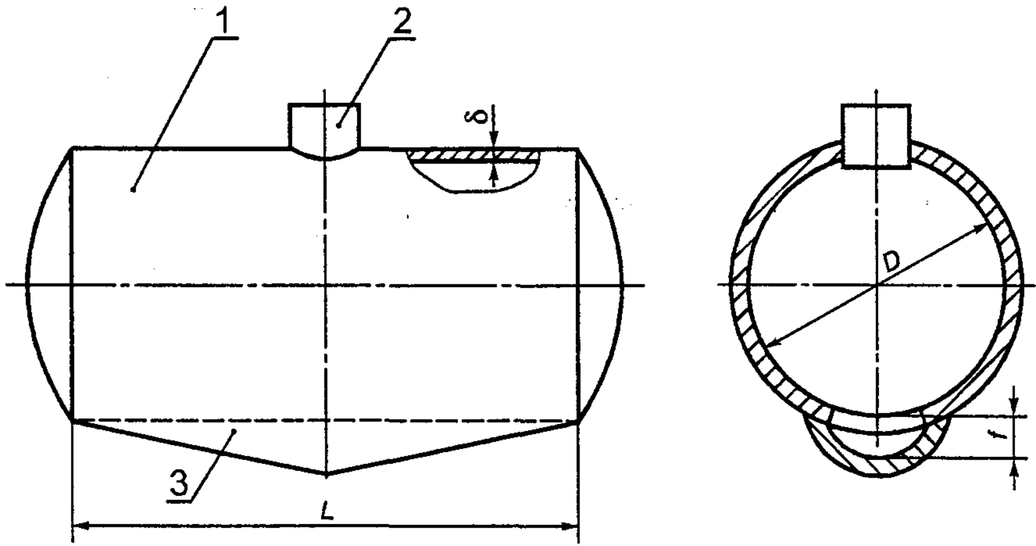
1 — котел цистерны; 2 — горловина; 3 — выштамповка уклона
