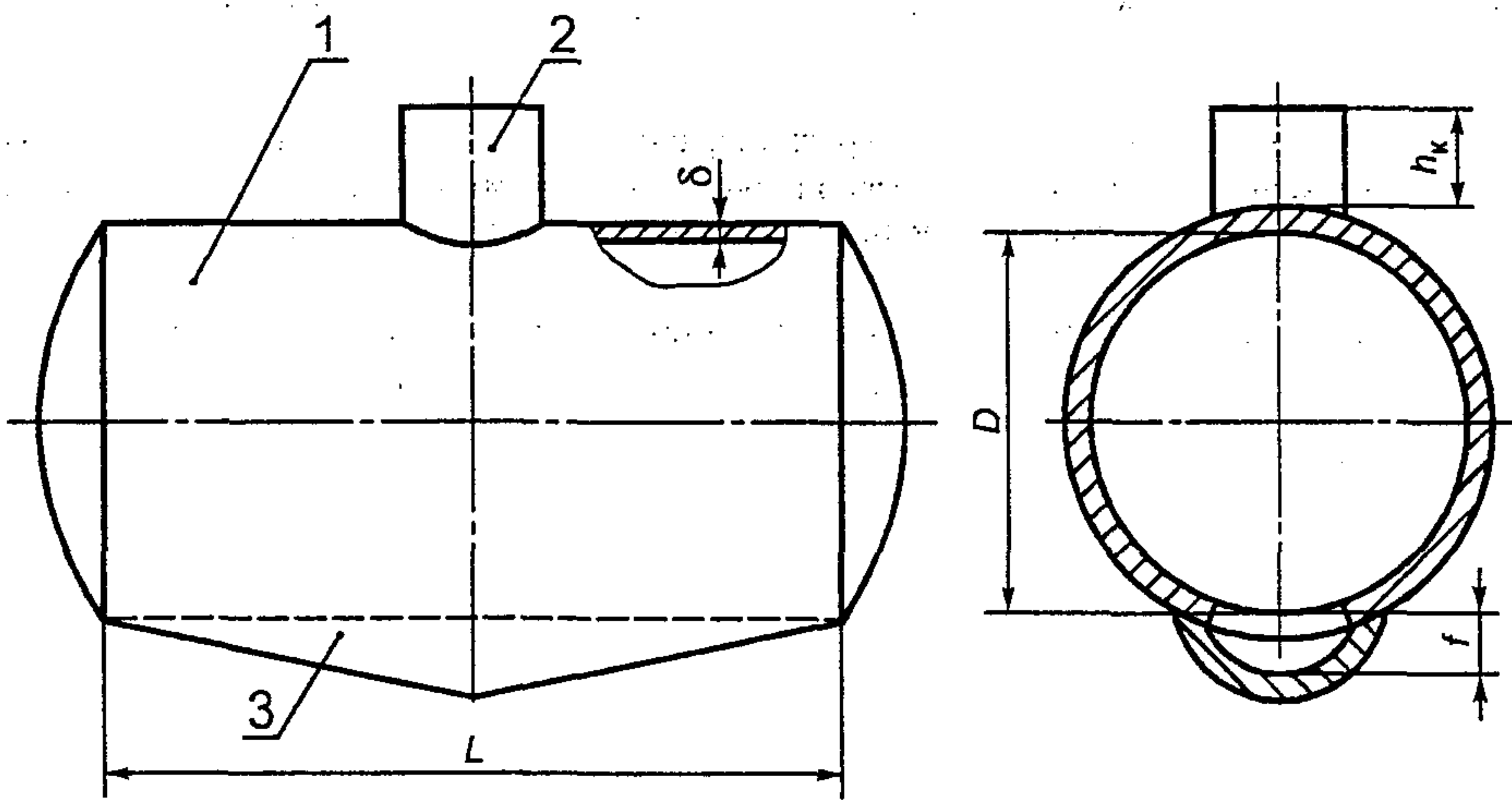
1 — котел цистерны; 2 — колпак; 3 — выштамповка уклона
