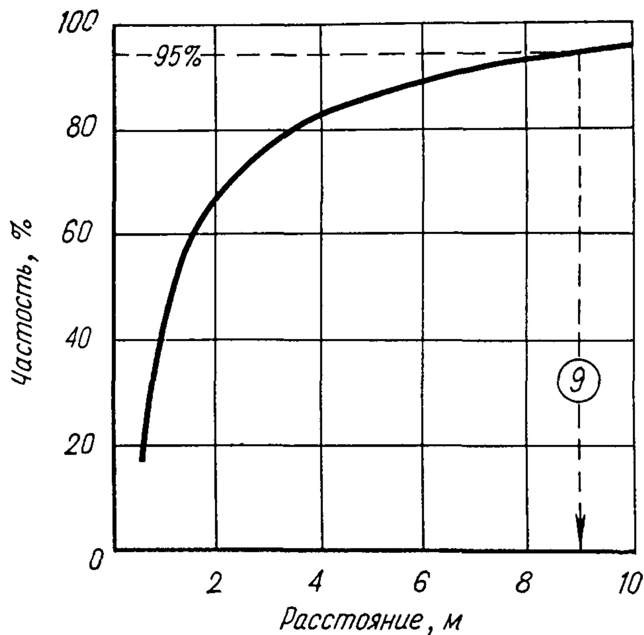
Рис. 13. Распределение количества автомобилей, съезжающих с откосов насыпей
