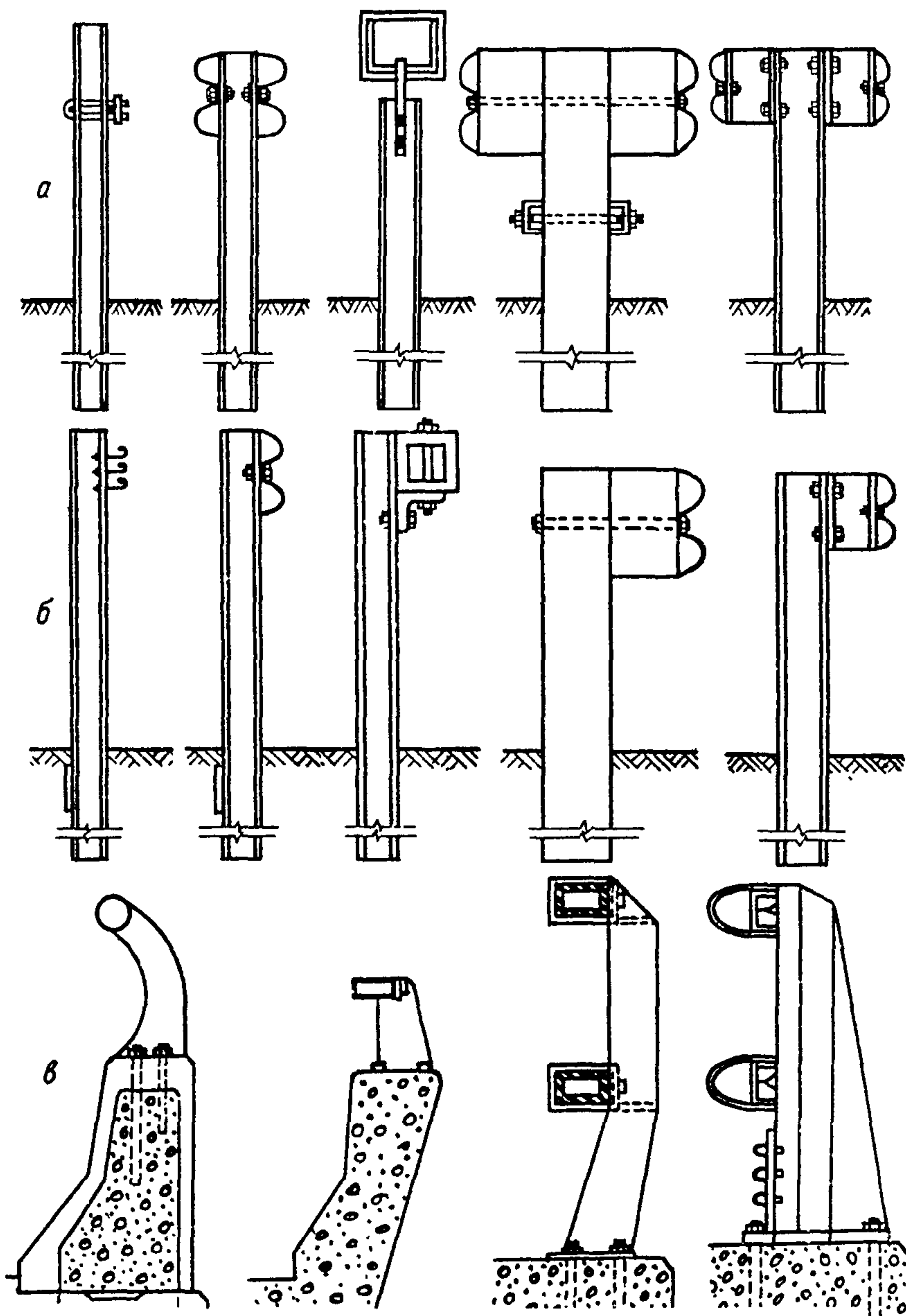
Рис. 6. Металлические ограждения, устанавливаемые на: а - разделительных полосах; б - обочинах дорог; в - мостах и путепроводах
