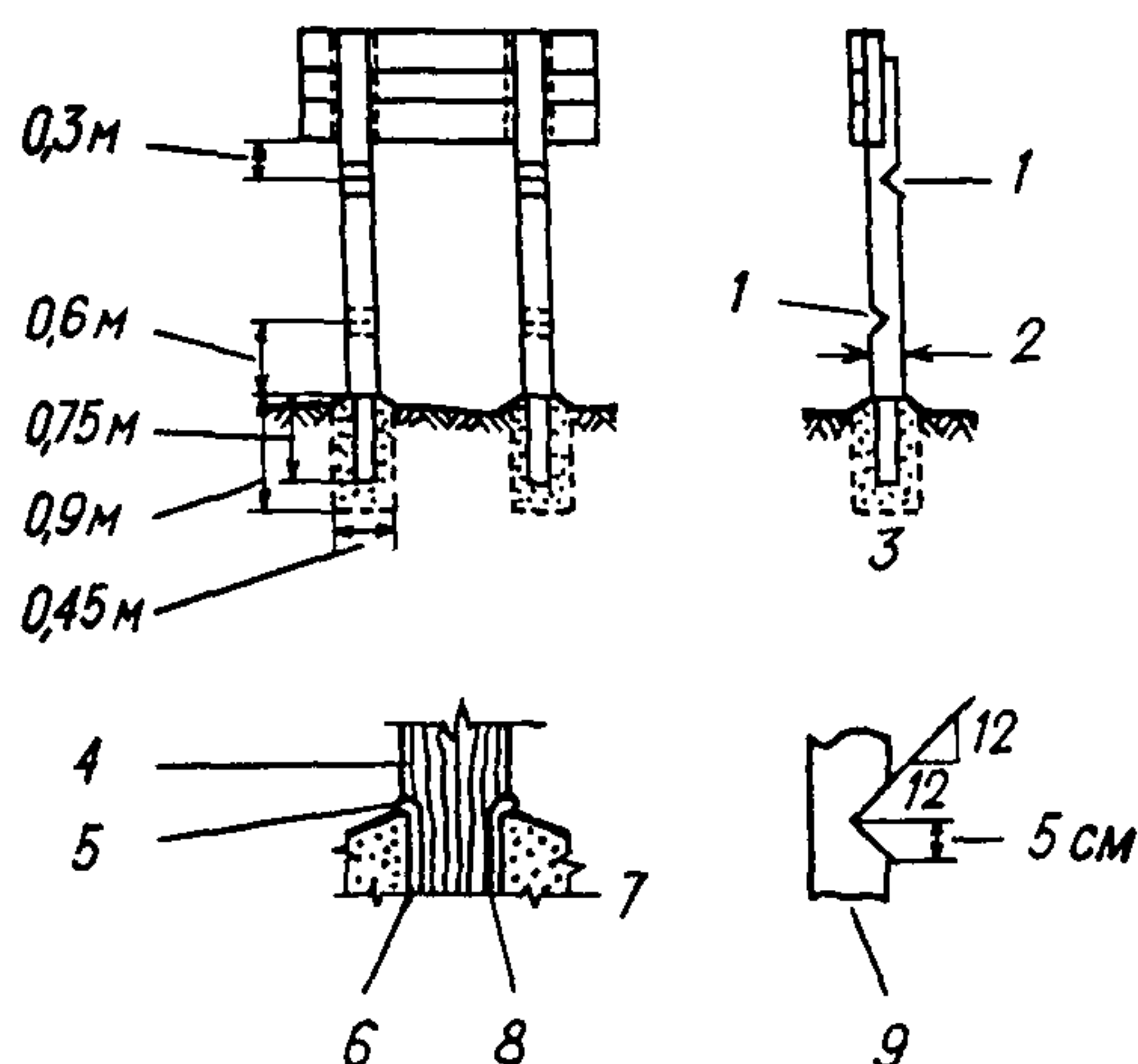
Рис. 7. Конструкция знака с деревянными разрушающимися опорами: 1 – надрез; 2 – номинальный диаметр 20 см; 3 – вид сбоку; 4 – деревянная стойка; 5 – битумная изоляция; 6 – оцинкованное железо; 7 – мастика; 8 – сечение по опорной части; 9 – деталь надреза
