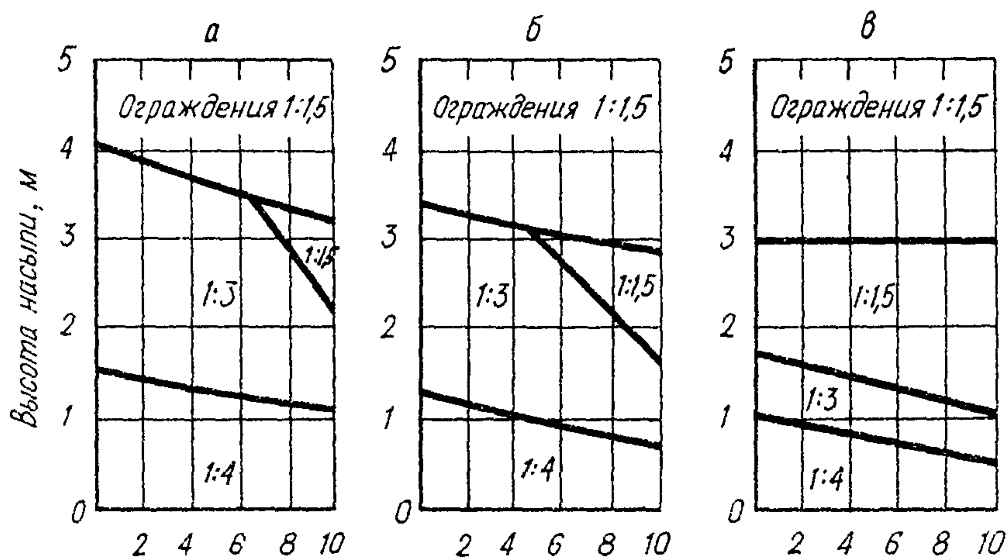
Рис. 17. Рекомендуемая крутизна откосов насыпи на дорогах III технической категории при возведении земляного полотна из привозных грунтов. Затраты, отнесенные к 1 \text{ м}^3 грунта: а – 0,5 руб.; б – 1 руб.
