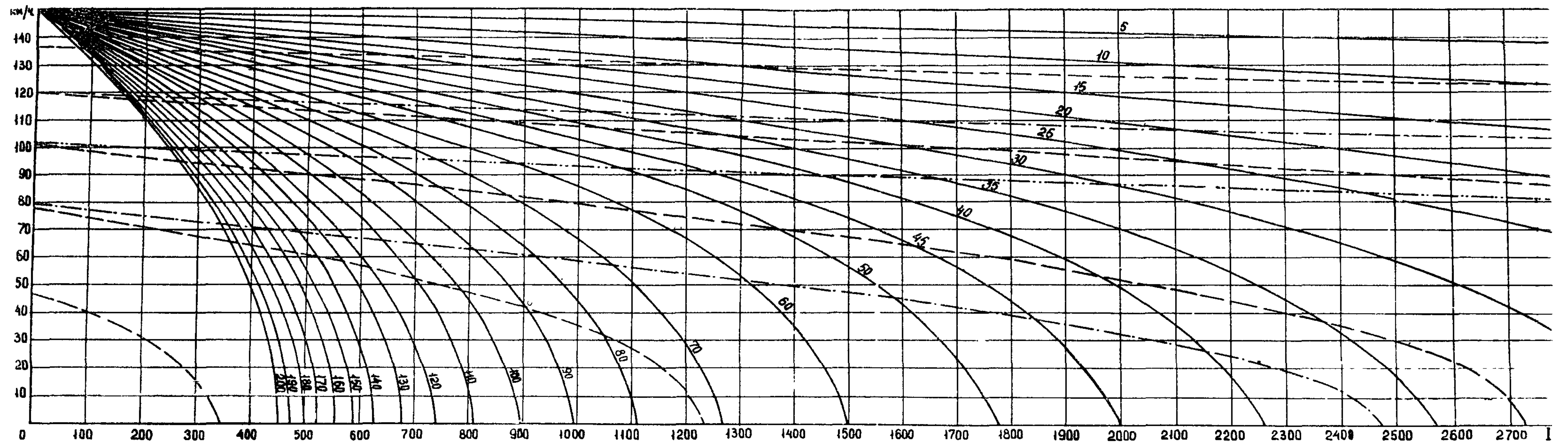
Рис. 7 График для определения инерционных расстояний
