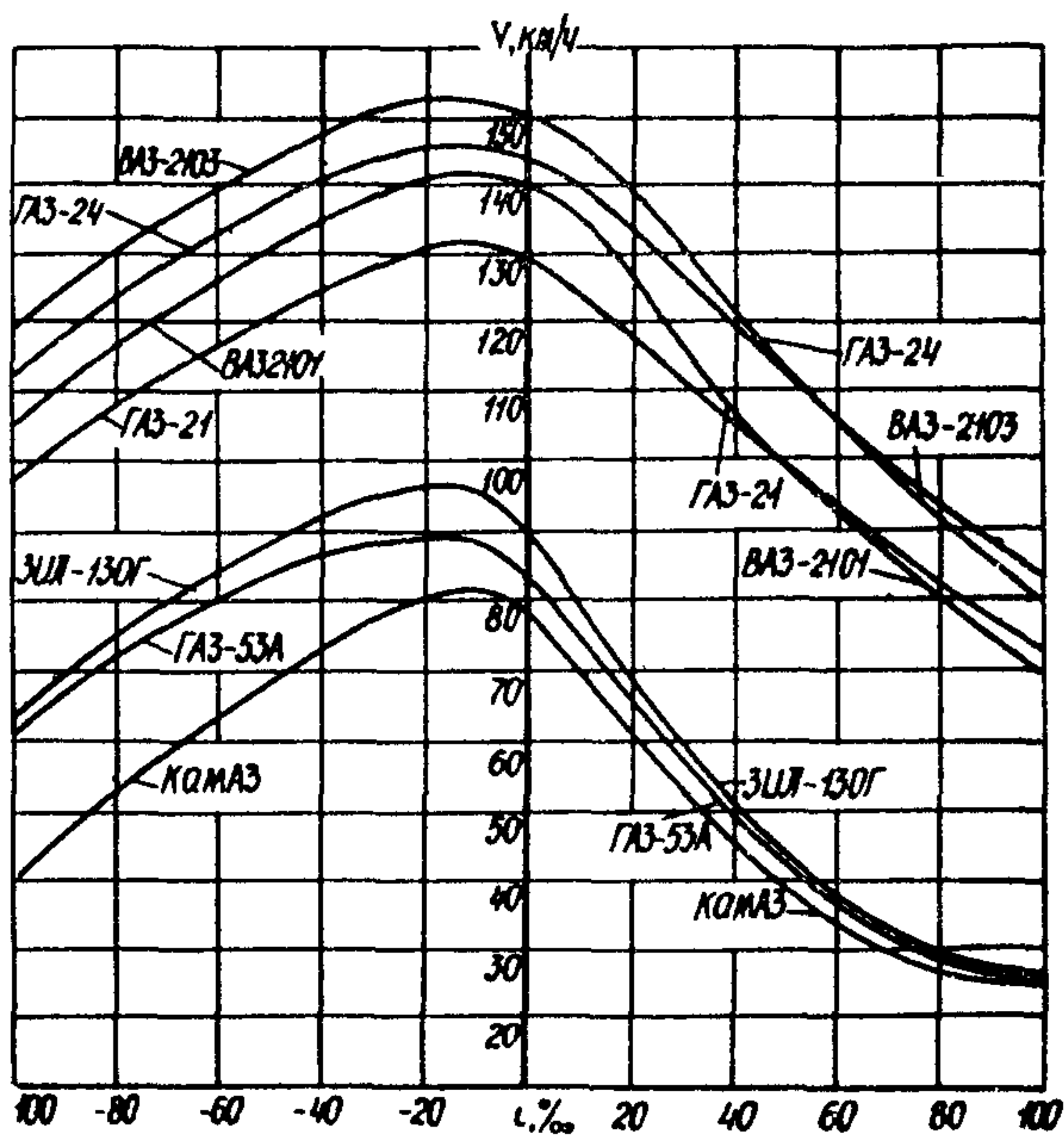
Рис.1. Графики для определения максимальных скоростей движения автомобилей в зависимости от продольных уклонов
