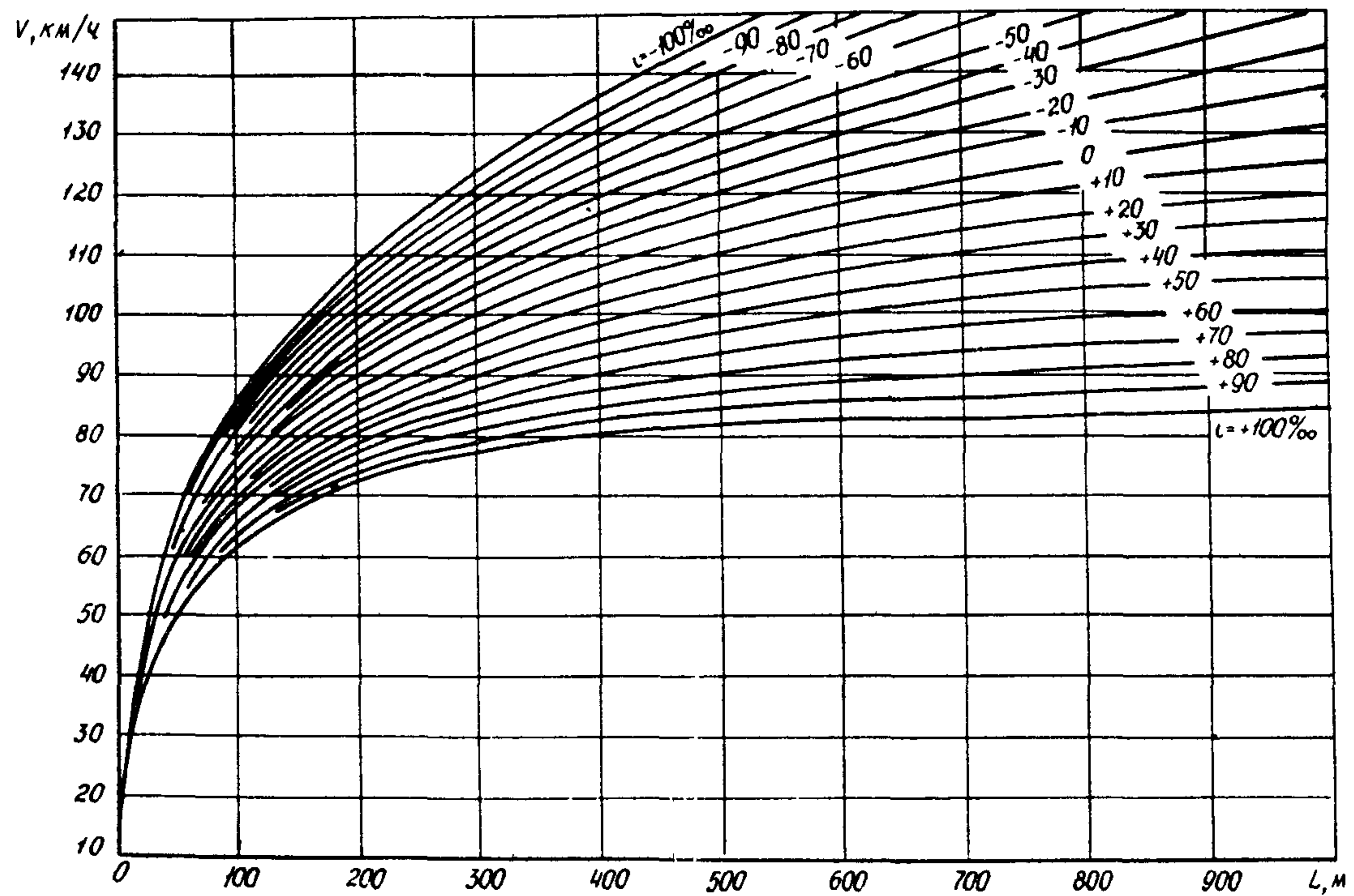
Рис. 2. Графики для определения путей разгона автомобиля ГАЗ-24
