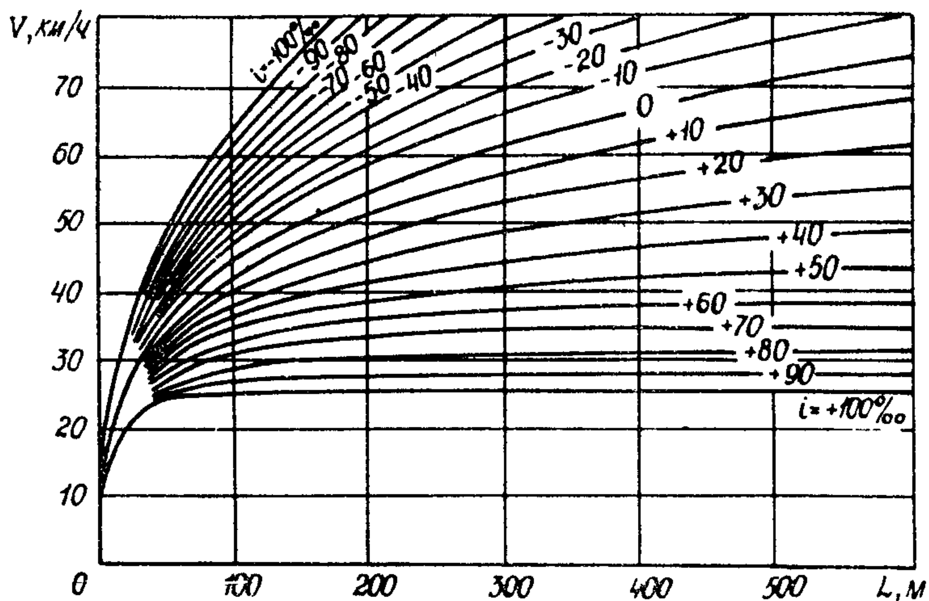
Рис.3. Графики для определения путей разгона автомобиля ЗИЛ-130
