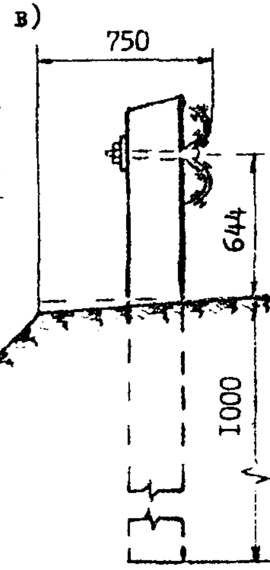
ю. 6.1. Схема крепления и конструктивные особенности металлических ограждений из прокатных профилей.
