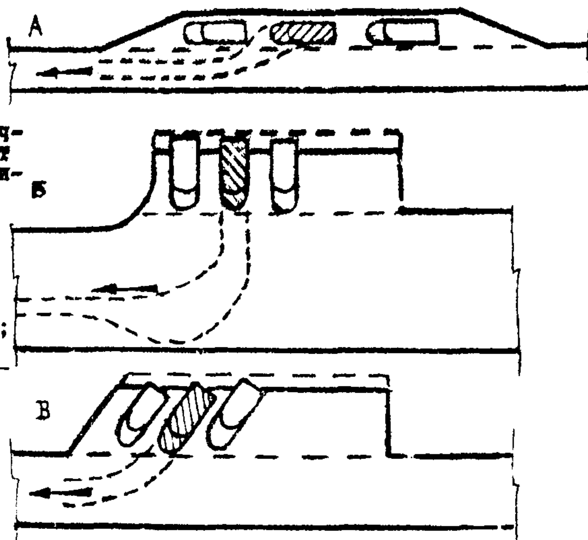
Рис. 3.22. Площадка для регулирования фар автомобилей определённых типов:
