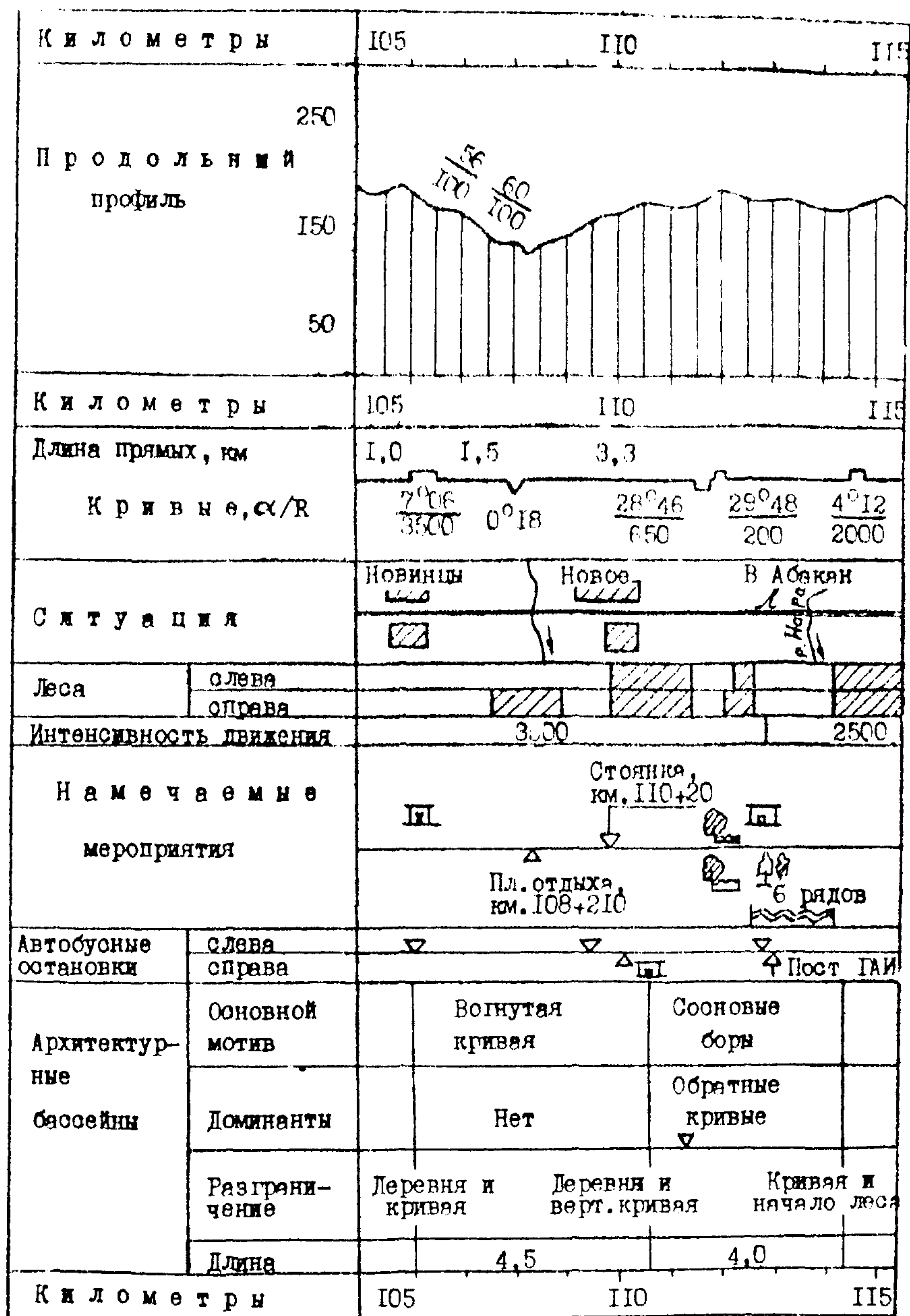
Рис. 3.1. Линейный архитектурный график дороги.
