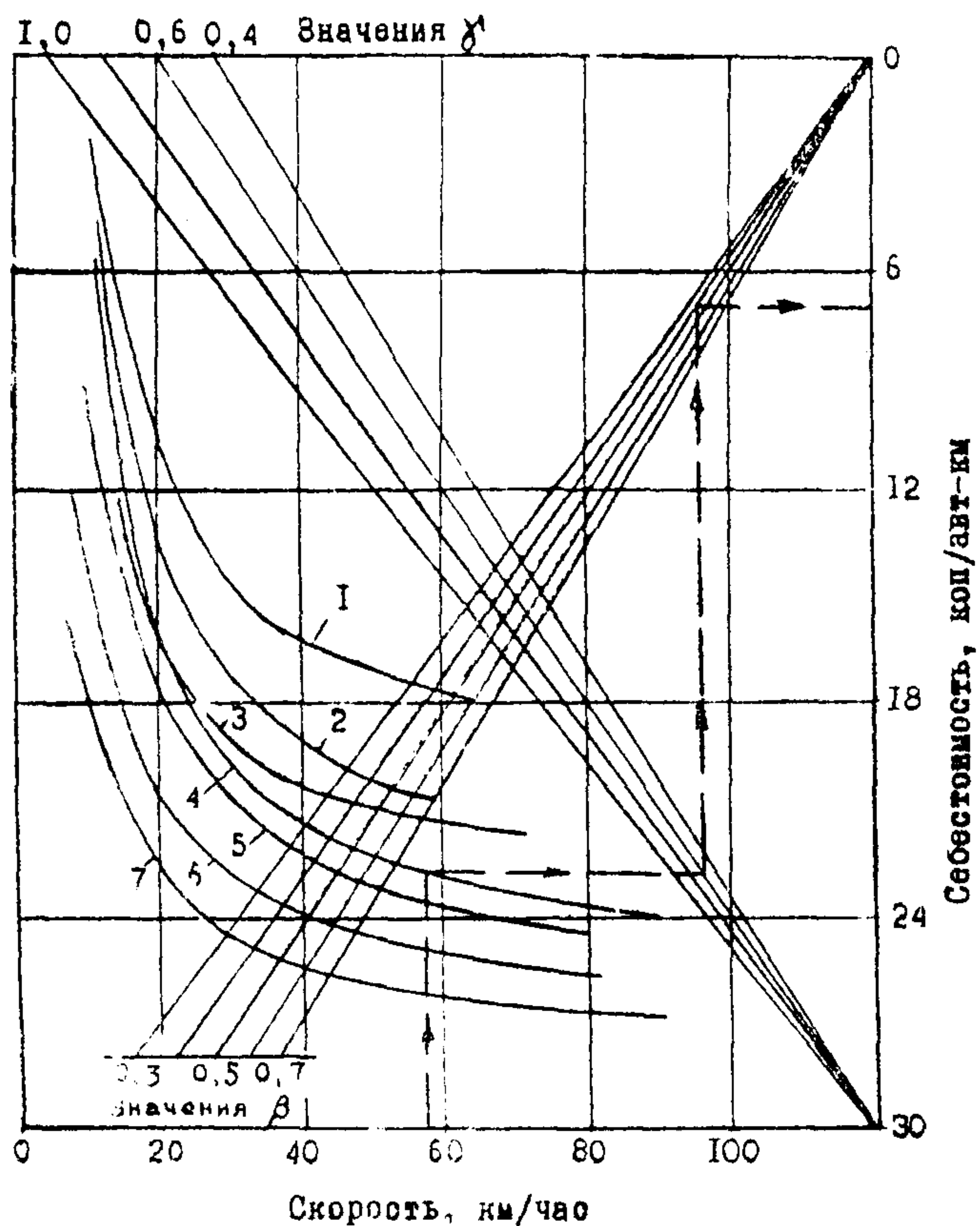
Фиг. 8.4. Номограмма для определения себестоимости I авт-км транспортной работы. Автомобили:
