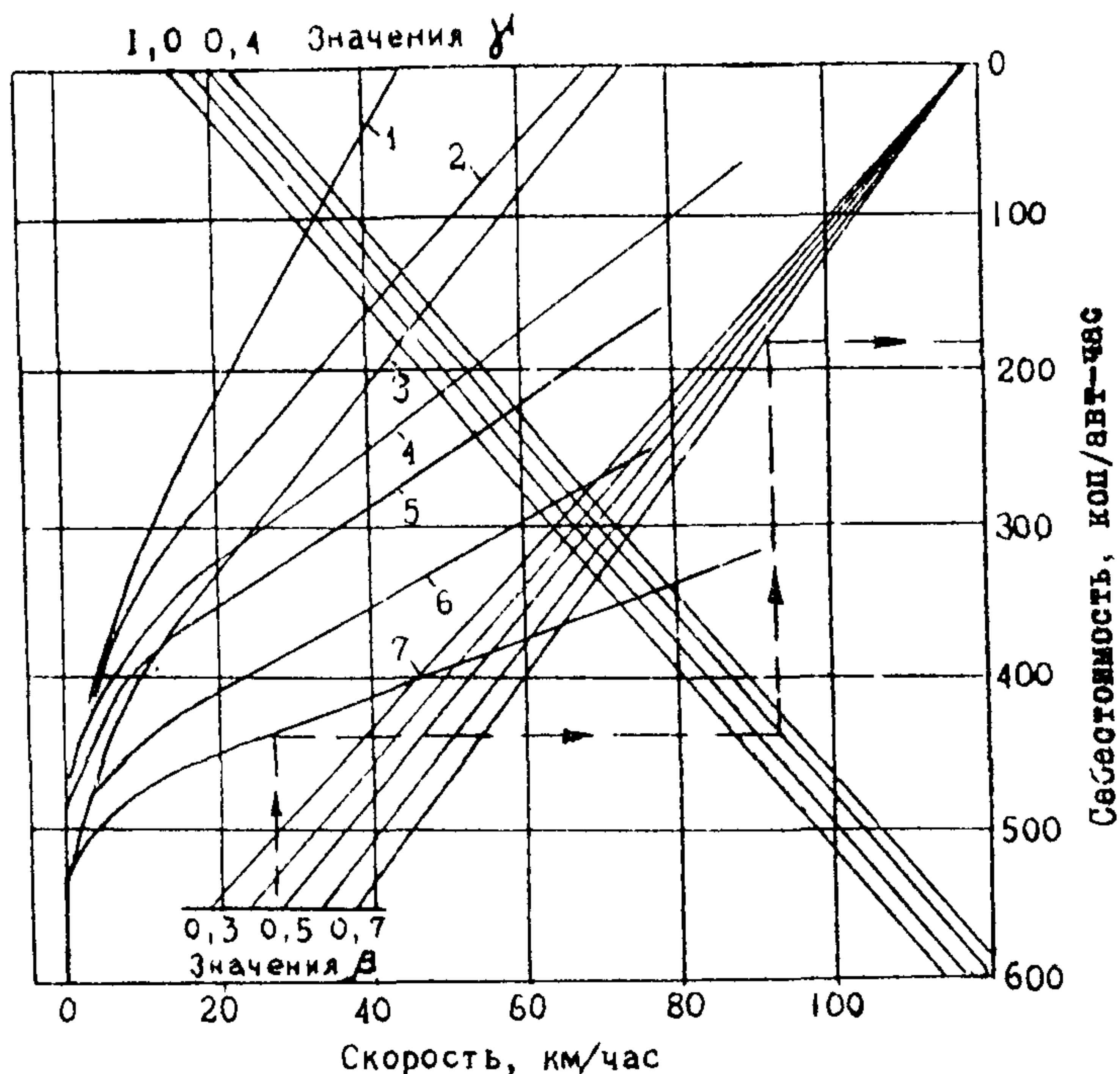
Рис. 8.5. Номограмма для определения себестоимости I авт-часов транспортной работы. Автомобили:
