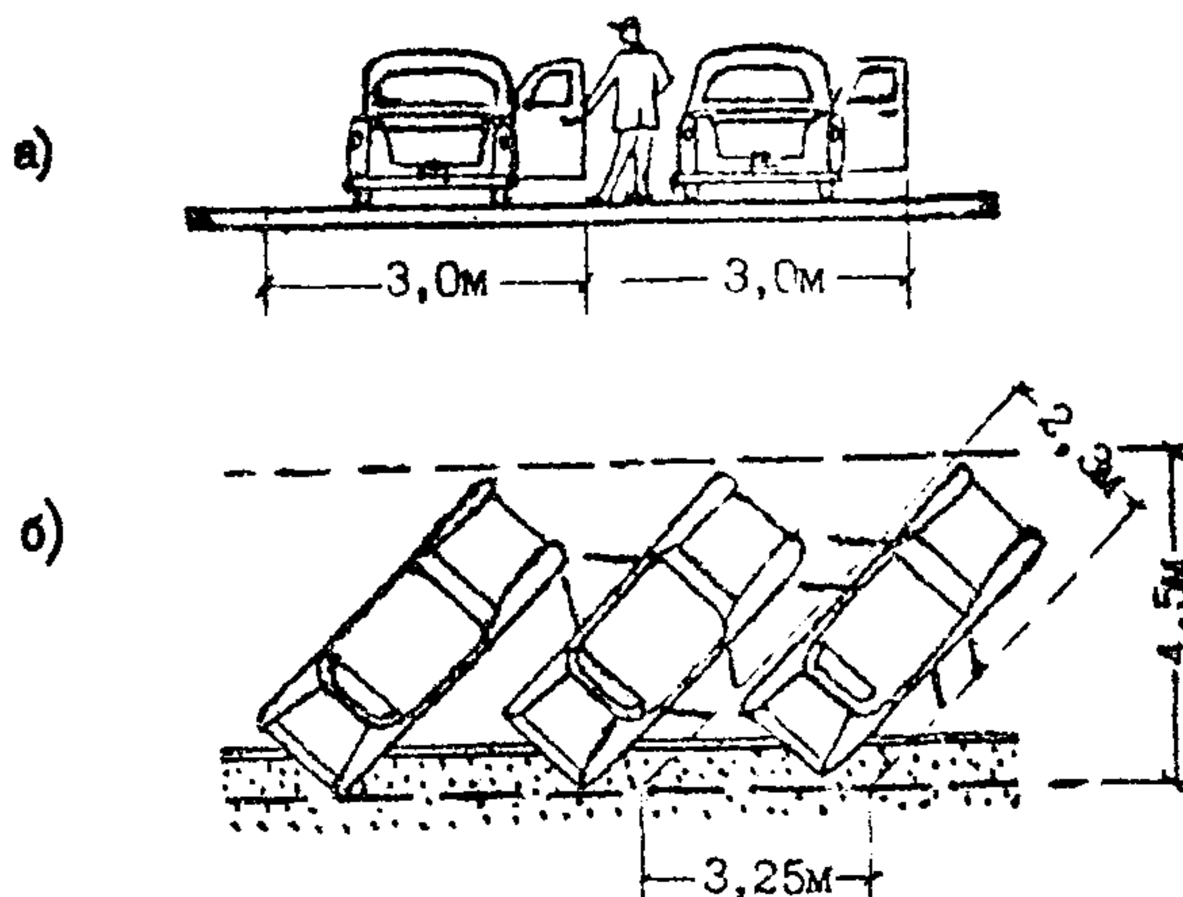
Рис. 3.20. Размеры места стоянки при косой установке автомобиля.
