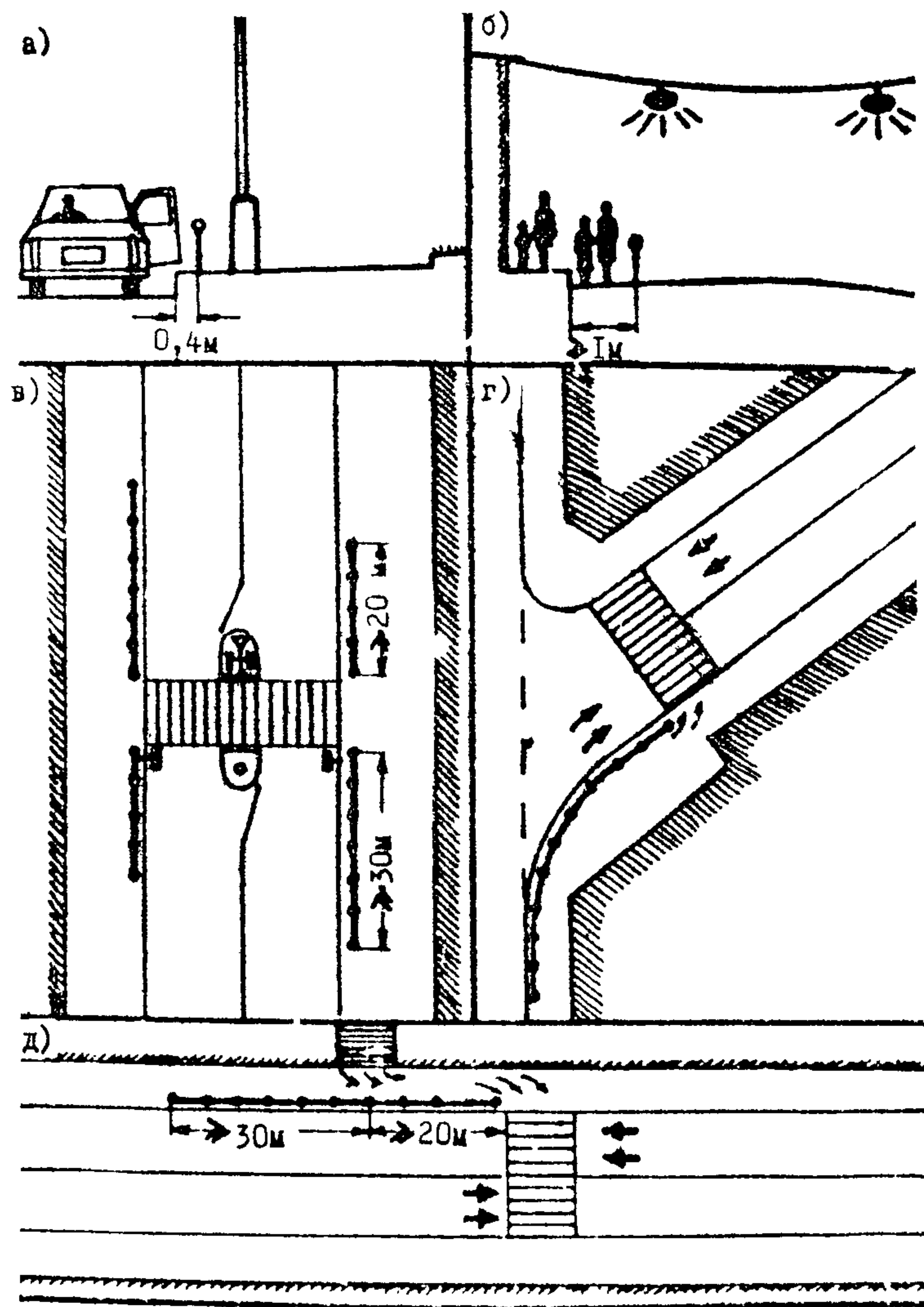
Рис. 6.4. Установка пешеходных ограждений в населённых пунктах.
