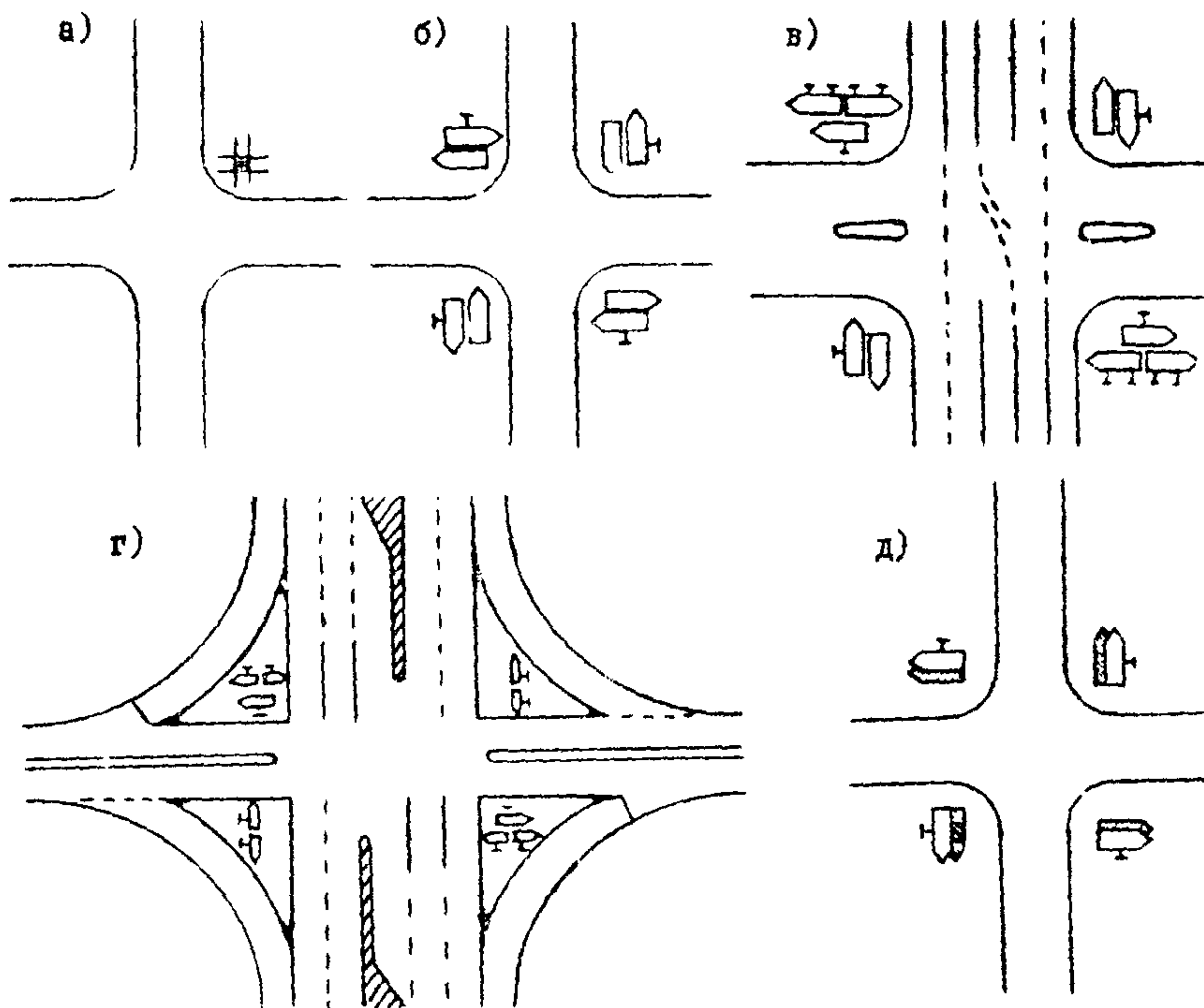
Рис. 5.15. Схемы установки знаков 4.15 "Указатель направлений" на пересечениях автомобильных дорог.
