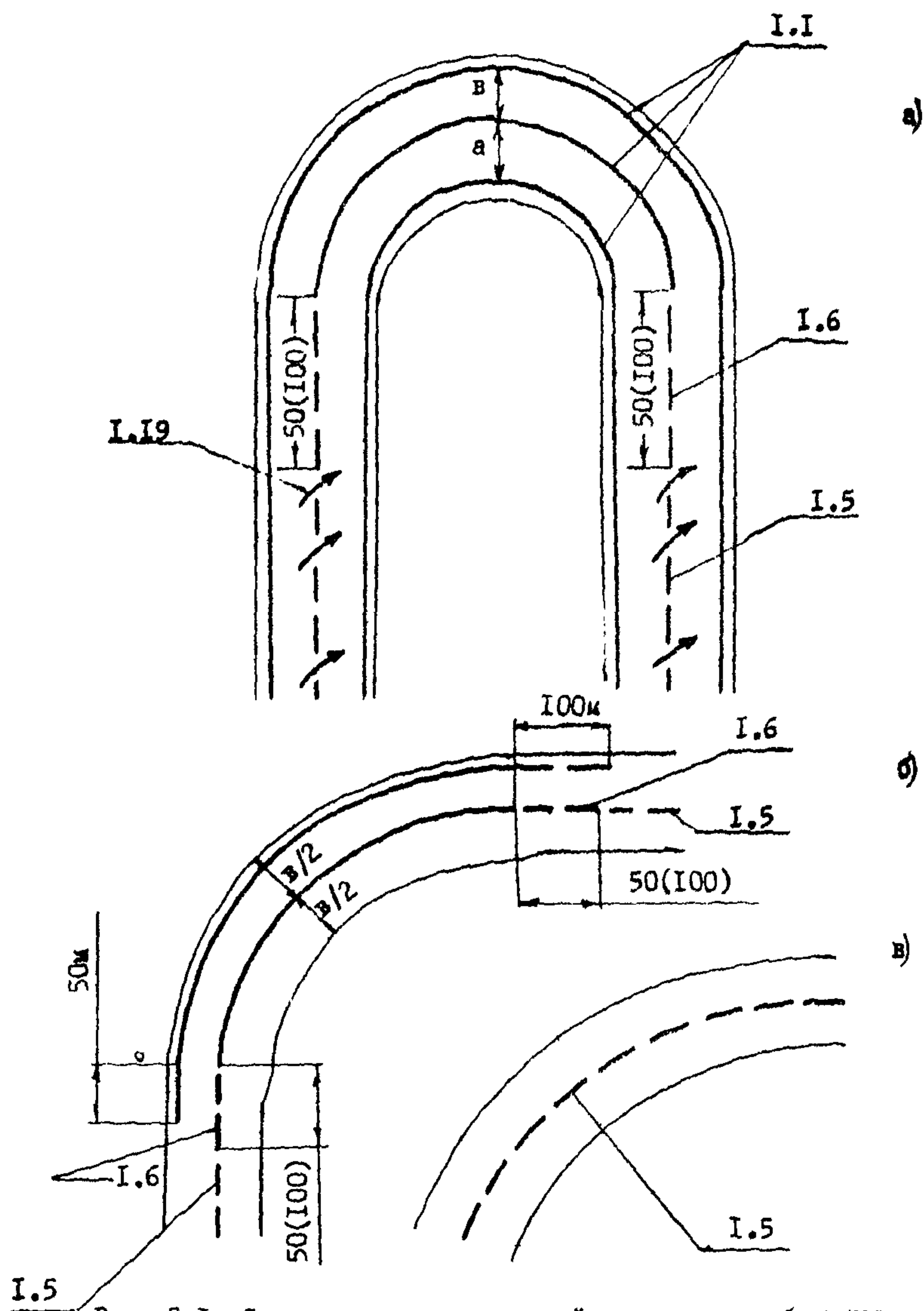
Рис. 5.1. Схемы разметки проезжей части автомобильных дорог на кривых в плане:
