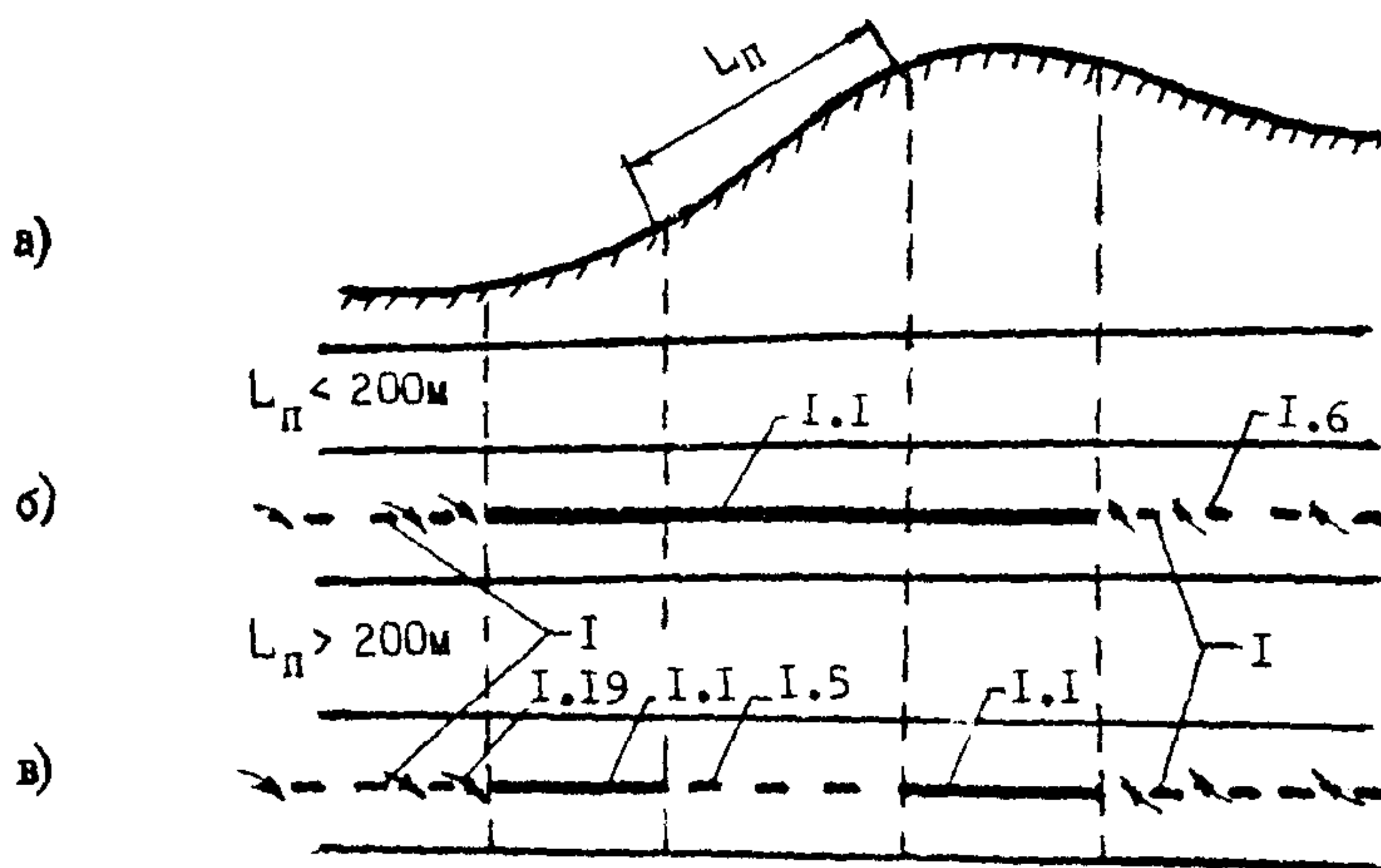
Рис. 5.4. Разметка проезжей части на подъёмах автомобильных дорог с обеспеченной видимостью при отсутствии дополнительной полосы для движения на подъём:
