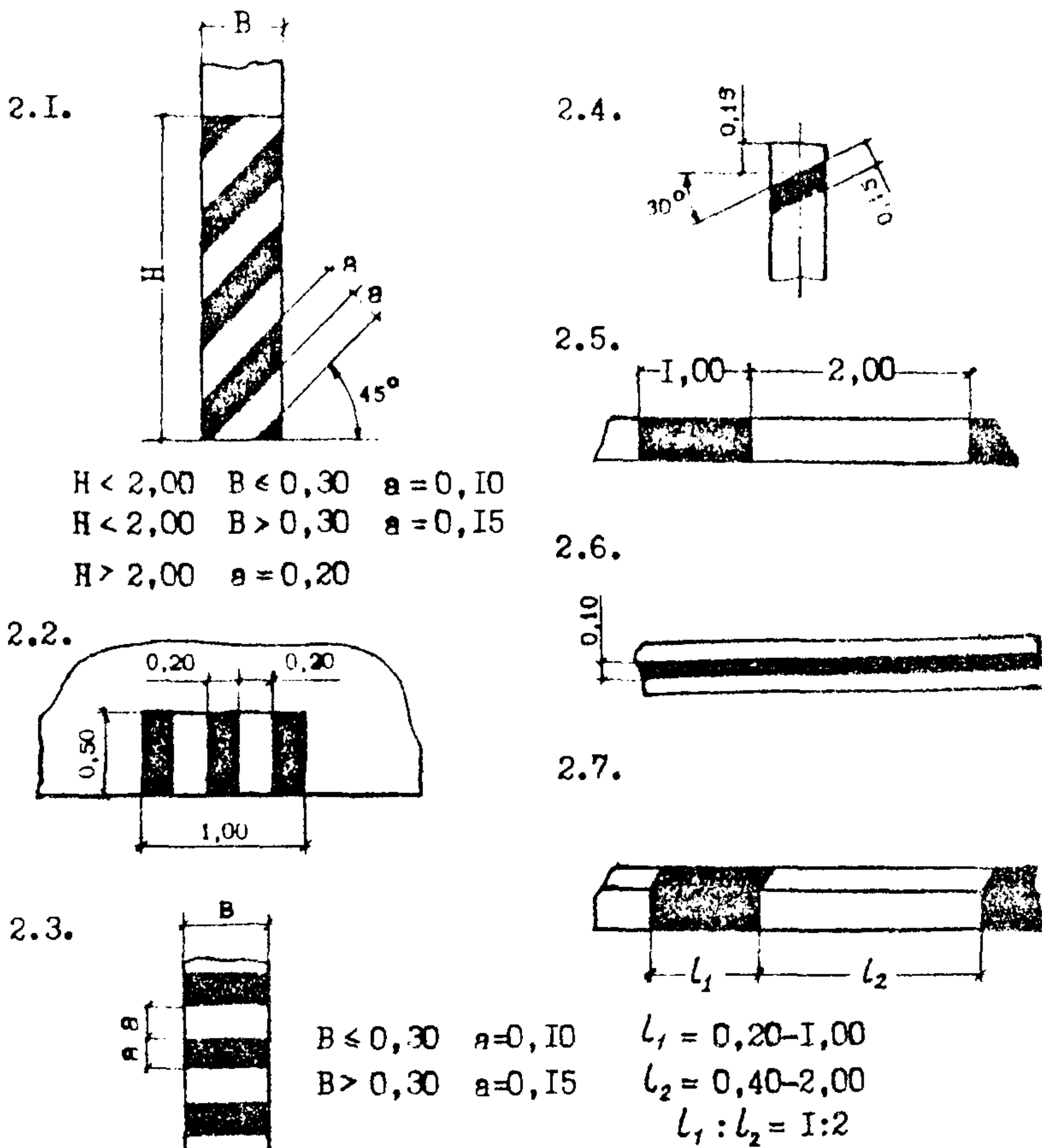
Рис. 2.3. Требования к форме и размерам (приведены в метрах) вертикальной разметки по ГОСТ 13508-74.
