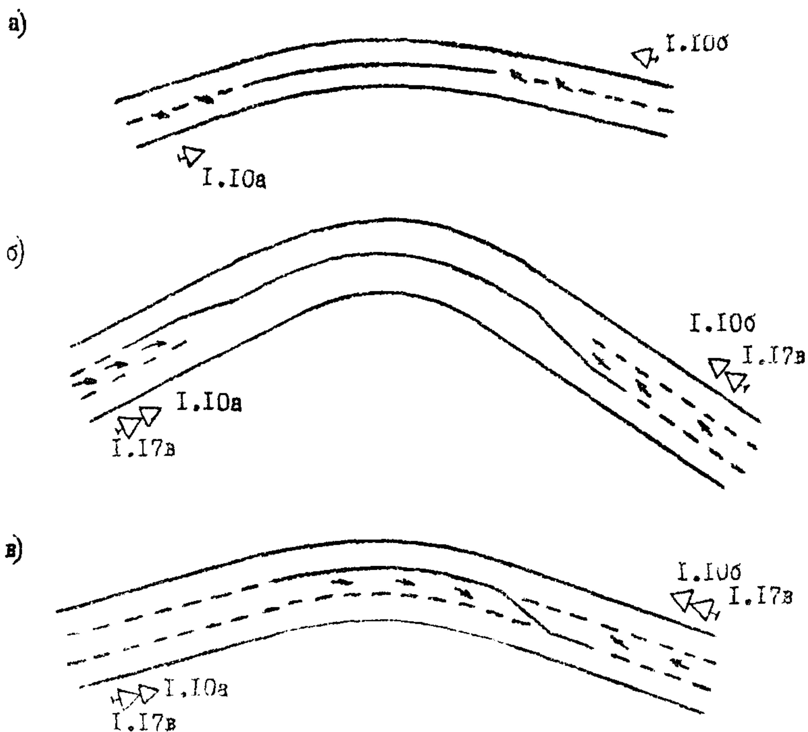
Рис. 5.3. Схема установки дорожных знаков на горизонтальных кривых автомобильных дорог:
