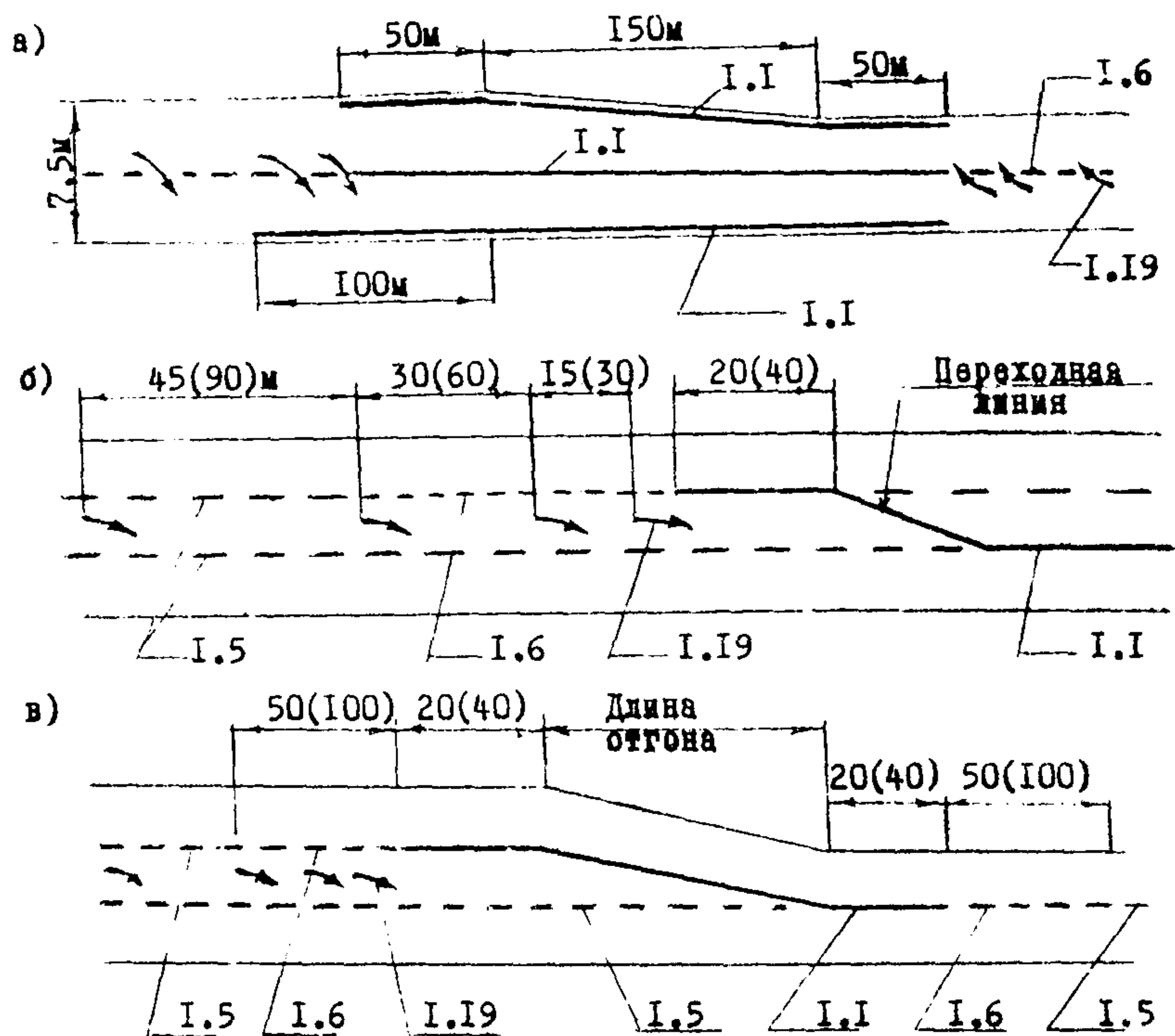
Рис. 5.19. Схемы разметки проезжей части на участках сужений:
