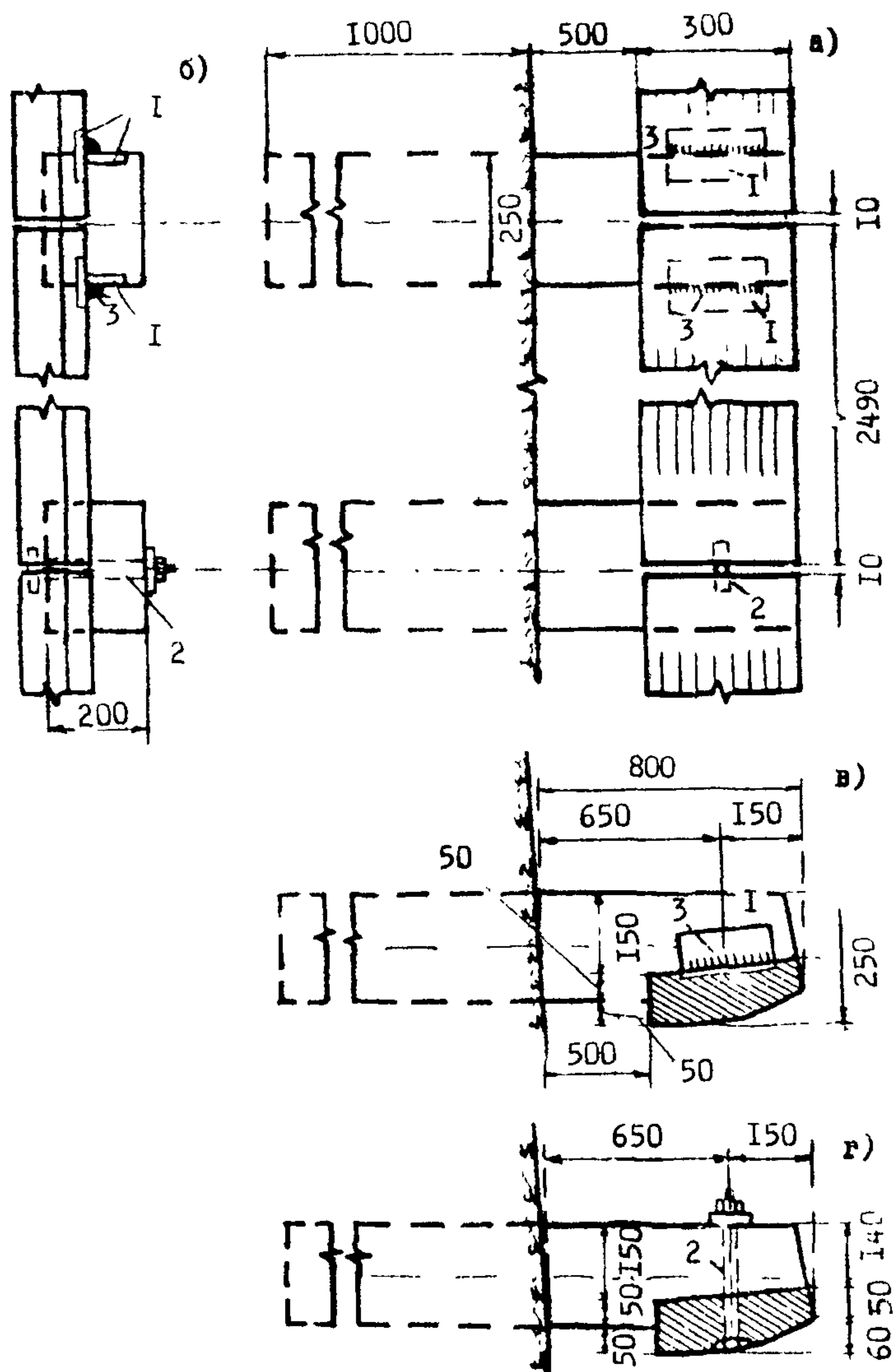
Рис. 6.2. Схема крепления и конструктивные особенности металлических ограждений: 1 - задняя пластина; 2.- болт; 3 - сварка.
