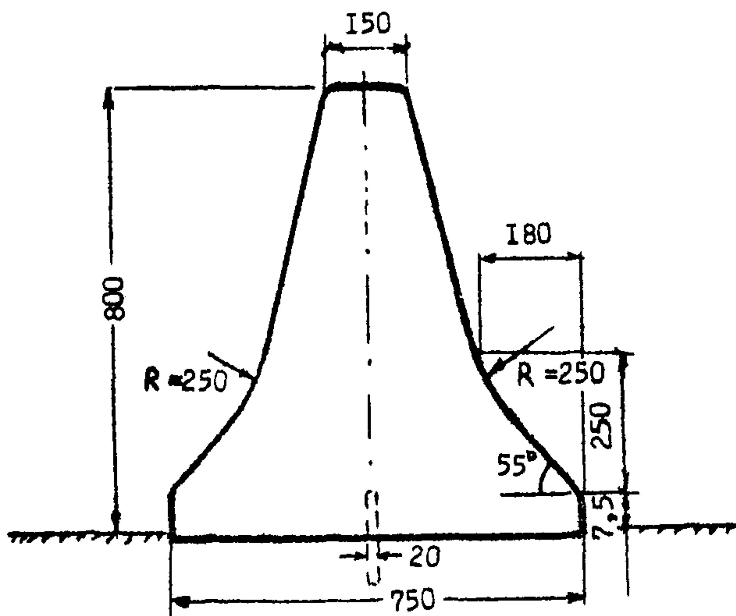
Рис. 6.6. Конструкция железобетонного ограждения парапетного типа.
