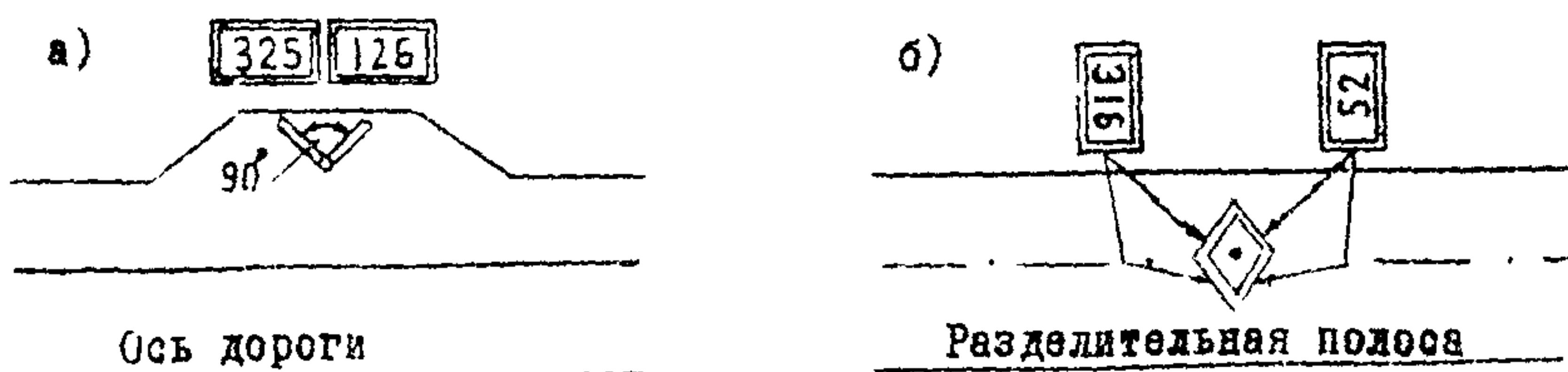
Рис. 5.16. Схемы установки километровых указателей 4.18:
