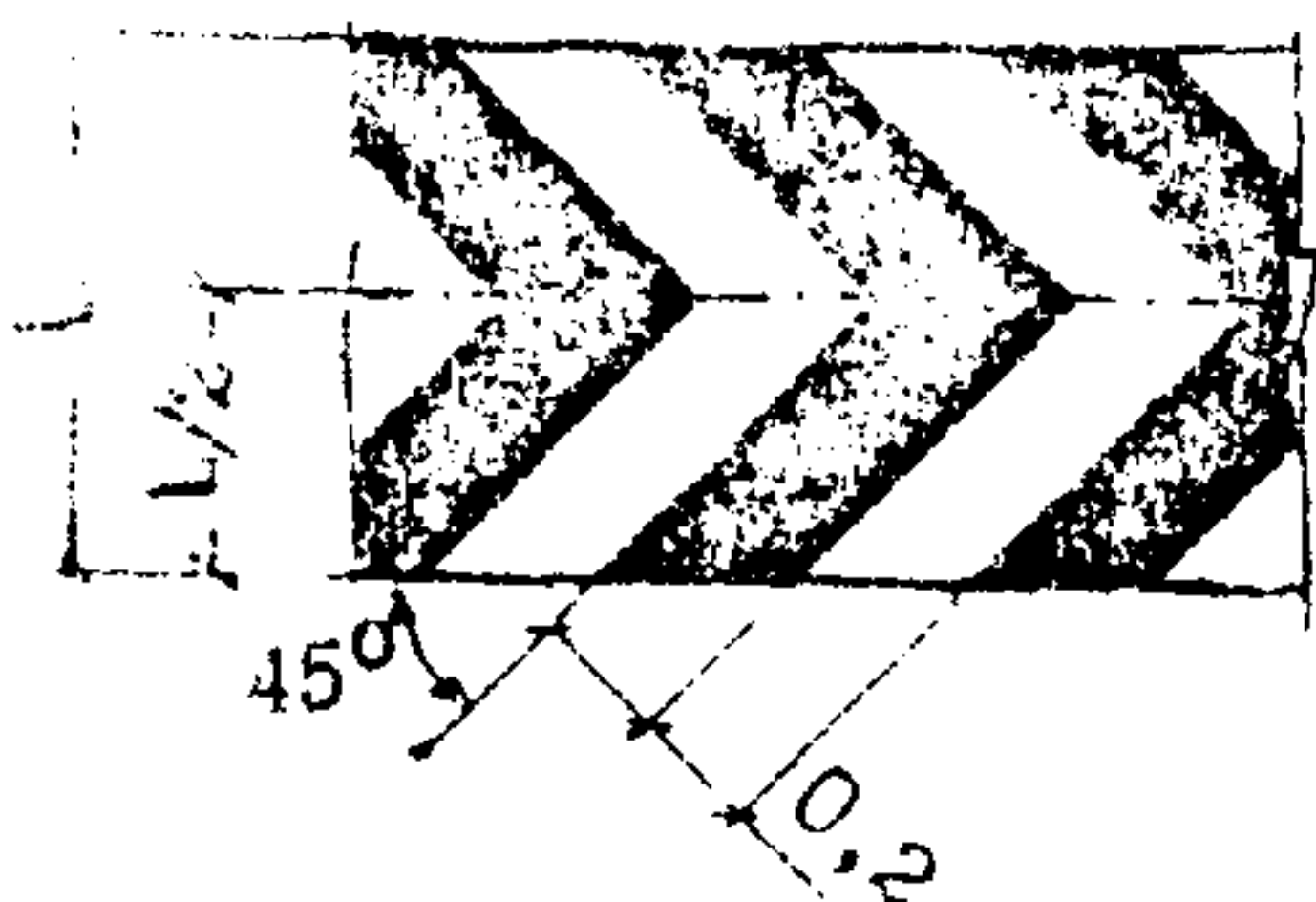
Рис. 2.7. Разметка поверхности ограждений на прямолинейных участках дорог.
