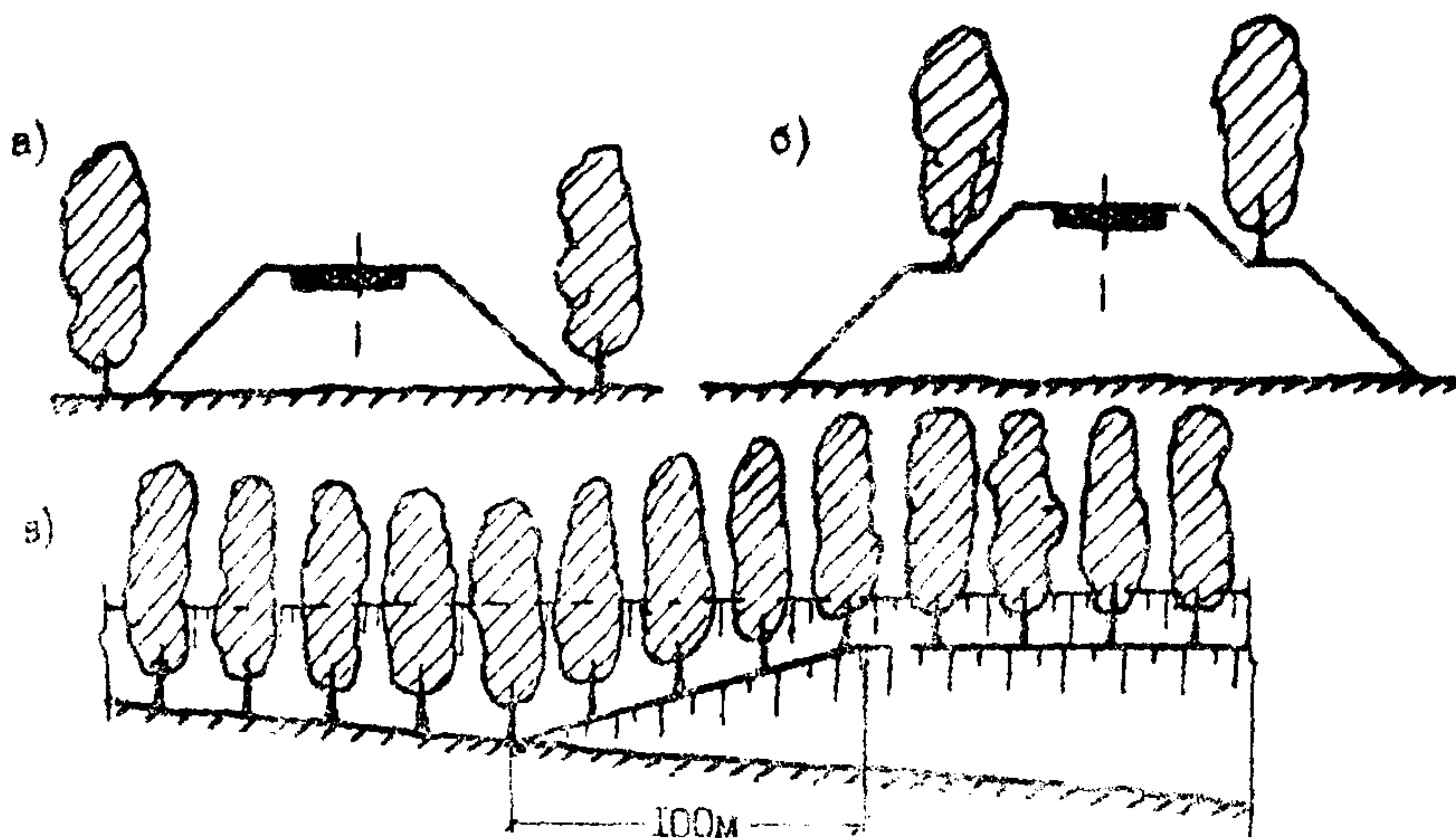
Рис. 3.8. Озеленение высоких насыпей: а - при высоте 6-8м; б - при высоте более 10м; в - устройство берма при переходе от насыпи высотой до 8м к насыпи высотой более 10м.
