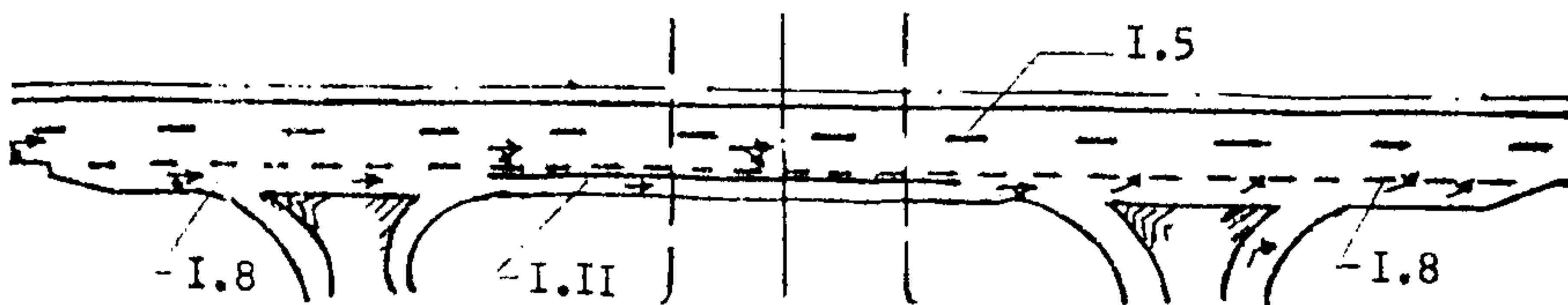
Рис. 5.9. Разметка проезжей части на участках въездов и съездов с основной дороги на пересечениях в разных уровнях.
