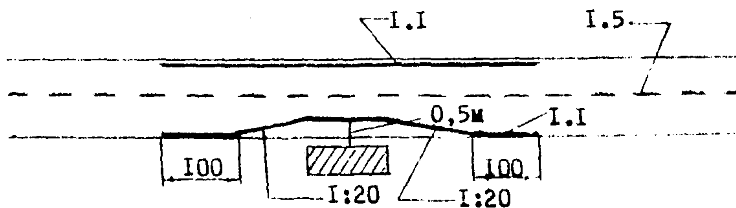
Рис. 5.20. Разметка проезжей части на участке с близко расположенным обрывом и препятствием.
