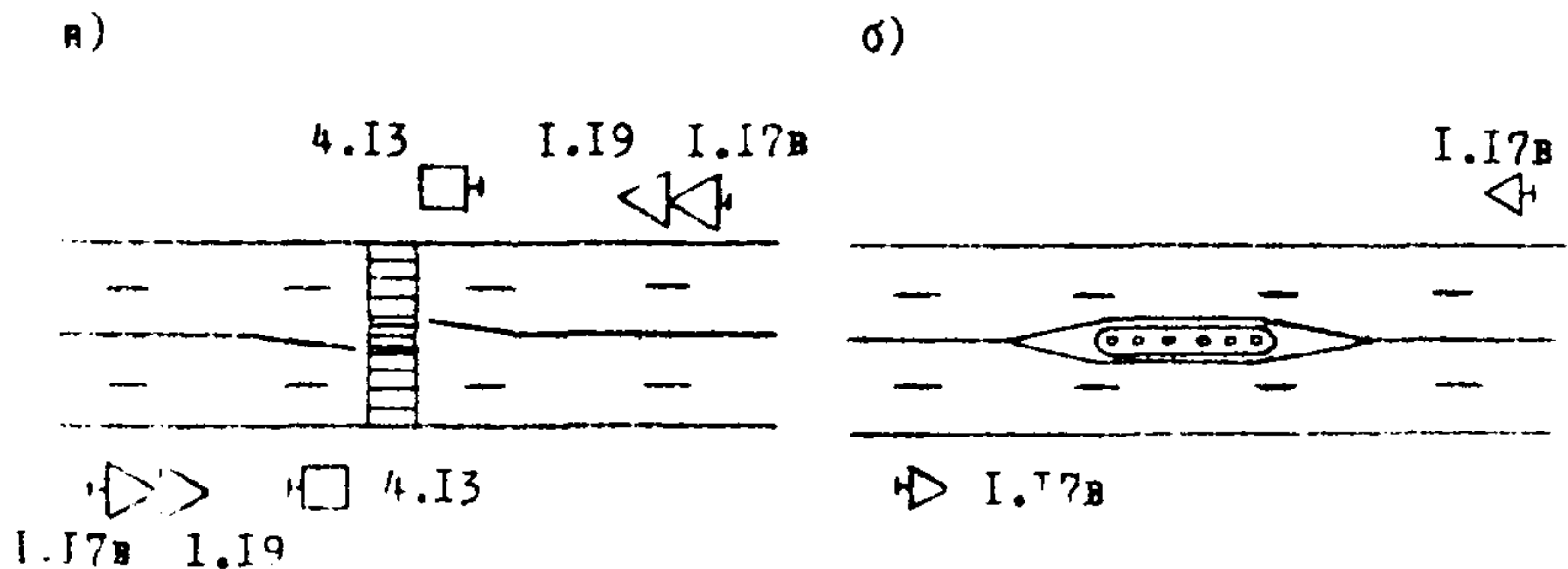
Рис. 5.21. Схемы расстановки дорожных знаков на участках сужений.
