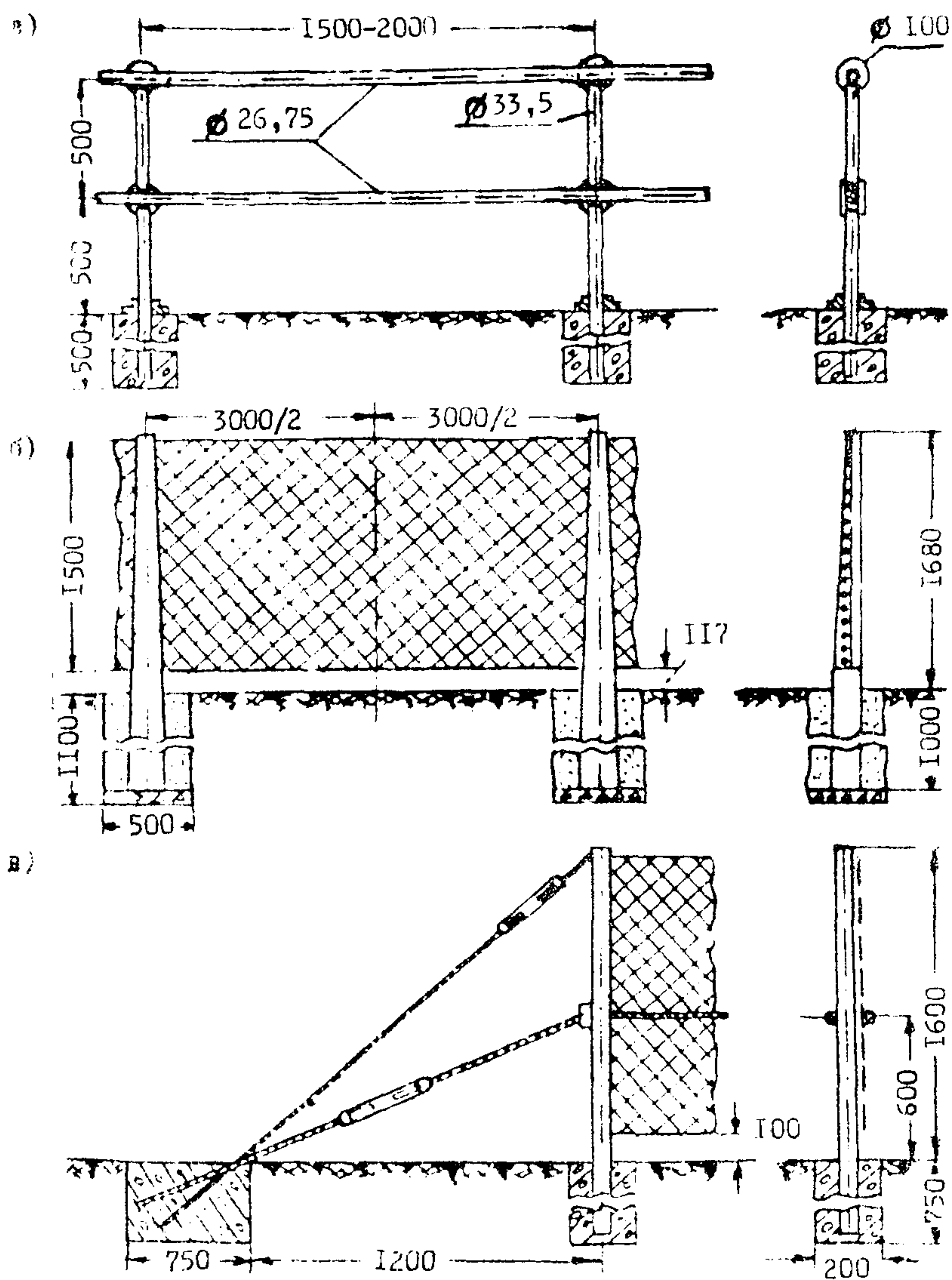
Рис. 6.3. Конструктивные особенности пешеходных ограждений на автомобильных дорогах.
