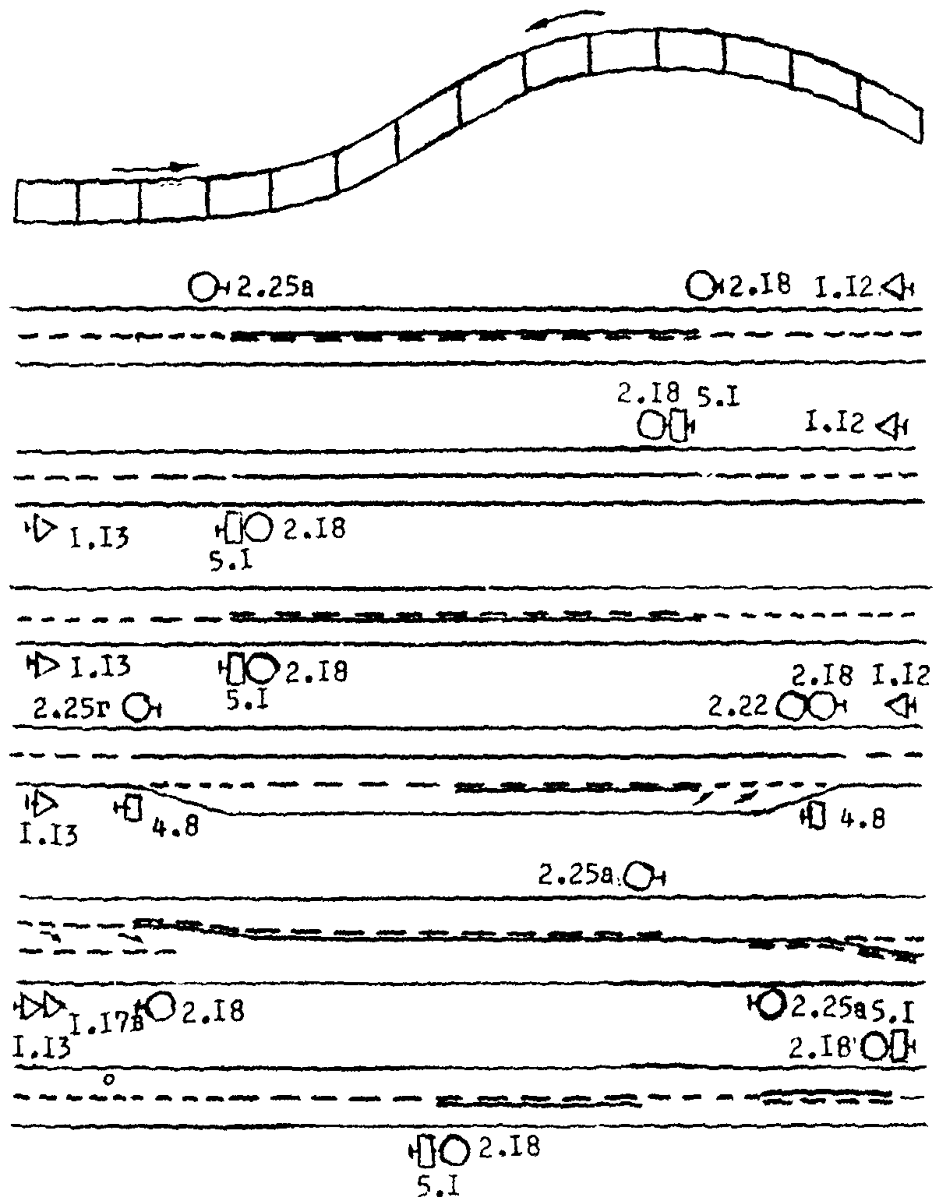
Рис. 5.7. Схемы установки знаков на подъёмах и опусках.
