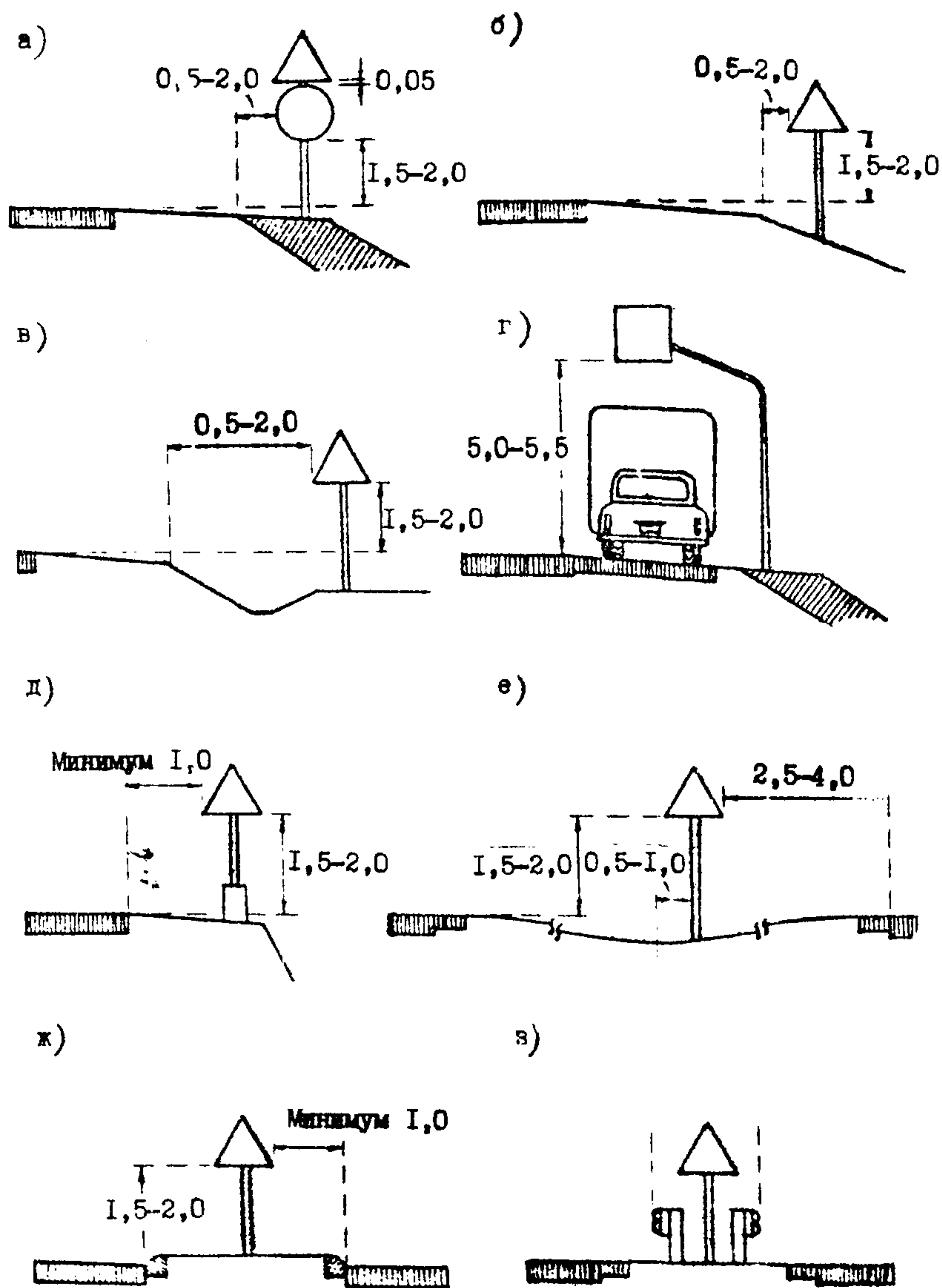
Рис. 4.2. Способы установки знаков на автомобильных дорогах.
