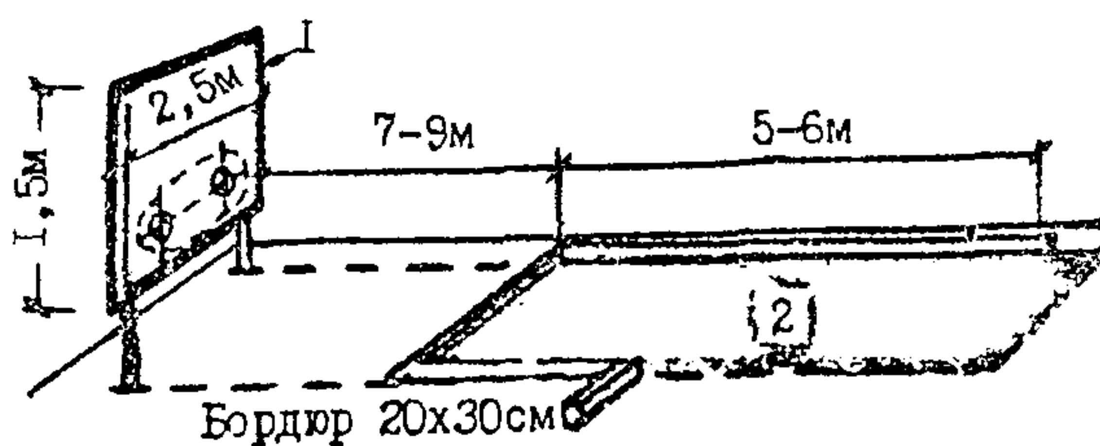
Рис. 3.22. Площадка для регулирования фар автомобилей определённых типов:
