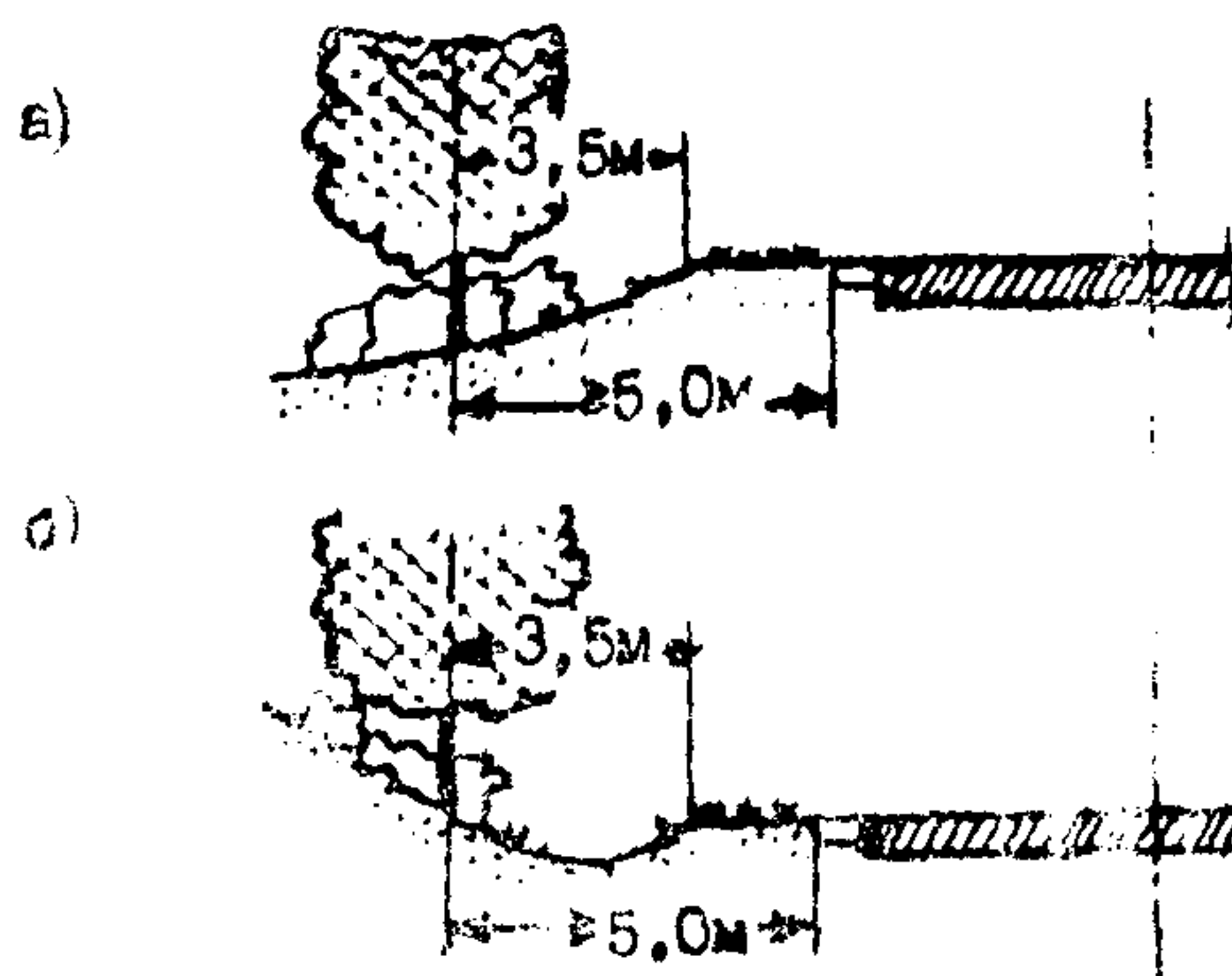
Рис. 3.2. Размещение придорожных насаждений по отношению к кромке проезжей части и бровке земляного полотна:
