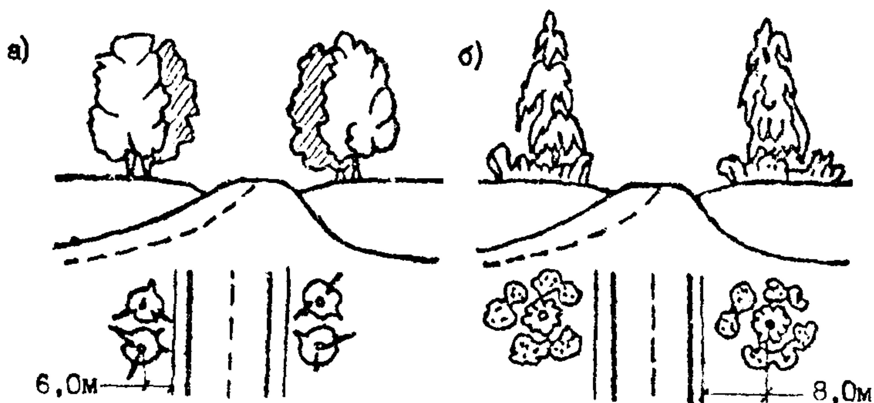
Рис. 3.14. Приёмы озеленения выпуклых переломов продольного профиля групповыми парными посадками /"ворота"/: а - в закрытой местности; б - в открытой местности.
