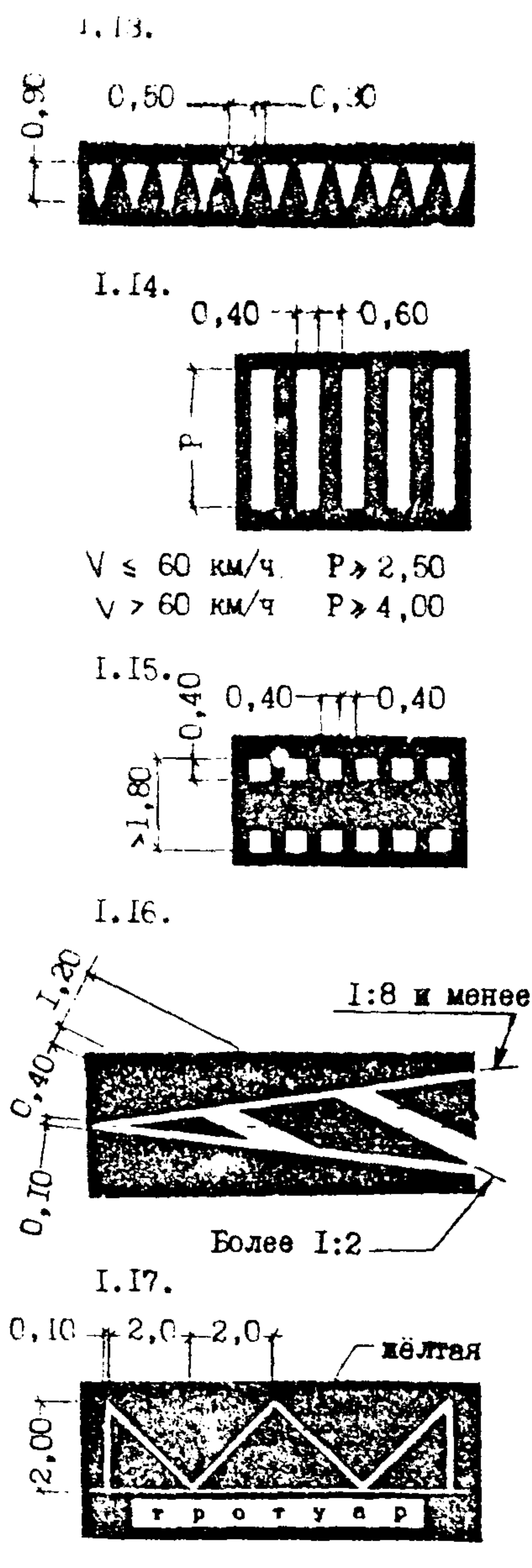
Рис. 2.1-б. Требования к цвету, форме и размерам /в метрах/ горизонтальной разметки по ГОСТ 13508-74.
