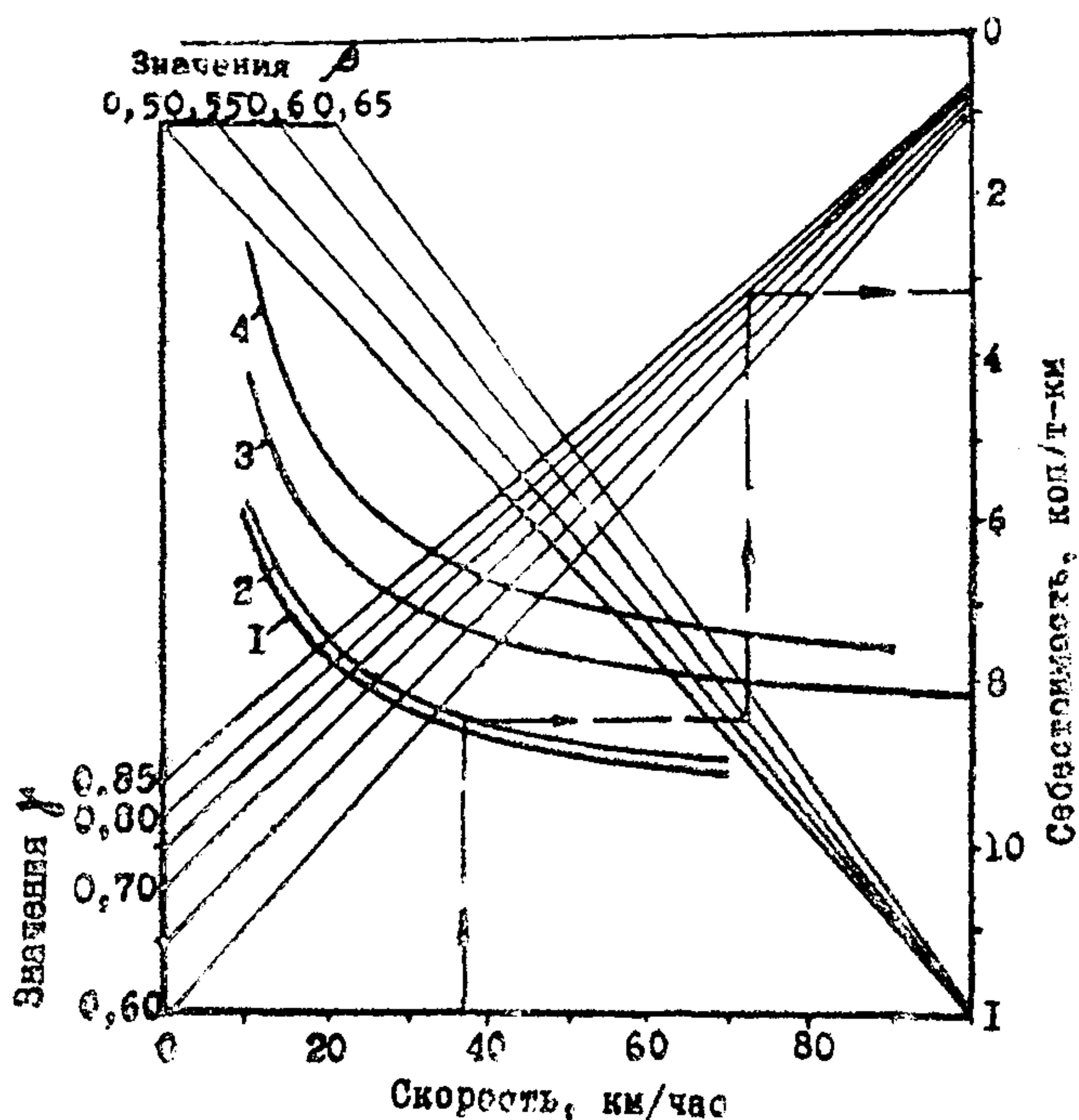
Рис. 8.3. Помогательная диаграмма для определения себестоимости 1 т-км грузовой работы. Автомобили
