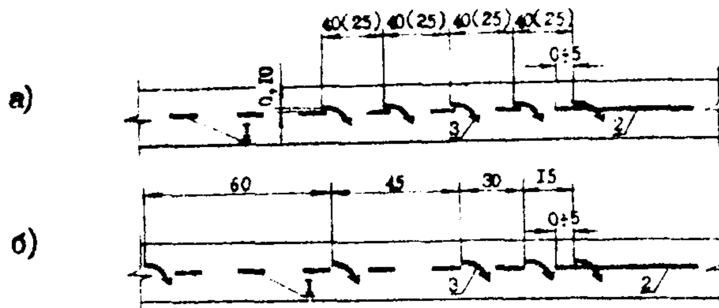
Рис. 2.2. Экспериментальная разметка с применением направляющих стрел: а, б – варианты расположения стрел на проезжей части при постоянном и убывающем расстоянии между ними; 1 – осевая прерывистая линия; 2 – разделительная сплошная линия; 3 – направляющие стрелы.
