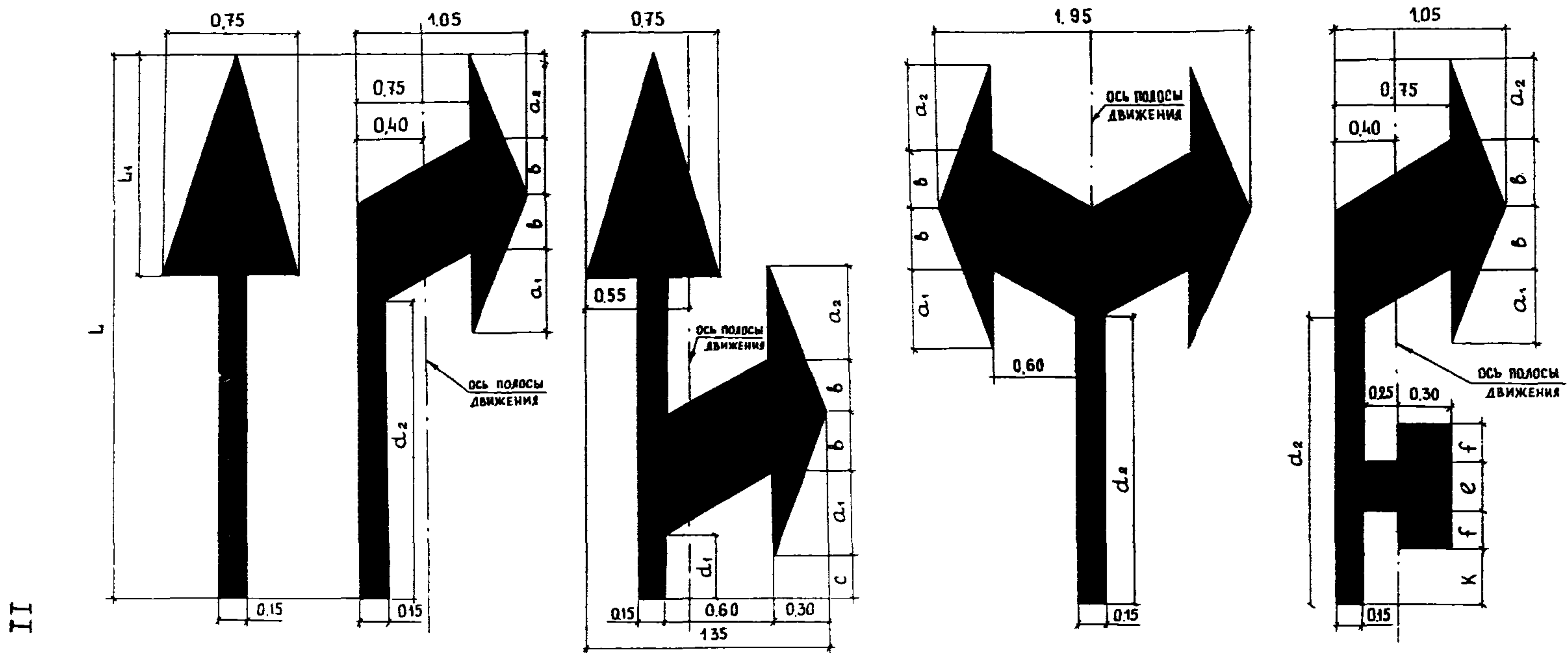
Рис.2. Стрелы для обозначения направлений движения по полосам
