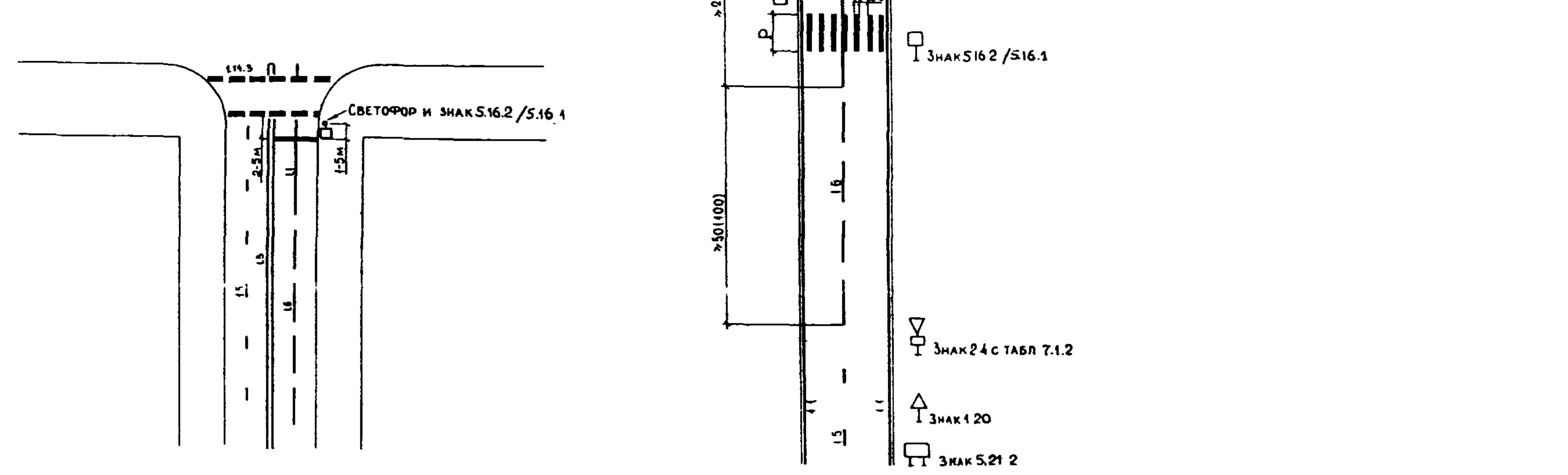
ВАРИАНТ РАЗМЕТКИ ПЕШЕХОДНОГО ПЕРЕХОДА В НАСЕЛЕННОМ ПУНКТЕ
