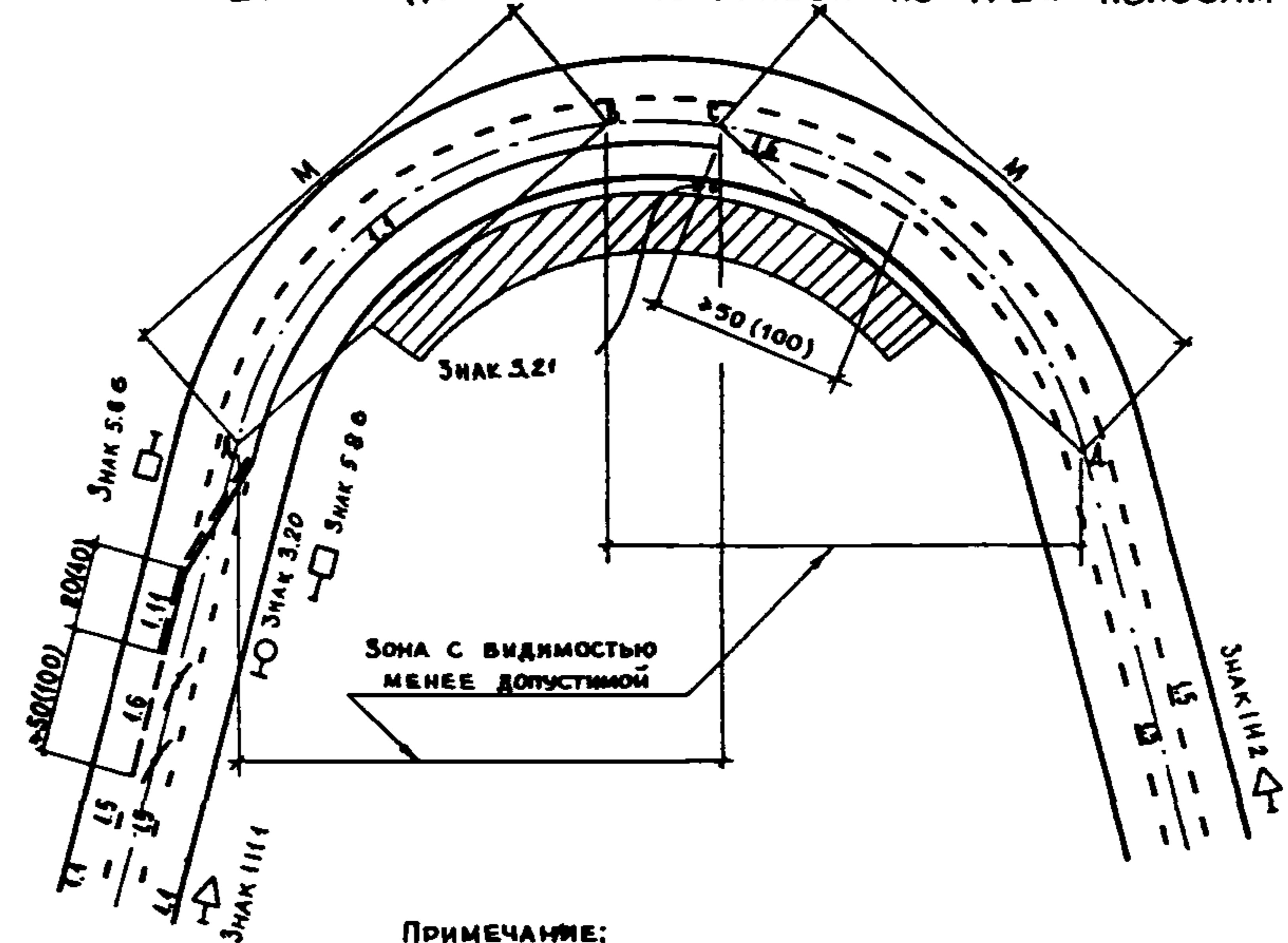
Б. При движении по кривой по трем полосам
