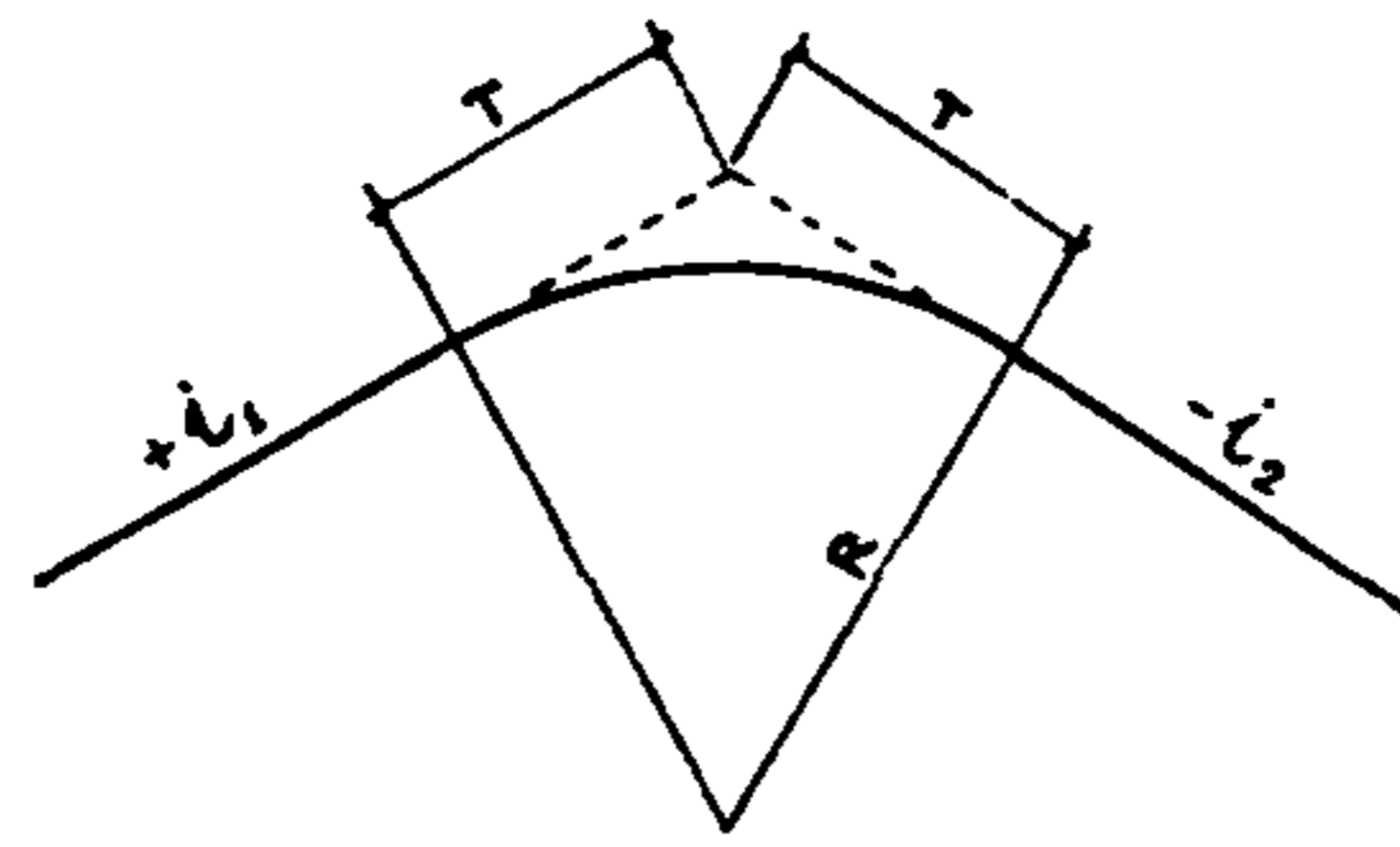
Рис. 10. Элементы вертикальной выпуклой кривой
