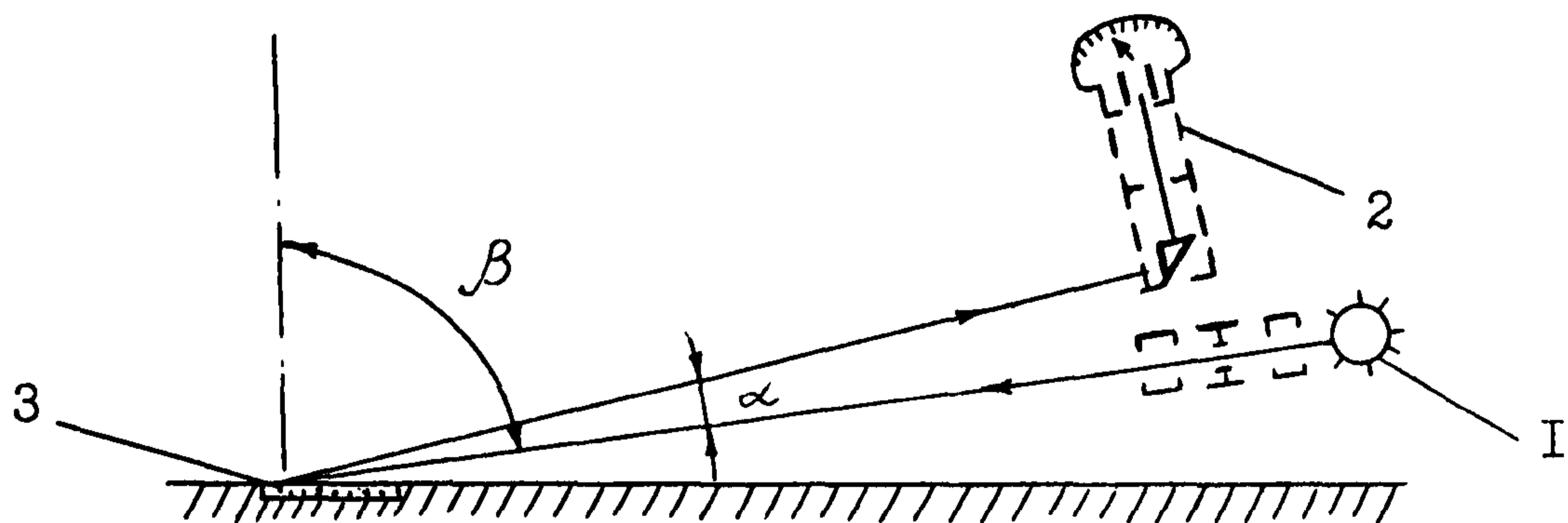
Схема измерения удельного коэффициента силы света
