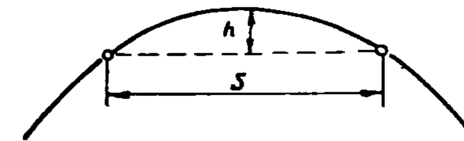
Рис. 13. Схема к определению радиуса закругления
