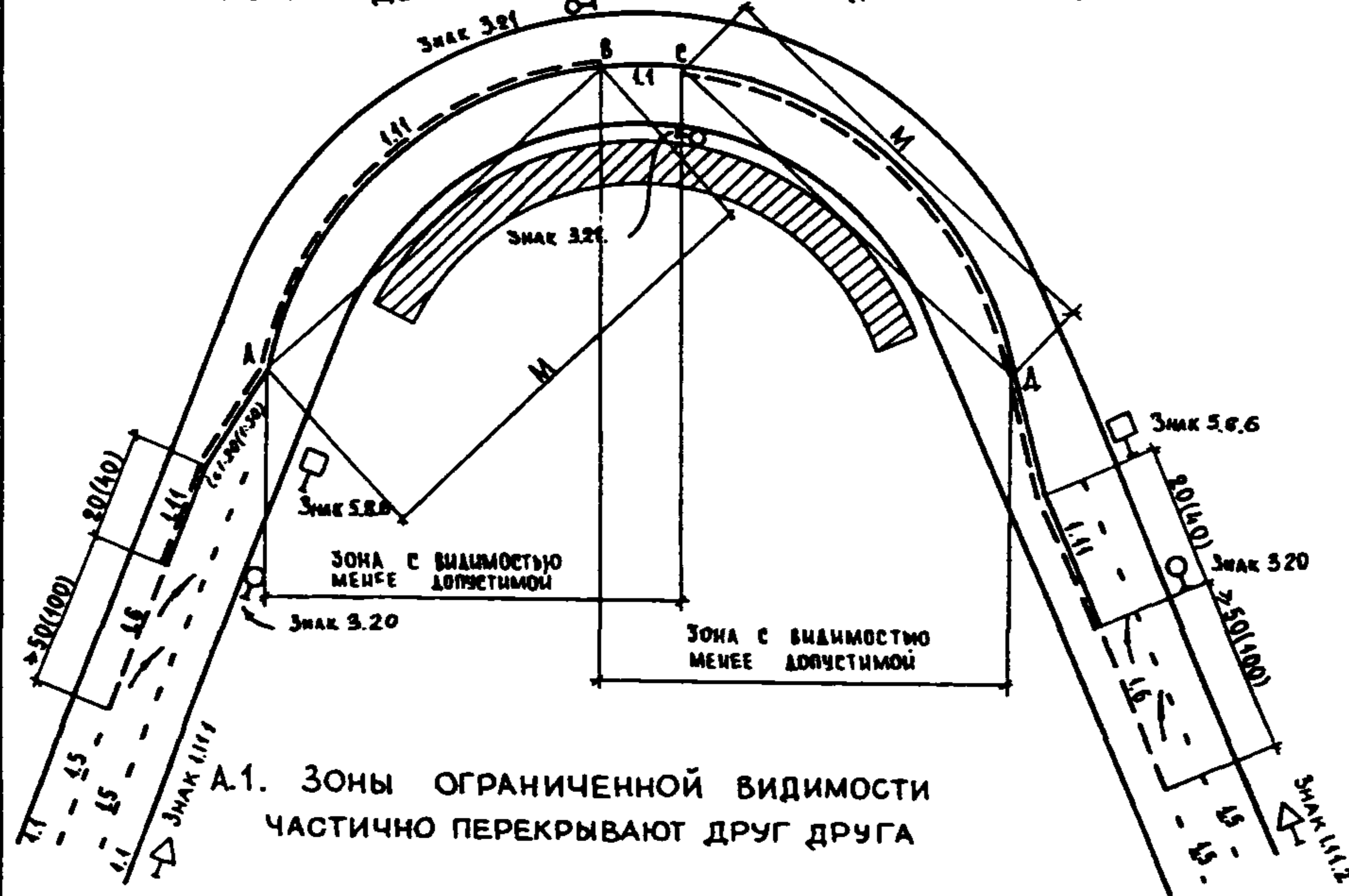
А. При движении по кривой по двум полосам
