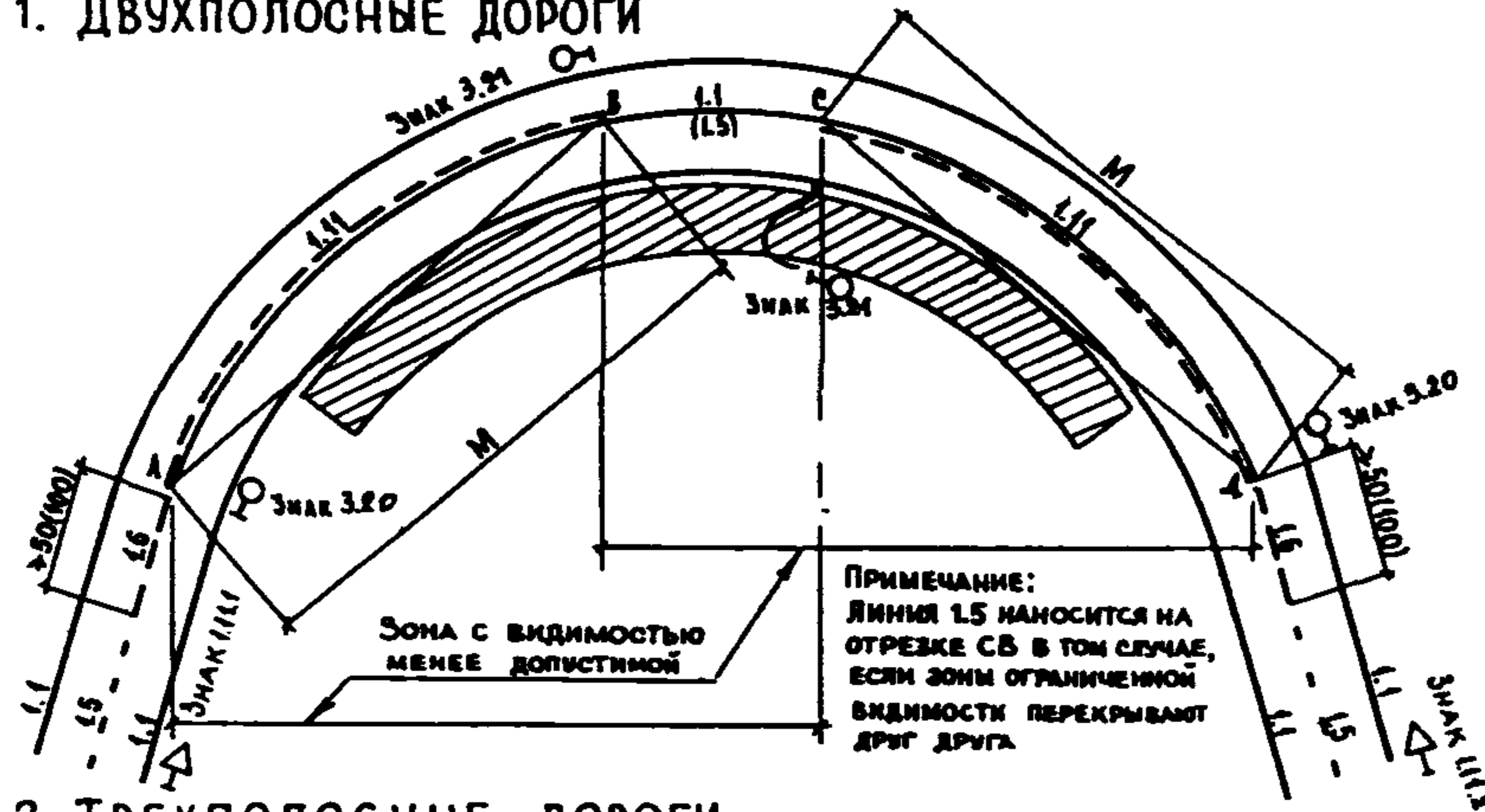
А. При движении по кривой по двум полосам
