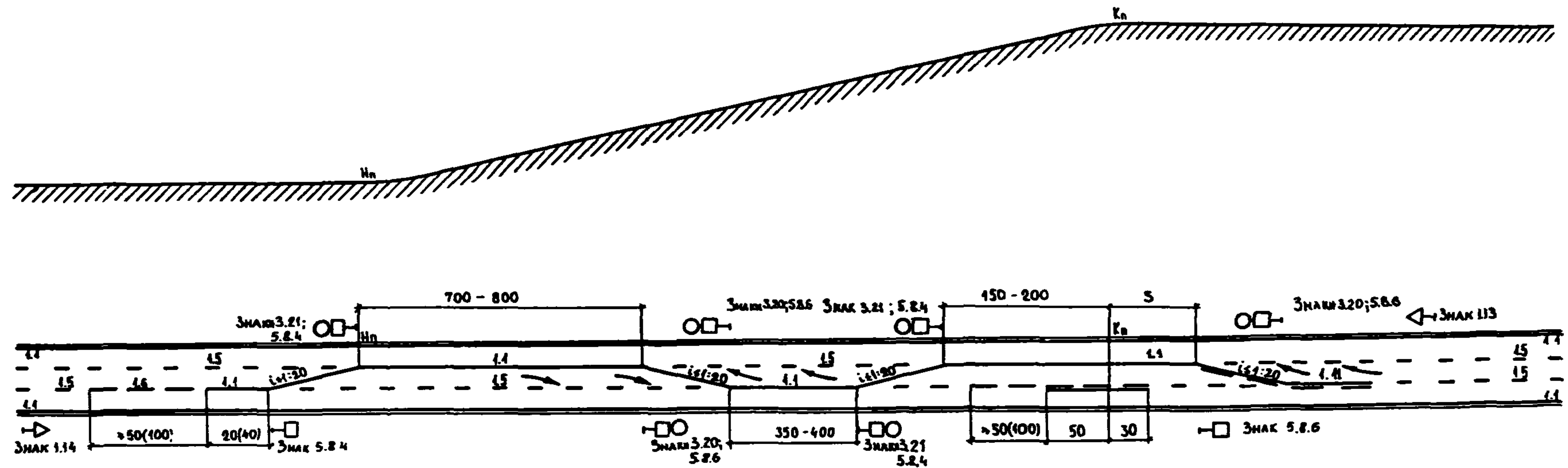
Б. НА ЗАТЯЖНЫХ ПОДЪЕМАХ ДЛИНОЙ БОЛЕЕ 1200 М
