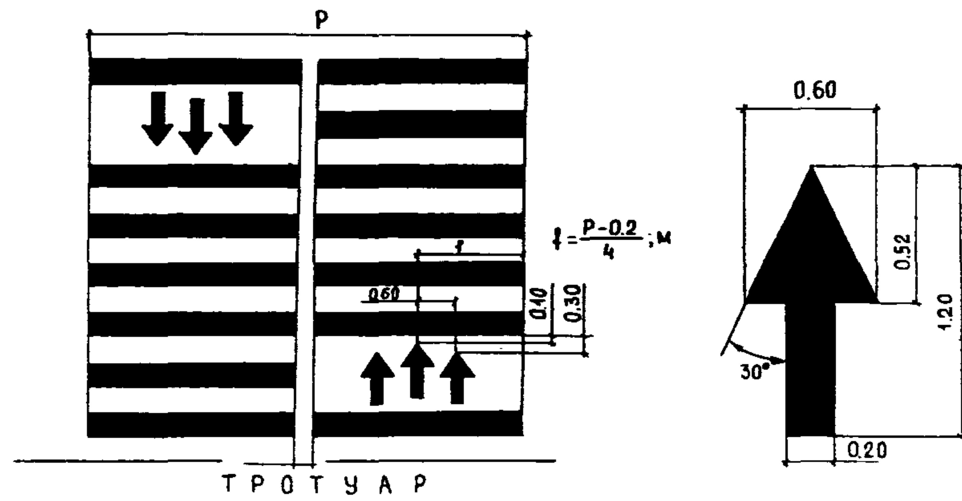
Рис.1. Разметка пешеходного перехода шириной 6,0 м и более
