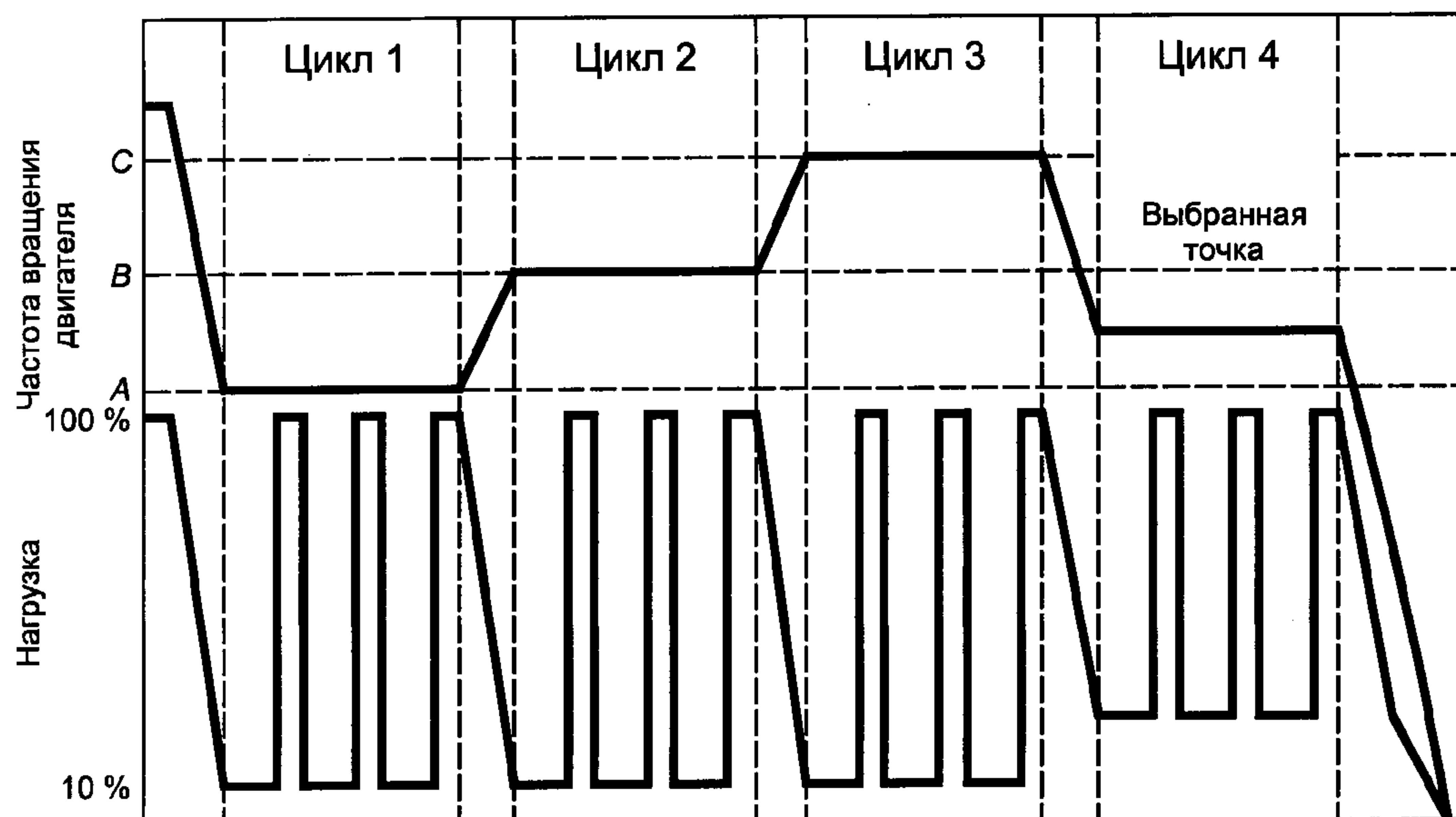
Рисунок Д.1 — Последовательность режимов в испытании ELR
