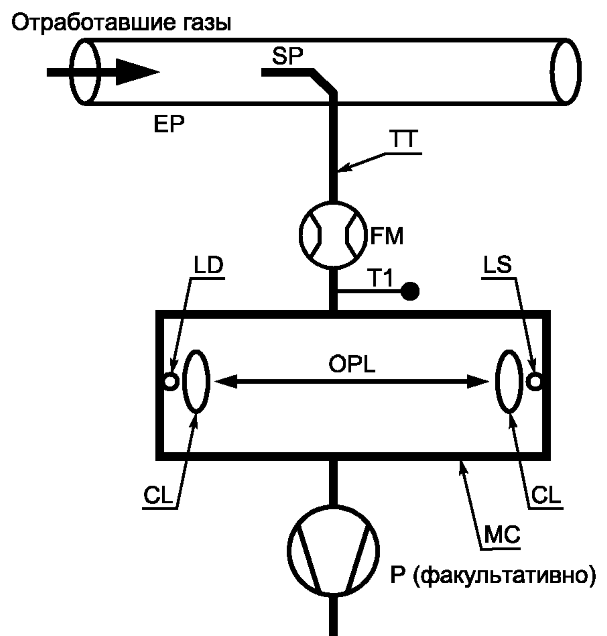
Рисунок Д.22 — Дымомер на частичном потоке
