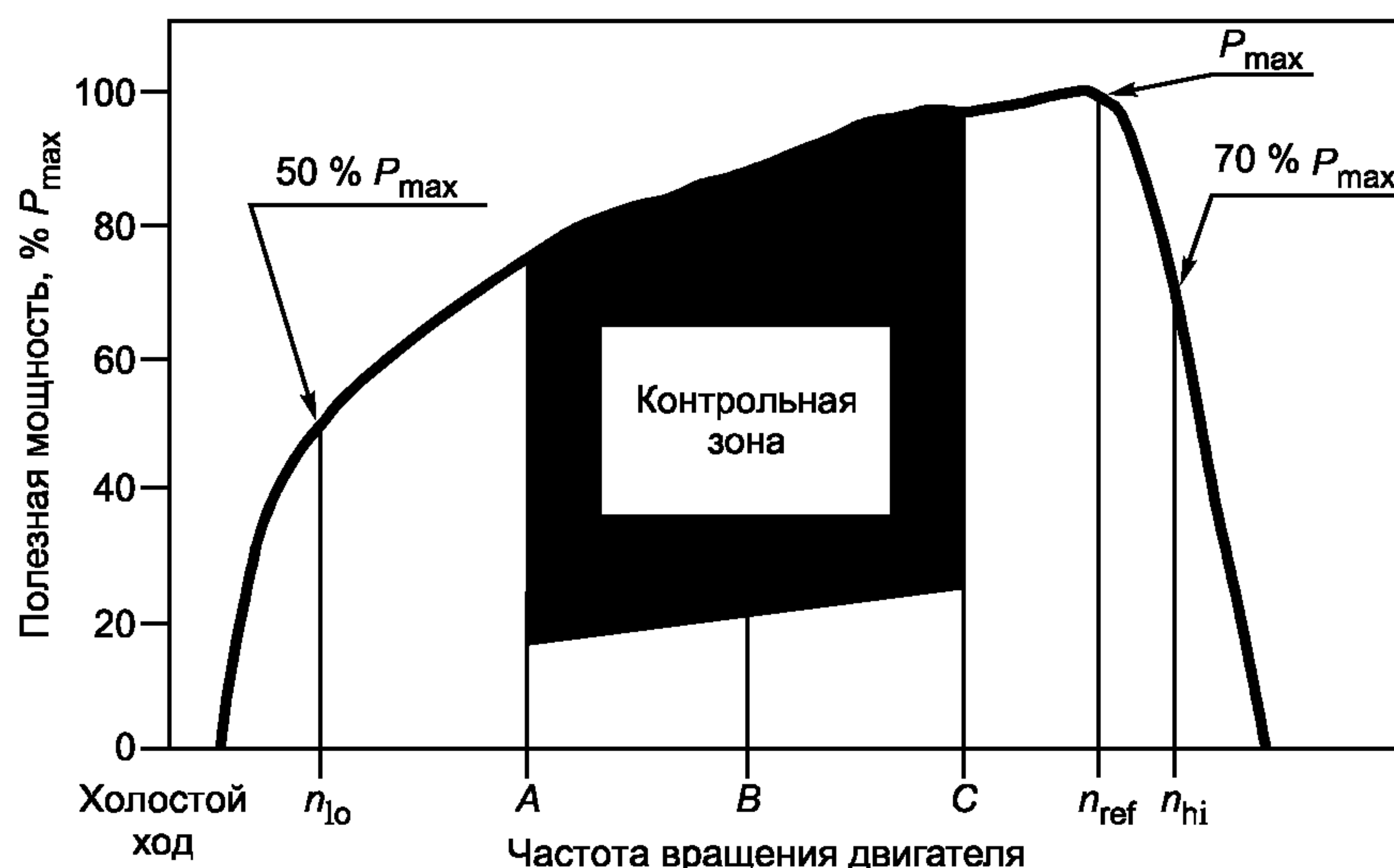
Рисунок 1 — Характерные элементы испытательного цикла
