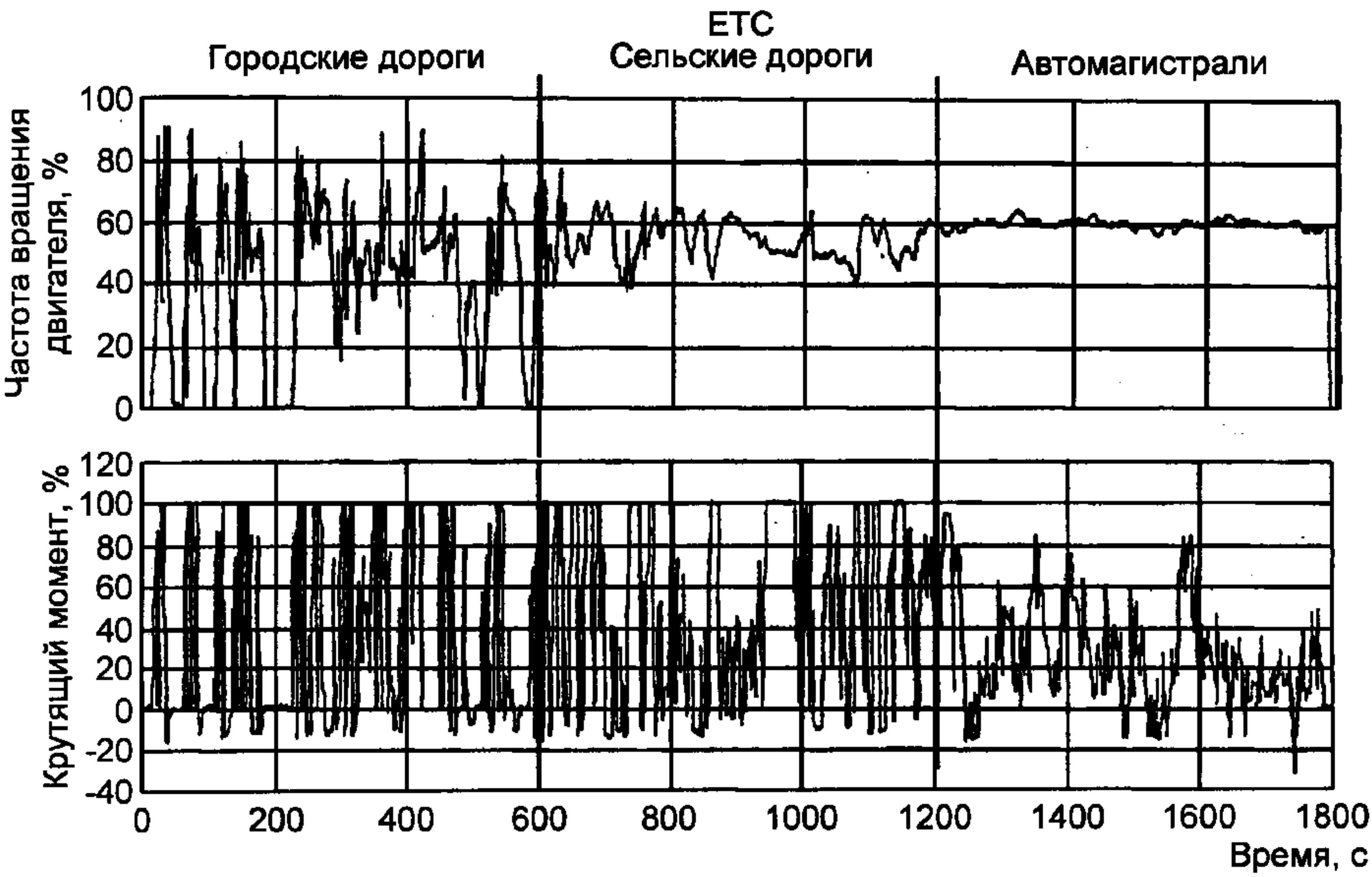
Рисунок Д.3 — Динамометрический график испытания ETC
