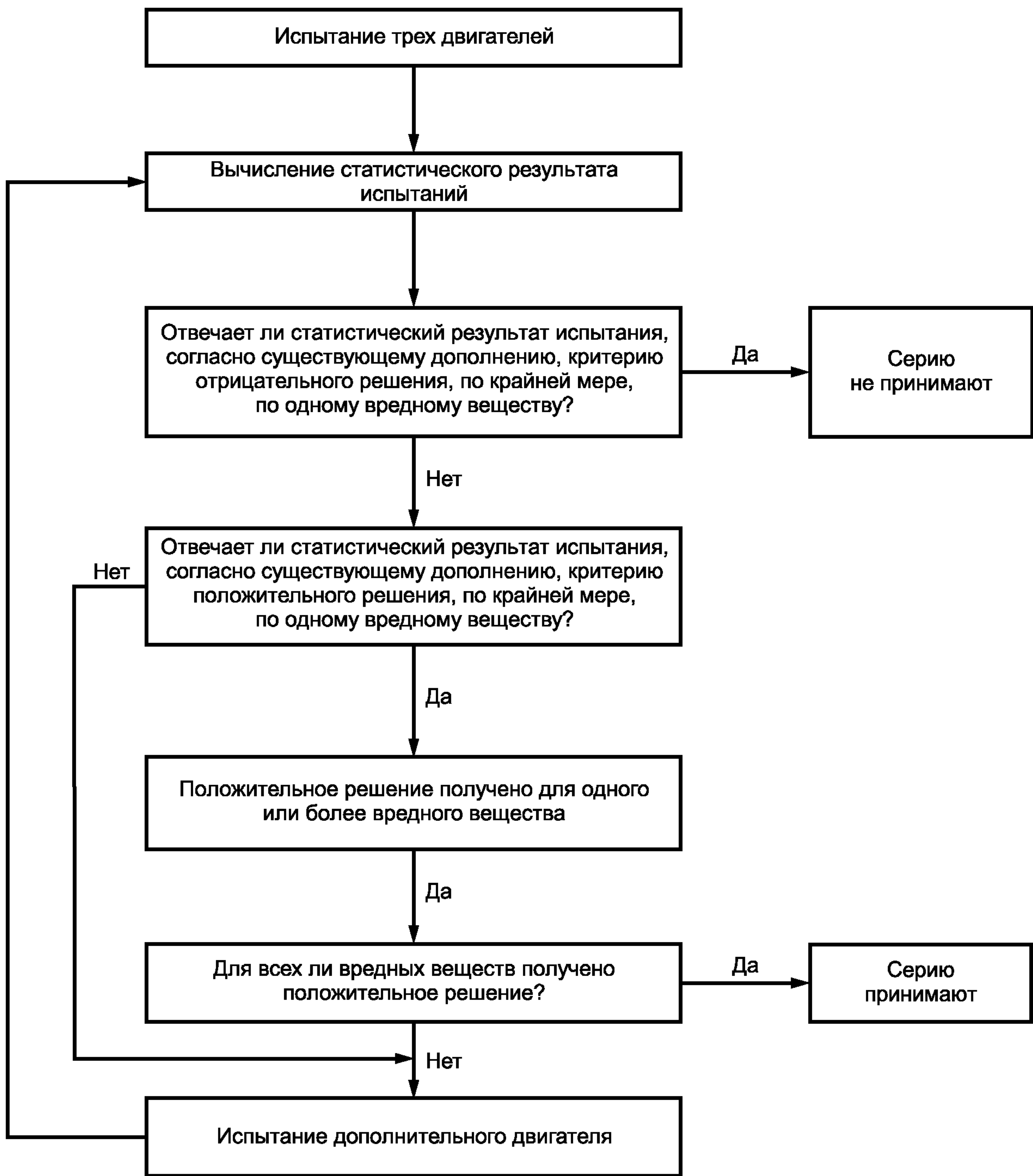
Рисунок 2 — Схема испытания на соответствие производства
