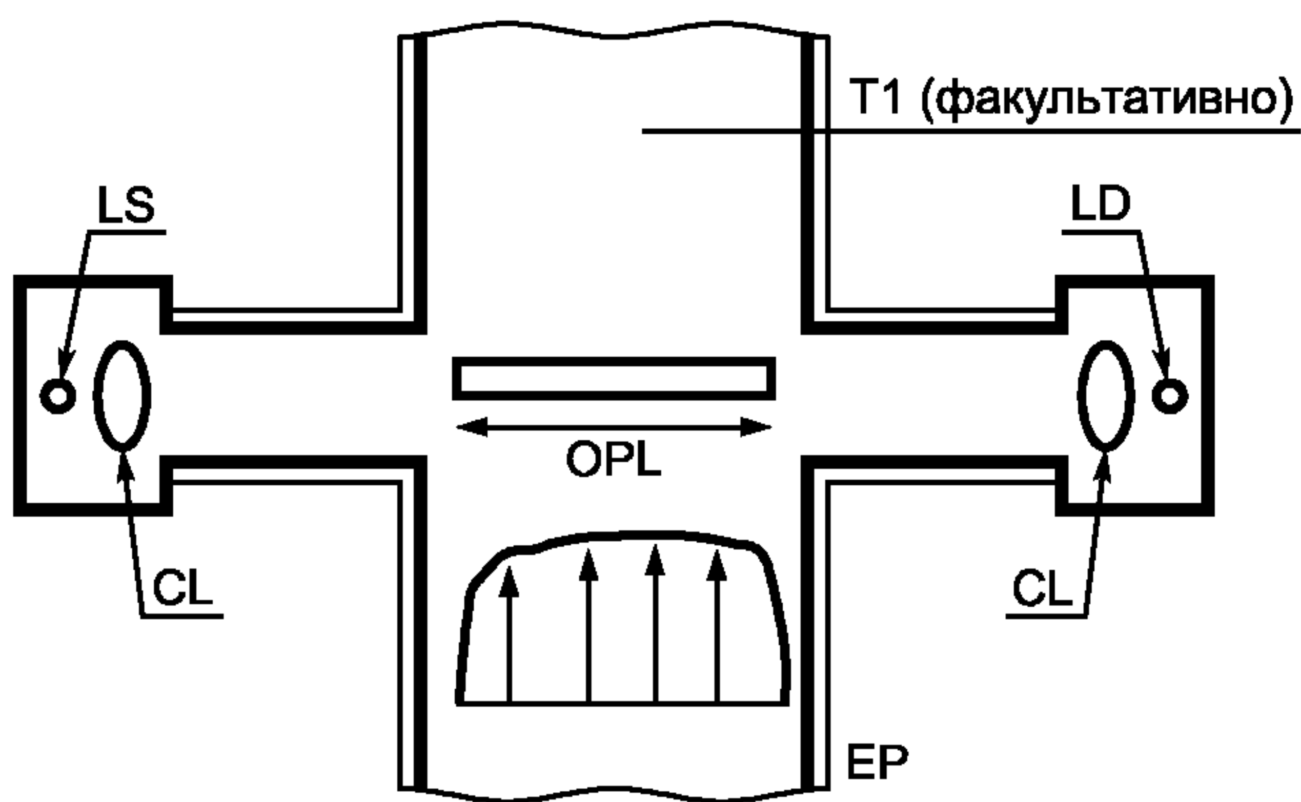
Рисунок Д.21 — Полнопоточный дымомер
