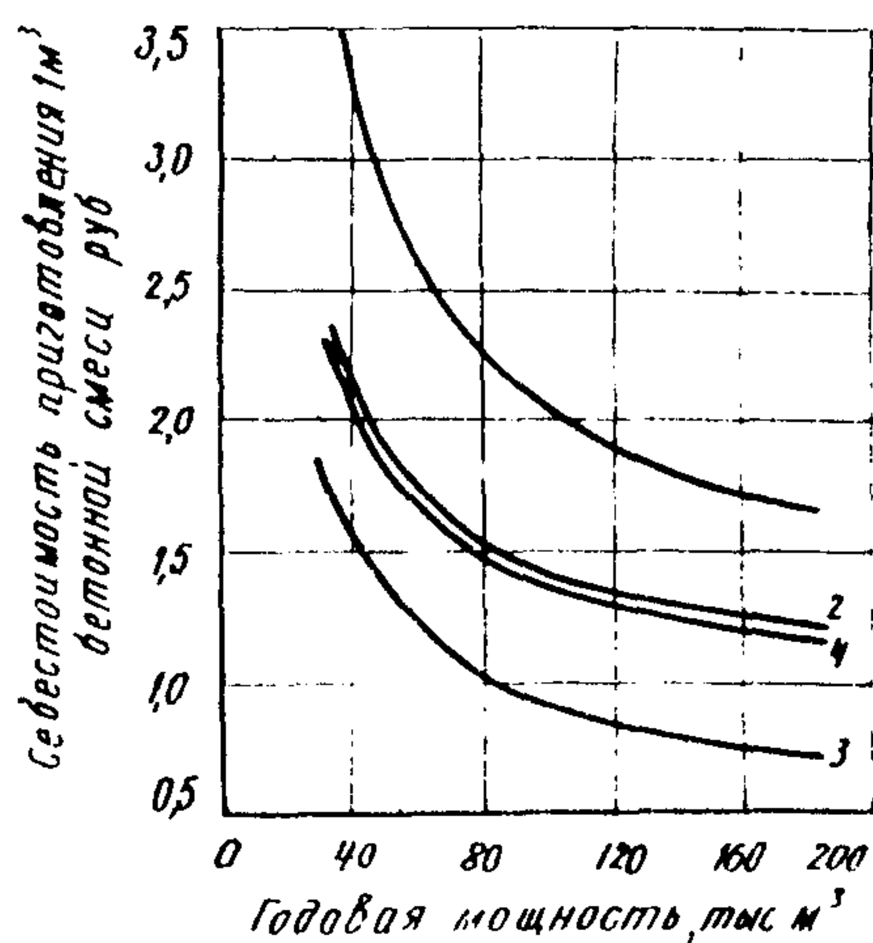
Рис.3. Зависимость себестоимости приготовления 1\text{ м}^3 бетонной смеси от мощности и типа ЦБЗ: 1-стационарные ЦБЗ; 2-инвентарные базы; 3-передвижные ЦБЗ (сборно-разборные); 4-передвижные ЦБЗ смонтированные на колесном ходу
