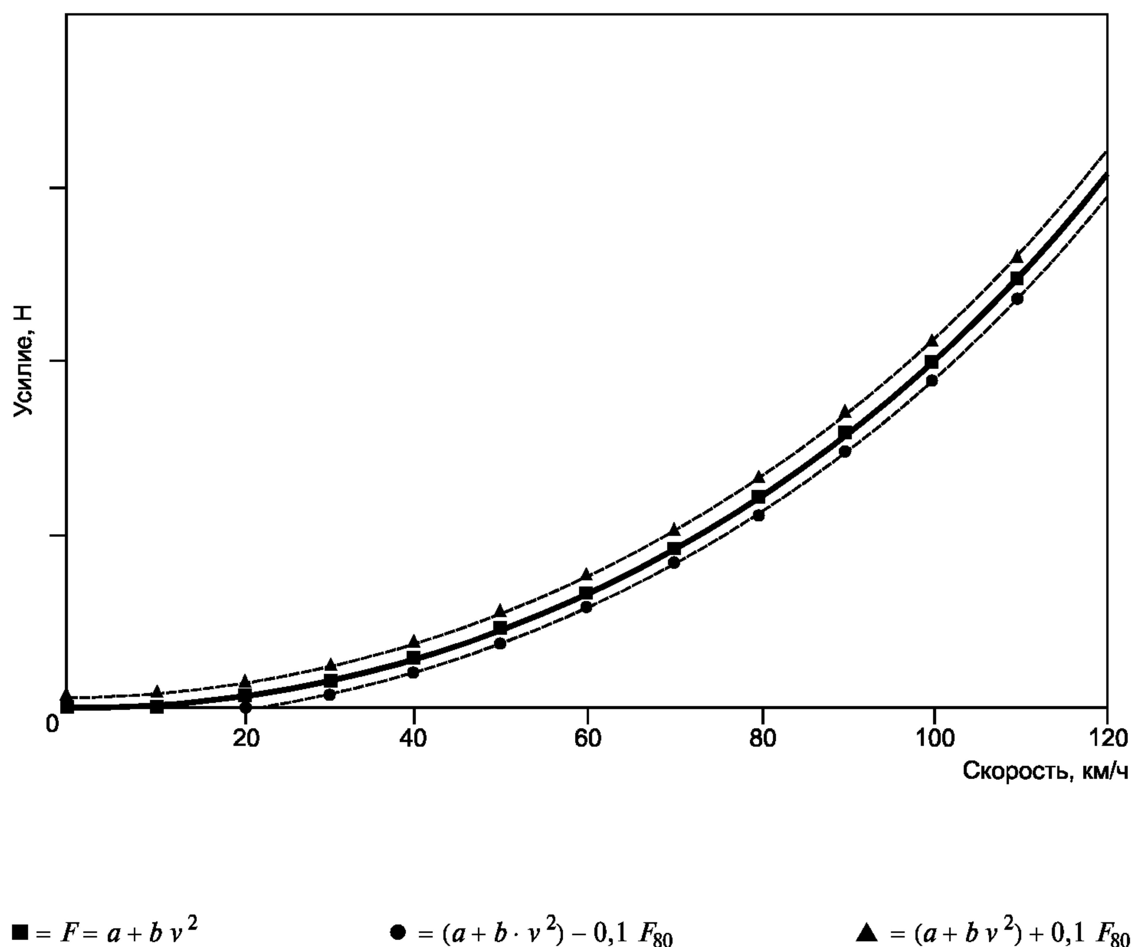
Рисунок Г.4 — График нагрузок, поглощенных динамометрическим стендом
