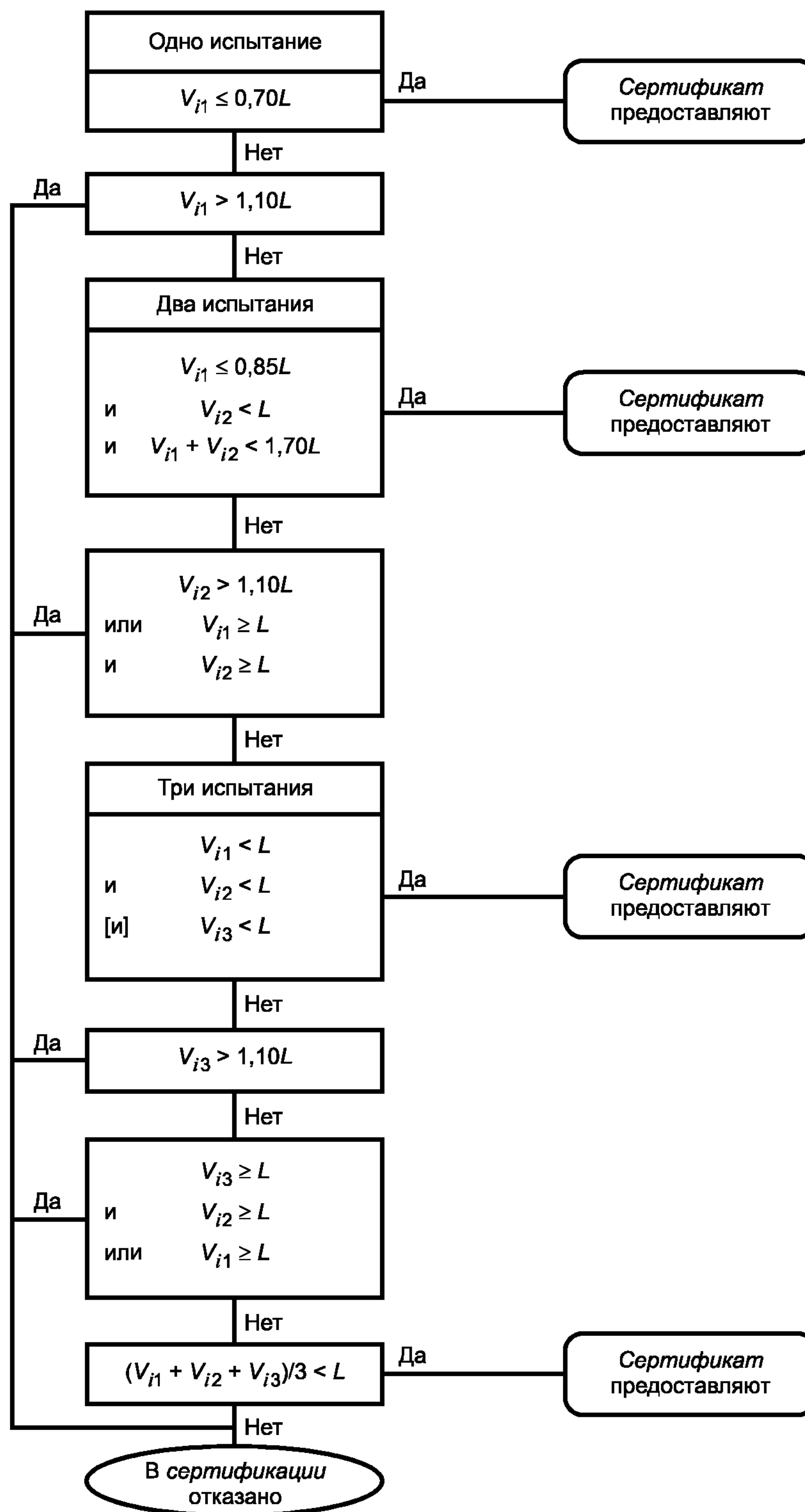
Рисунок 1 — Схема проведения сертификационных испытаний типа I
