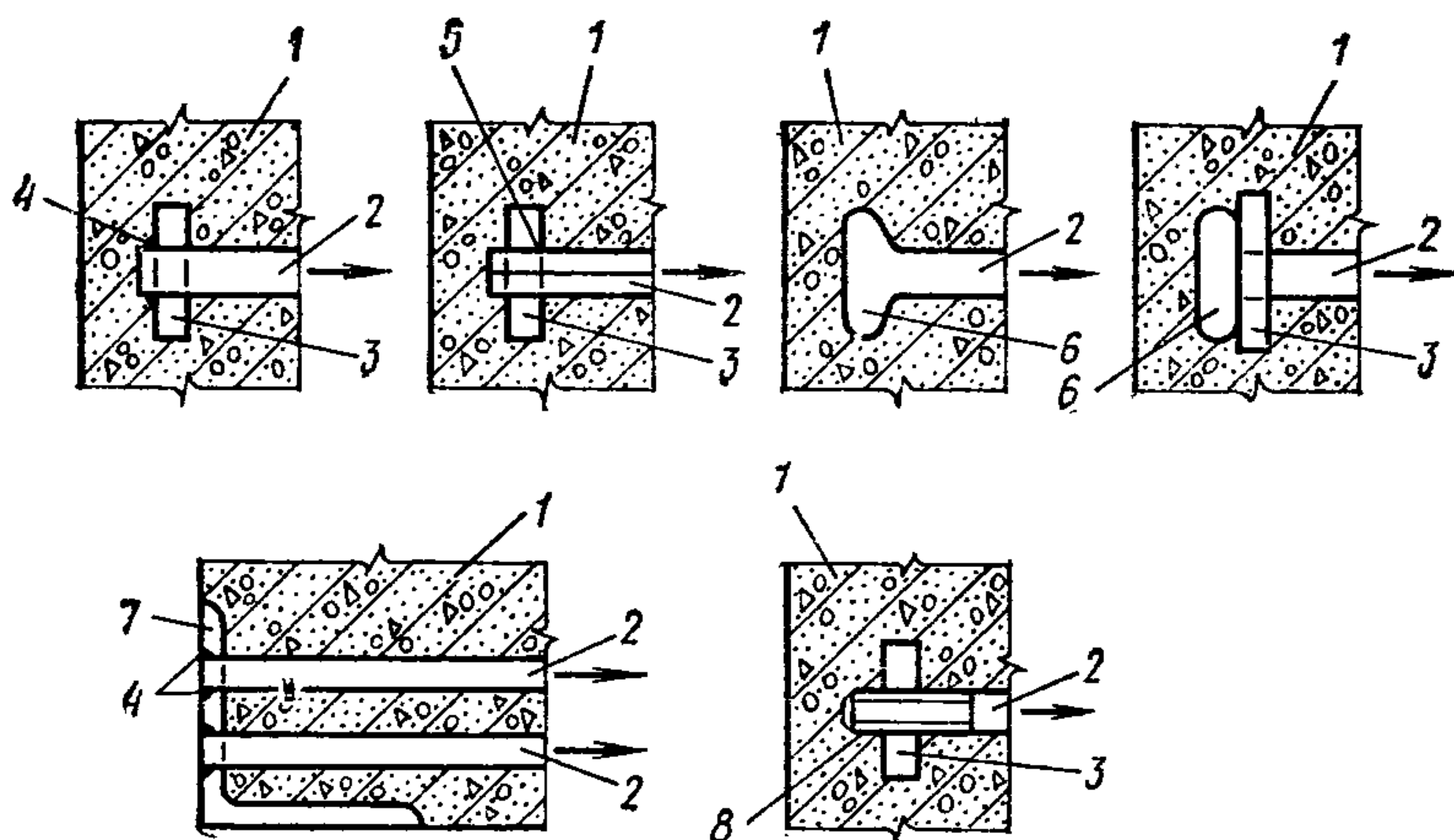
Рис. 25. Анкеровка продольного стержня с помощью специальных устройств
