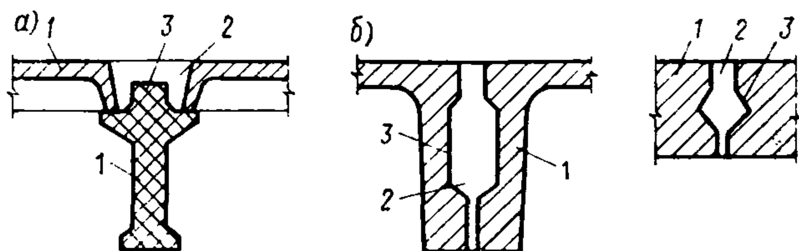
Рис. 110. Сопряжения сборных элементов с дополнительно уложенным бетоном
