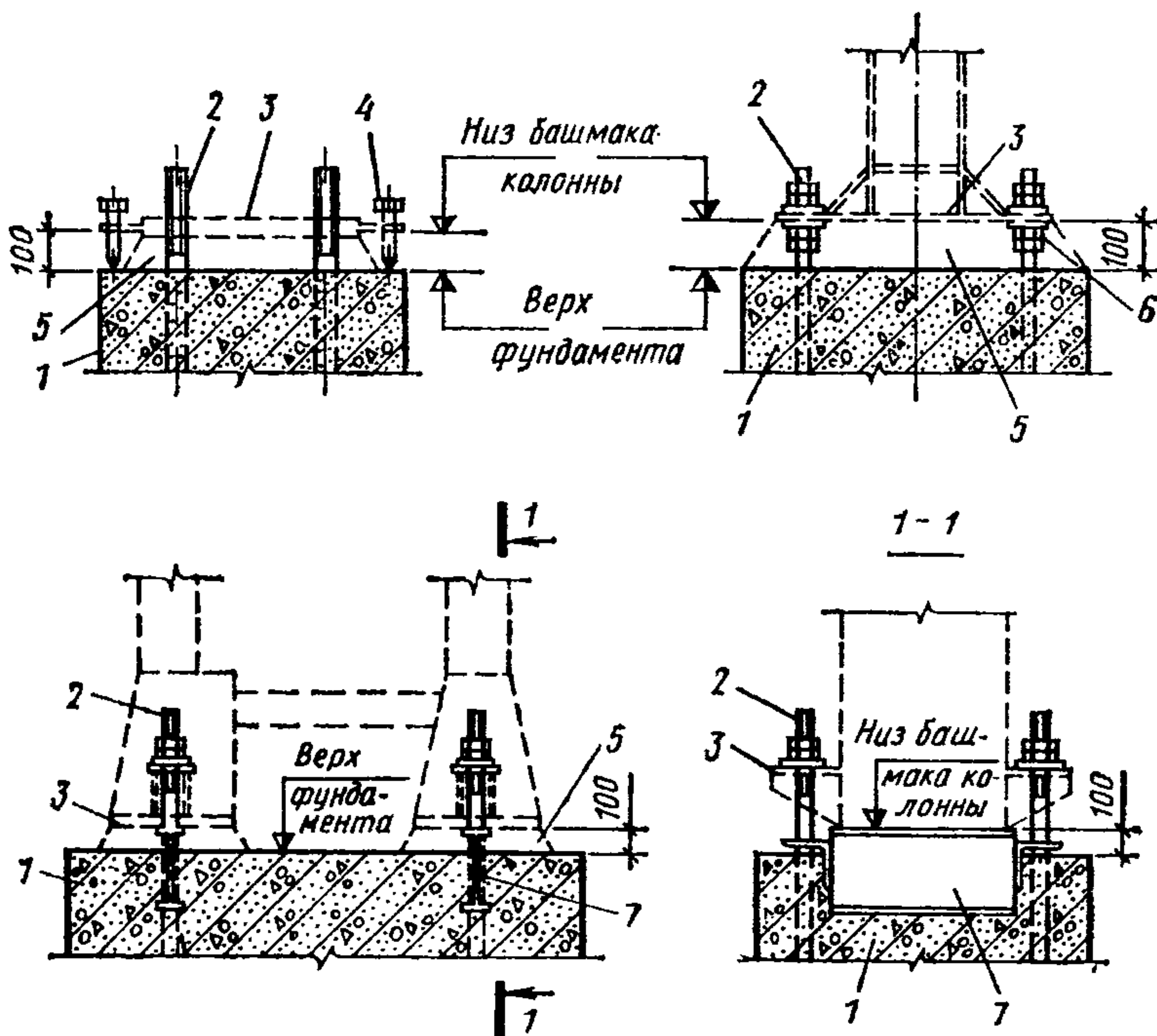
Рис. 65. Опираие стальных конструкций колонн на железобетонные фундаменты
