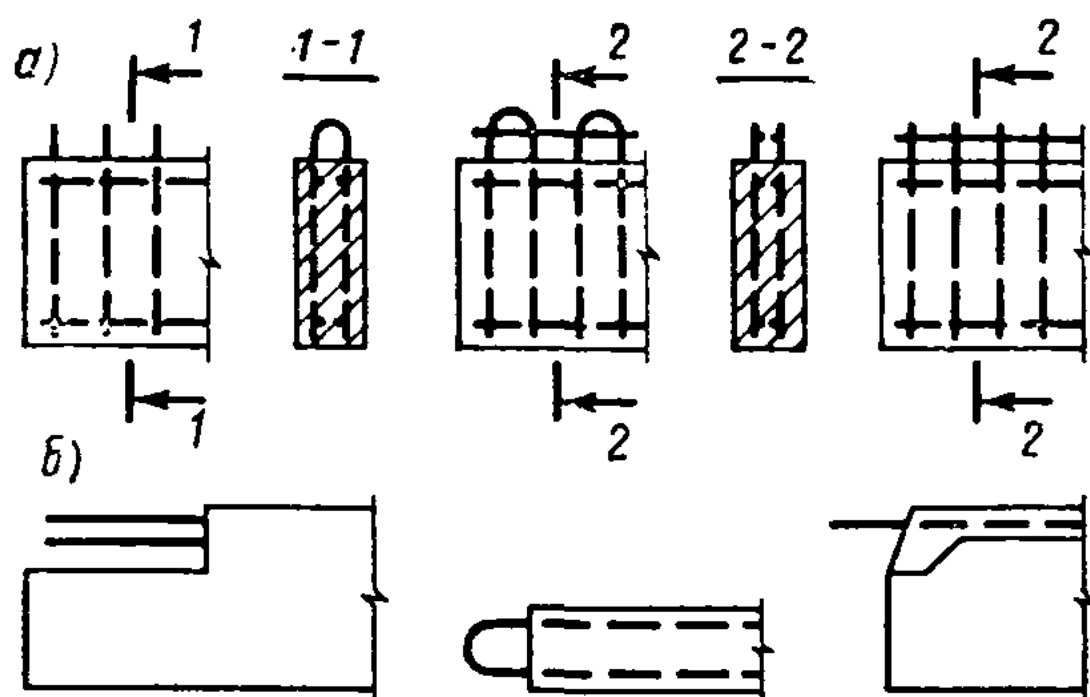
Рис. 111. Выпуски арматуры из сборных элементов
