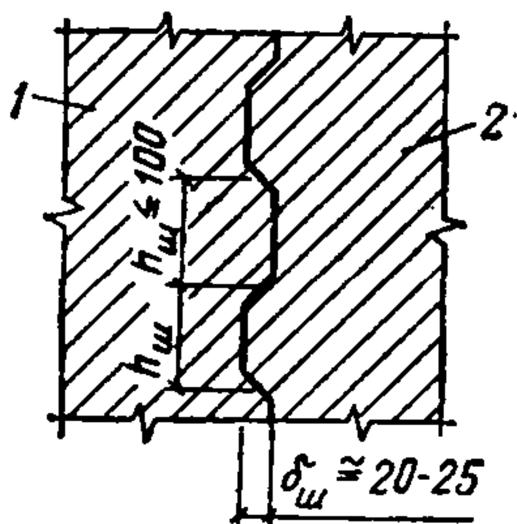
Рис. 82. Деталь сопряжения сборной колонны с бетоном замоноличивания стакана фундамента 1 — сборная колонна; 2 — бетон замоноличивания
