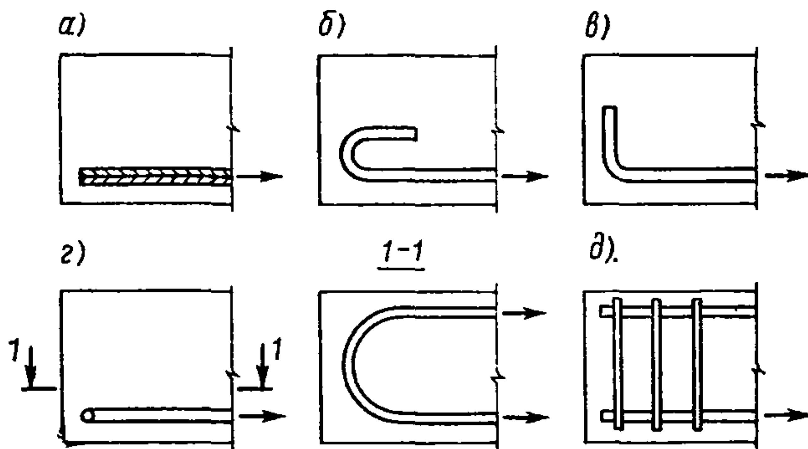
Рис. 22. Анкеровка рабочей арматуры в бетоне элемента
