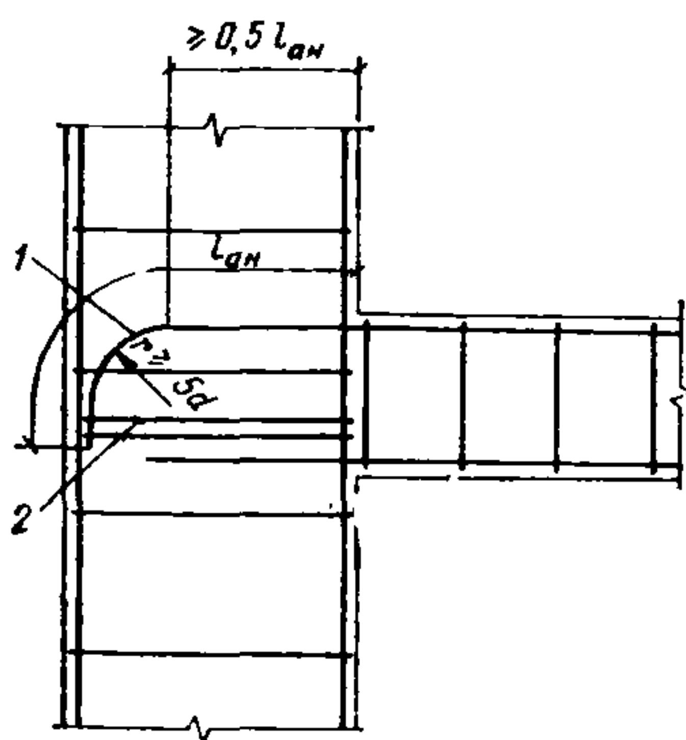
Рис. 26. Анкеровка продольного стержня посредством его отгиба
