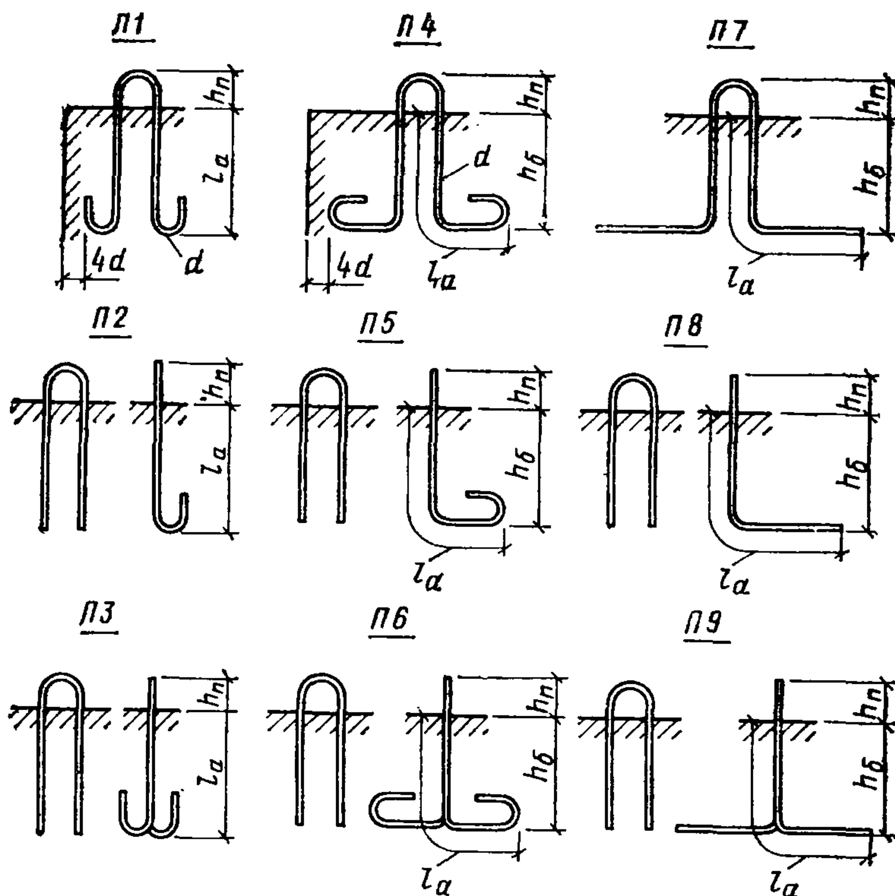
Рис. 40. Рекомендуемые типы строповочных петель
