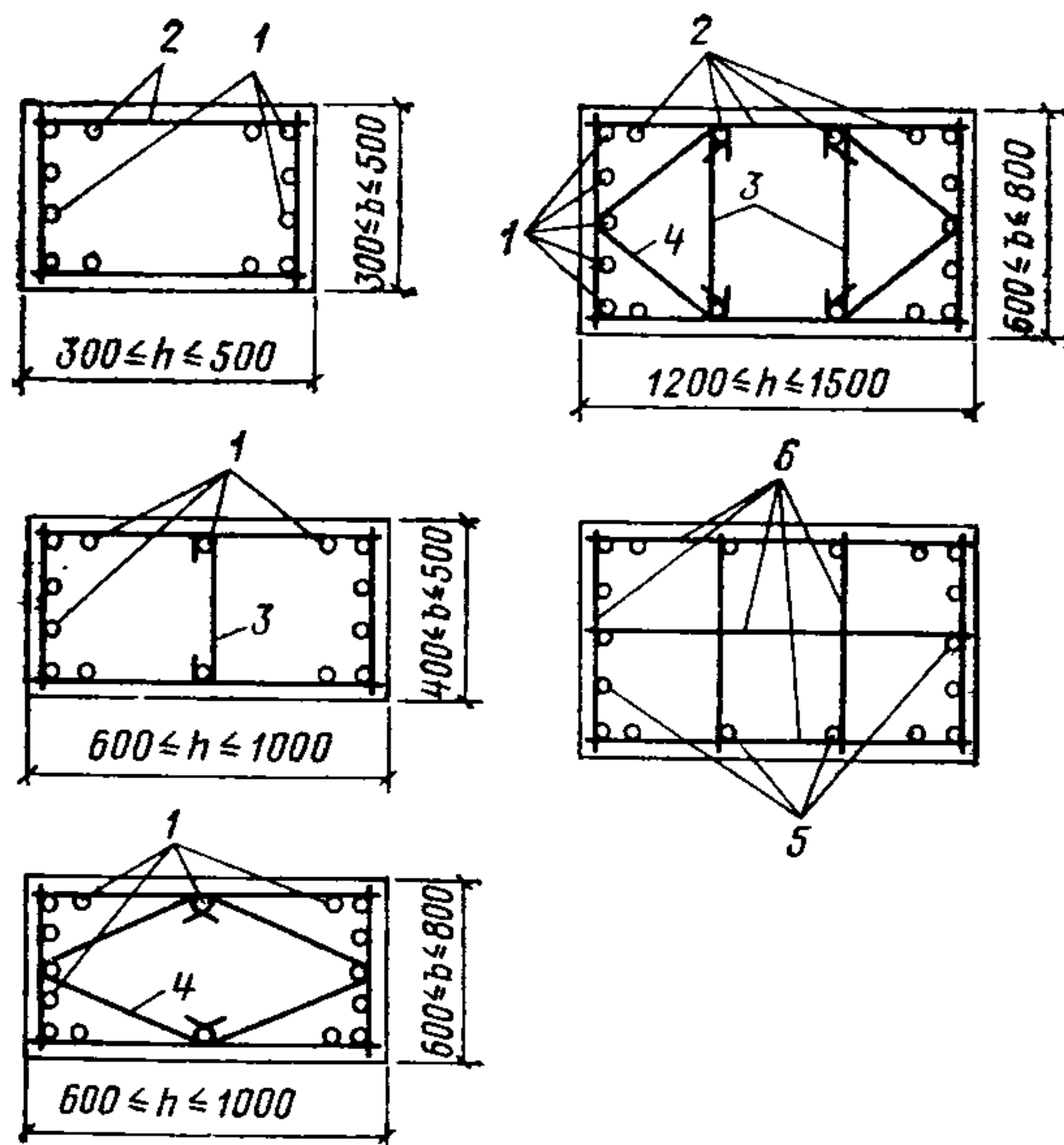
Рис. 72. Примеры армирования сечений колонн с рекомендуемым числом стержней сварными сетками
