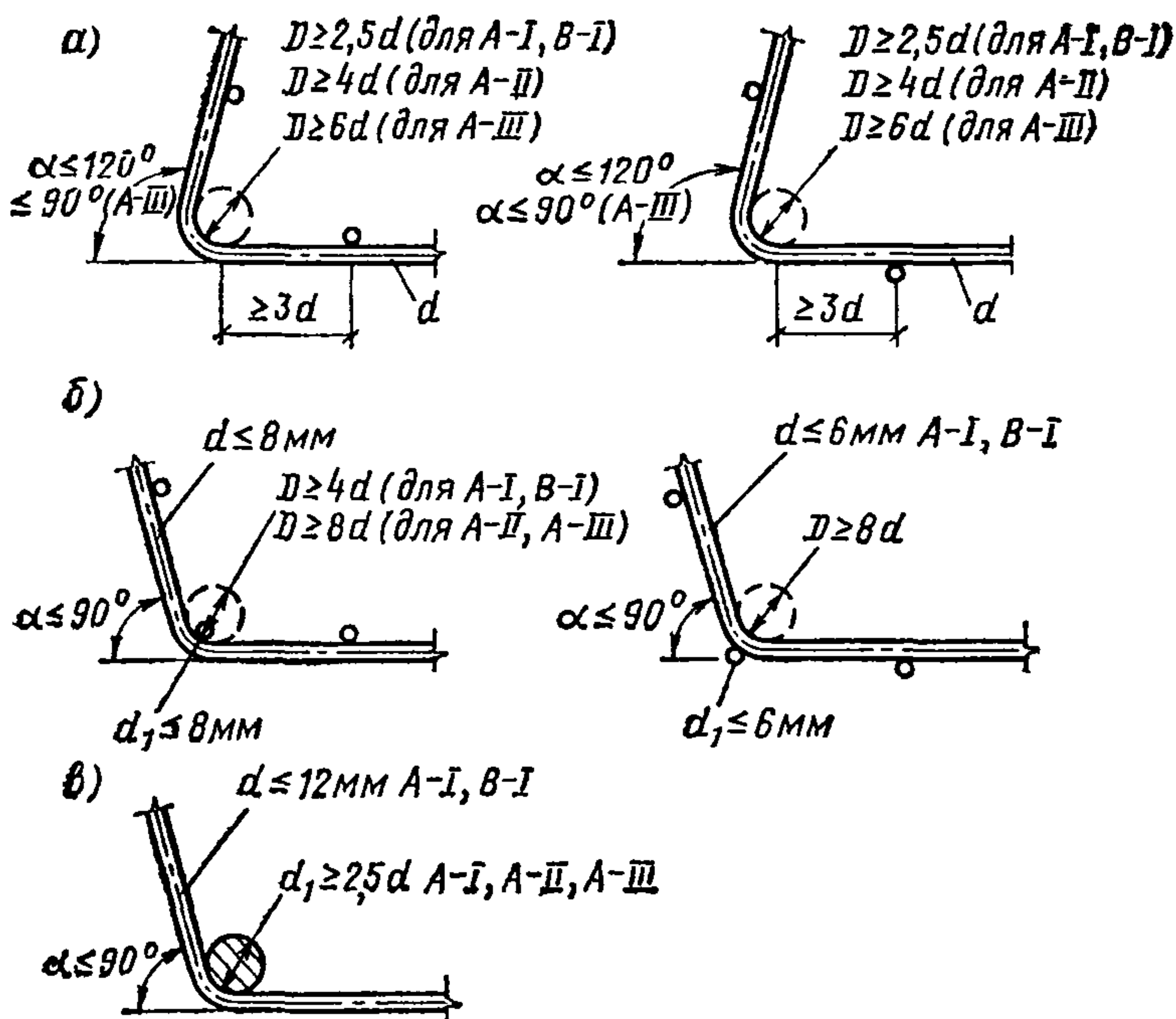
Рис. 8. Конструирование мест сгиба сеток
