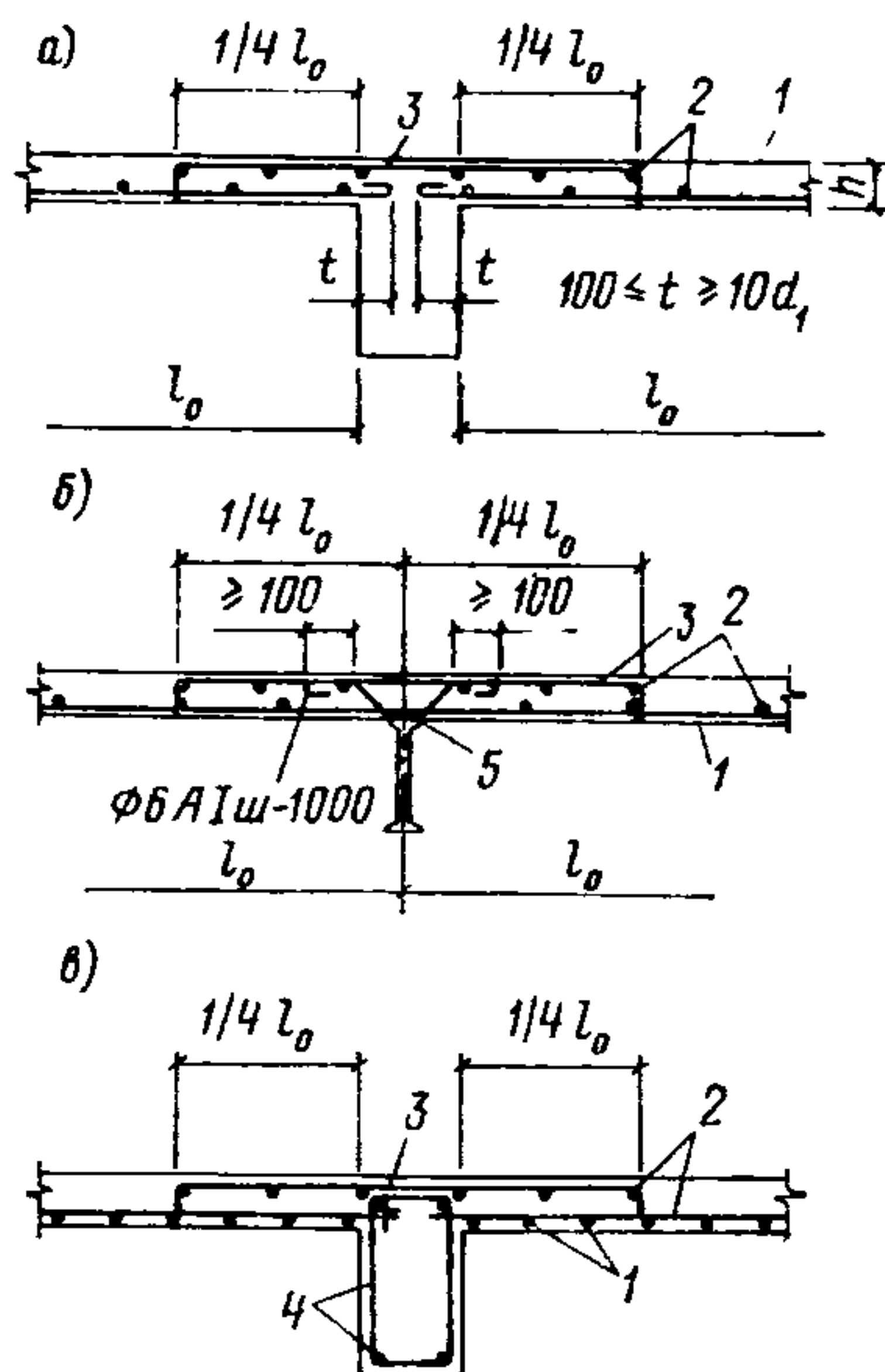
Рис. 107. Армирование средних опор монолитной плиты отдельными стержнями
