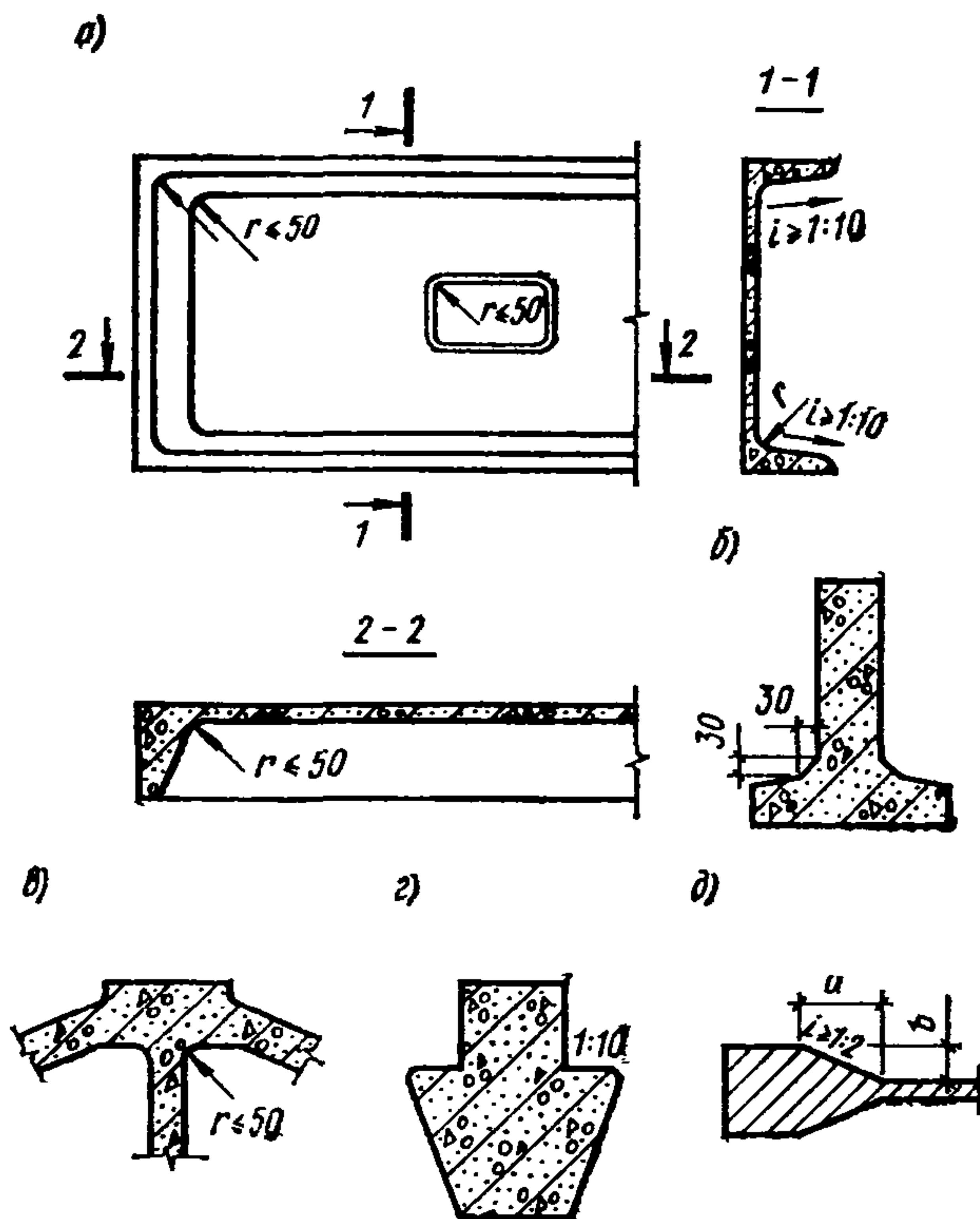
Рис. 46. Фаски, закругления и скосы в железобетонных элементах
