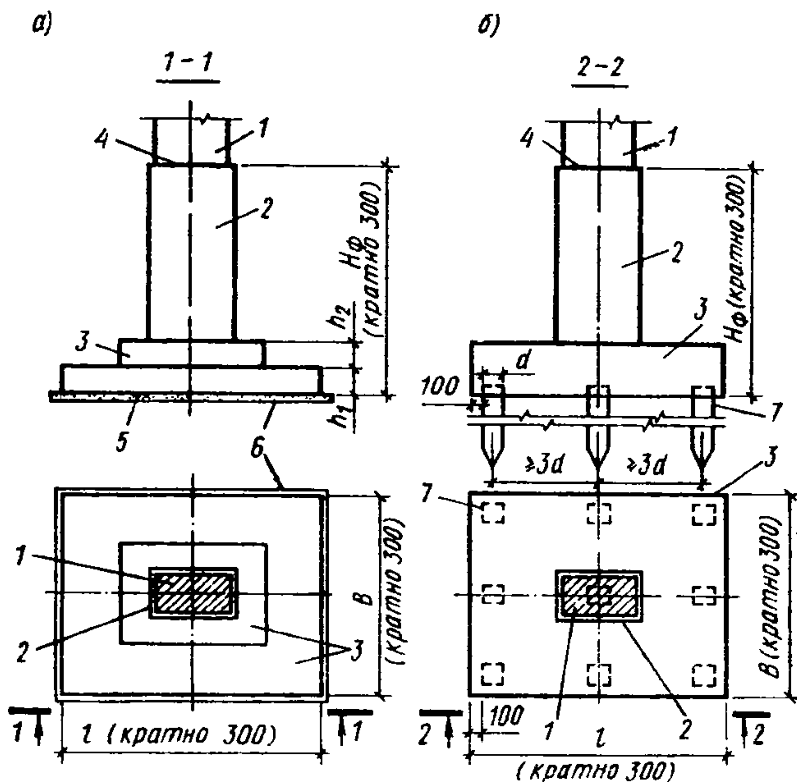
Рис. 48. Отдельные ступенчатые фундаменты
