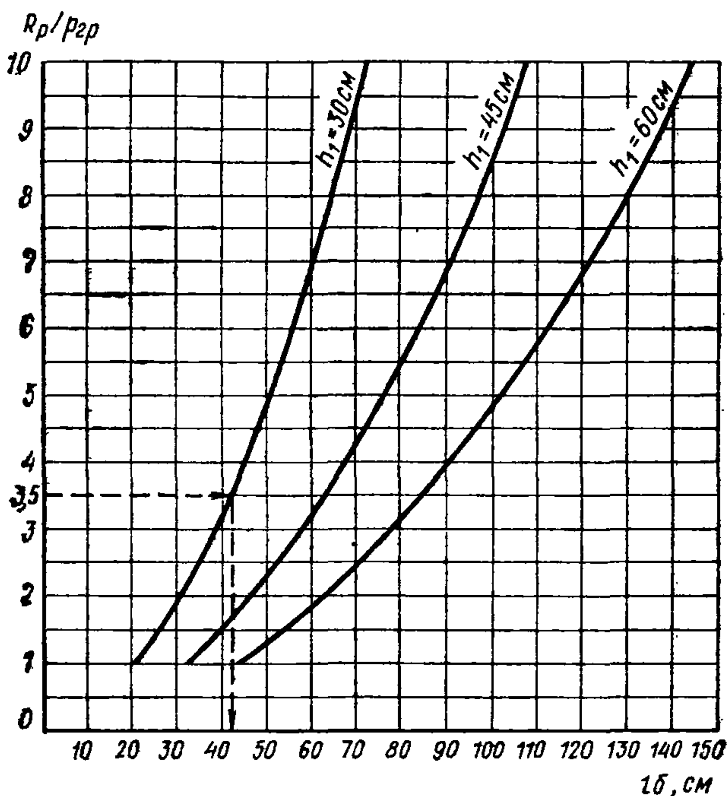
Рис. 53. График для определения длины участка l_6 , на которой прочность наклонных сечений обеспечивается бетоном нижней ступени фундамента
