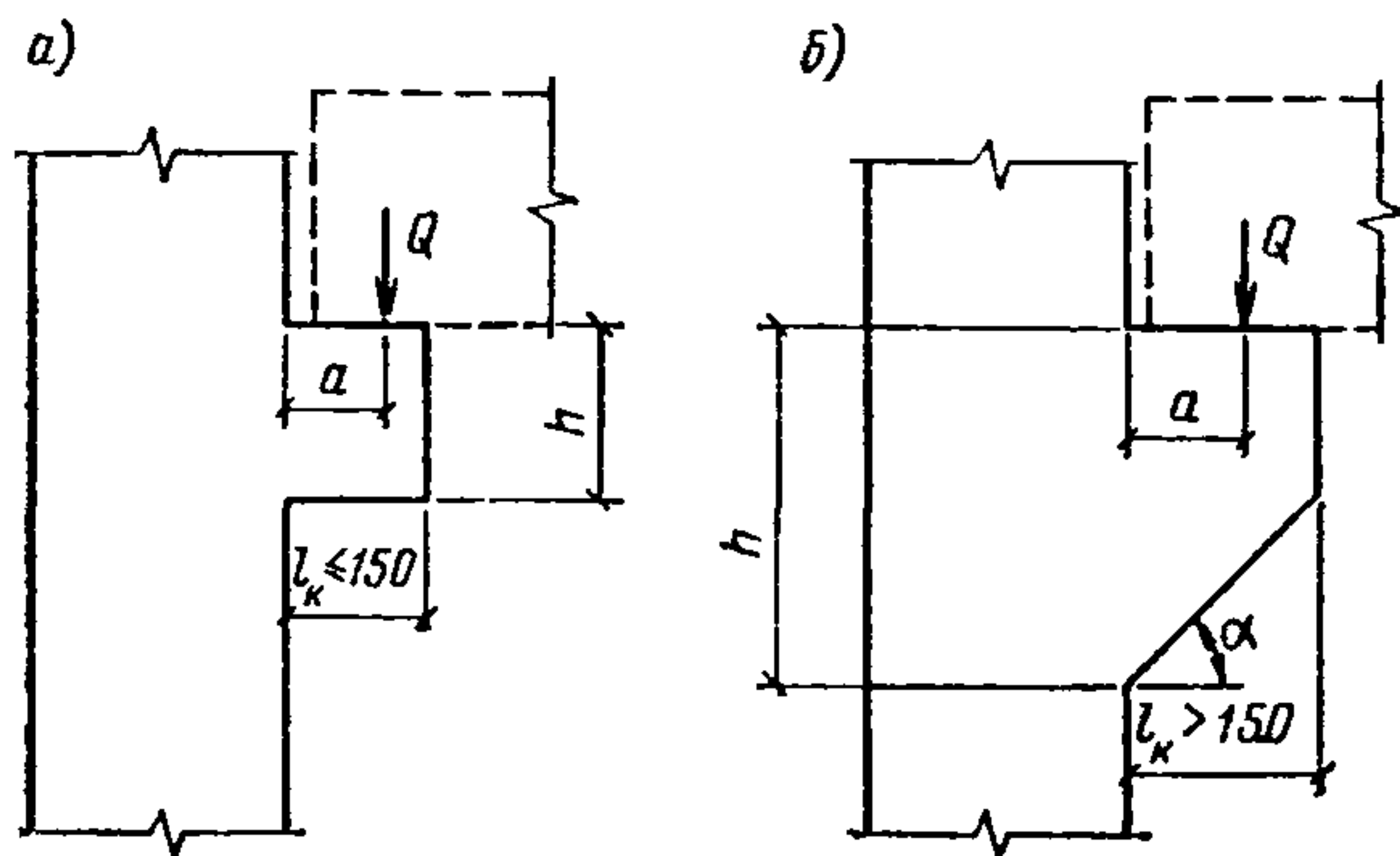
Рис. 77. Короткие консоли колонны
