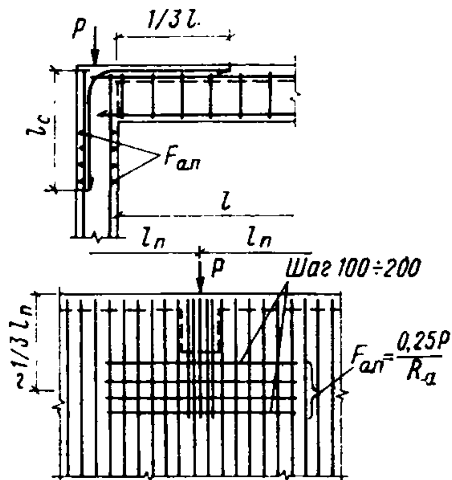
Рис. 117. Схема армирования узла сопряжения ригеля перекрытия со стеной подвала
