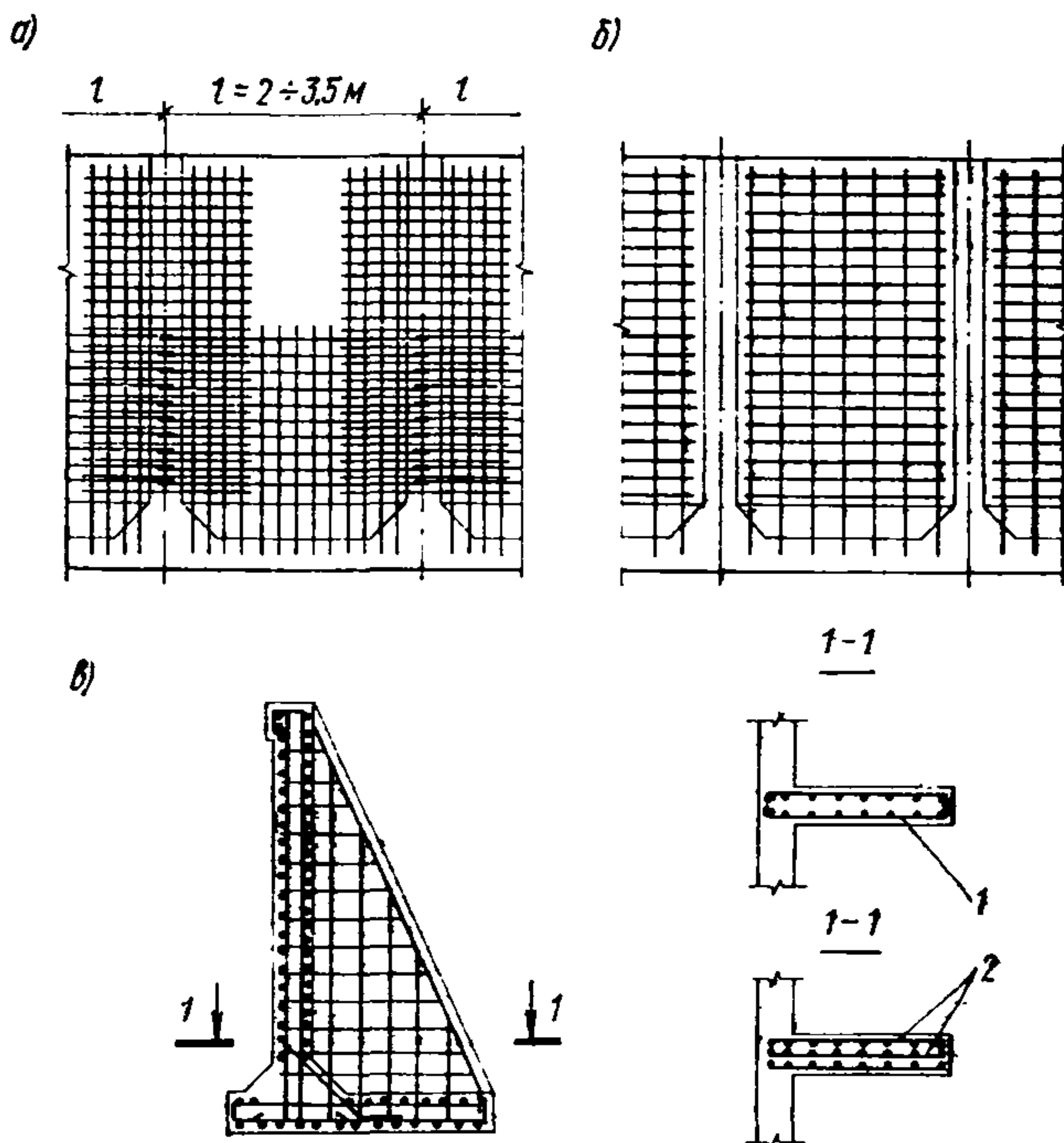
Рис. 120. Пример конструирования монолитной подпорной стены с контрфорсами
