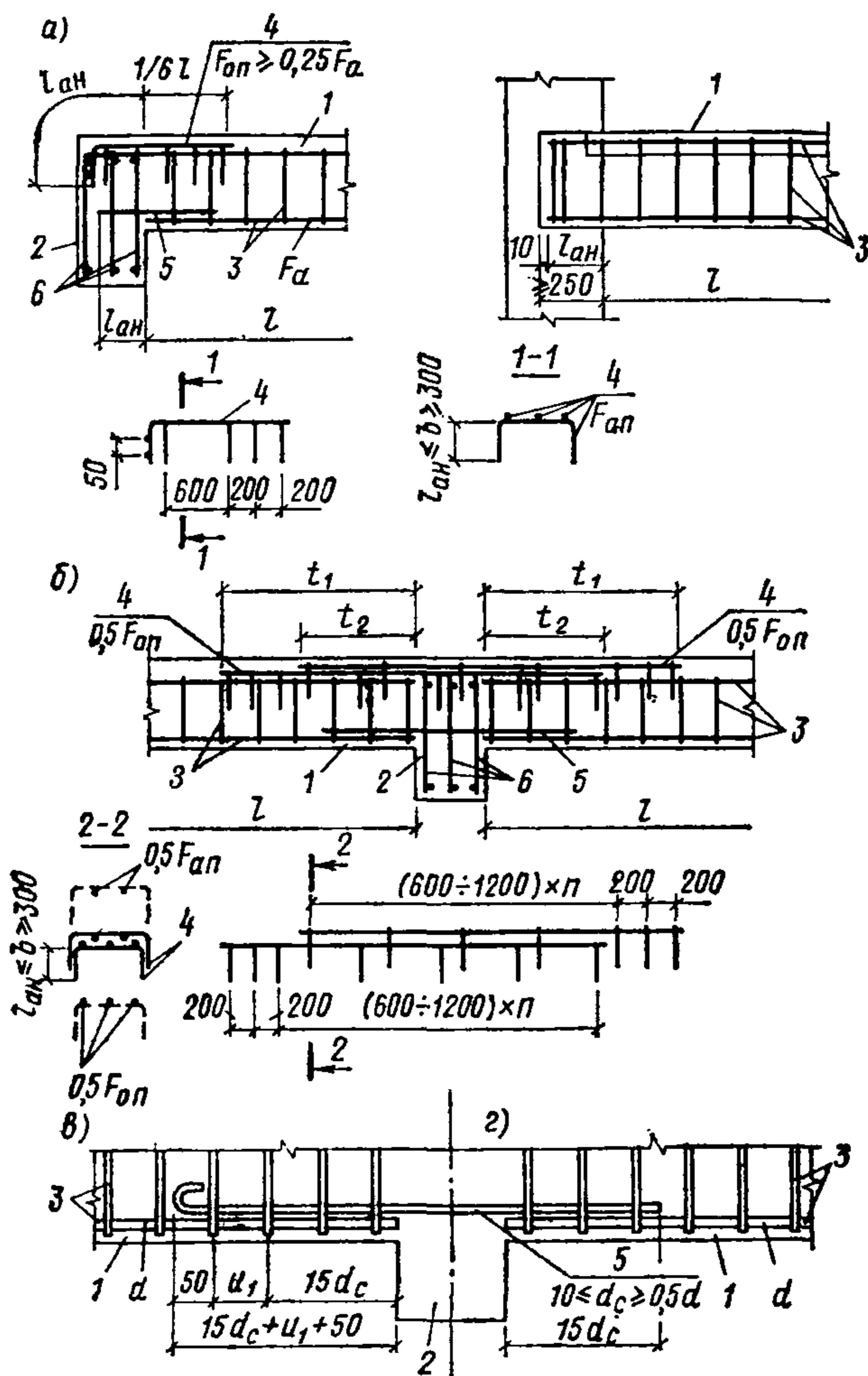
Рис. 86. Армирование второстепенных монолитных балок сварными сетками
