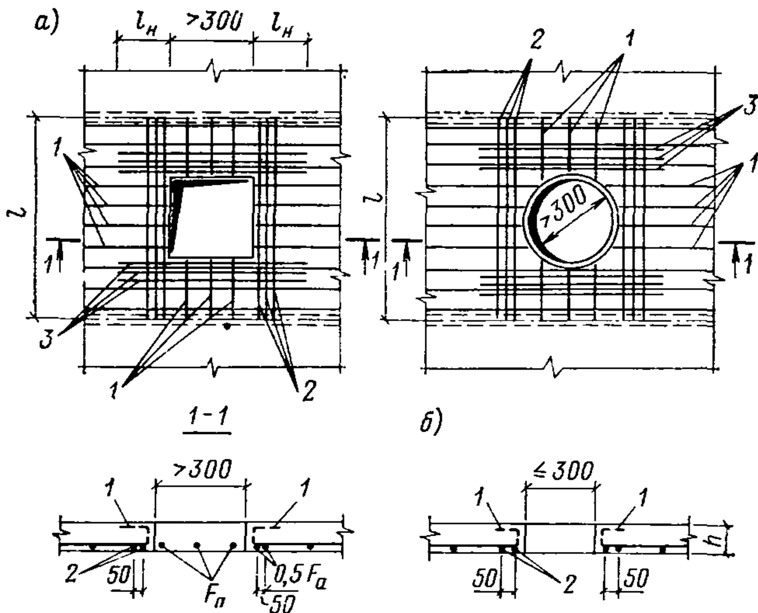
Рис. 108. Армирование плит в местах отверстий
