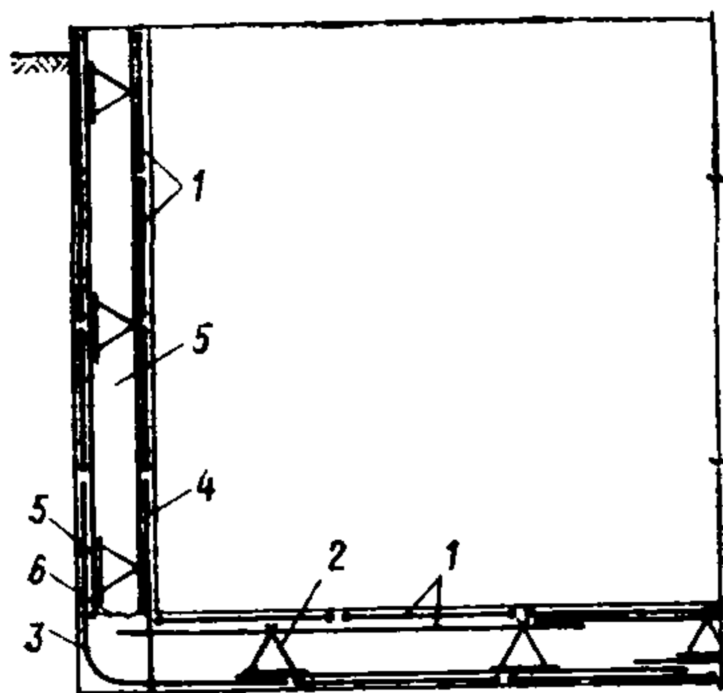
Рис. 116. Армирование стен и днища подвалов (прямок и т. п.)
