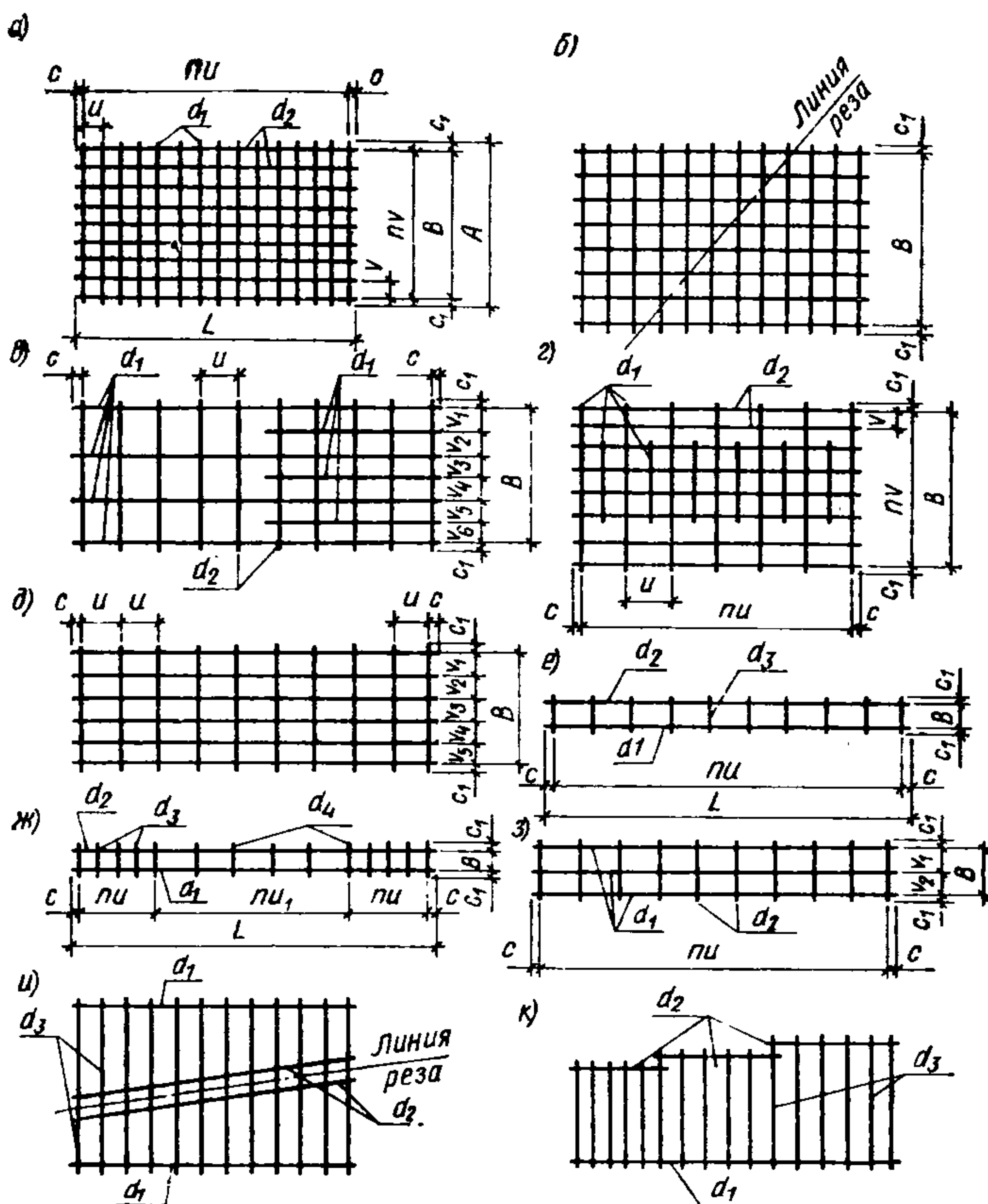
Рис. 5. Основные виды сварных сеток
