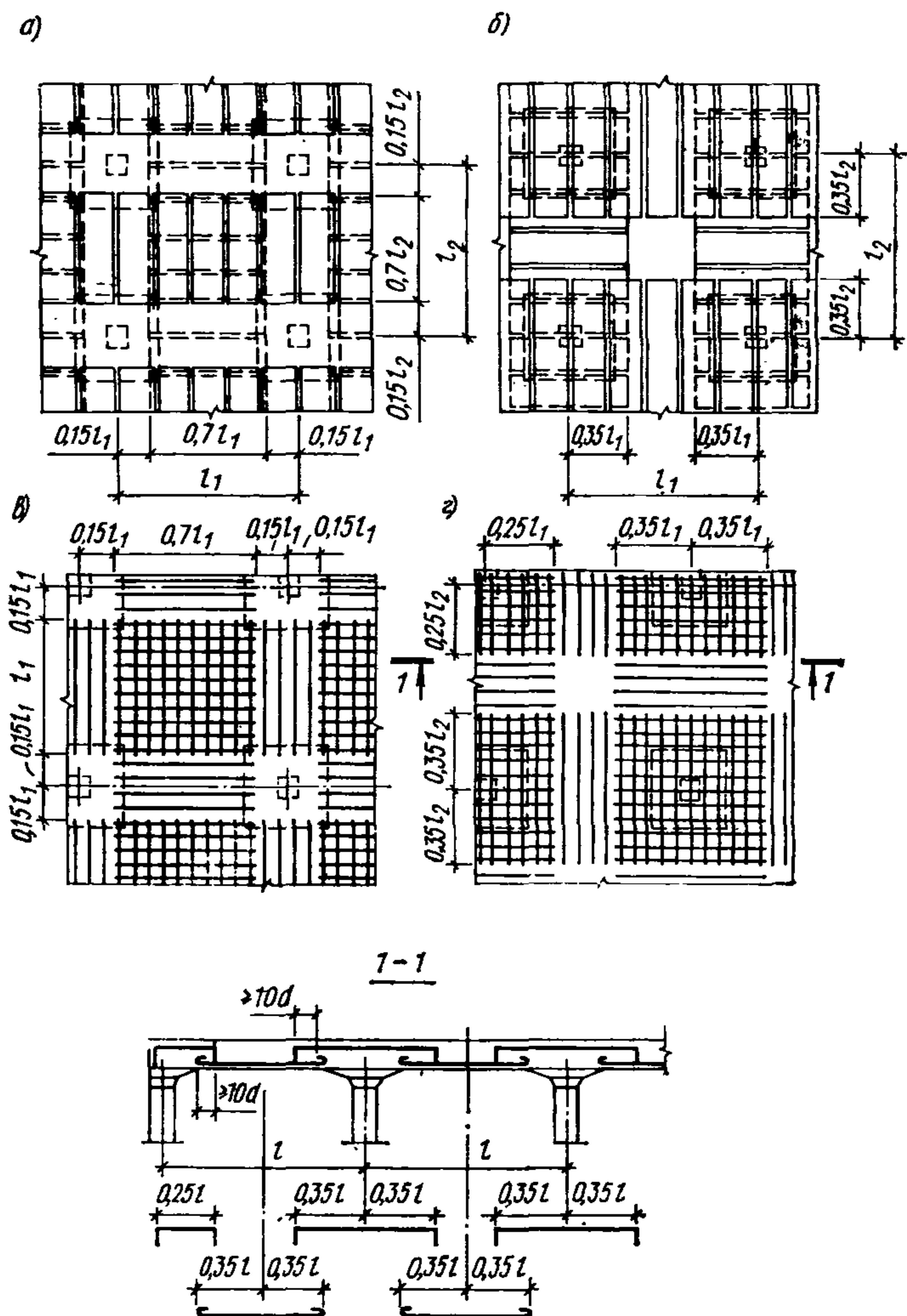
Рис. 115. Схема армирования безбалочных перекрытий
