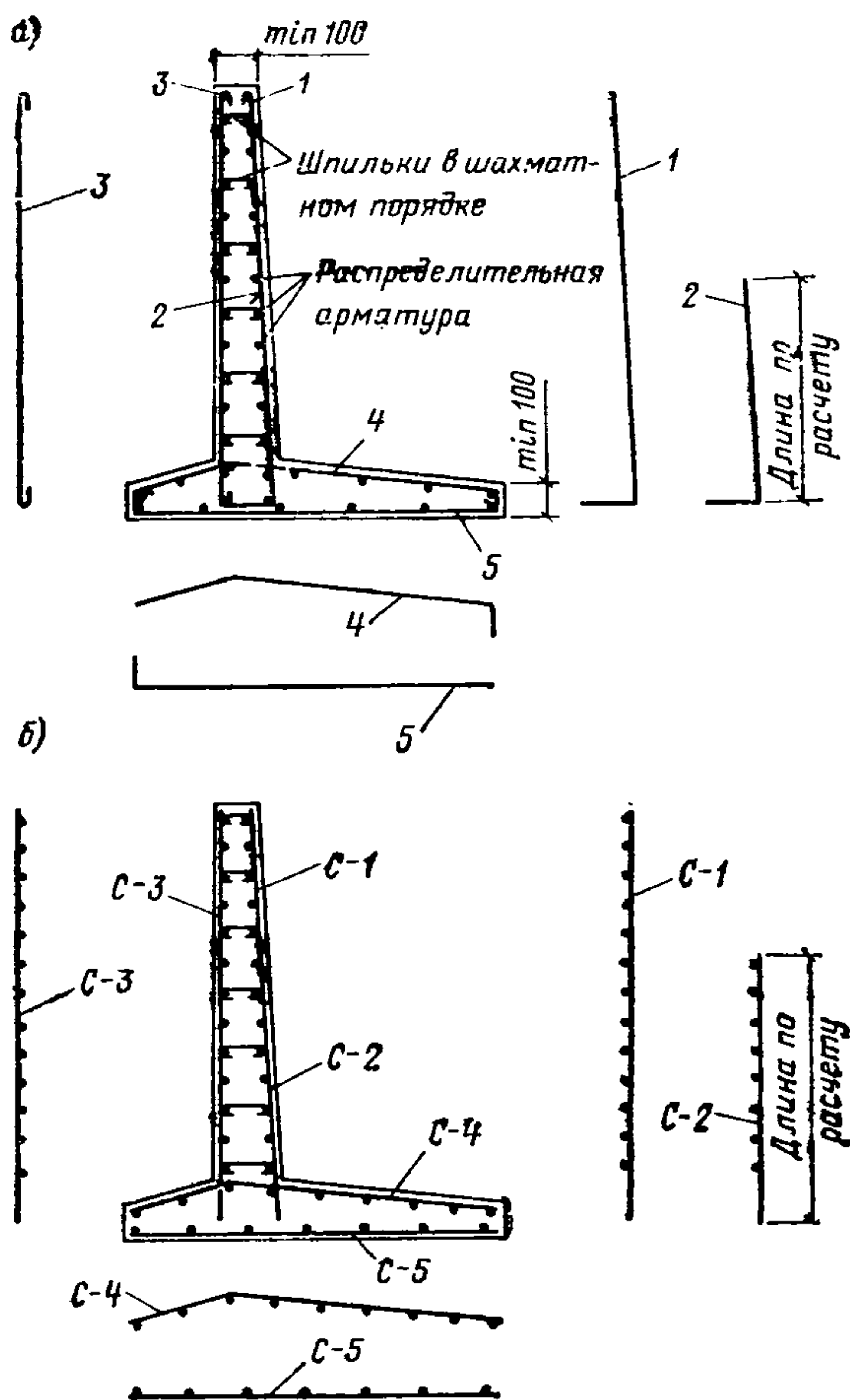
Рис. 119. Схема армирования монолитной гладкой подпорной стены а — отдельными стержнями; б — сварными сетками; 1—5 — арматурные стержни; С-1—С-5 — сварные сетки
