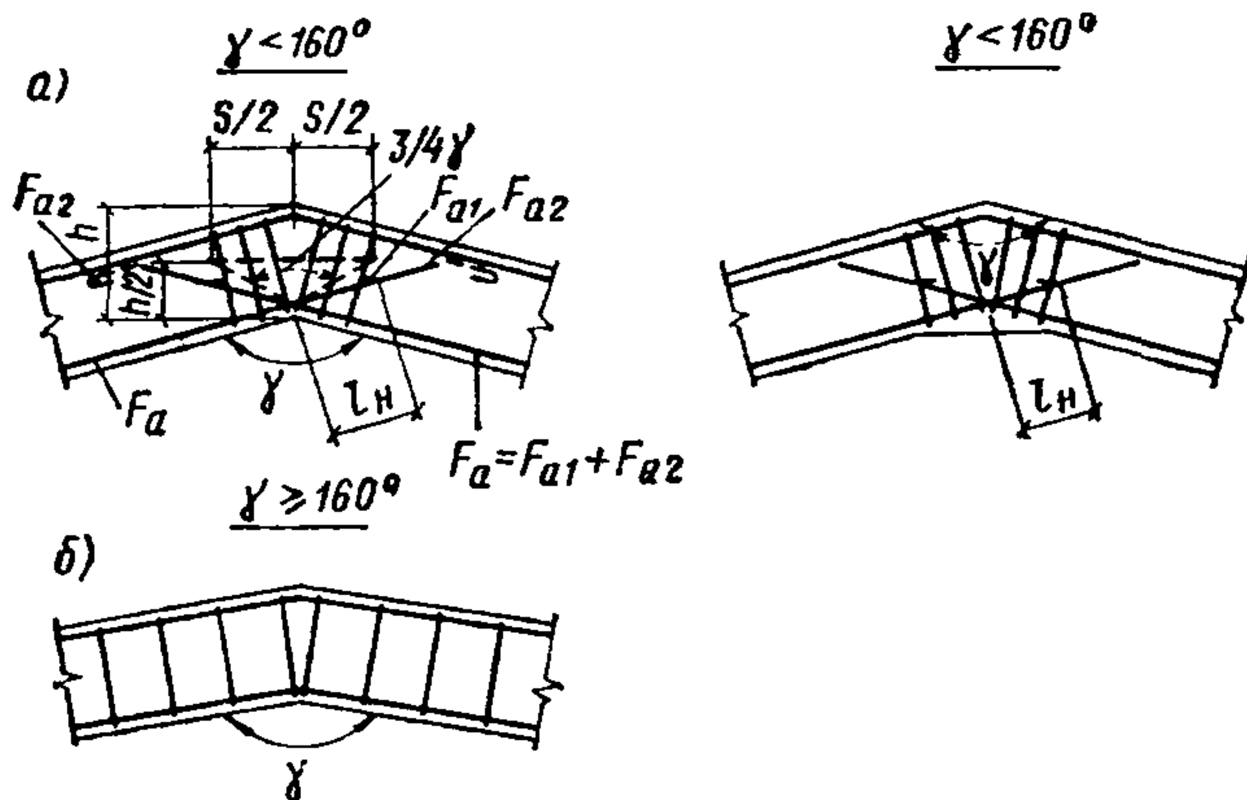
Рис. 95. Схема армирования узла сопряжения ломаного ригеля
