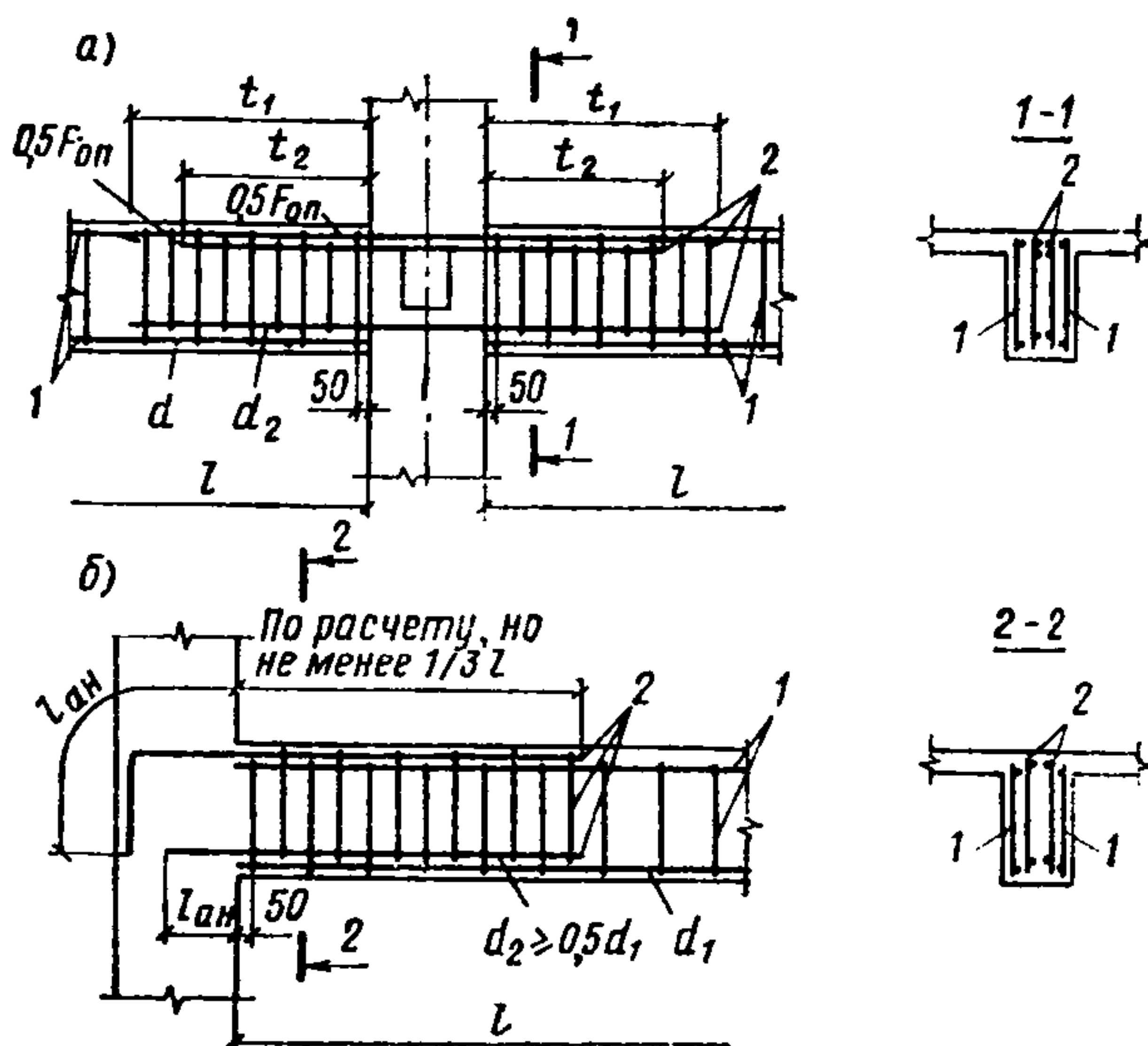
Рис. 88. Армирование опор монолитных главных балок сварными сетками
