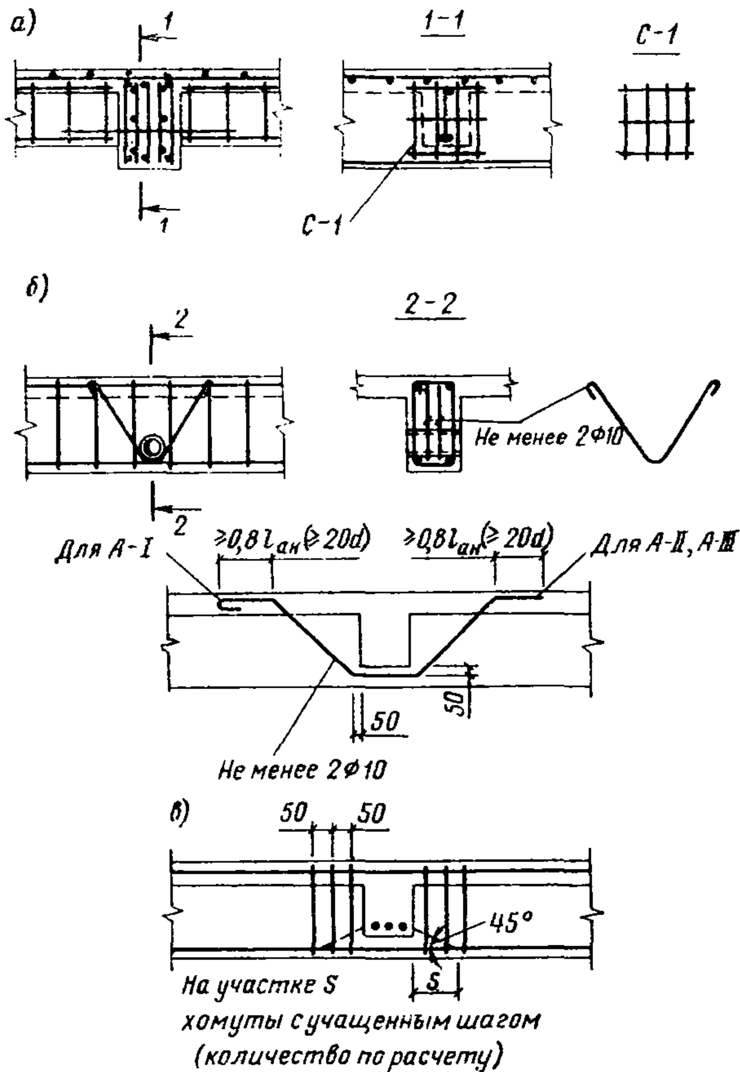
Рис. 92. Дополнительное армирование балок в местах сосредоточенных нагрузок
