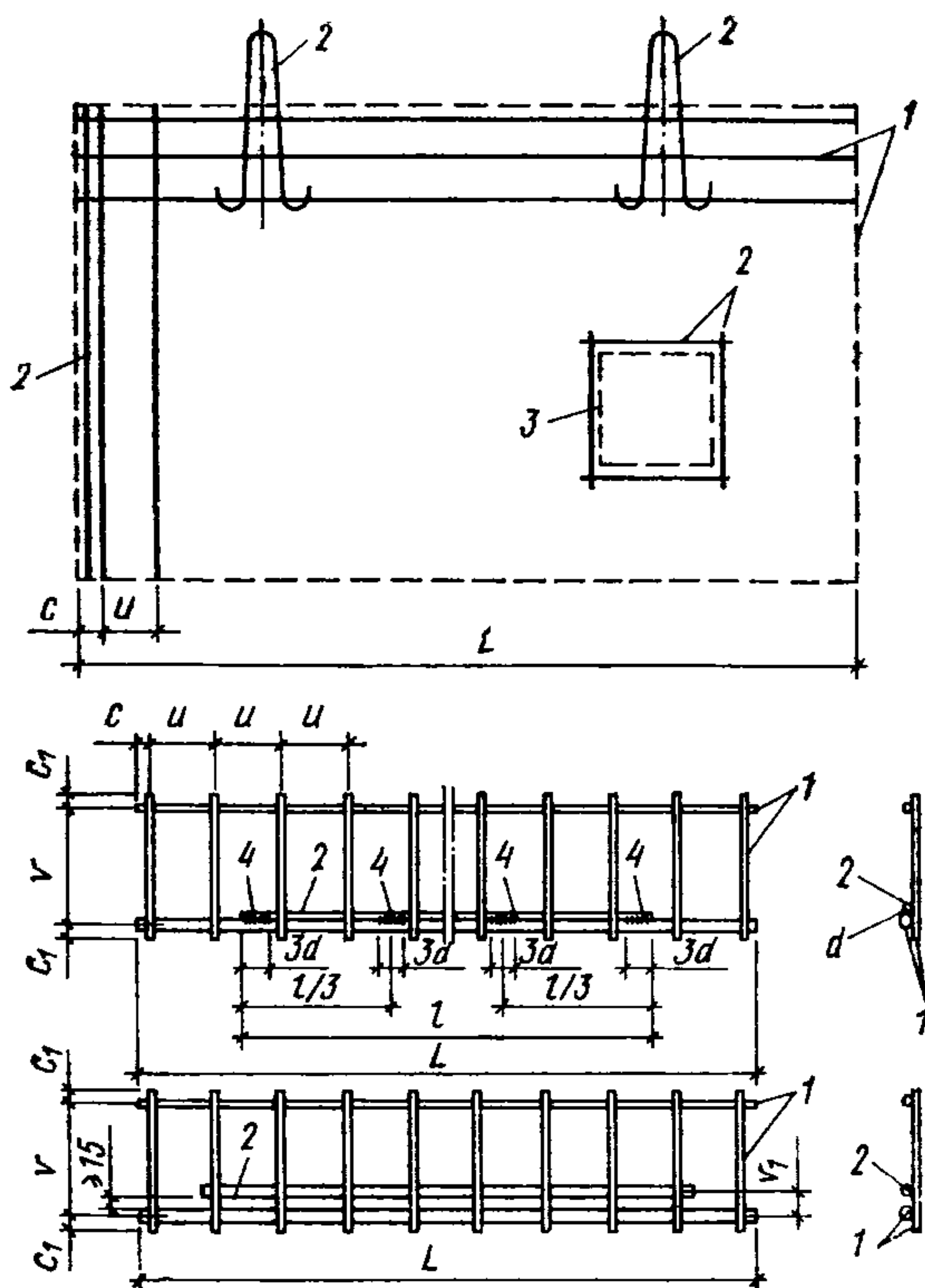
Рис. 6. Виды доработки сеток
