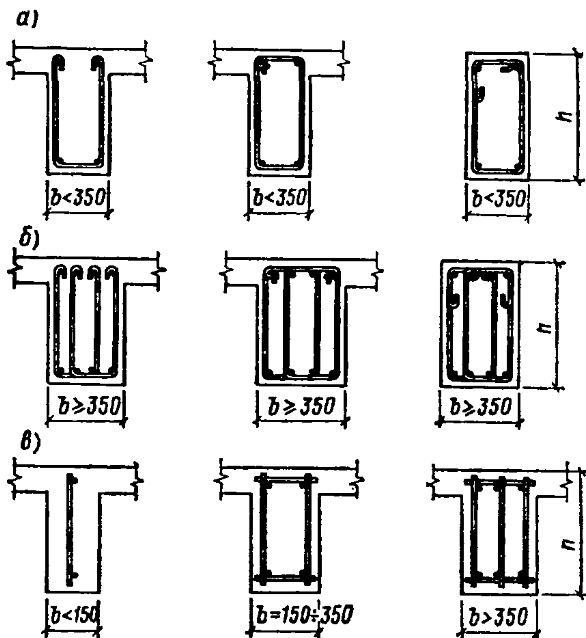
Рис. 85. Схемы армирования сечений балок
