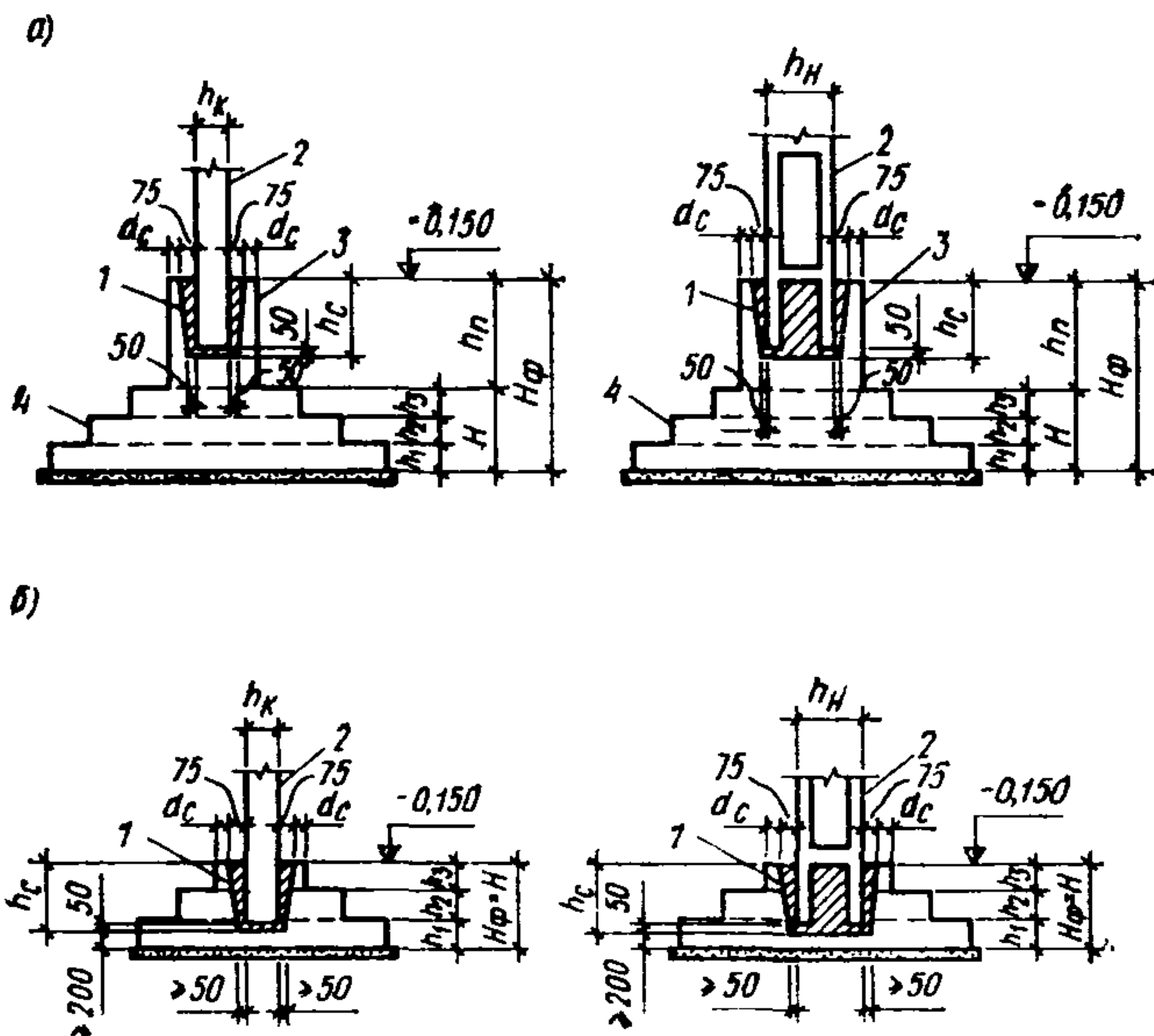
Рис. 59. Монолитные фундаменты сборных колонн
