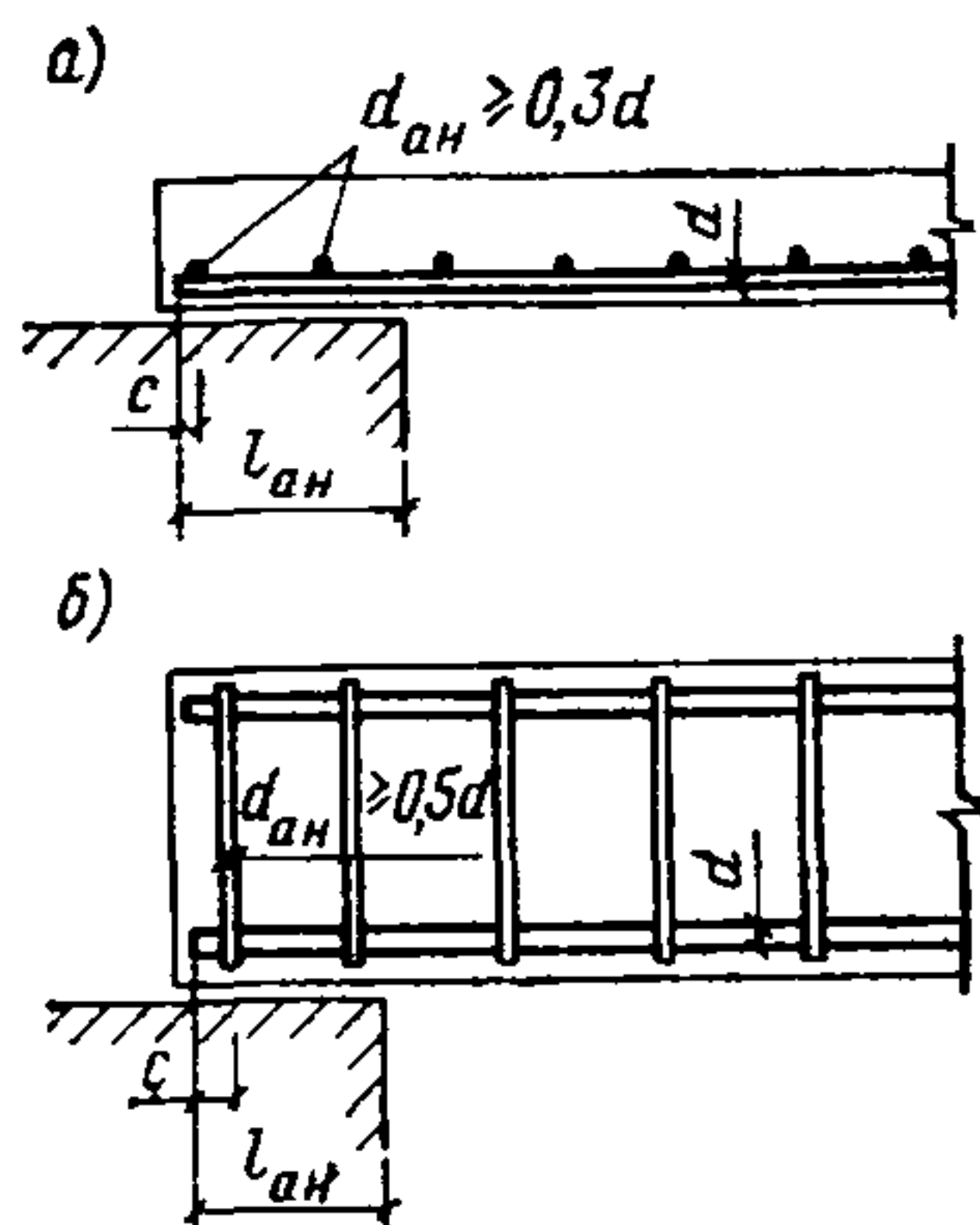
Рис. 27. Анкеровка гладких стержней продольной растянутой сварной арматуры на крайних свободных опорах изгибаемых элементов
