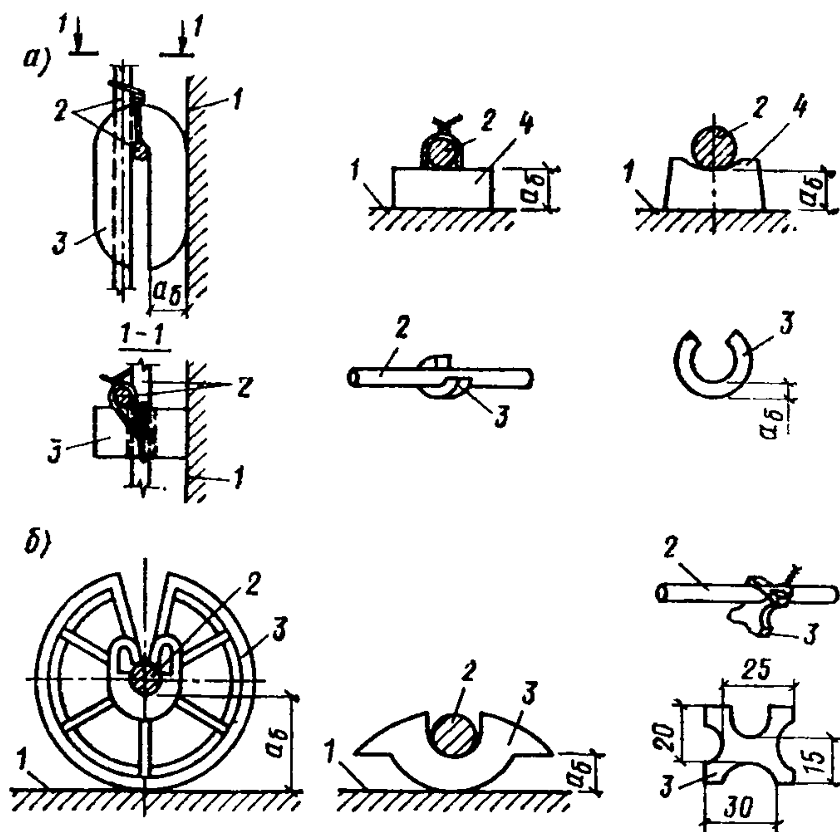
Рис. 43. Пластмассовые и цементно-песчаные фиксаторы однократного использования
