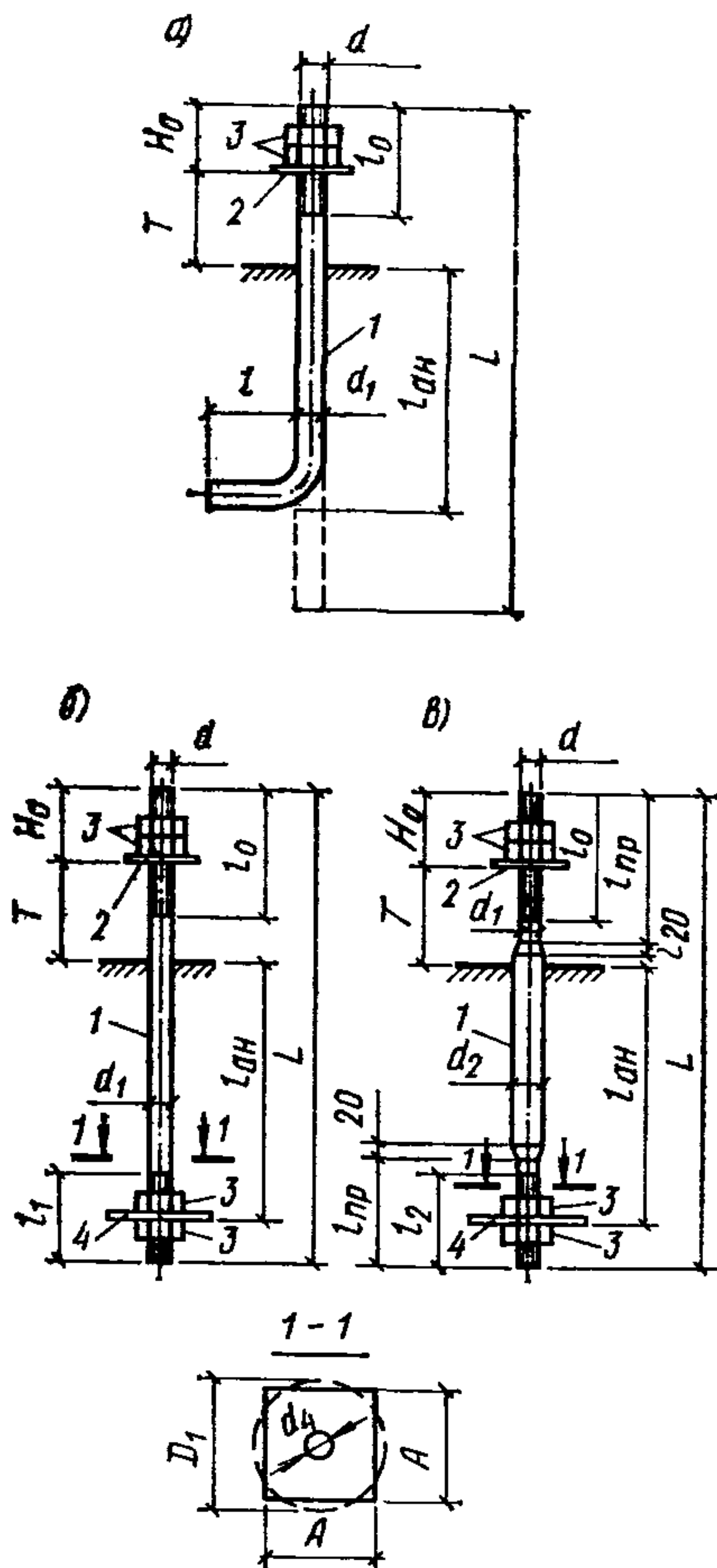
Рис. 67. Фундаментные болты для крепления стальных колонн
