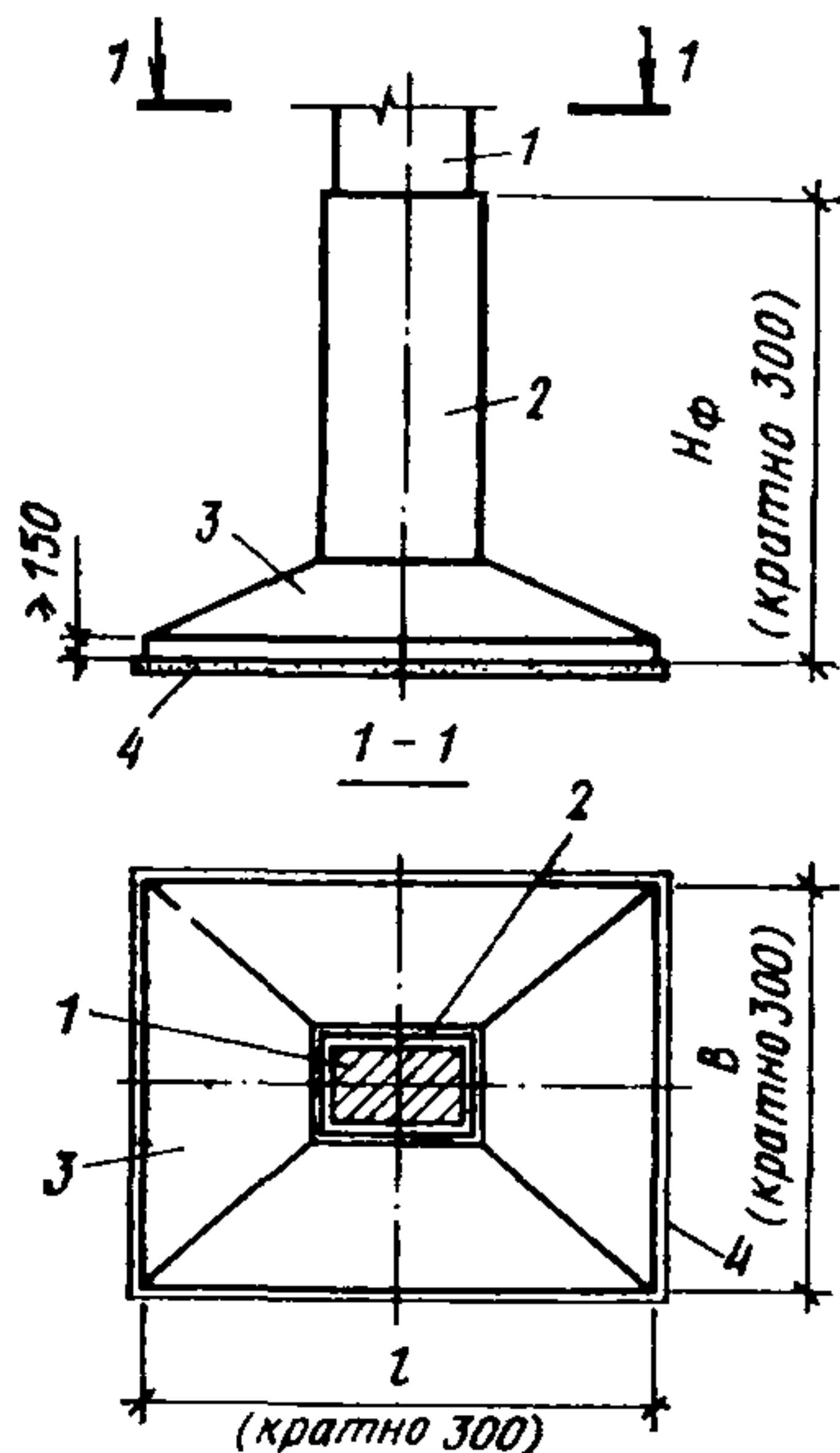
Рис. 49. Отдельный пирамидальный фундамент
