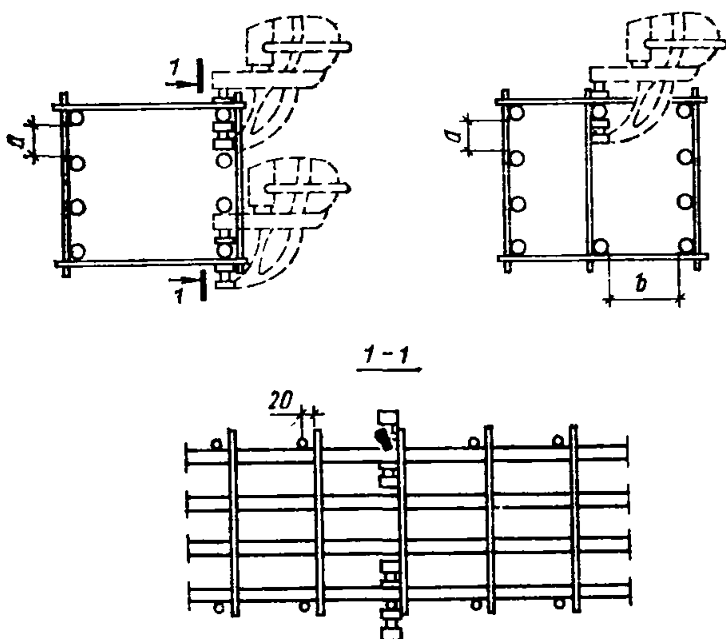
Рис. 14. Положение сварочных клещей при сварке каркаса
