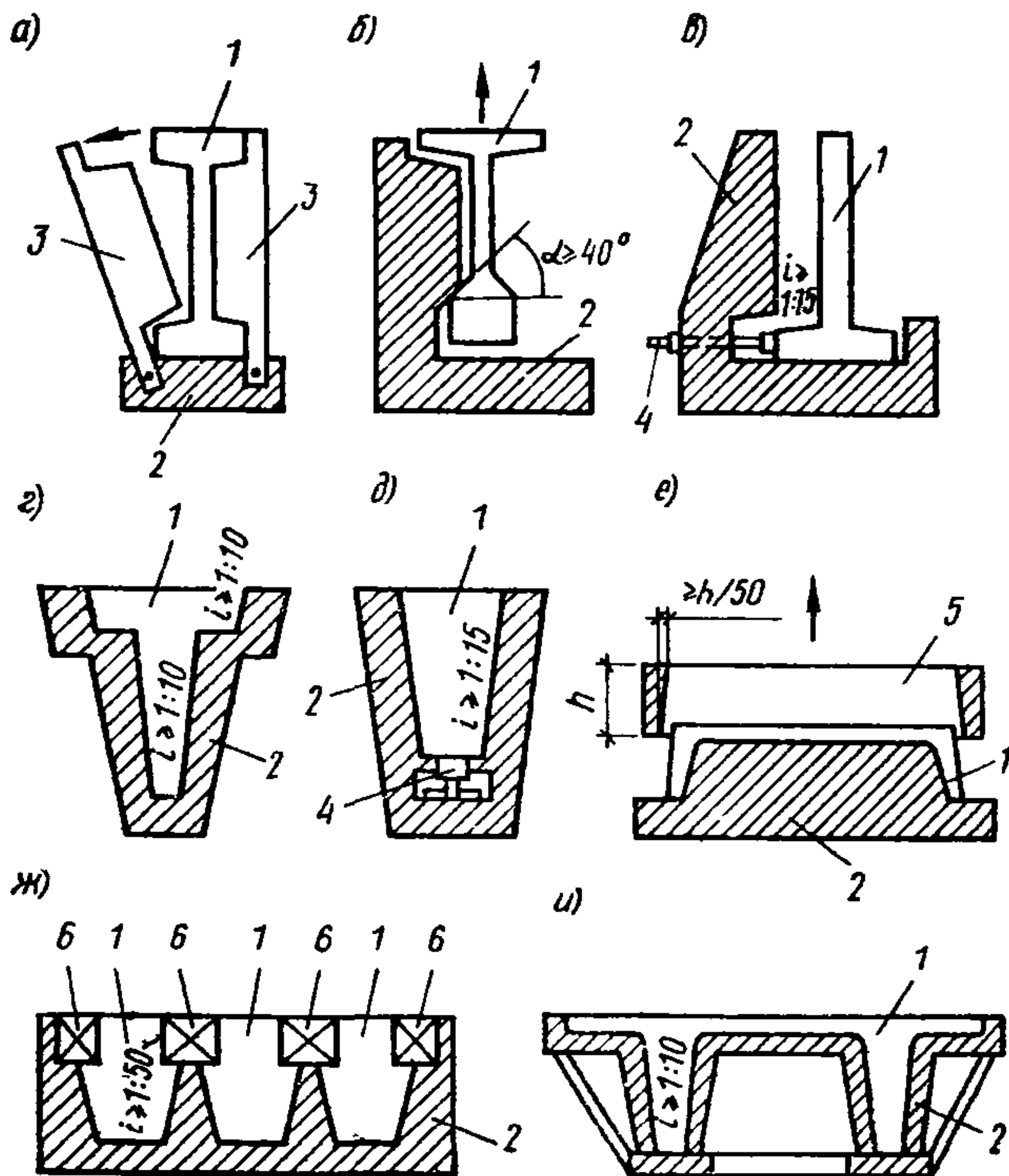
Рис. 47. Технологические уклоны в железобетонных элементах
