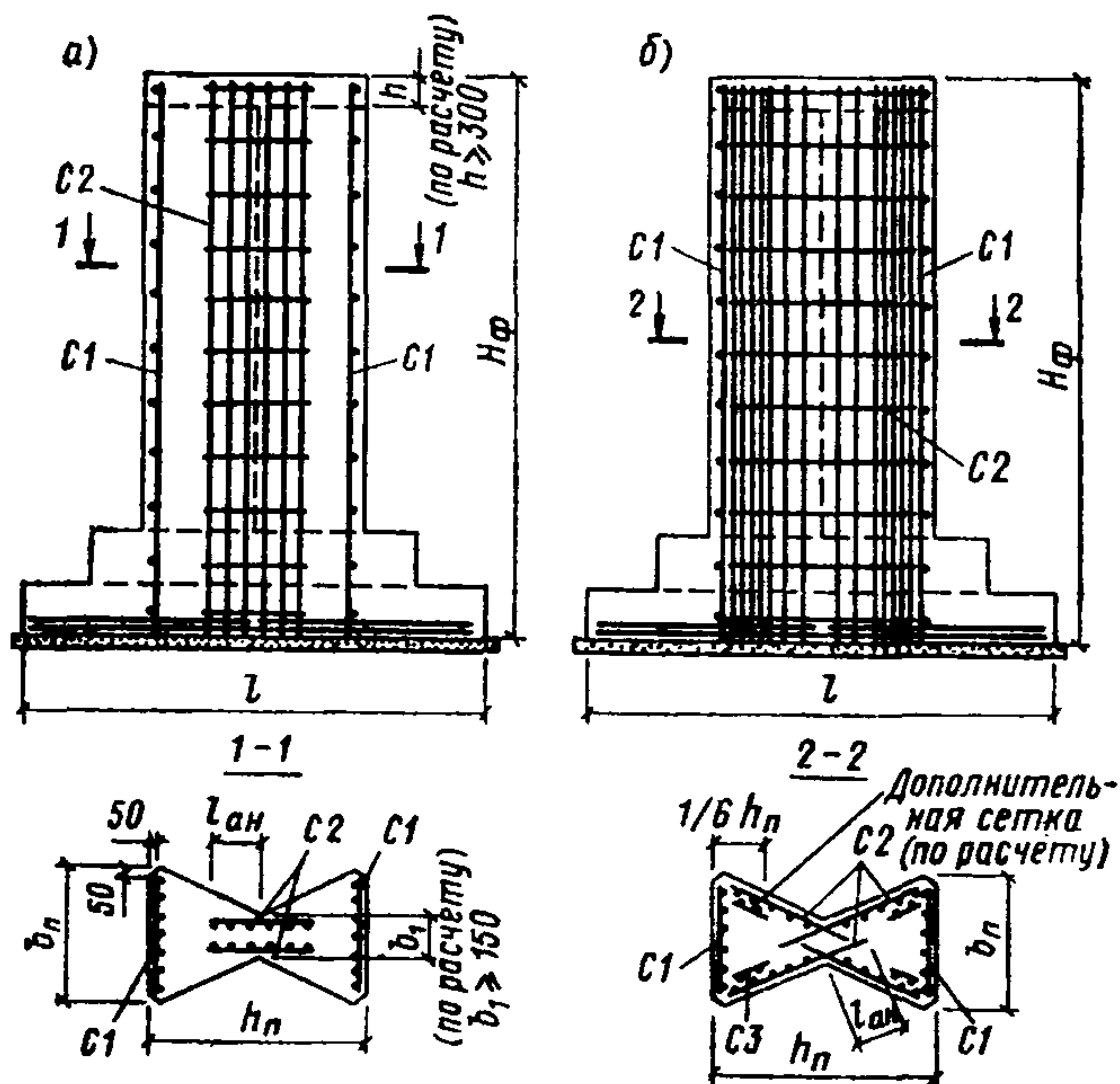
Рис. 55. Армирование подколонников X-образного сечения сварными сетками
