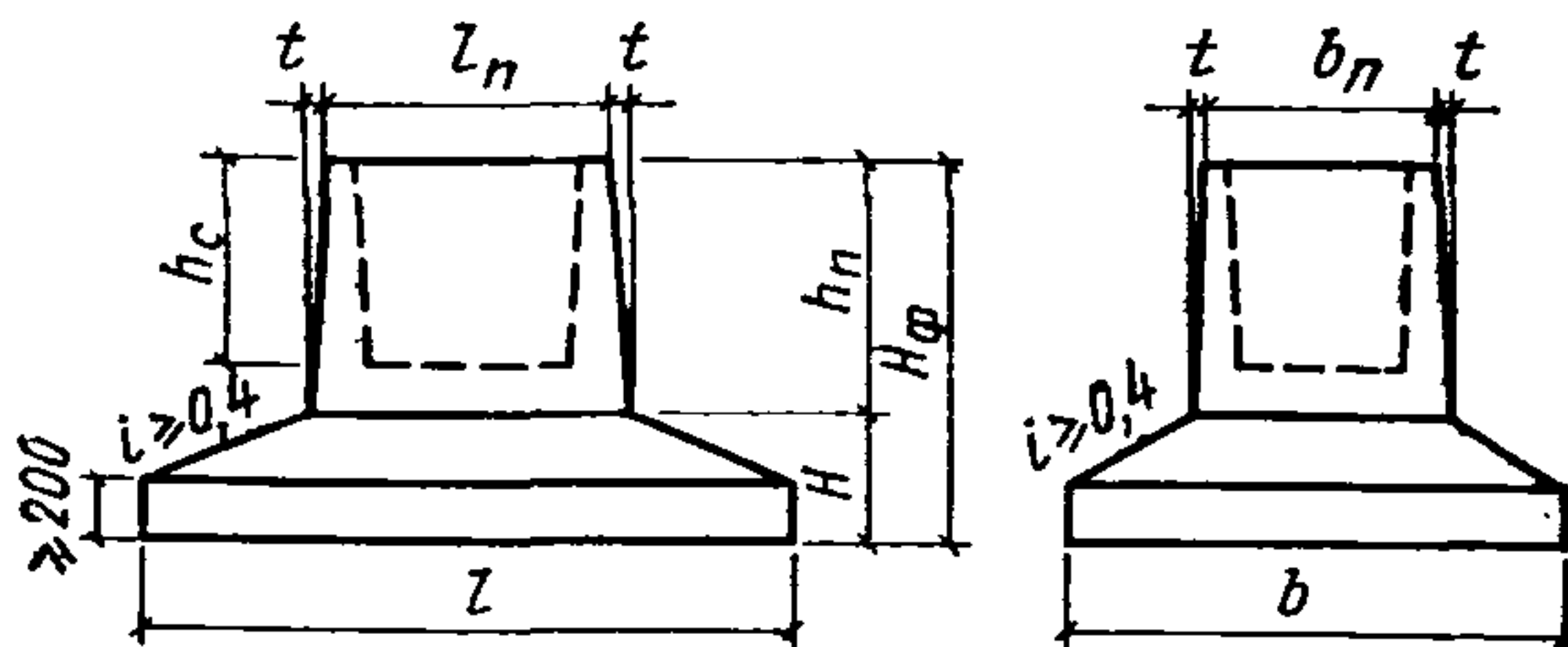
Рис. 50. Сборный железобетонный фундамент
