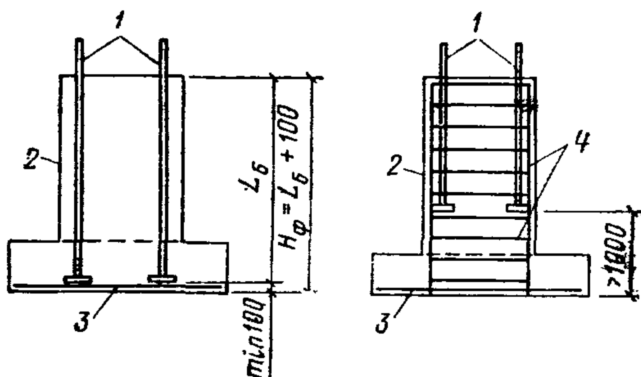
Рис. 68. Положение фундаментных болтов по высоте фундамента
