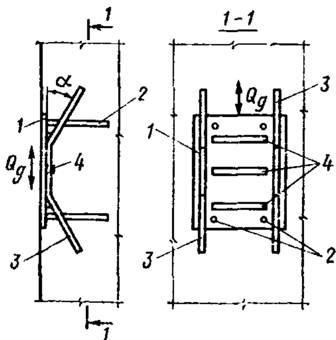
Рис. 125. Закладная деталь при сдвигающей динамической знакопеременной нагрузке
