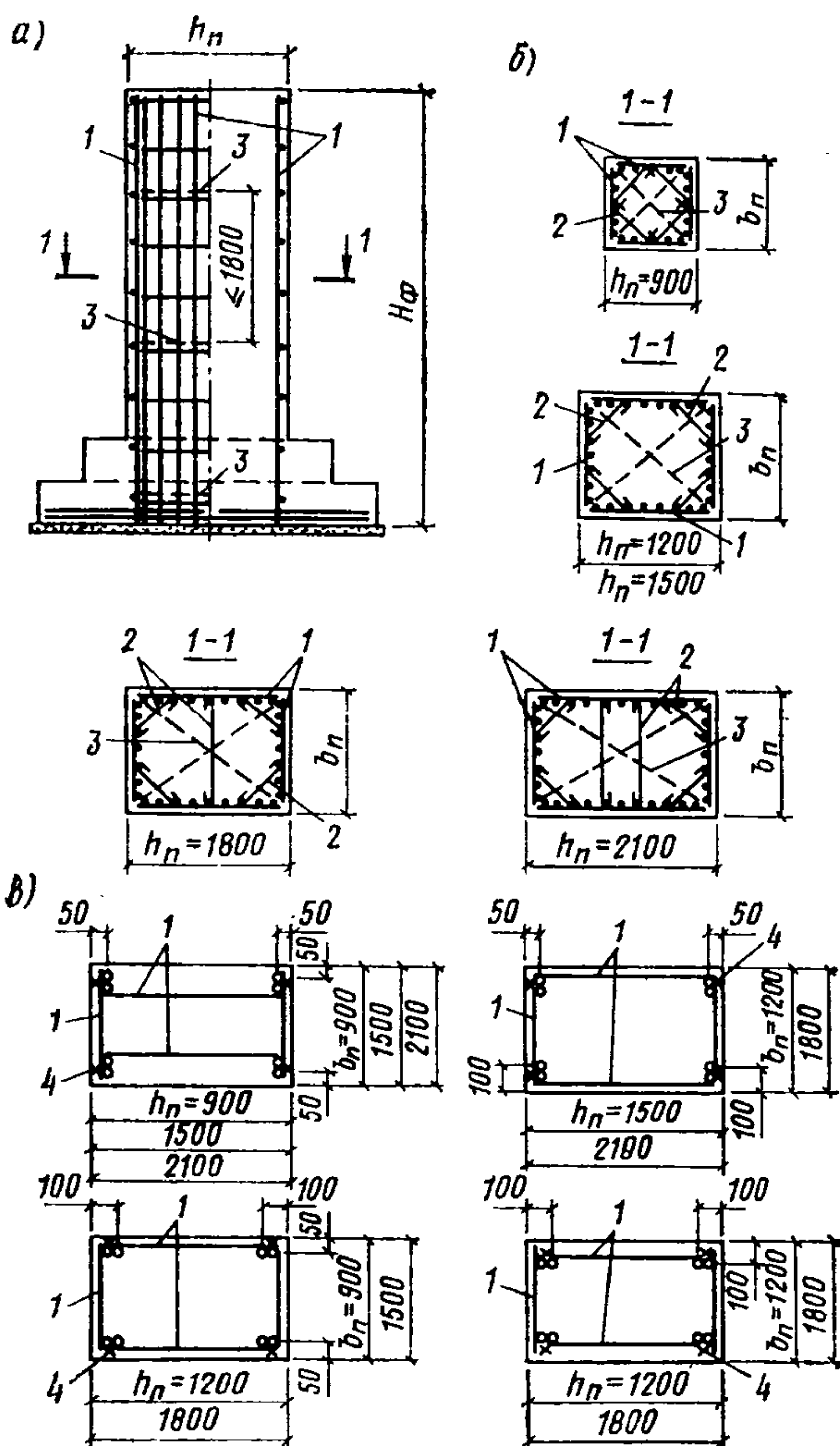
Рис. 56. Армирование подколонников самонесущими каркасами, собираемыми из сеток
