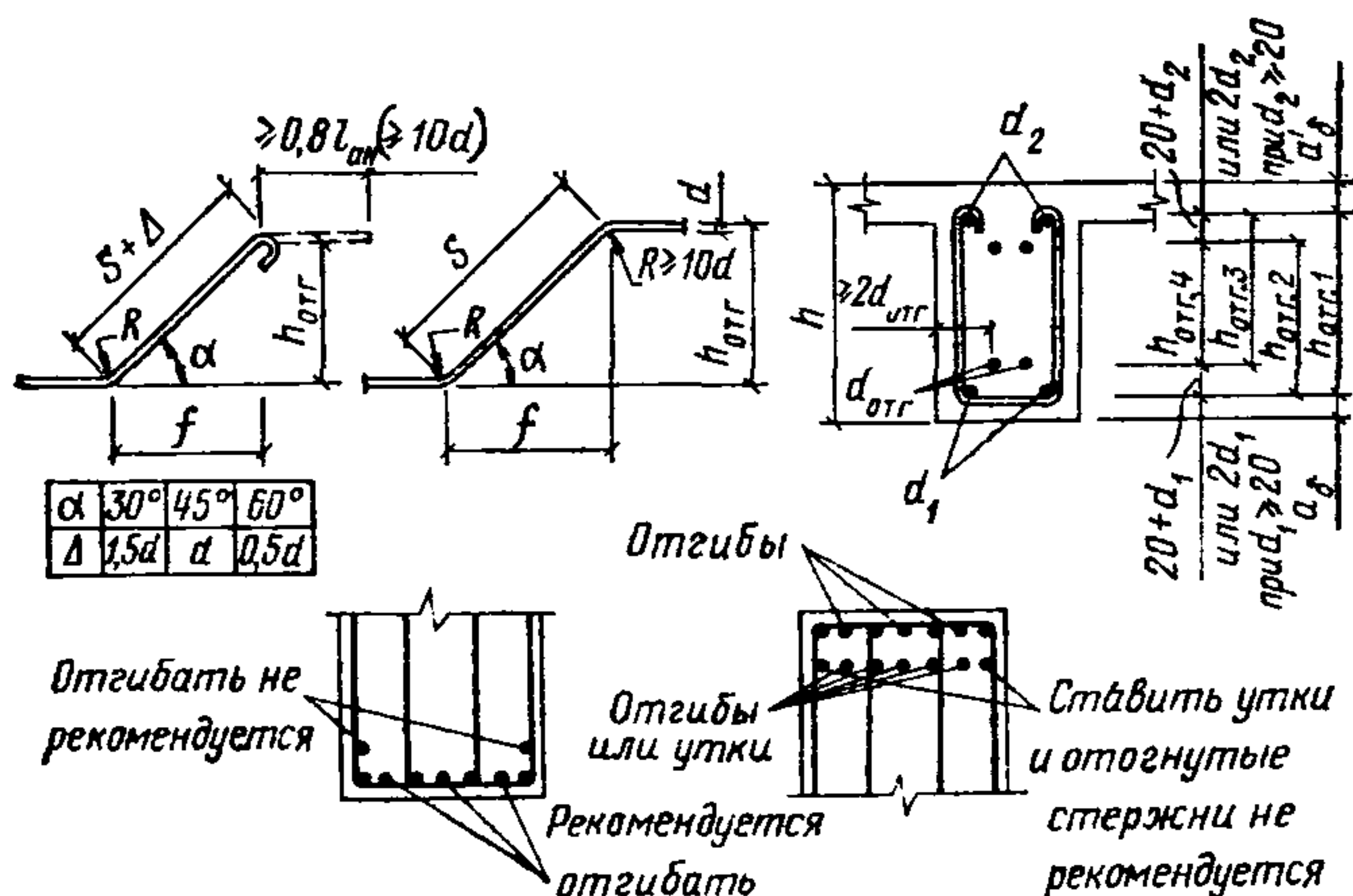
Рис. 91. Конструирование отогнутых стержней
