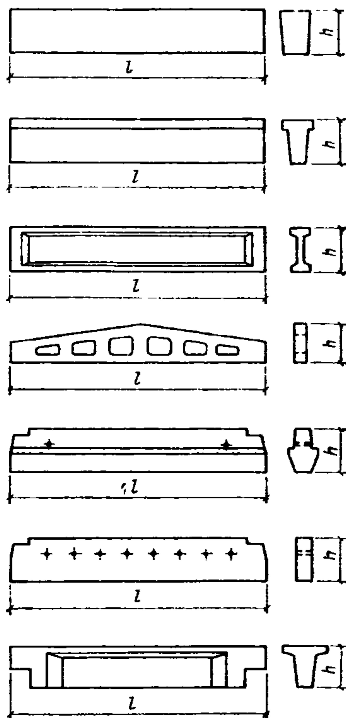
Рис. 83. Примеры конструкций сборных железобетонных балок
