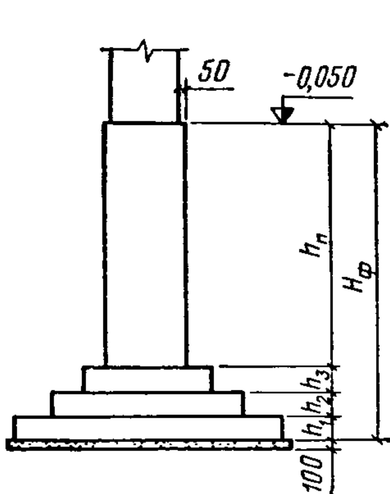
Рис. 61. Фундамент монолитной железобетонной колонны
