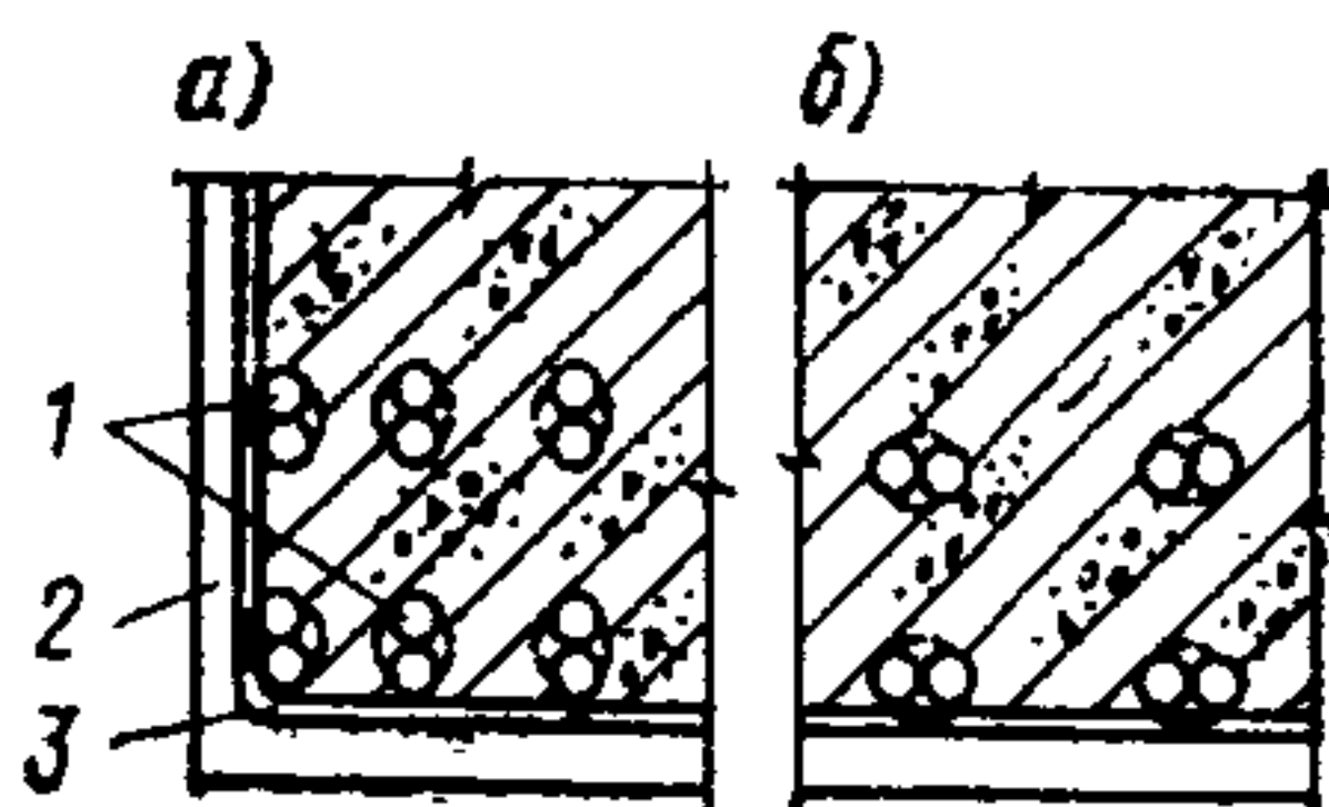
Рис. 4. Групповое расположение стержней
