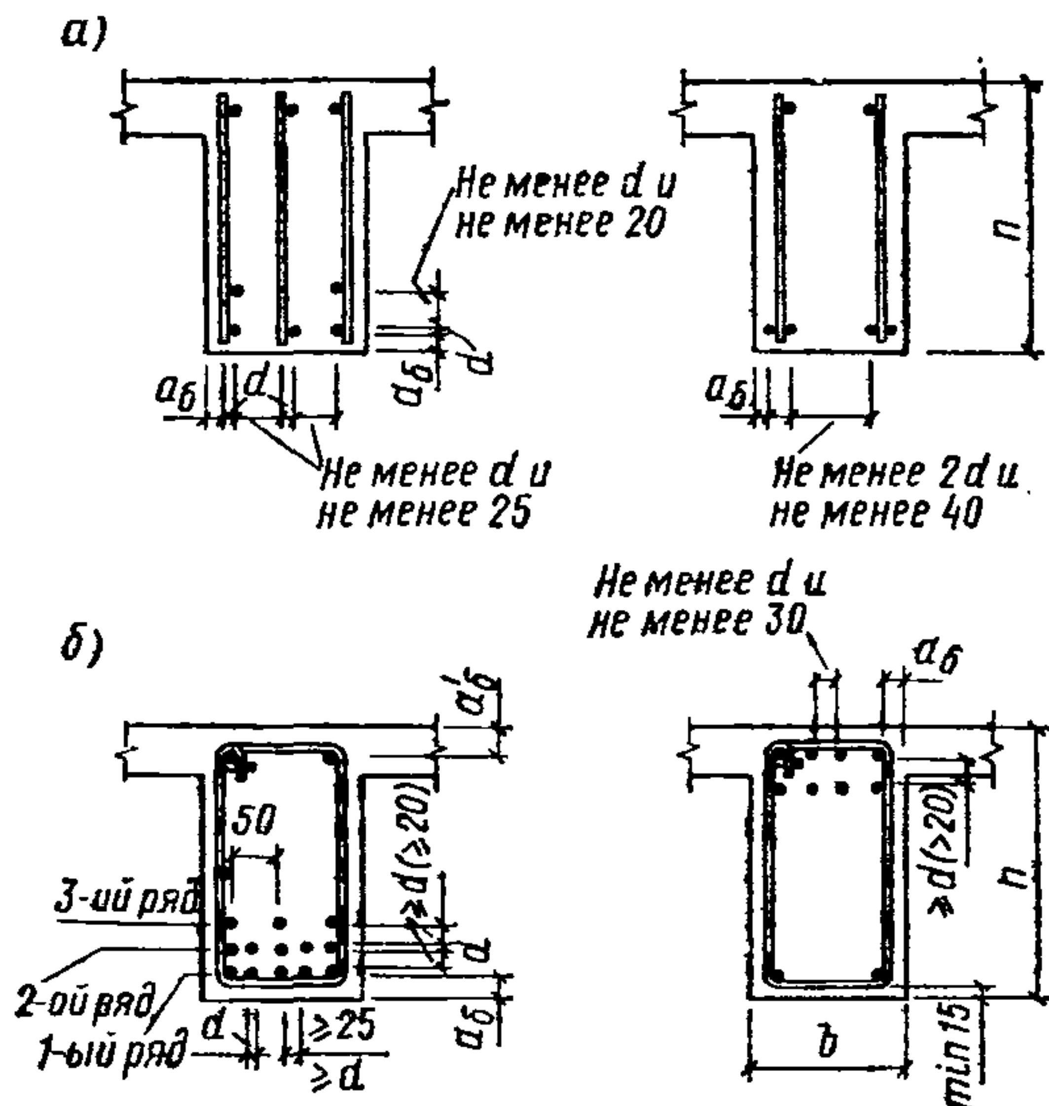
Рис. 84. Расположение продольной арматуры в поперечном сечении балки
