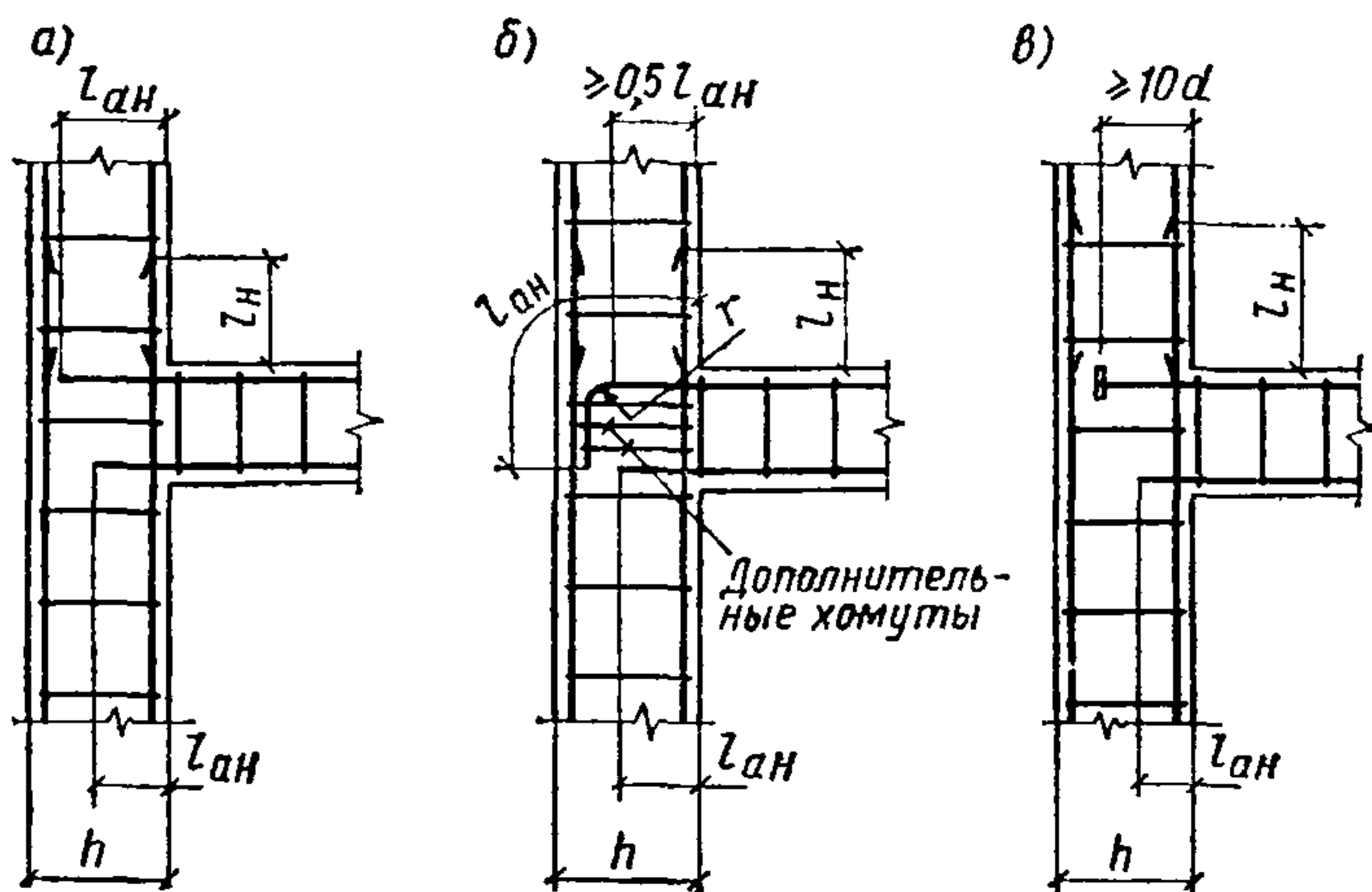
Рис. 94. Армирование сопряжения промежуточного ригеля со стойкой
