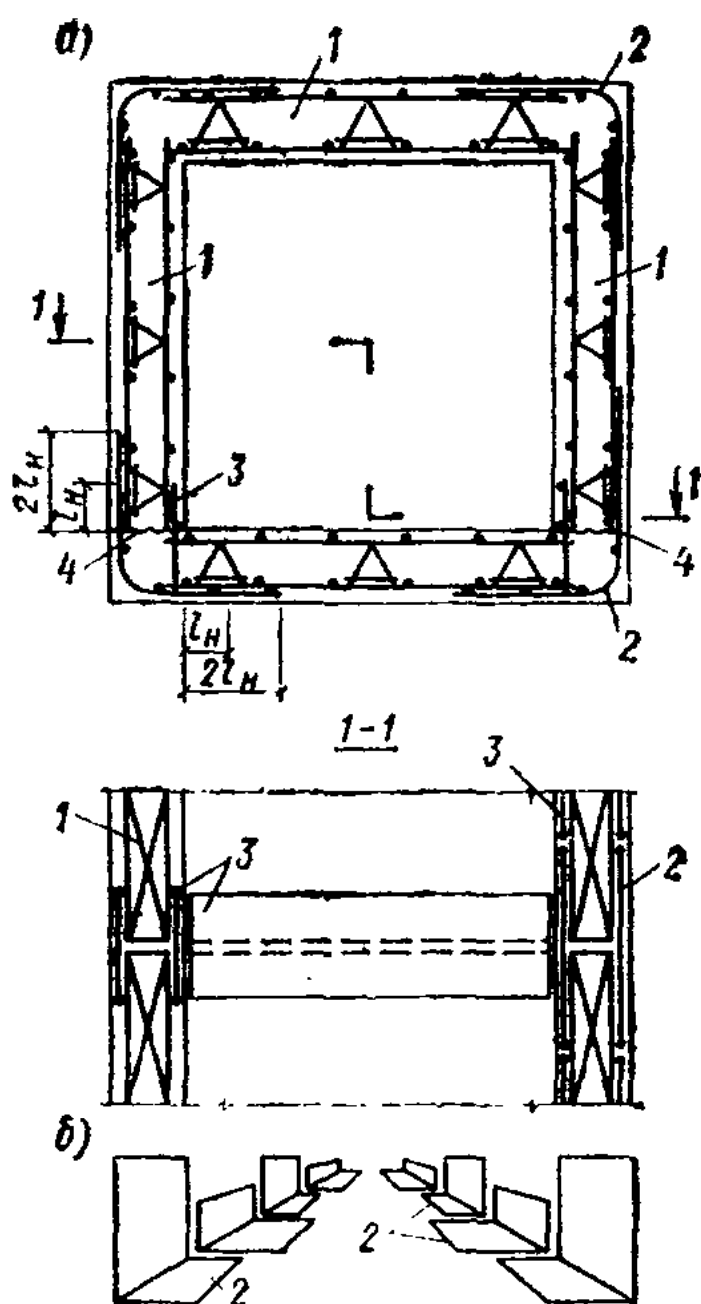
Рис. 121. Схема армирования тоннеля самонесущими арматурными блоками
