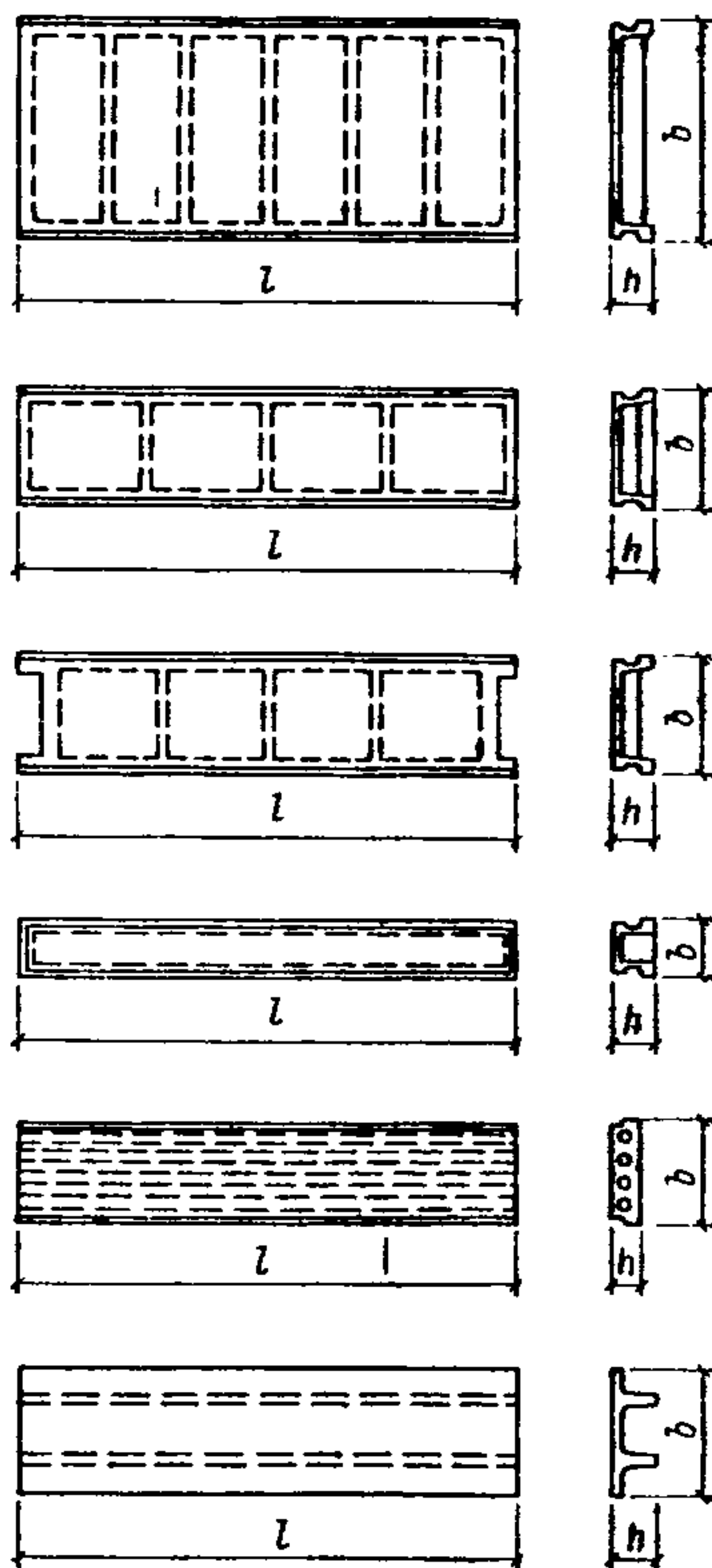
Рис. 96. Примеры конструкций сборных плит
