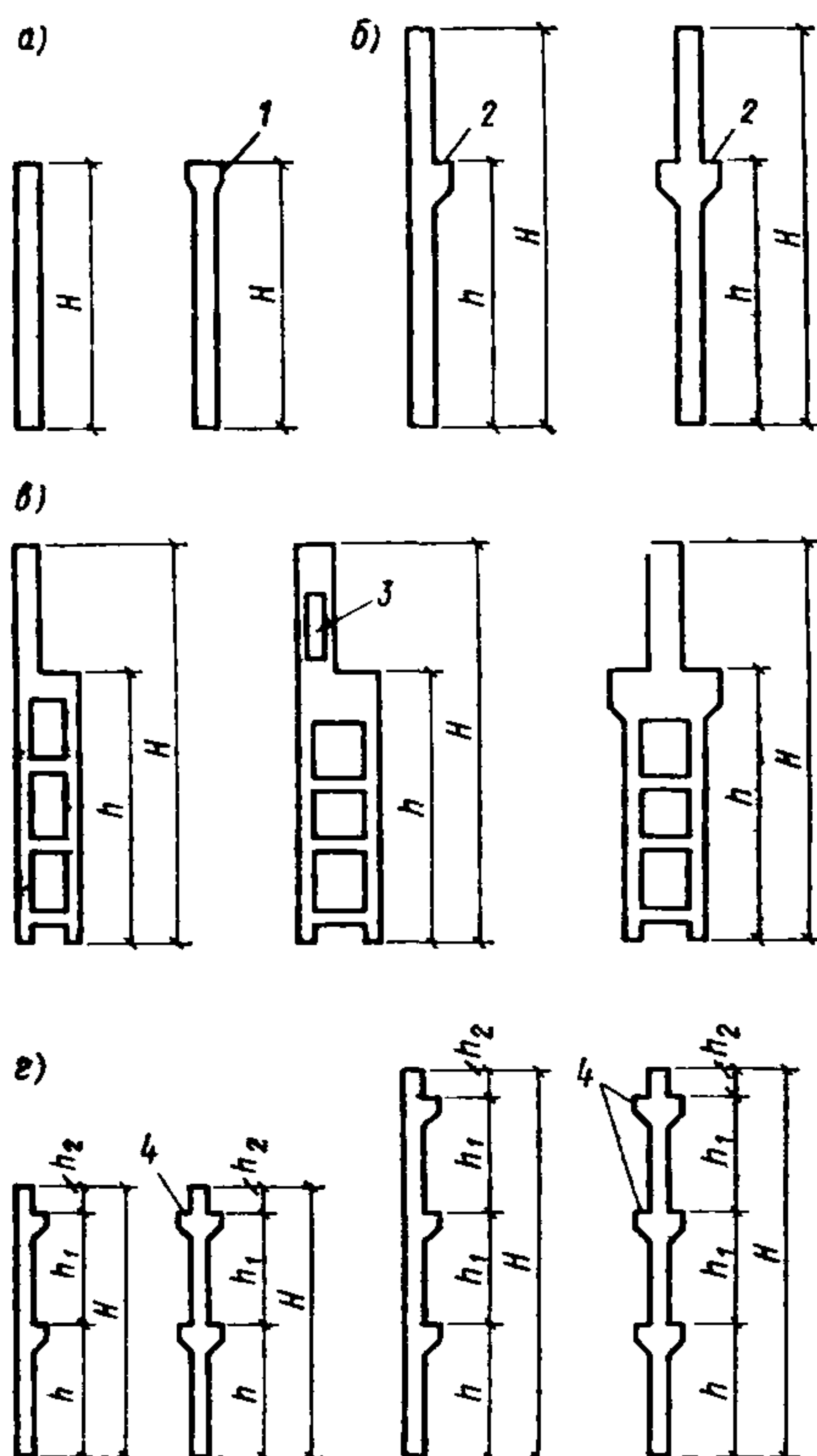
Рис. 70. Типы сборных колонн
