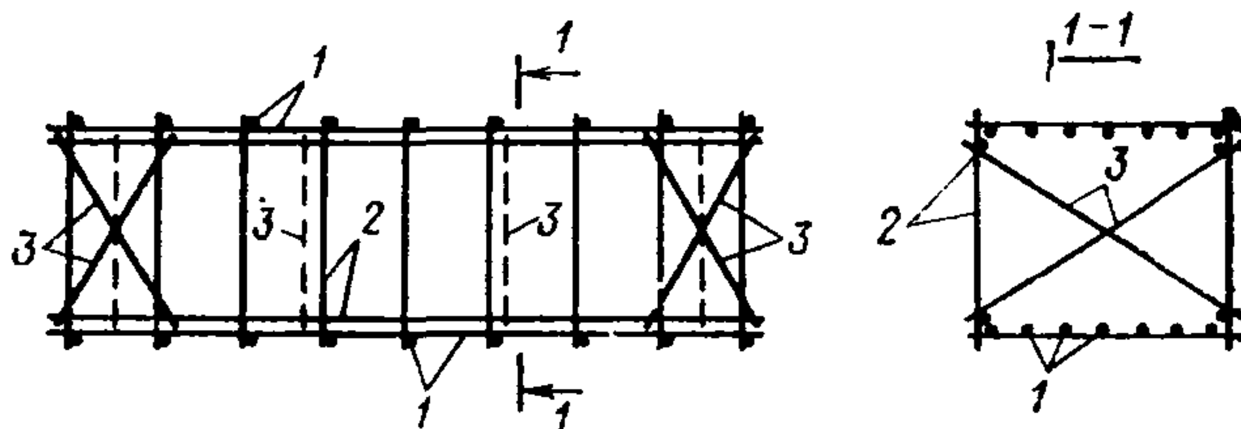
Рис. 21. Пример арматурного каркаса толстой железобетонной плиты
