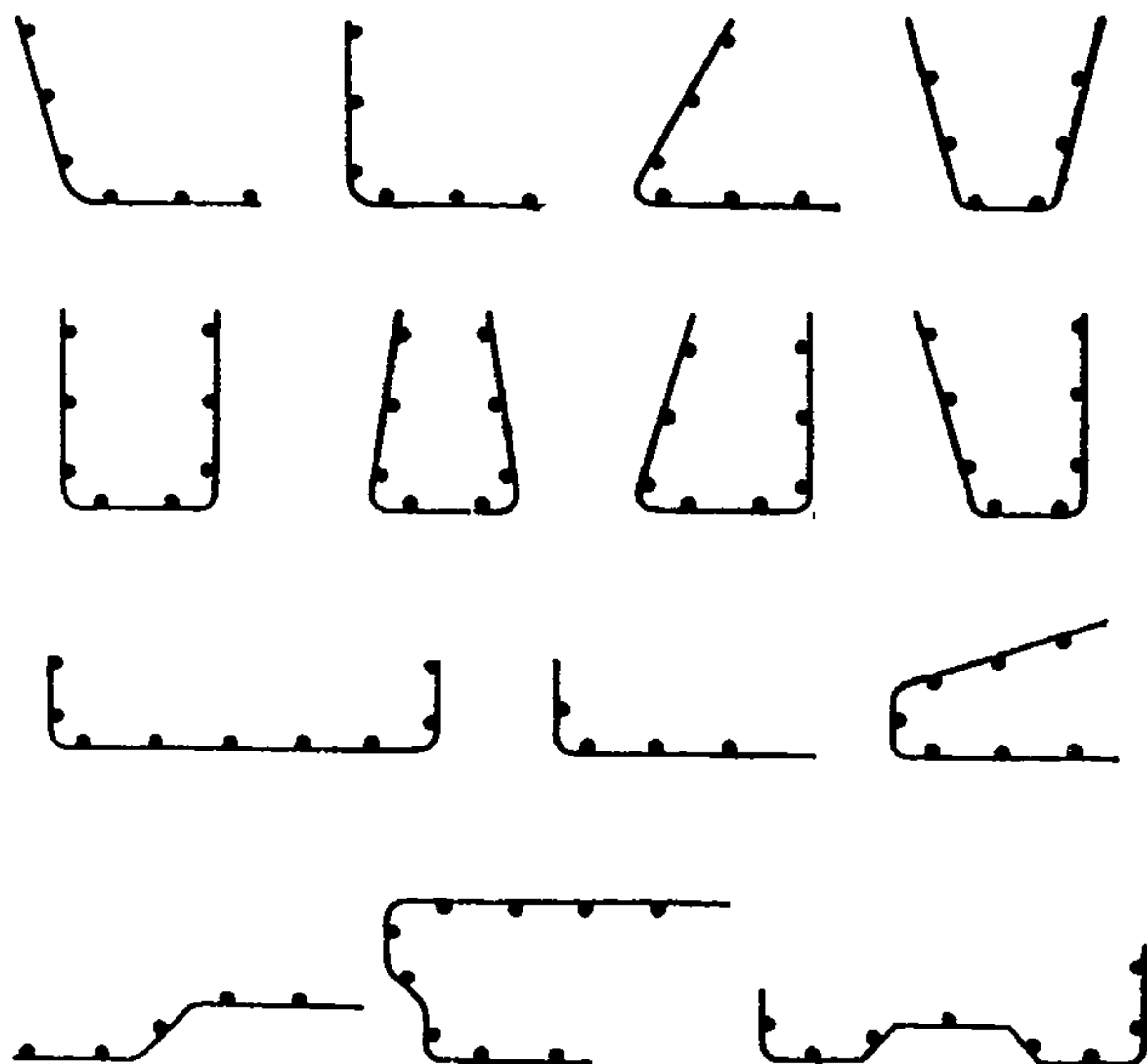
Рис. 7. Рекомендуемые очертания гнутых сеток
