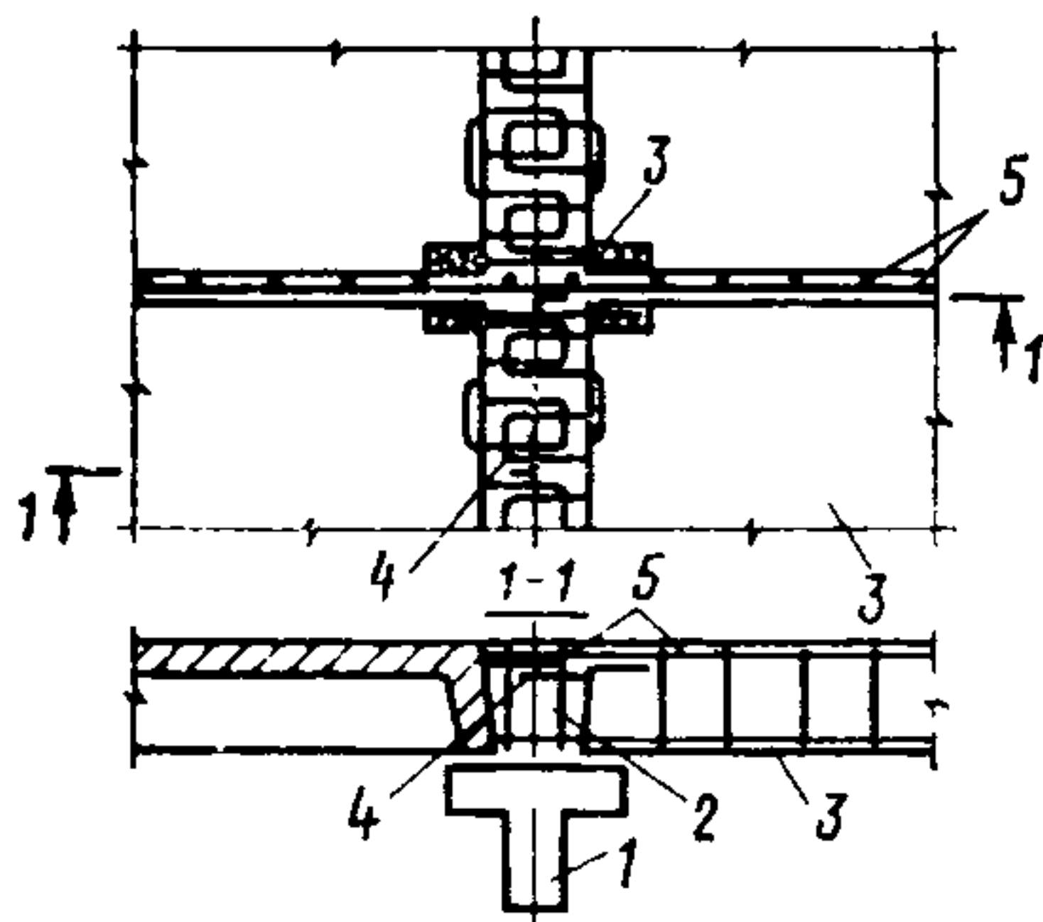
Рис. 113. Сопряжение плит
