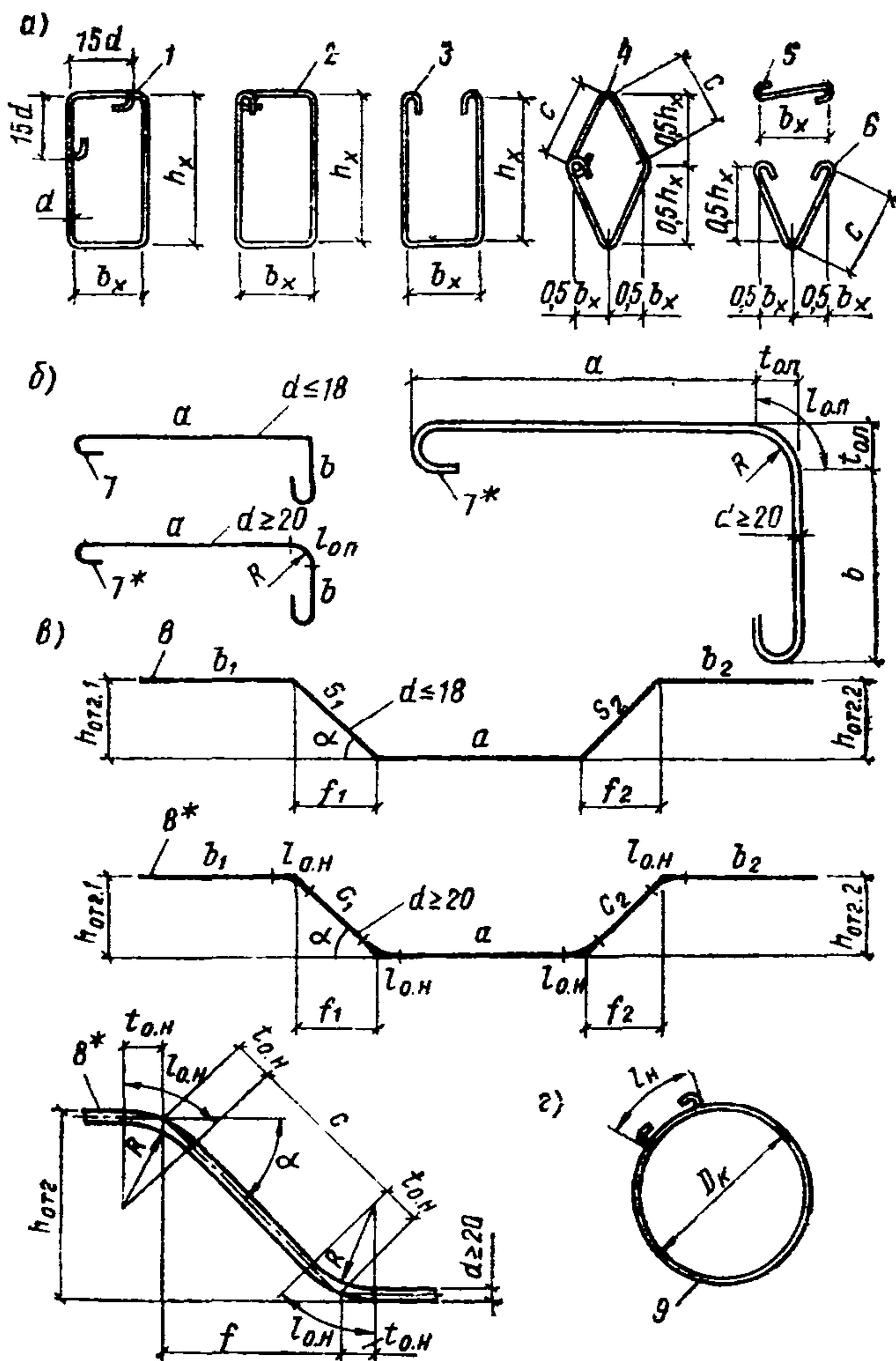
Рис. 1. Гнутые арматурные стержни
