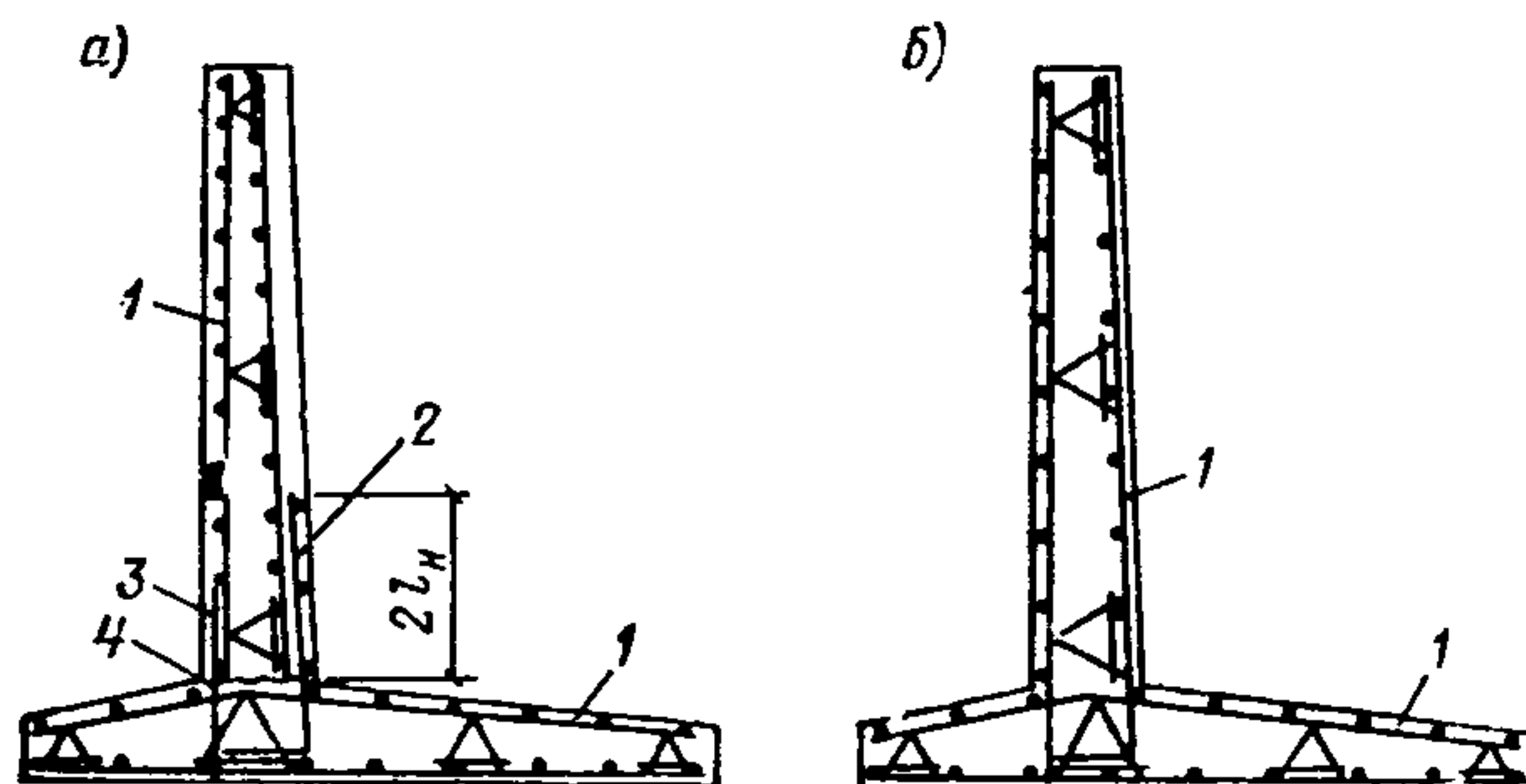
Рис. 118. Схема армирования подпорных стен самонесущими арматурными блоками
