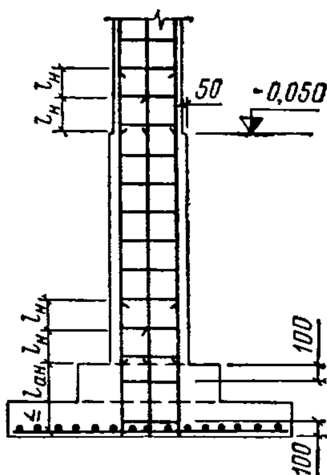
Рис. 62. Армирование фундамента монолитной колонны
