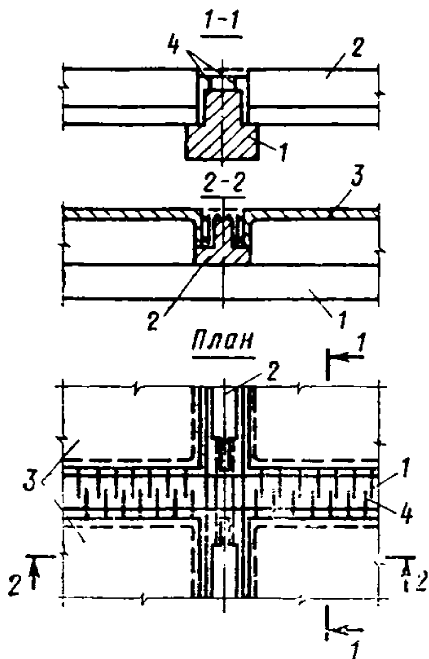
Рис. 112. Сопряжение балок и плит
