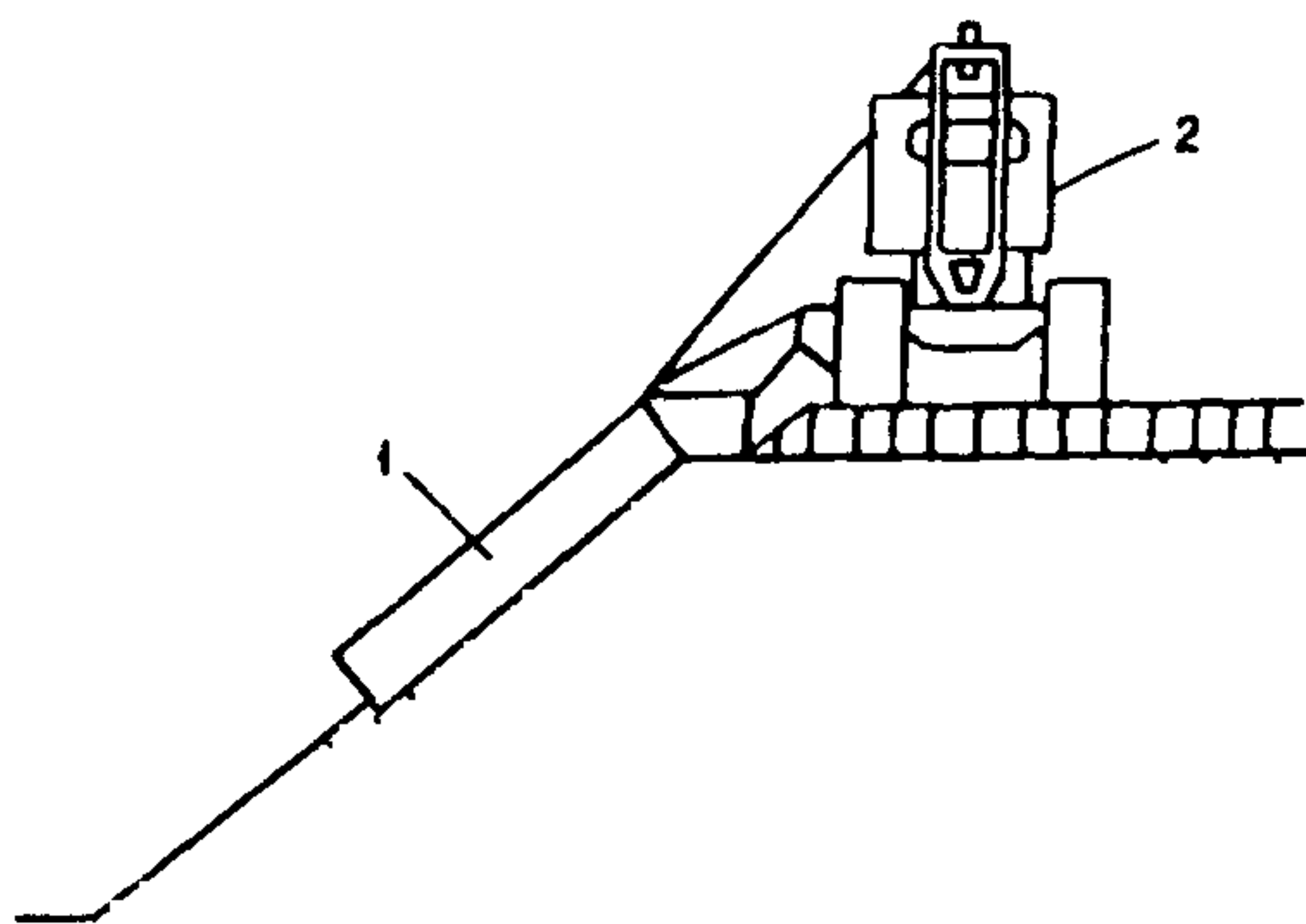
Рис.7. Схема расположения навесного откосопланировщика при укреплении откосов: 1–откосник; 2–трактор
