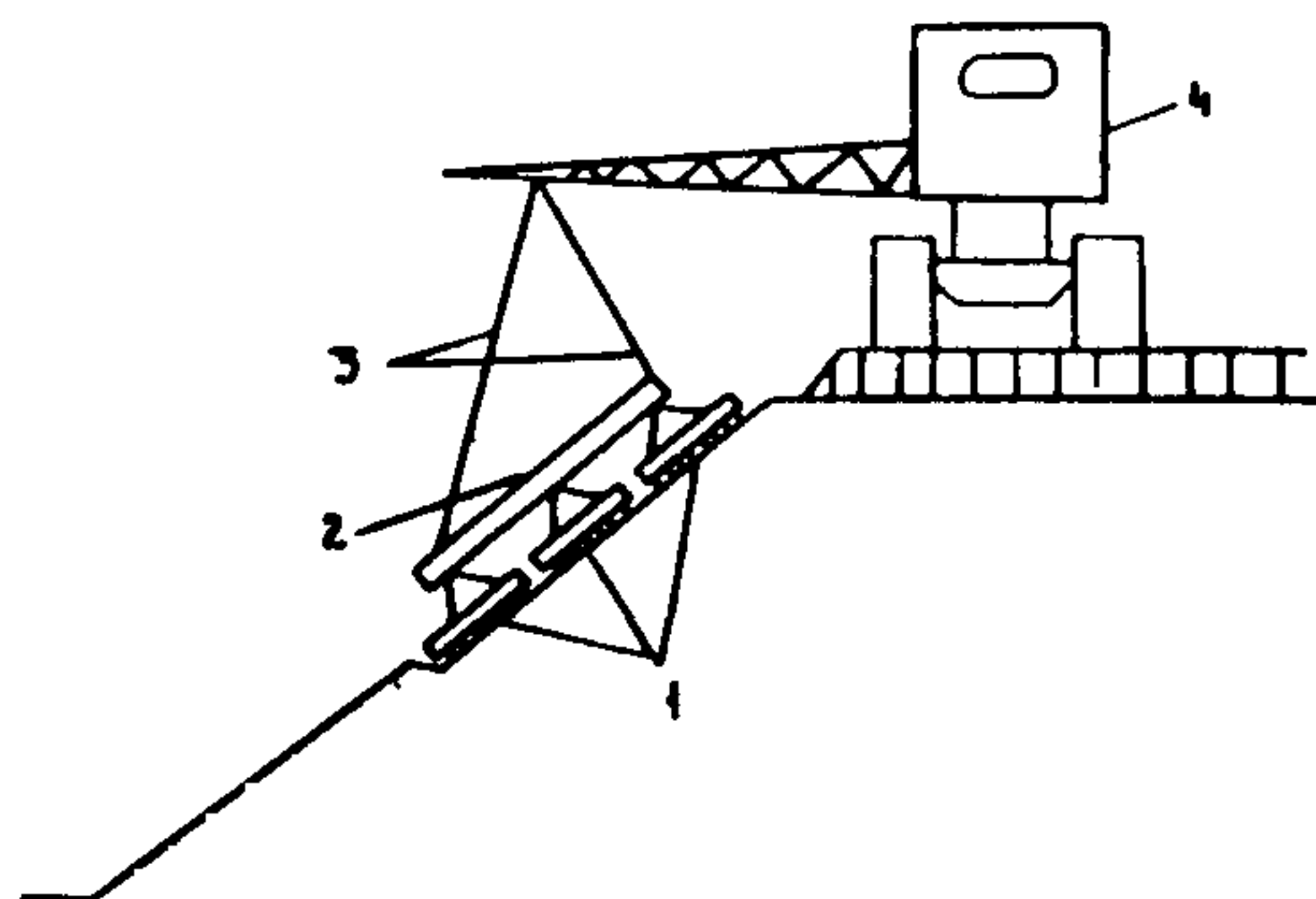
Рис.8. Схема установки комплекта борон: 1-борона; 2-траверса; 3-тросы; 4-трактор
