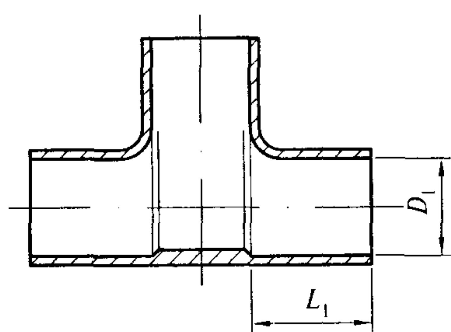
Рисунок Д.5 — Тройник равнопроходный
