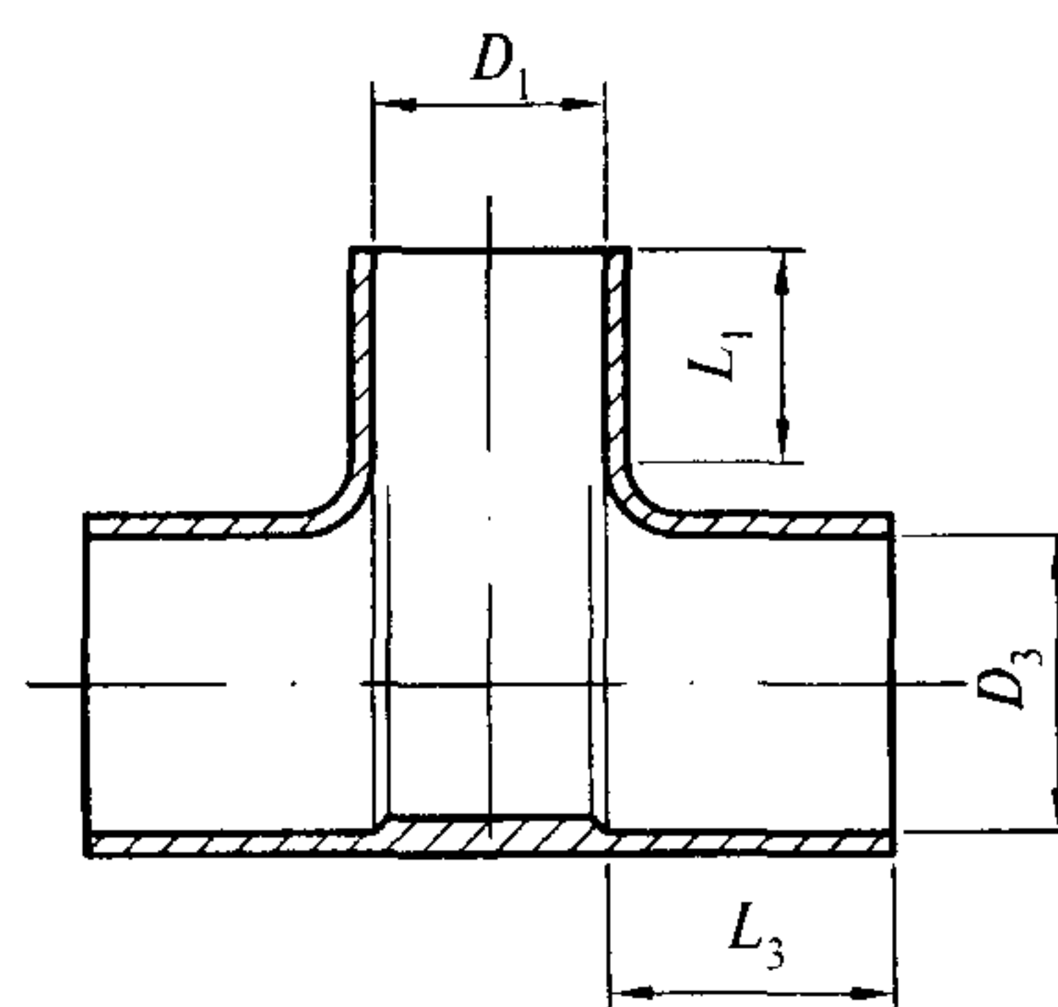
Рисунок Д.6 — Тройник переходный
