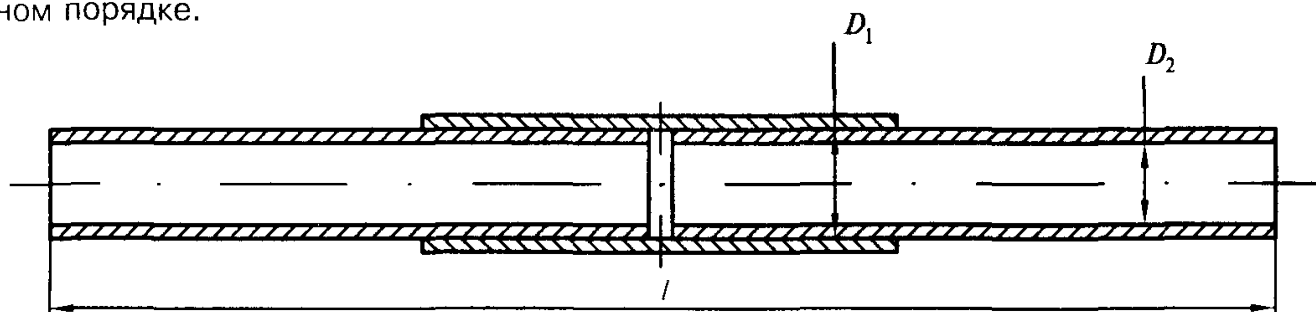
Рисунок 8 — Допускное соединение
