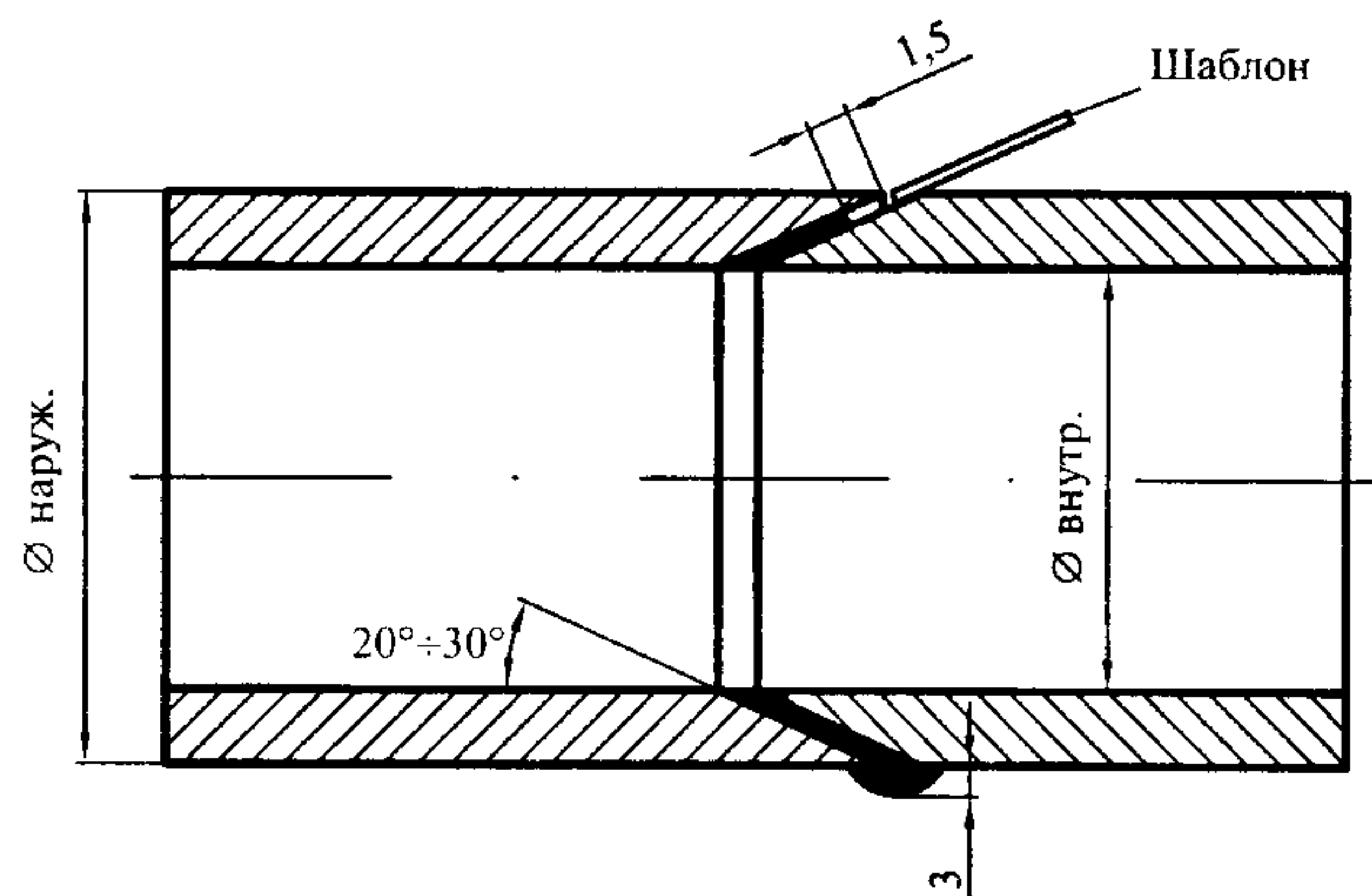
Рисунок 11 — Паяное соединение стальных труб
