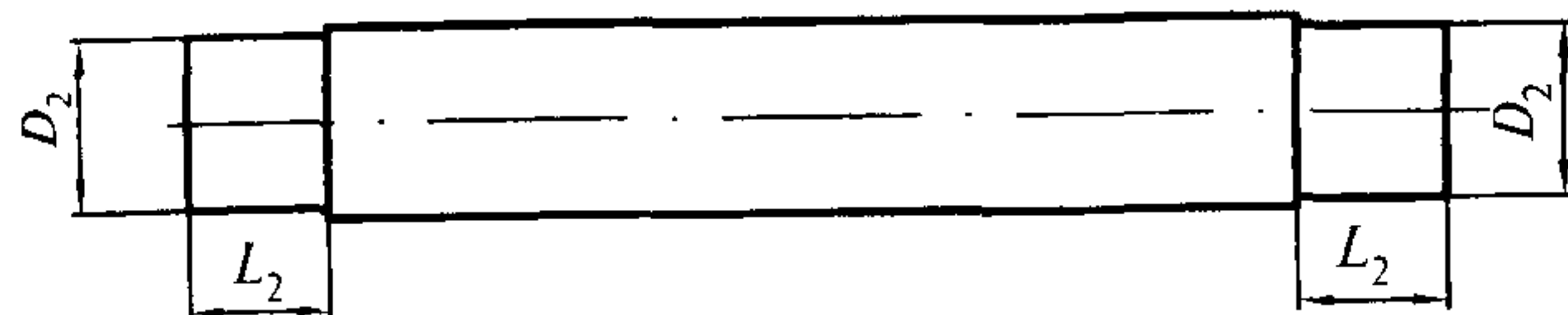
Рисунок 15 — Схема калибровки медных труб перед монтажом
