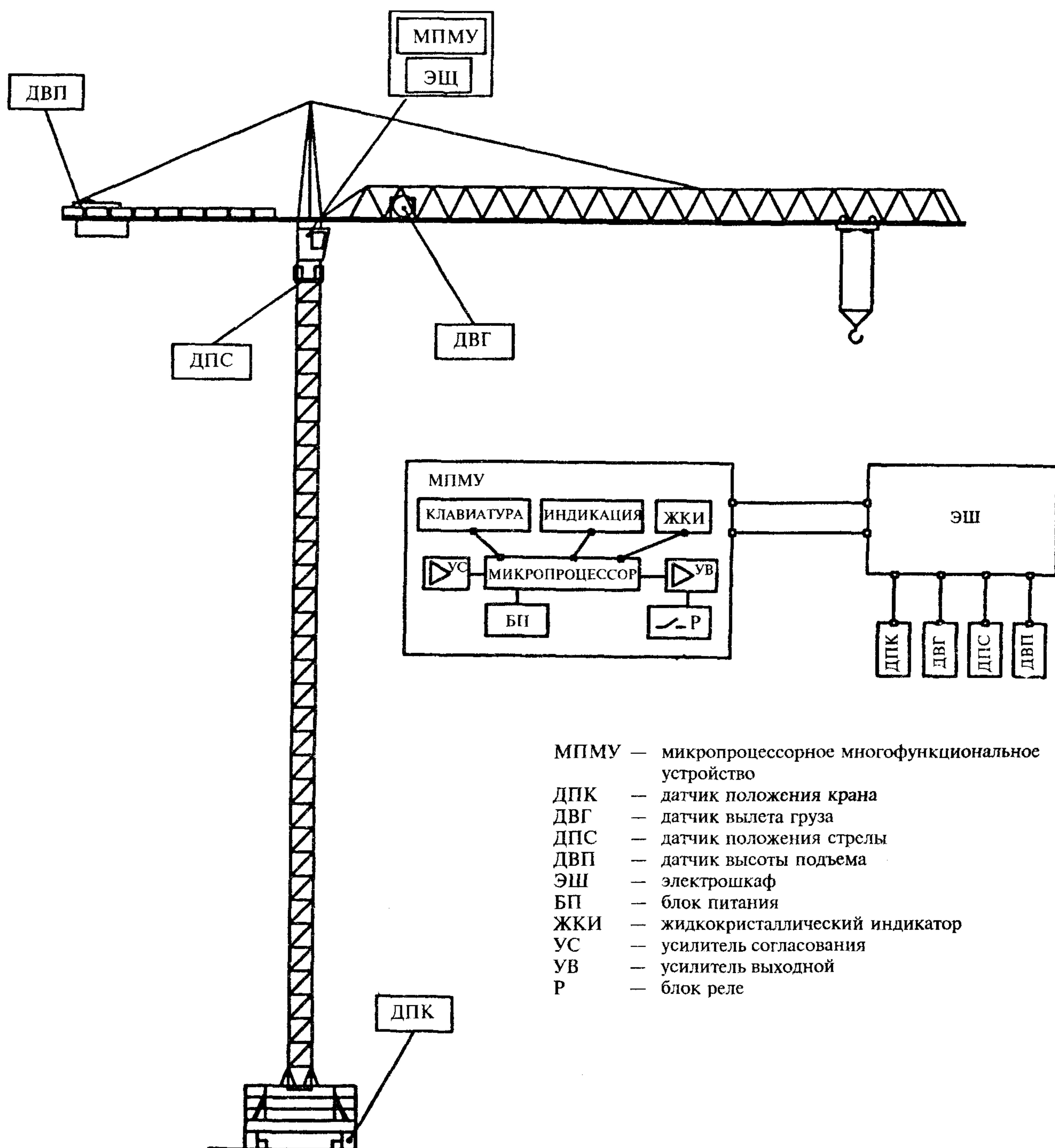
Рисунок 2 — Расположение датчиков на кране
