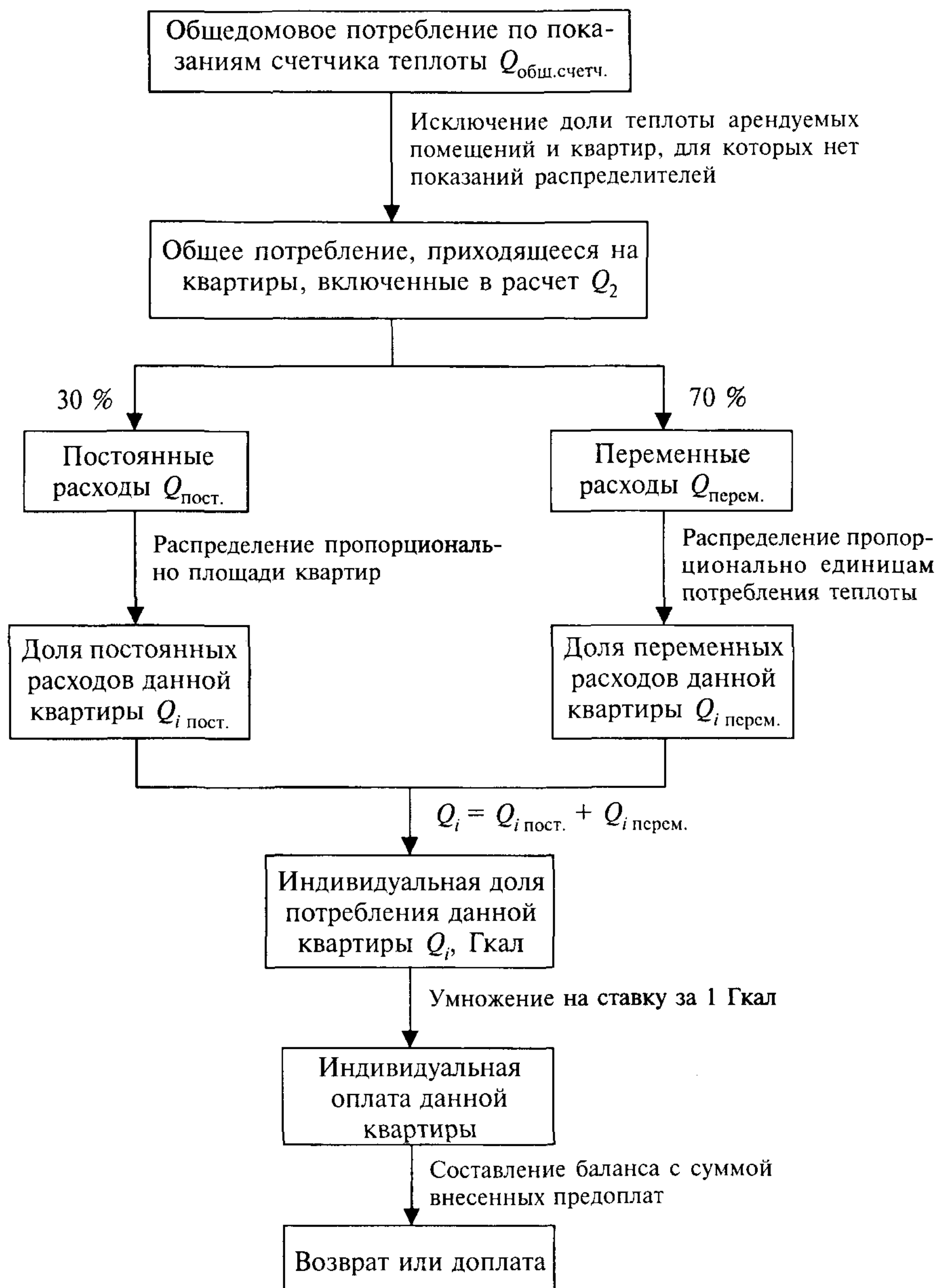
Рис.1. Обобщенная схема распределения общедомовых затрат тепловой энергии
