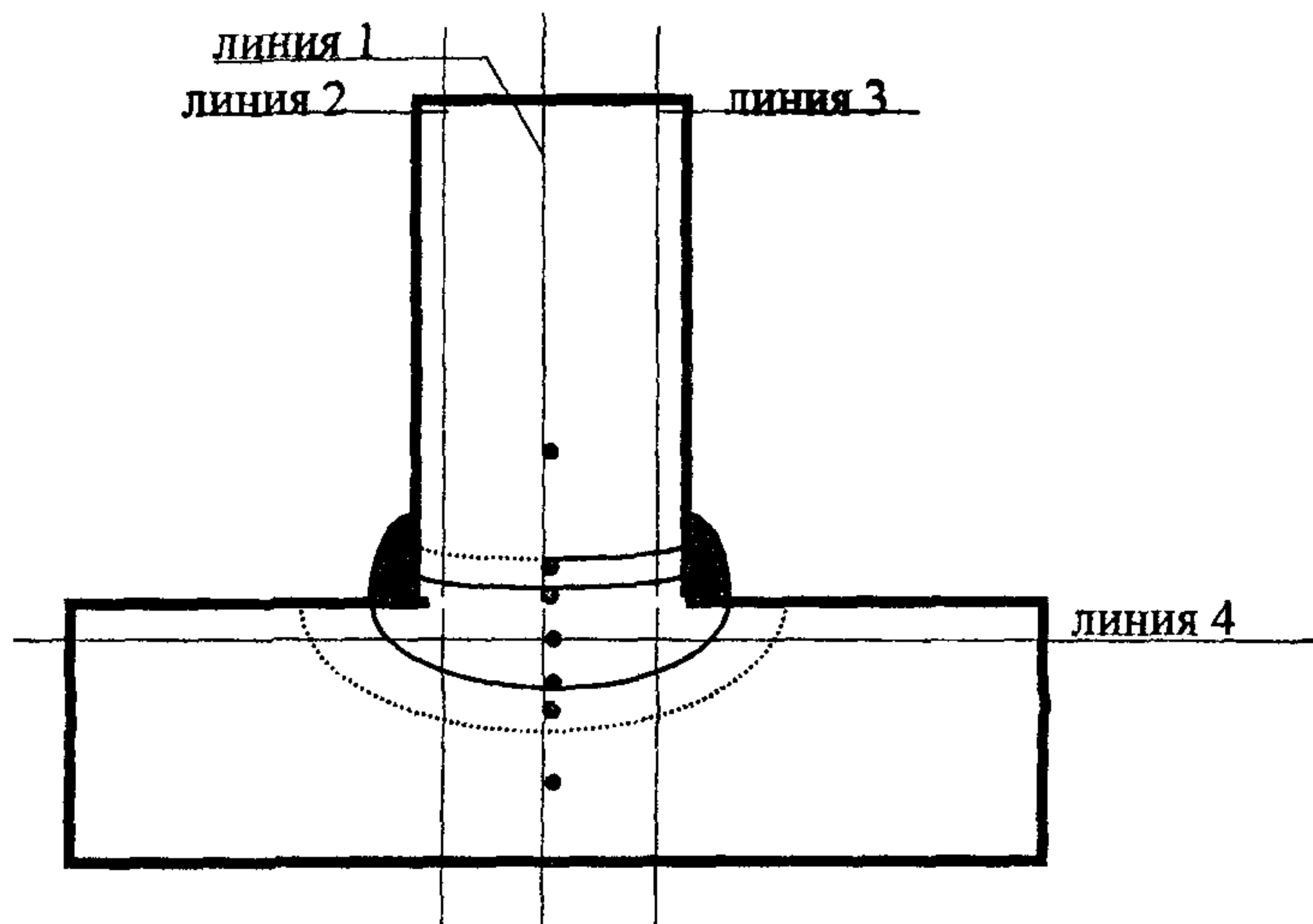
Рис. Б.5. Измерения твёрдости упора
