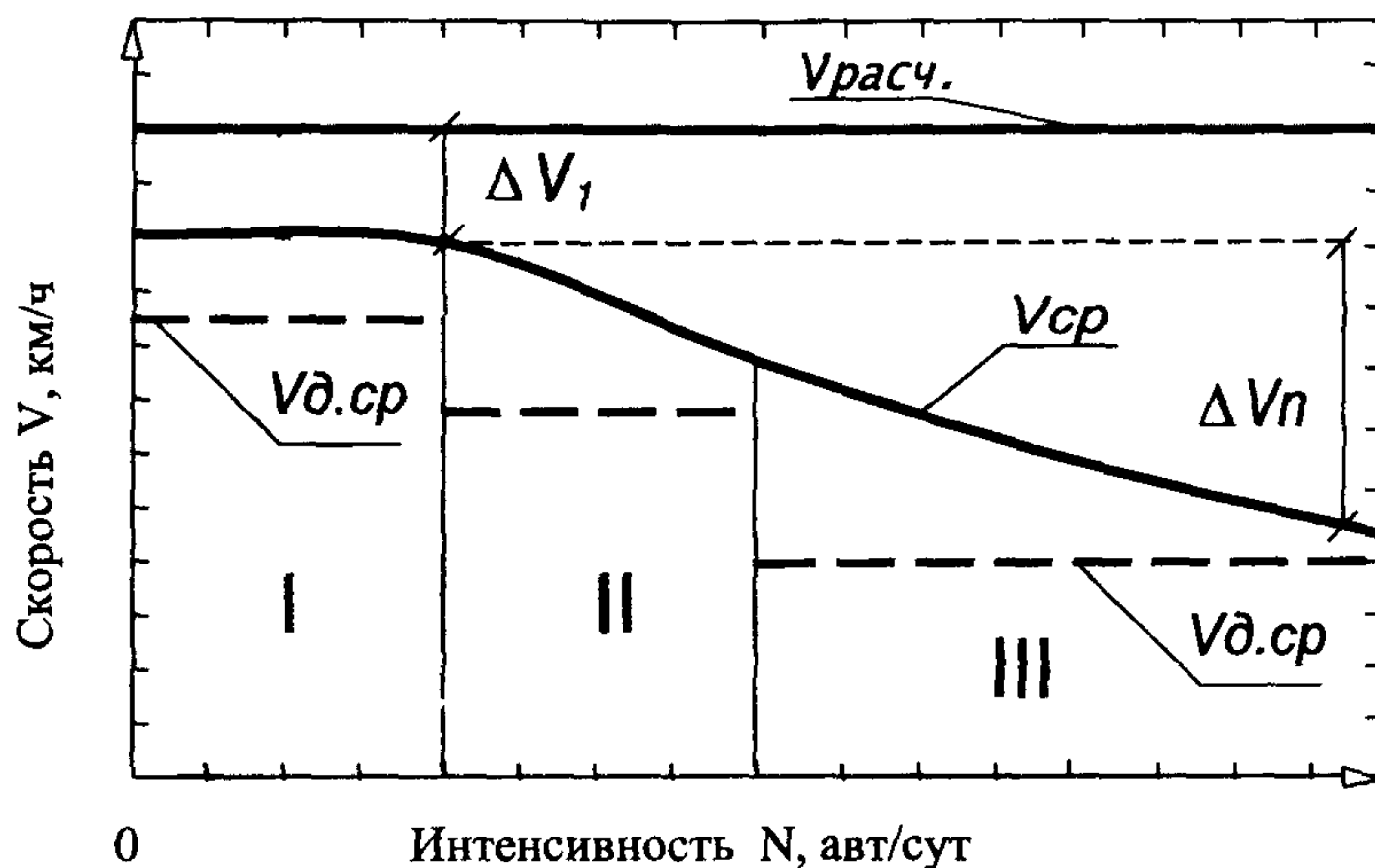
Рис. 2. Связь между средней скоростью транспортного потока и интенсивностью движения:
