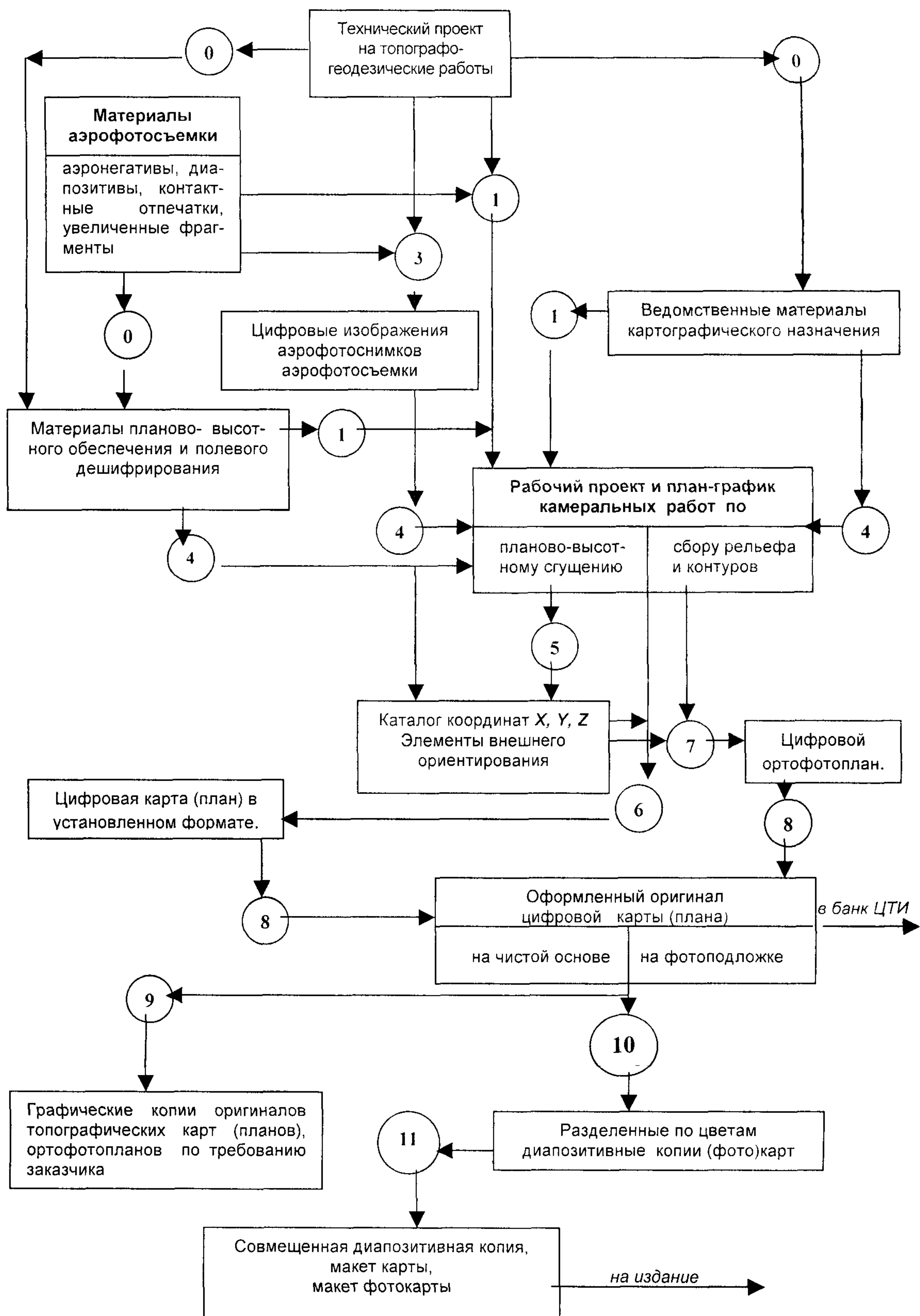
Рис. 2. Технологическая схема камеральных работ при создании цифровых топокарт и планов в масштабах 1:500 - 1:25 000 на цифровых фотограмметрических приборах по стереоснимкам
