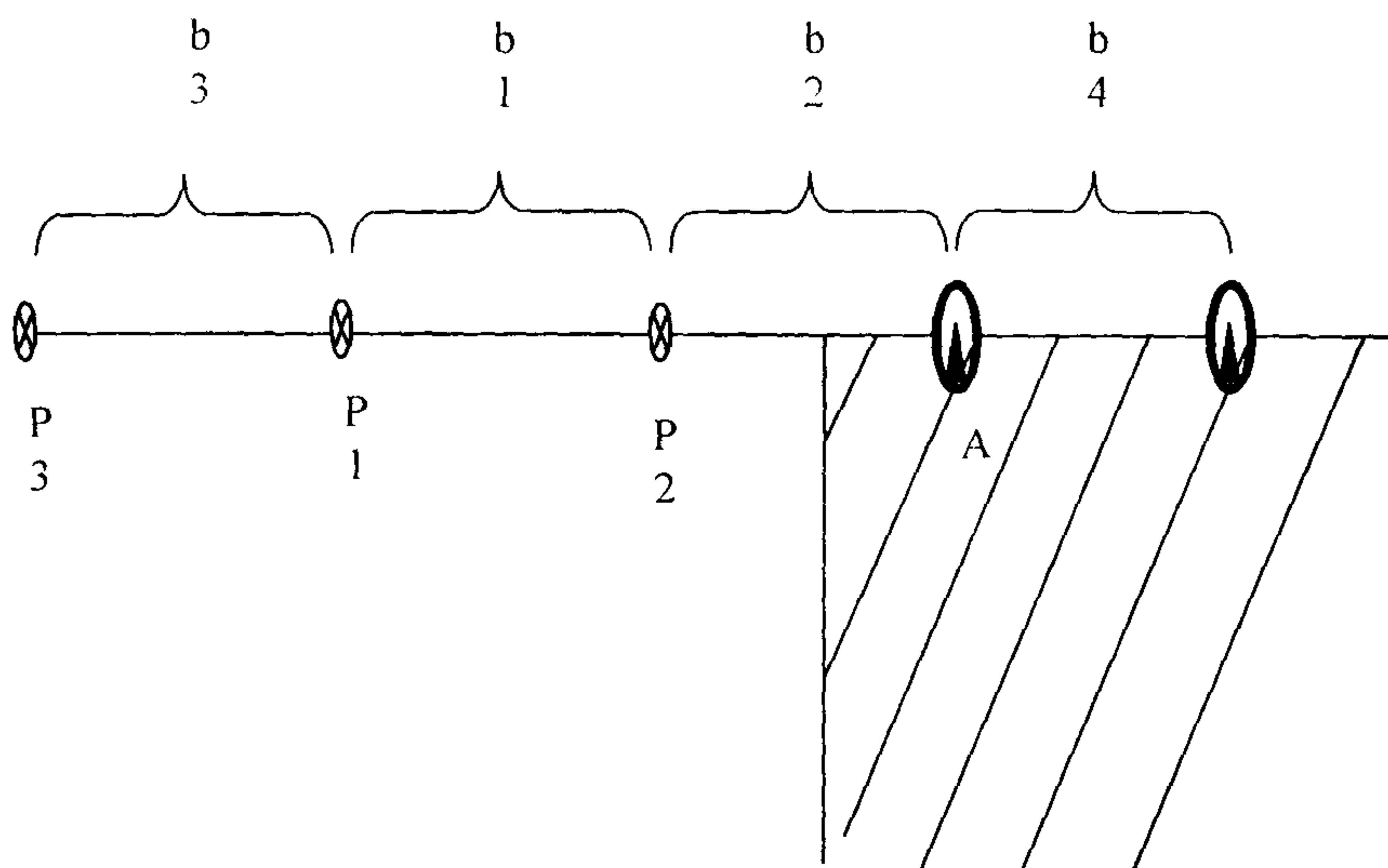
Рис.3. Схема определения пространственных координат стенных пунктов наземной сети по спутниковым наблюдениям на вспомогательных точках одного створа.
