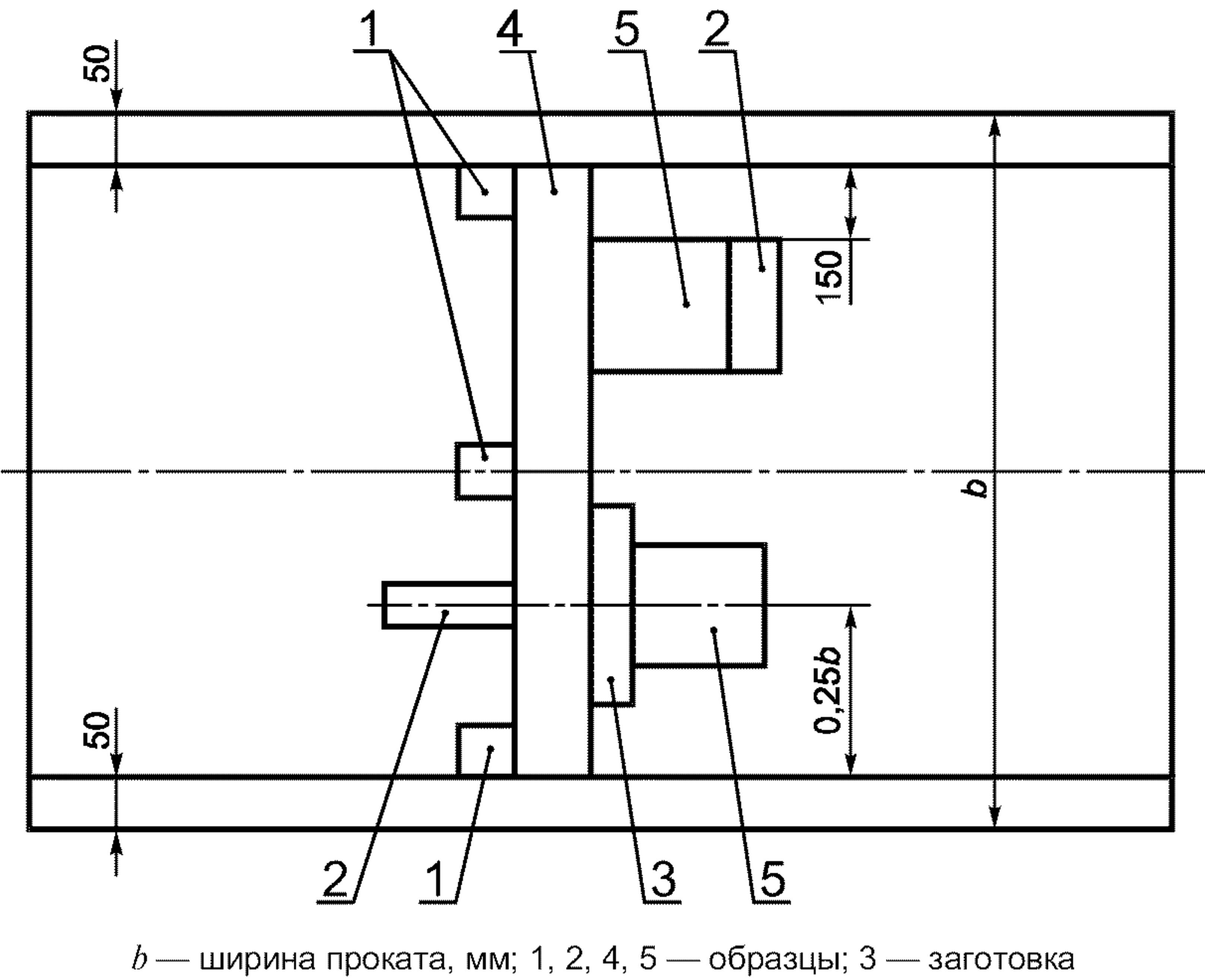
Рисунок 1 — Схема вырезки заготовок и образцов
