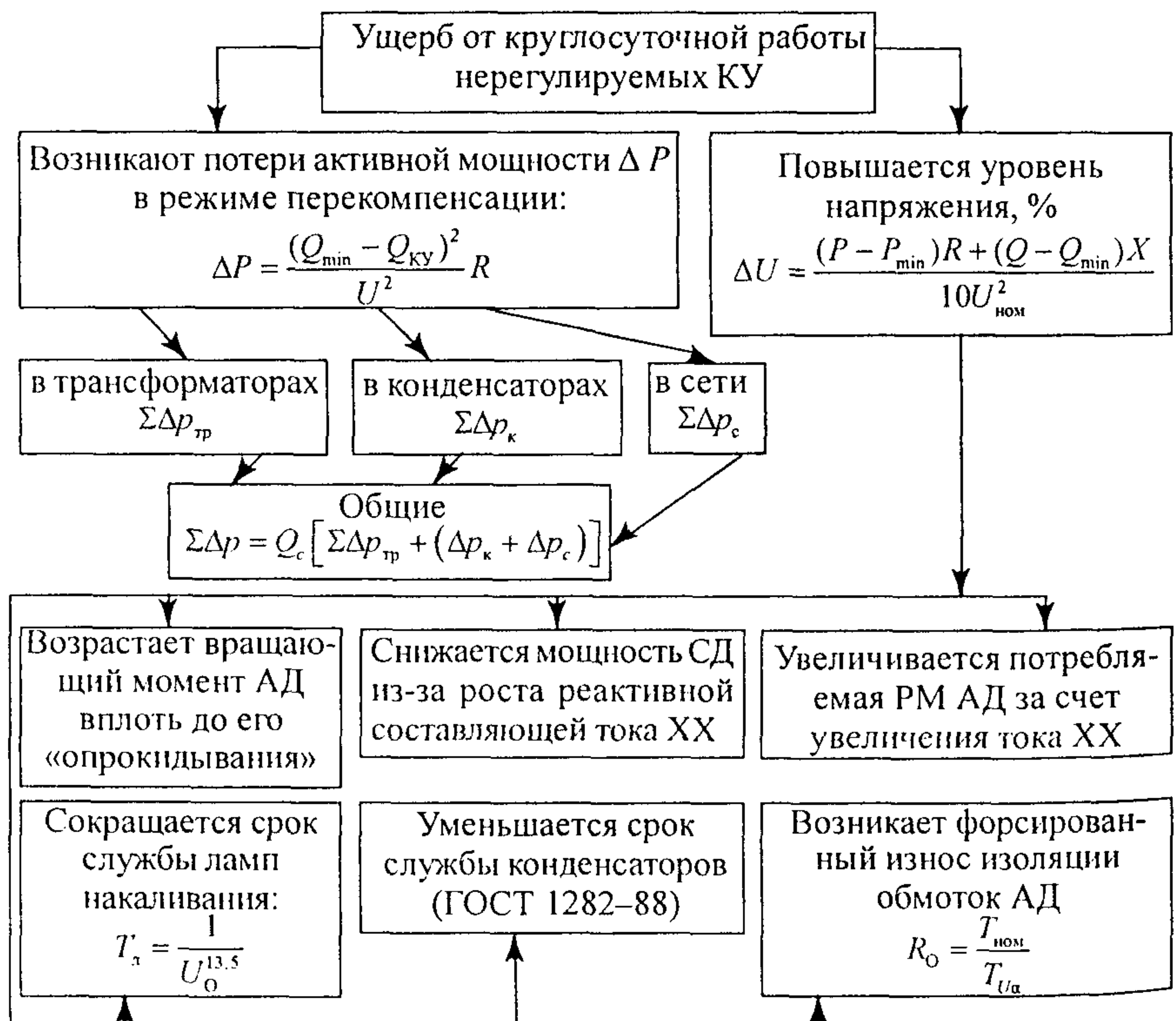
Рис. 6. Составляющие ущерба от круглосуточной работы нерегулируемых КУ
