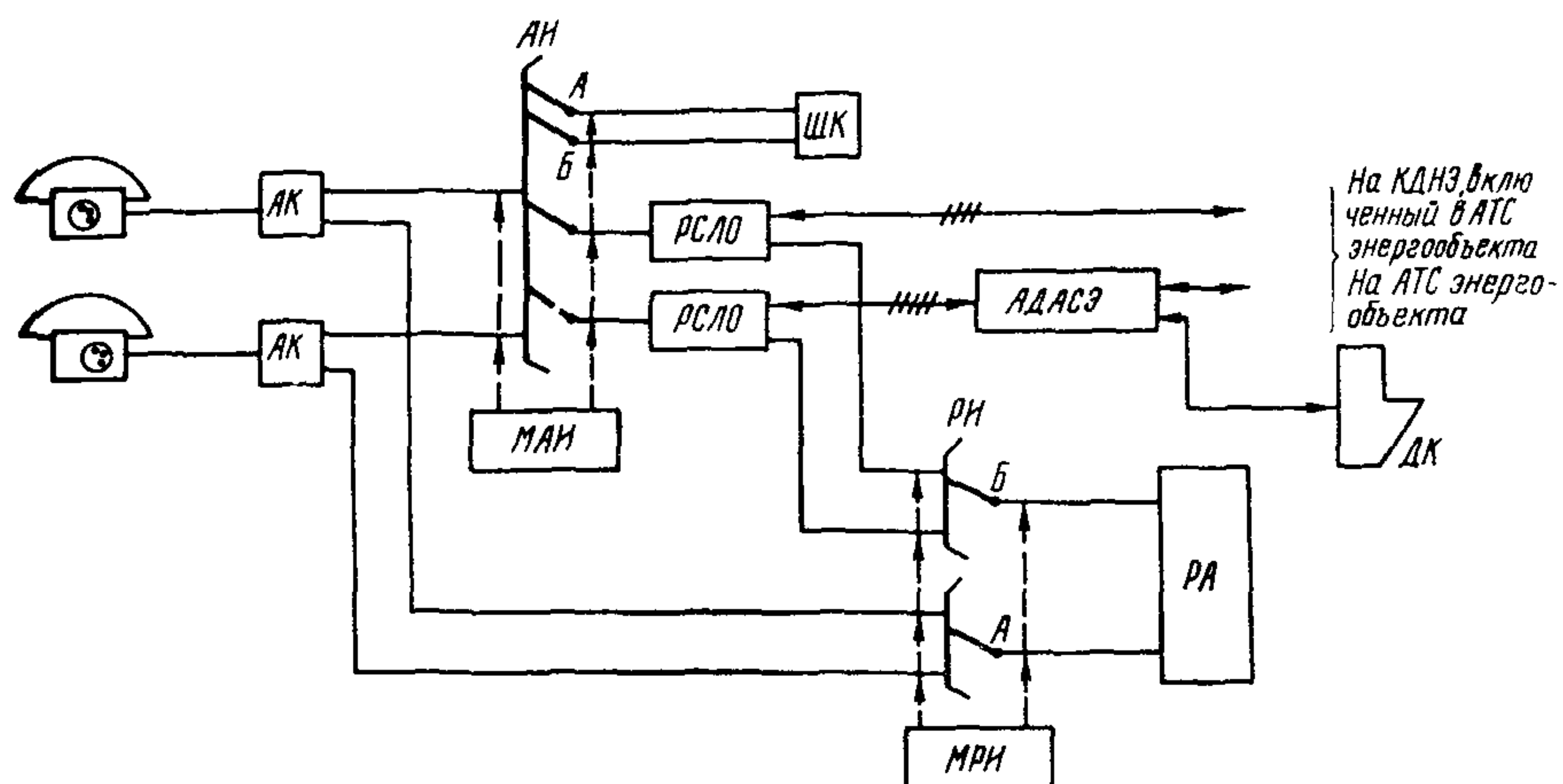
Рис. 7. Структурная схема включения аппаратуры АДАСЭ-50/200 в АТС-50/200-ОС
