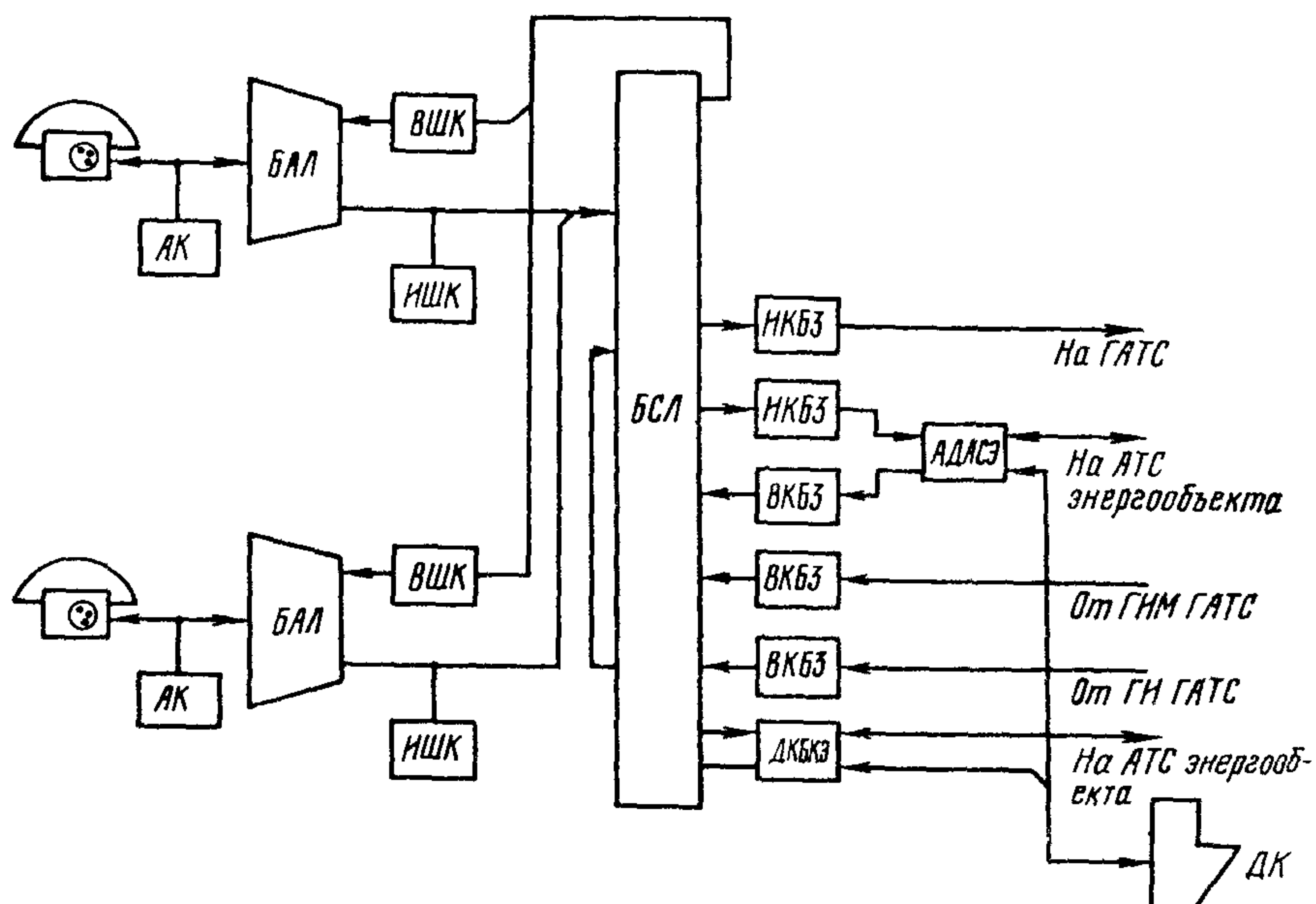
Рис.10. Структурная схема включения аппаратуры АДАСЭ-П(М), АДАСЭ-У в АТС КЭ-ОС
