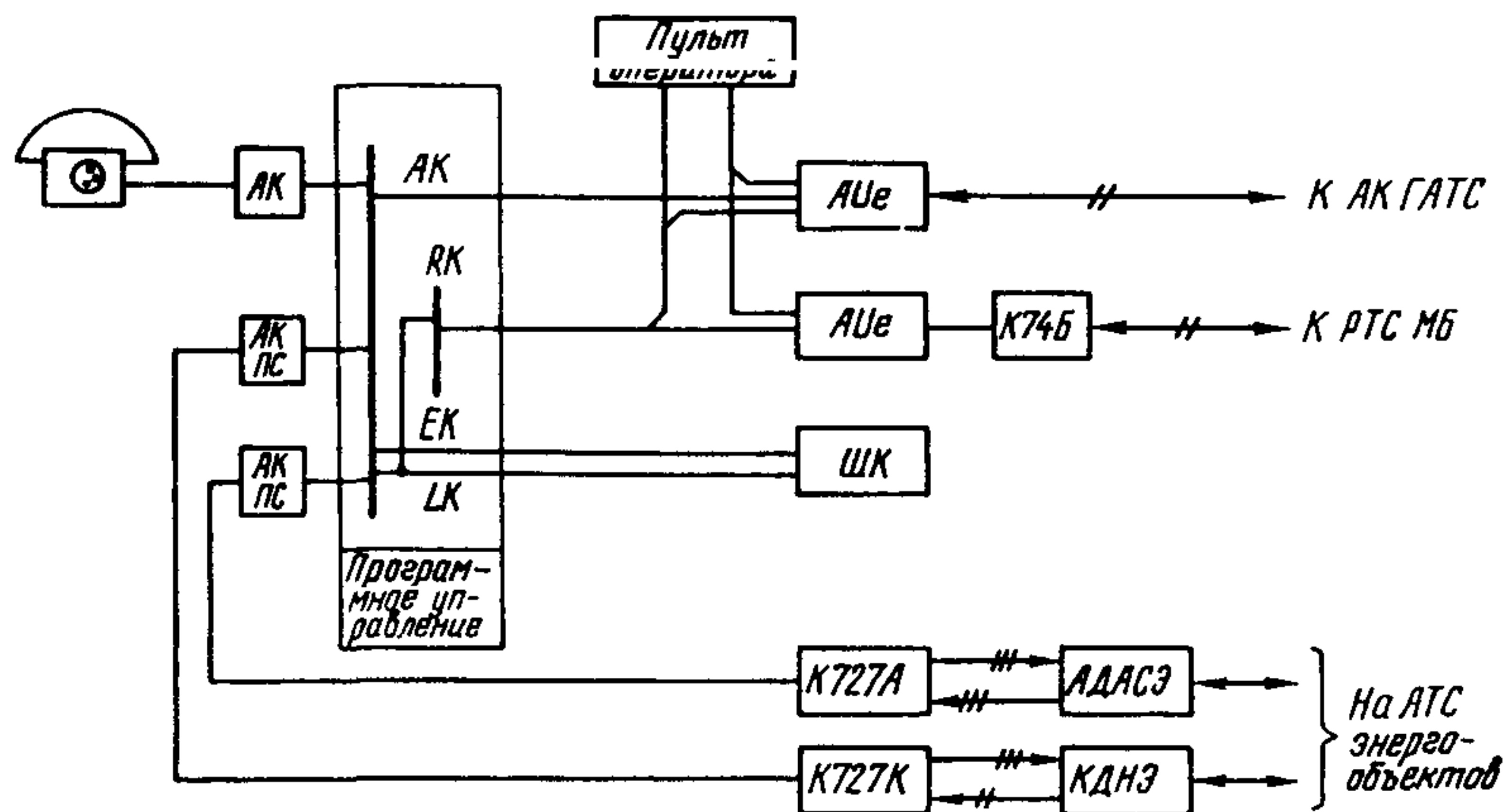
Рис. 4. Структурная схема включения аппаратуры ДАС типов АДАСЭ-П(М), АДАСЭ-У и КДНЭ в ЕСК-400Е емкостью 10-25 номеров
