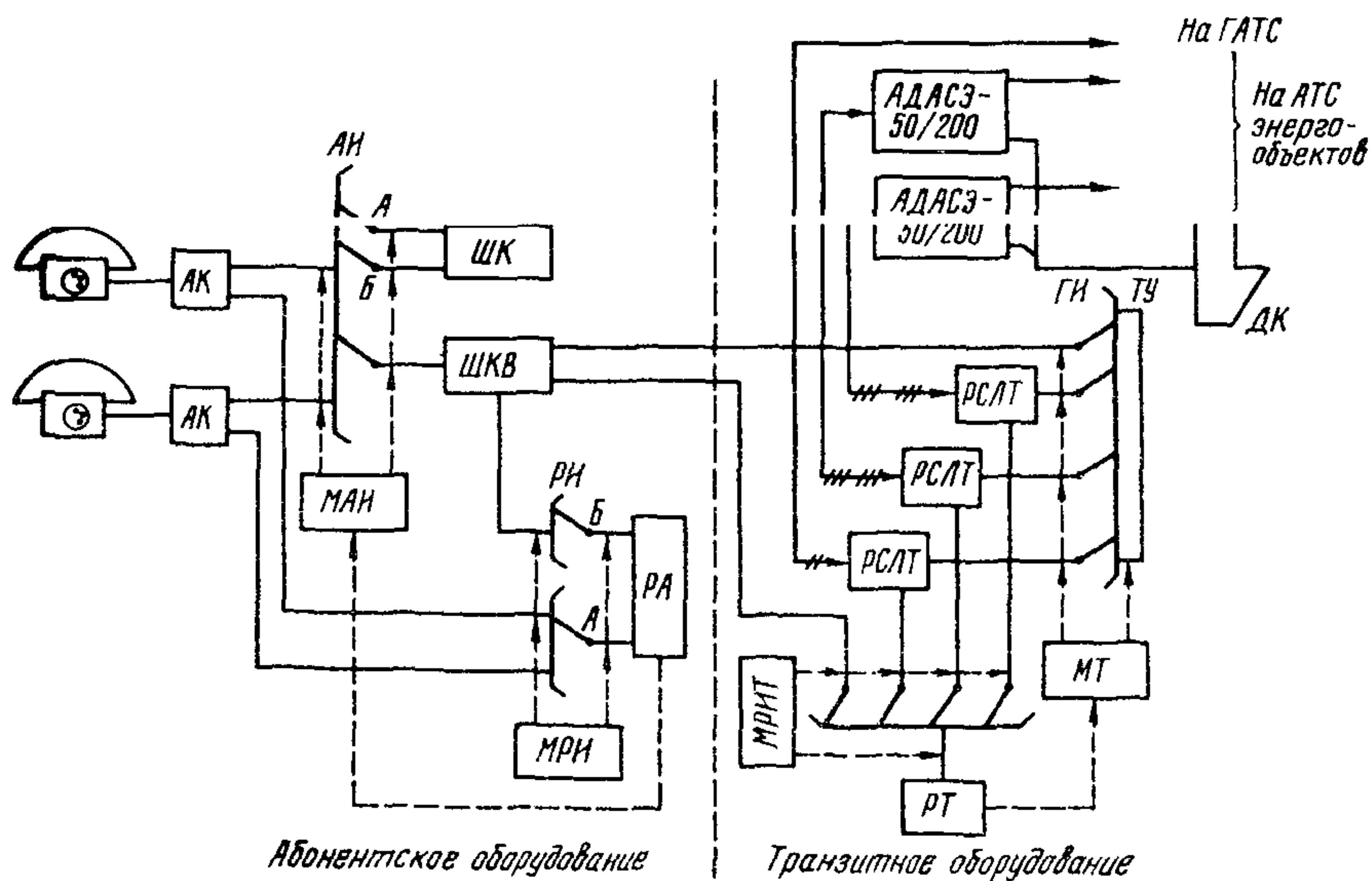
Рис. 8. Структурная схема включения аппаратуры АДАСЭ-50/200 в АТС-50/200-СУ
