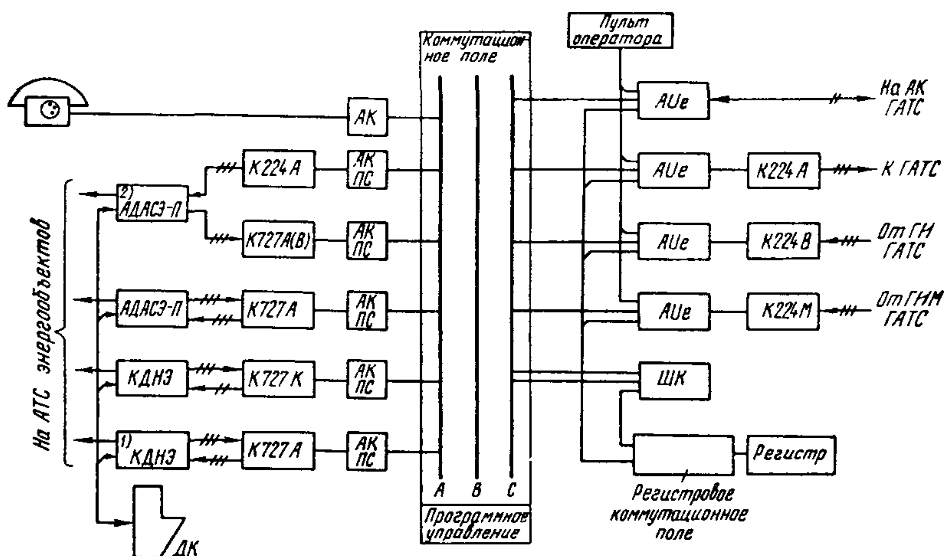
Рис.3. Структурная схема включения аппаратуры ДАС типов АДАСЭ-П(М), АДАСЭ-У и КДНЭ в ЕСК-400Е емкостью 50-400 номеров. Примечания: 1. При соответствующих изменениях в схеме КДНЭ. 2. При необходимости ограничений в выходе на направления внешней связи
