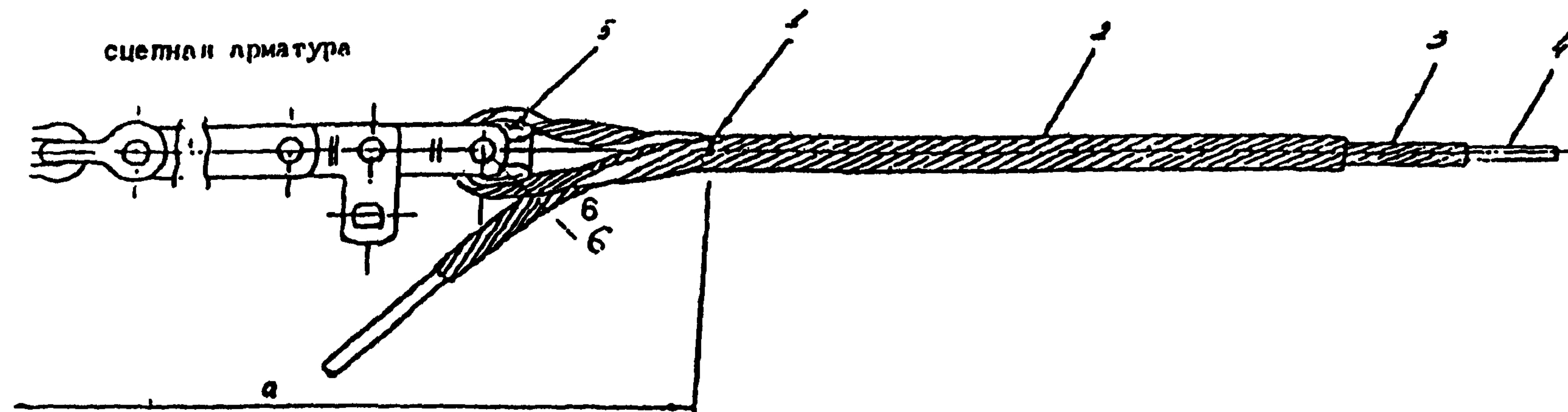
Рис П9 9 Анкерное крепление грозотроса с ОК с помощью натяжного спирального зажима 1-цветная метка на натяжном спиральном зажиме-начало его намотки на грозотрос, 2-натяжной спиральный зажим, 3-прокладка-протектор, 4-грозозащитный трос с ОК, 5-хоуш, 6-шарнир натяжной
