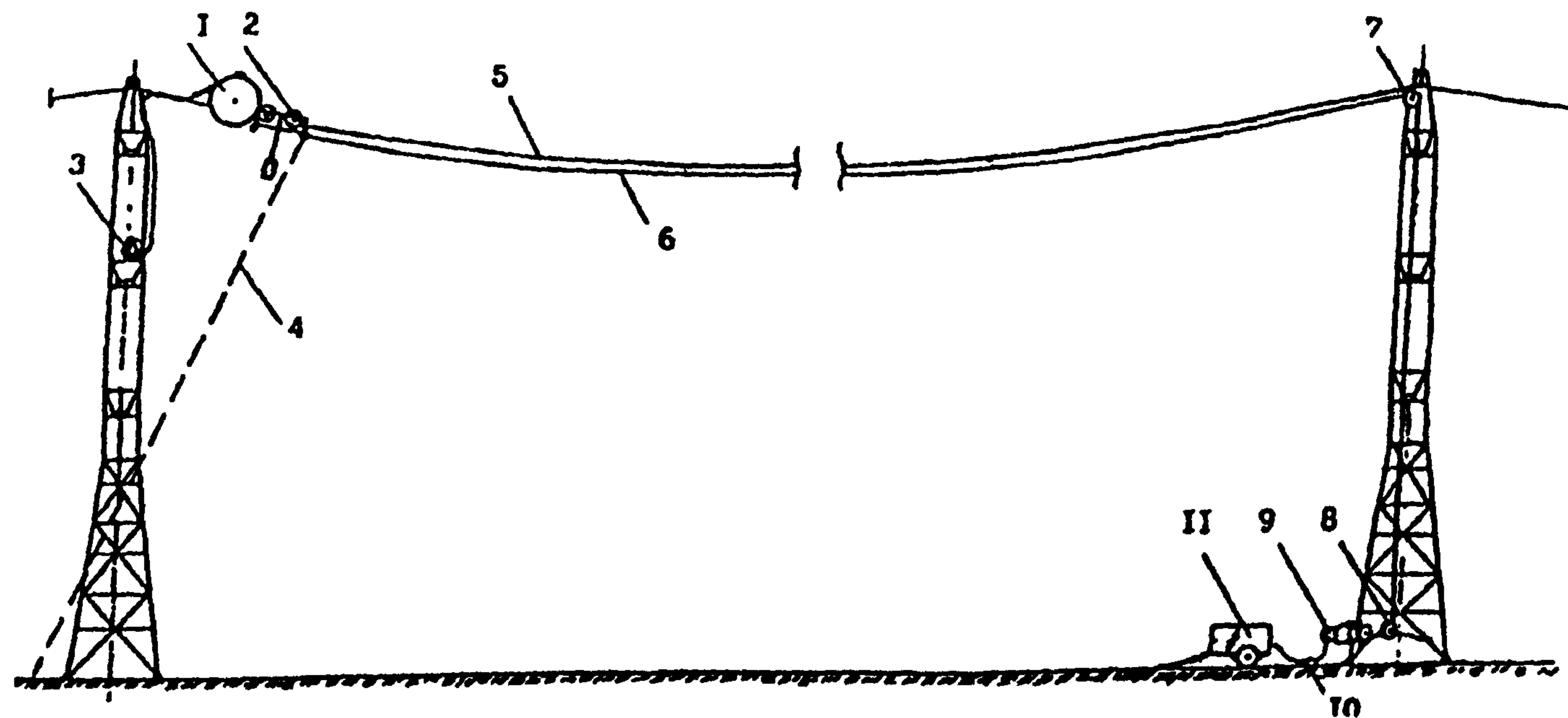
Рис П9 8 Схема расстановки механизмов и приспособлений для навивки ОКНН в пролете ВЛ 1-навивочная машина, 2-стабилизирующая тележка, 3-ОК, смотанный в бухту на граничной опоре 4-тормозной фал, 5-грозотрос, 6-тяговый канат, 7-блок типа МІР-5, 8-отводной блок, 9-электрокабестан, 10-ножной выключатель, 11- источник 3-х фазного тока напряжением 380 В
