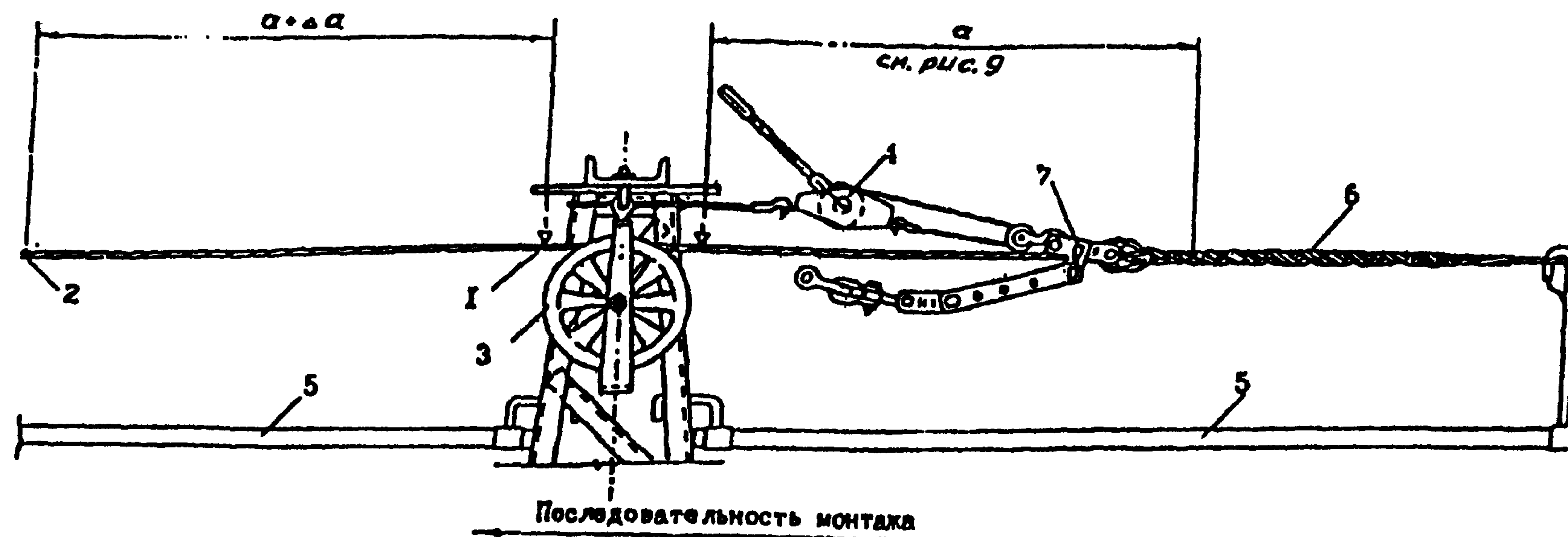
Рис. П9.12. Нанесение меток на ОКГТ и установка спирального натяжного зажима 1-отметка на ОКГТ от узла крепления к опоре, 2-отметка начала намотки натяжного зажима (должна совпадать с цветными метками на протекторе и зажиме), 3-раскаточный ролик, 4-ручная лебедка, 5-монтажный трос, 6-спиральный натяжной зажим, 7-монтажное звено а-длина ОКГТ, необходимая для образования петли грозотроса вокруг тросостойки-
