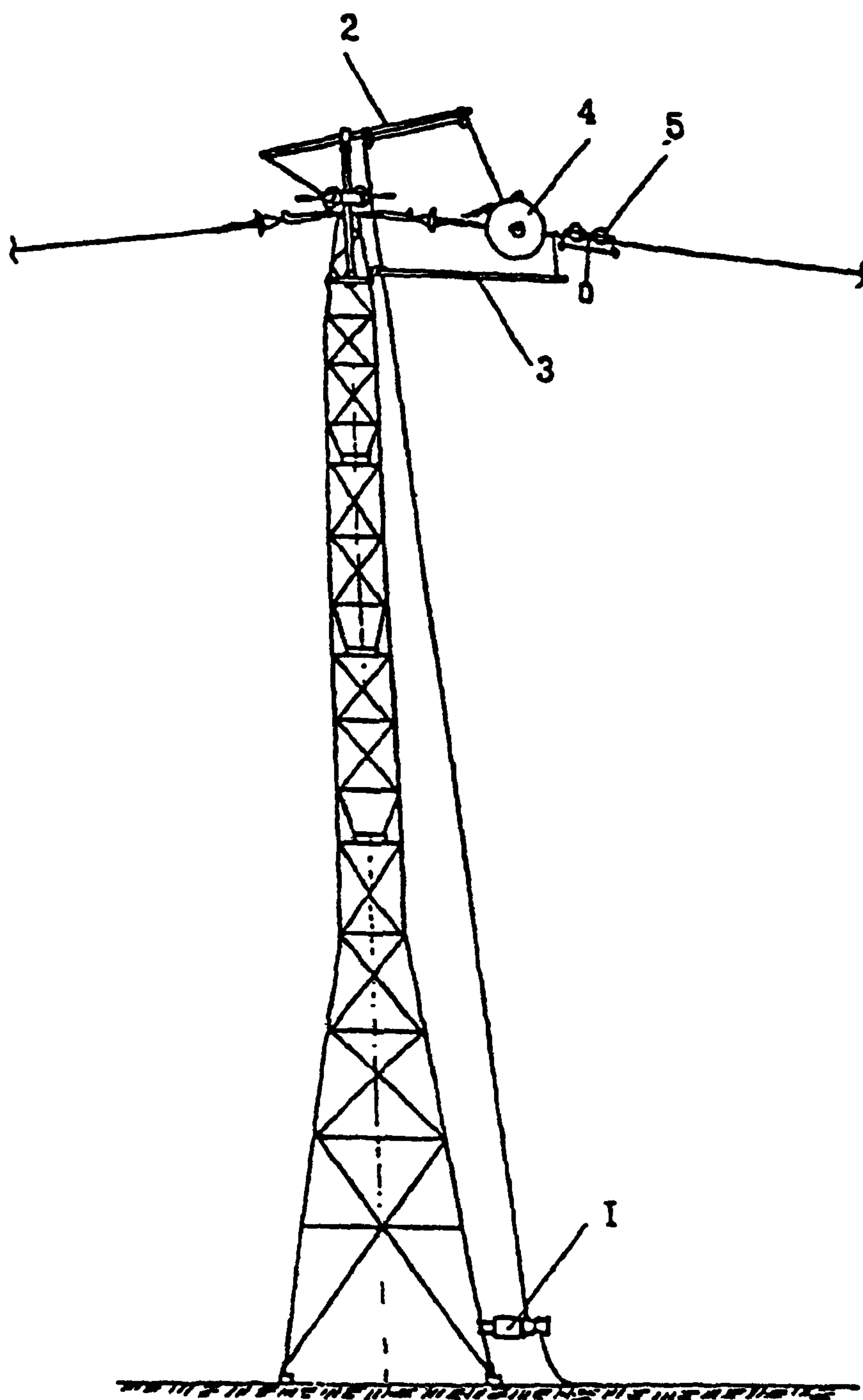
Рис. П9.7. Схема расстановки механизмов и приспособлений на опоре для навивки ОКНН
